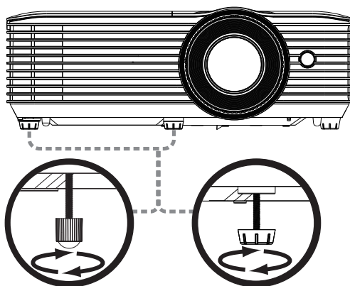
Rotella di regolazione dell'inclinazione
