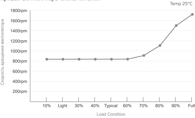
Кривая вентилятора блока питания
