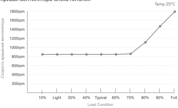
Кривая вентилятора блока питания
