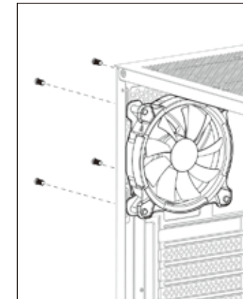
(6d) Install Rear Fan
