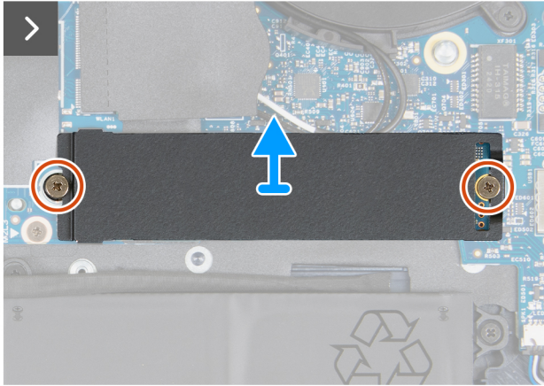
Figura 27. Rimozione dell'unità SSD M.2 2280 dallo slot SSD1
