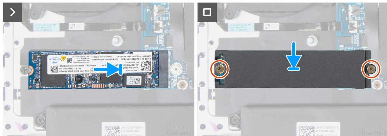
Figura 30. Installazione dell'unità SSD M.2 2280 nello slot SSD2
