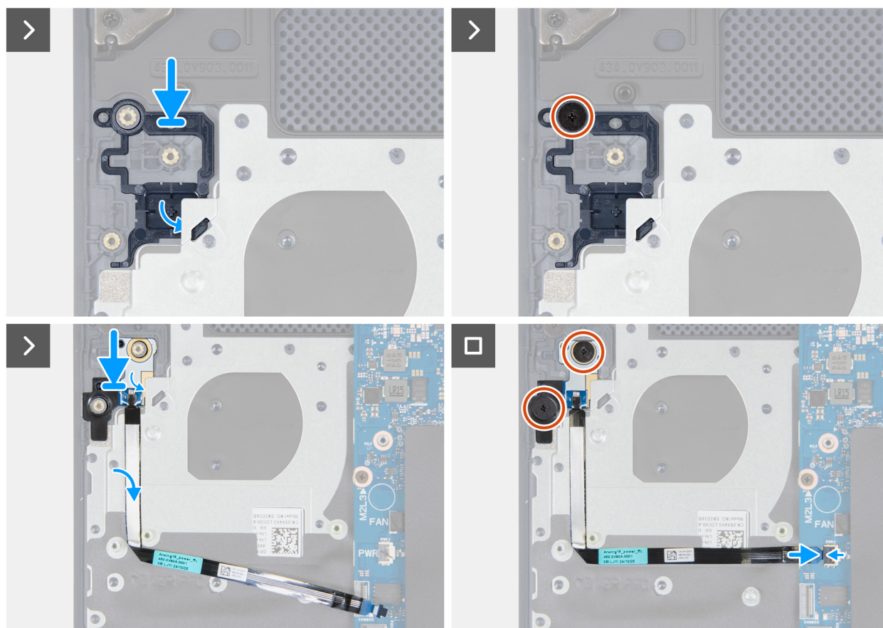
Figura 59. Installazione del pulsante di accensione e della relativa scheda
