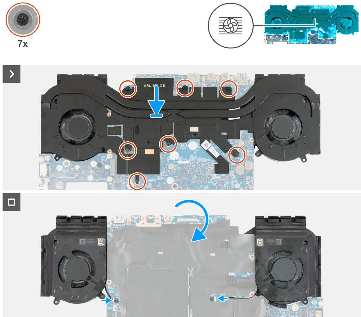
Figura 61. Installazione del gruppo ventola e dissipatore di calore
