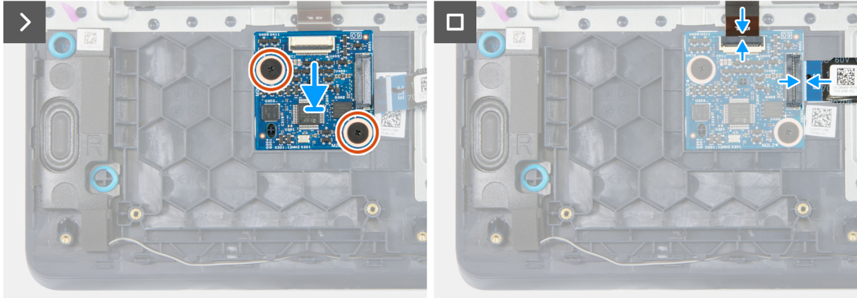
Figura 46. Installazione della scheda del controller di retroilluminazione della tastiera (ELC)
