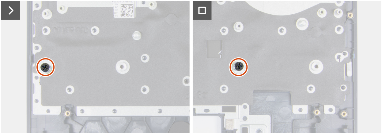
Figura 77. Rimozione dei supporti per viti dell'unità SSD
