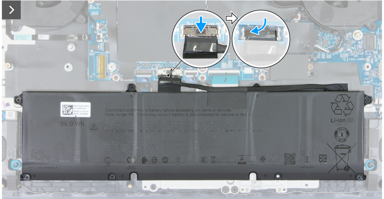
Figura 14. Collegamento del cavo della batteria
