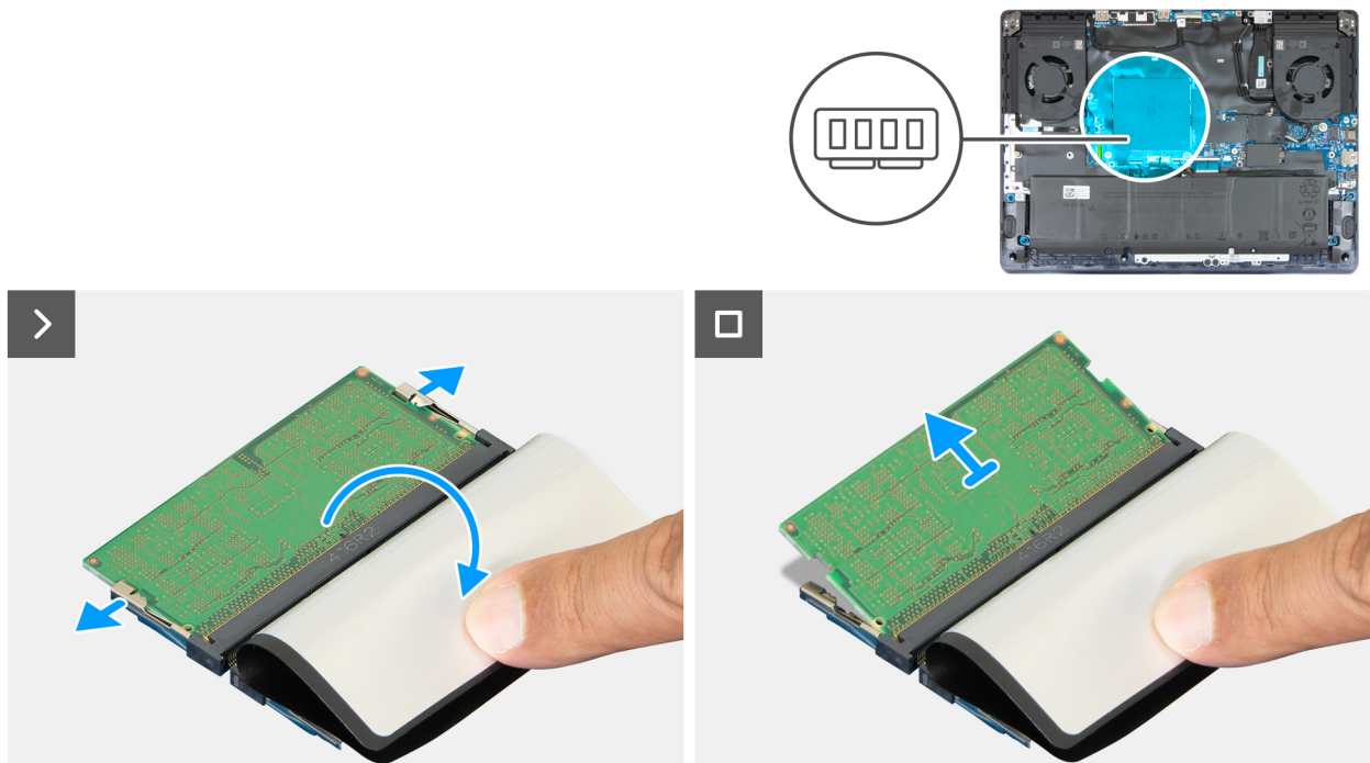
Figura 21. Rimozione del modulo di memoria
