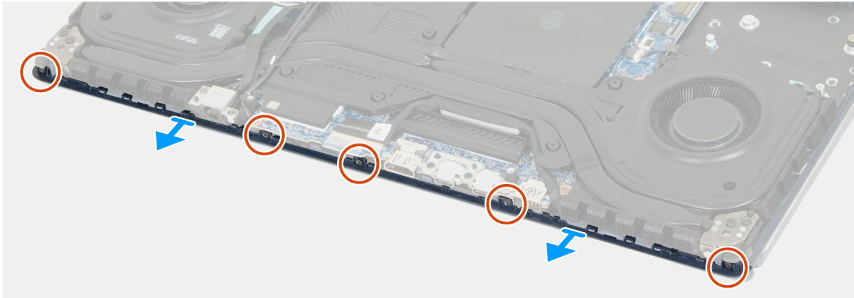
Figura 64. Rimozione del pannello posteriore
