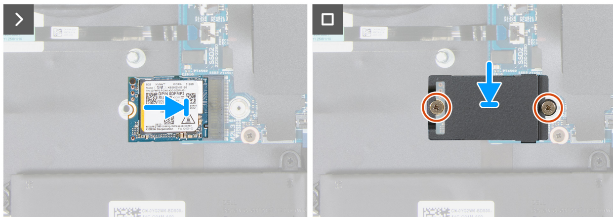
Figura 26. Installazione dell'unità SSD M.2 2230 nello slot SSD2
