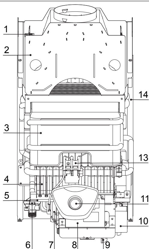
Vista complessiva - schema idraulico
