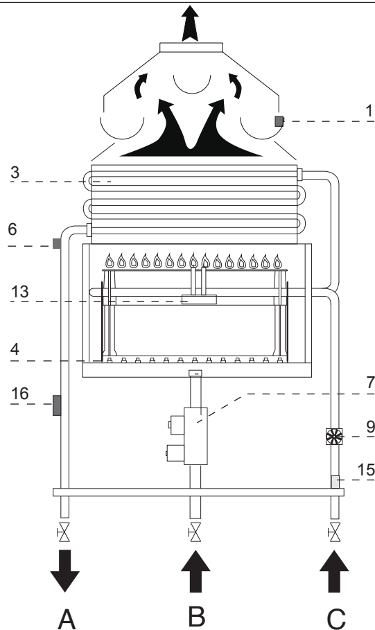
Vedere de Ansamblu - Schema hidraulică
