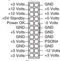
C ATX_PWR
