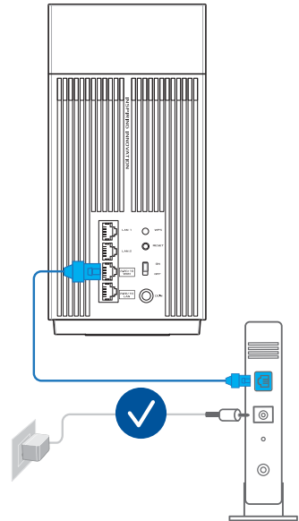
Achterkant modem
