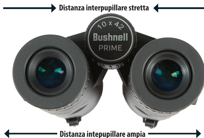
Fig. 3 Regolazione della distanza interpupillare
