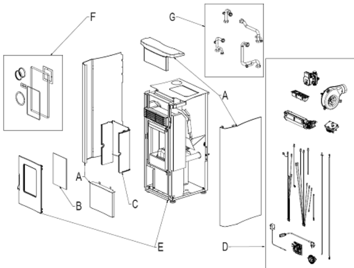
Fig. 1 - Esploso
