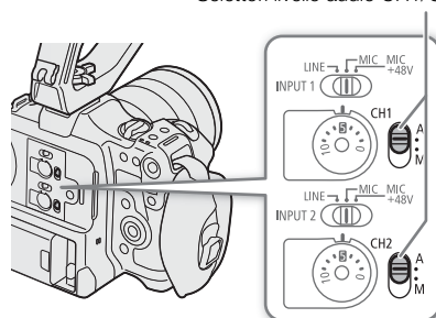
Selettori livello audio CH1/CH2
