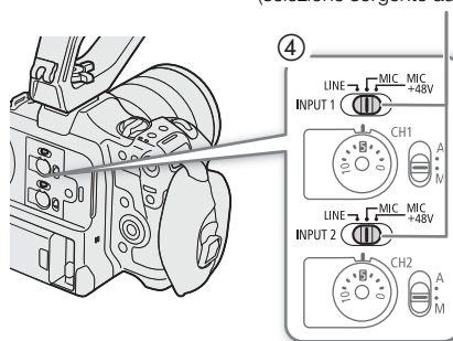
Selettori INPUT 1 / INPUT 2 (selezione sorgente audio)
