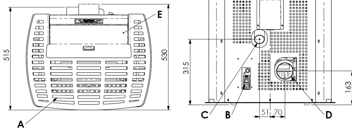
Medidas de la estufa de pellets AURORA
