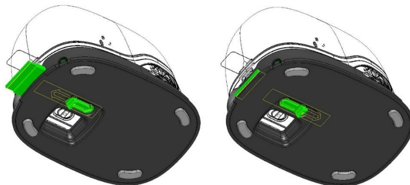
Imm. 19: Estrazione del tergicristallo della testina di stampa
