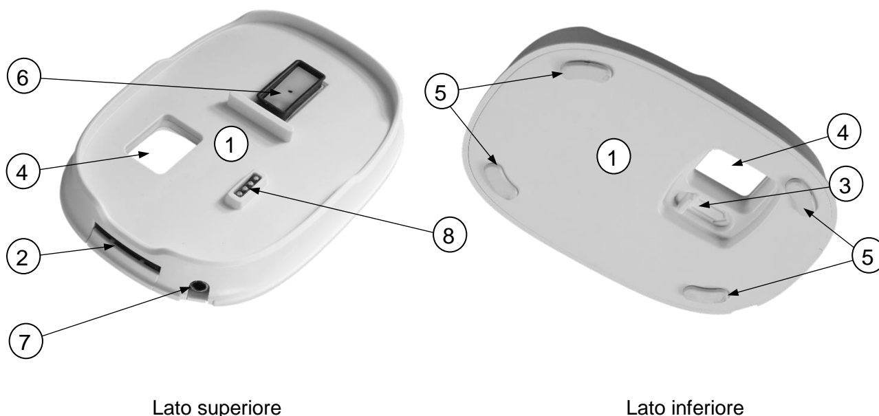
Imm. 5: Struttura della docking station
