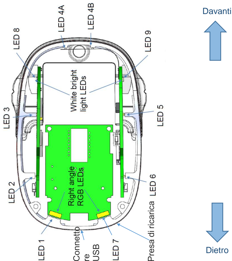
Imm. 16: Indicazioni della direzione light guide
