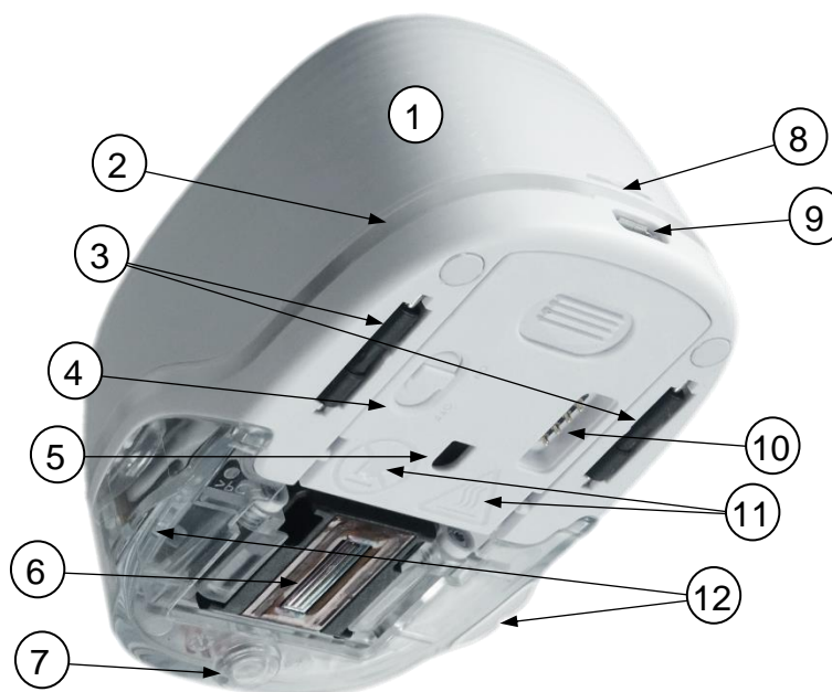
Imm. 4: Struttura del dispositivo di marcatura
