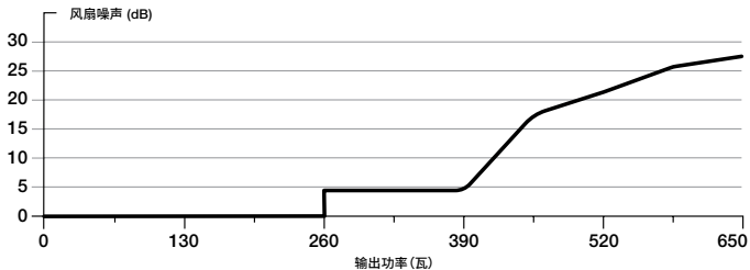
CORSAIR RM650x 电源风扇噪音曲线
