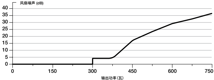
CORSAIR RM750x 电源风扇噪音曲线
