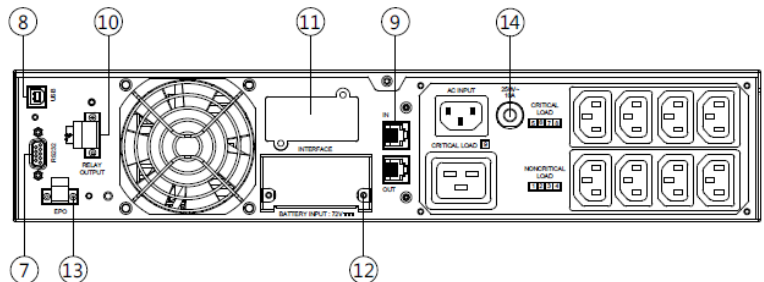
OL2000ERTXL2U
