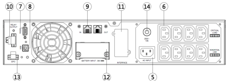
OL1000ERTXL2U / OL1500ERTXL2U
