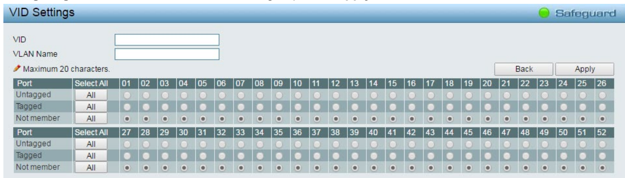
Figure 4.49 – Configuration > 802.1Q VLAN > Add VID
