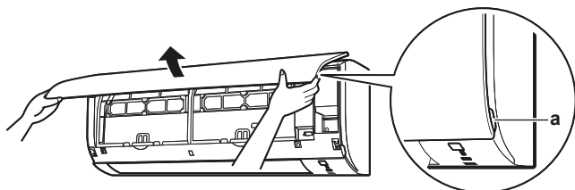
a Blendenlaschen
