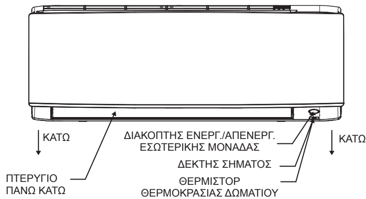
ΜΠΡΟΣΤΙΝΗ ΑΠΟΨΗ
