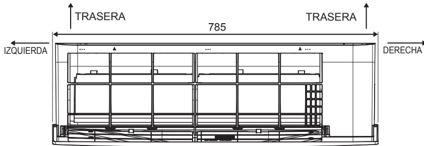
VISTA SUPERIOR
