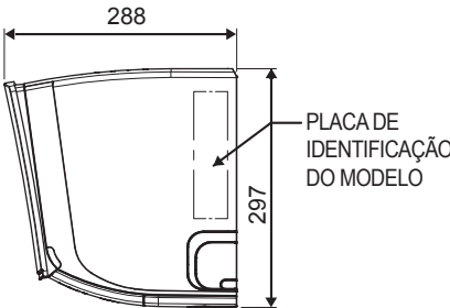
VISTA LATERAL
