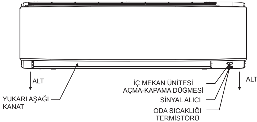
ÖN GÖRÜNÜM
