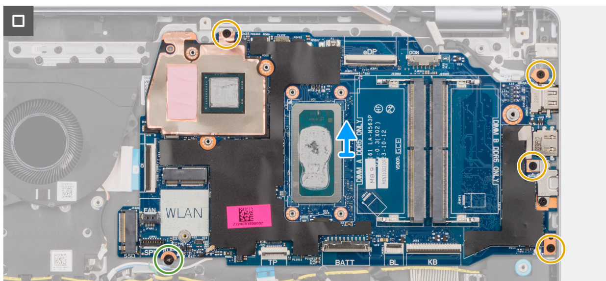
Figura 82. Rimozione della scheda di sistema
