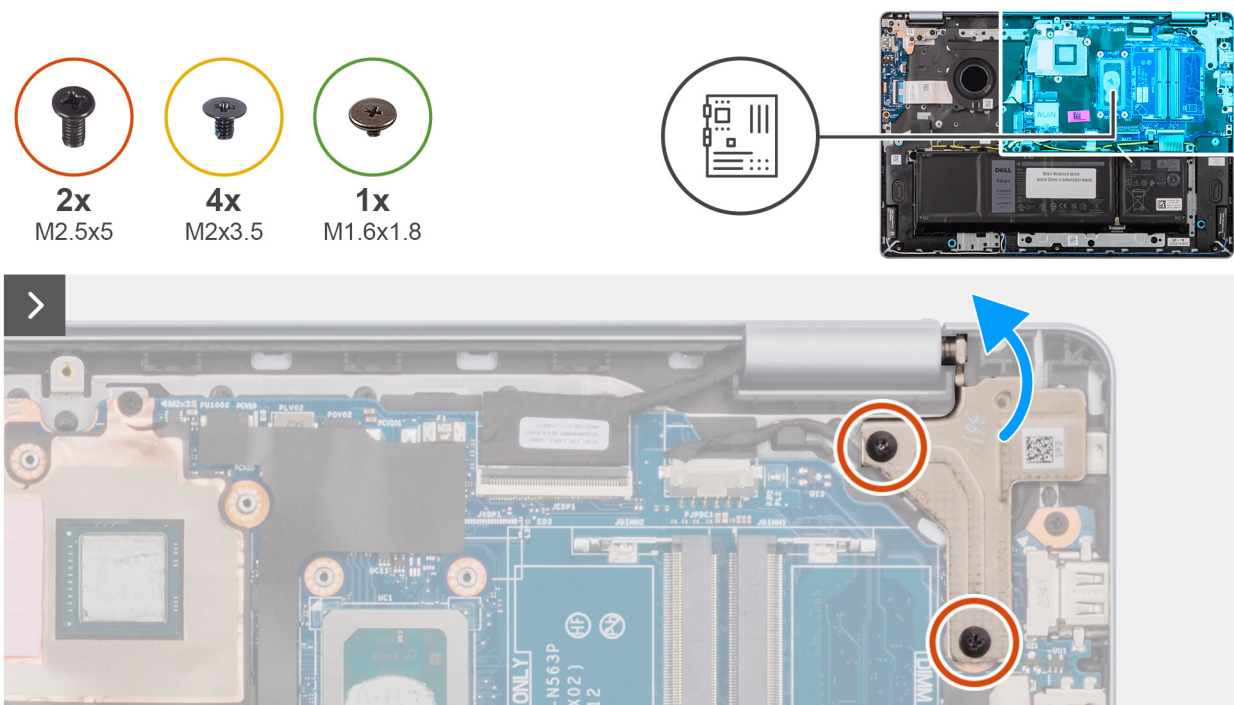
Figura 80. Rimozione della scheda di sistema
