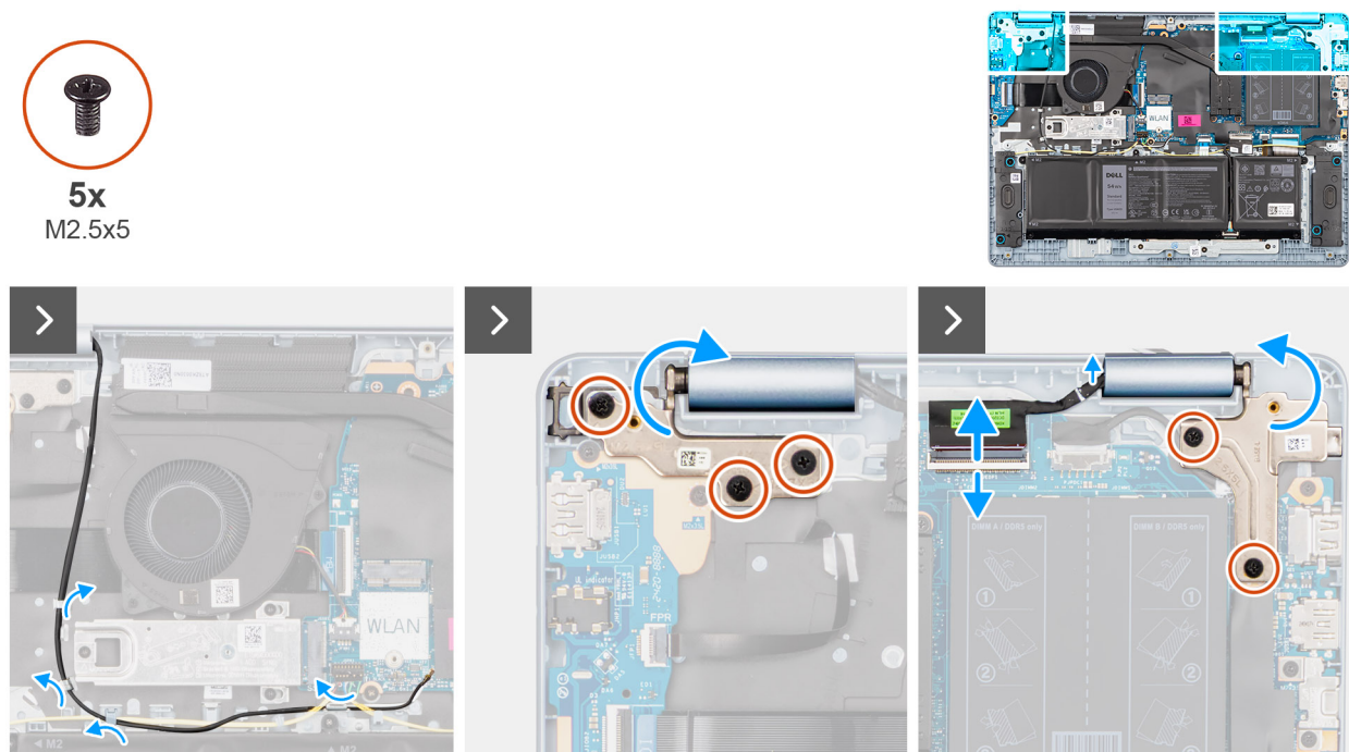
Figura 50. Rimozione del gruppo del display
