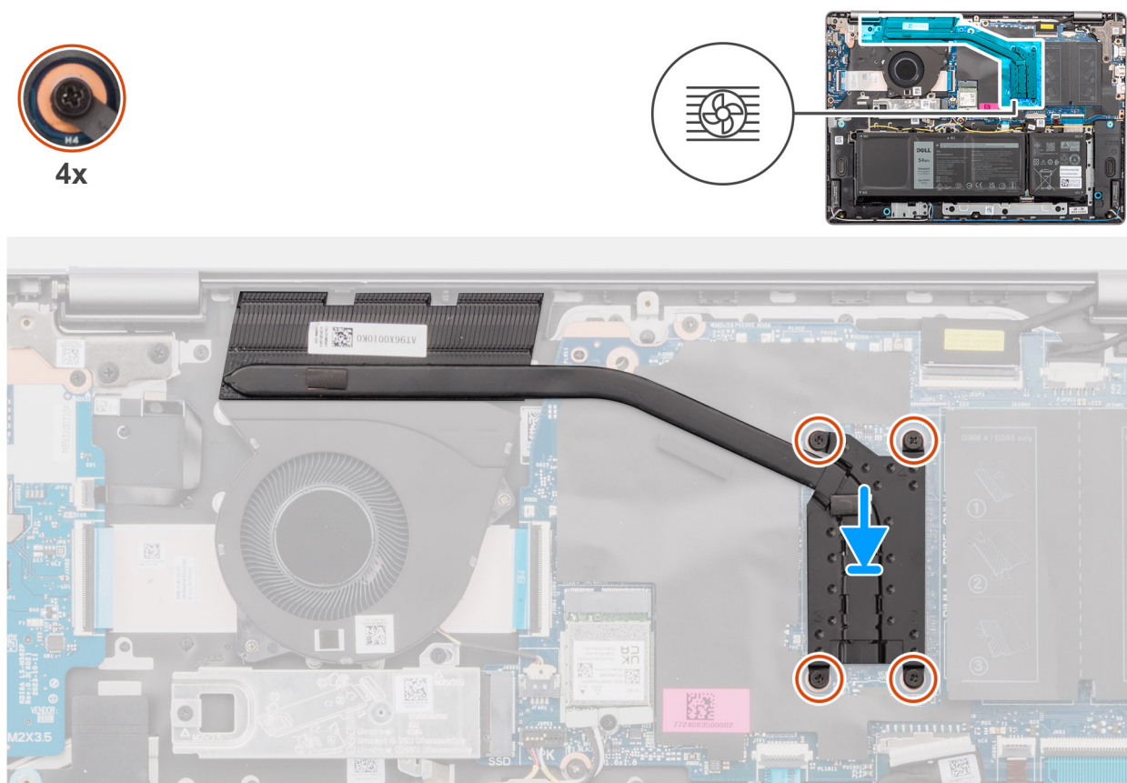
Figura 41. Installazione del dissipatore di calore - per computer forniti con scheda grafica integrata
