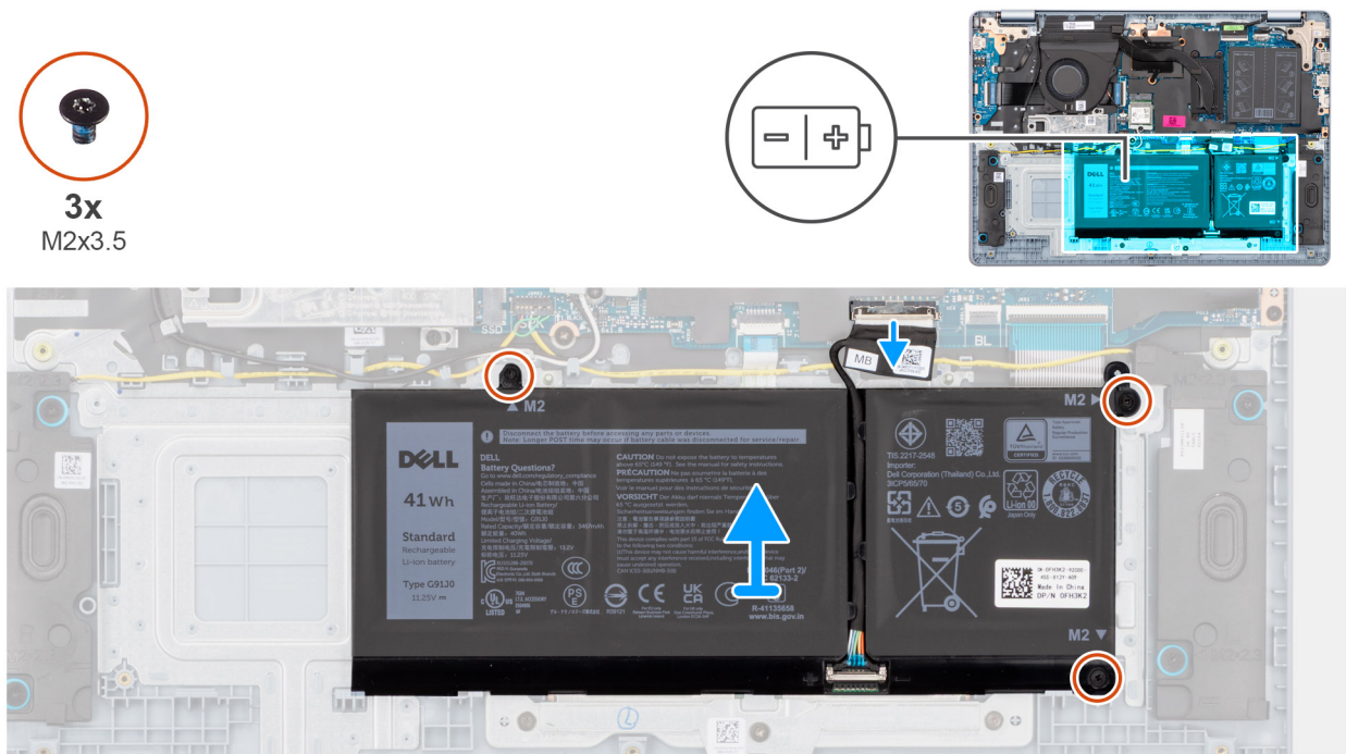
Figura 16. Rimozione della batteria a 3 celle
