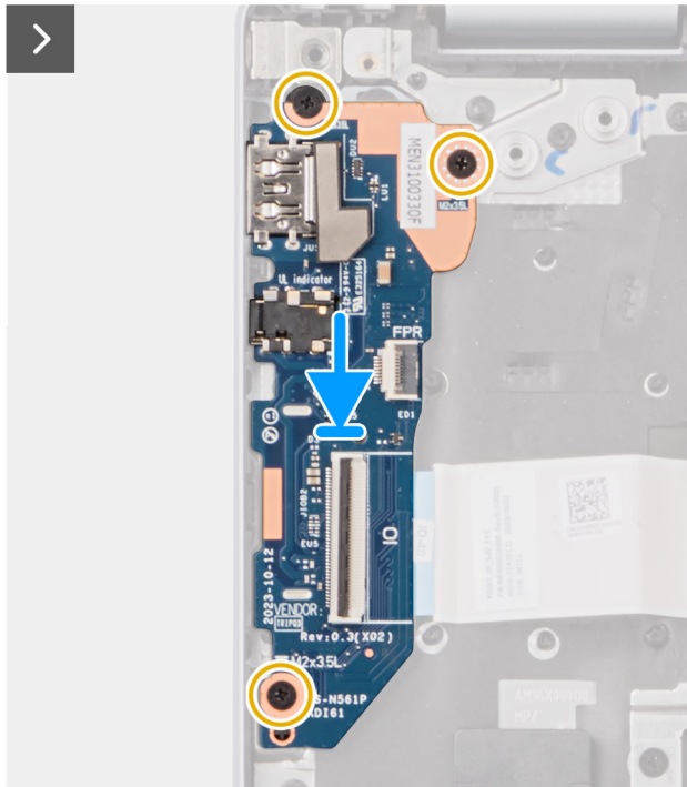
Figura 49. Installazione della scheda di I/O
