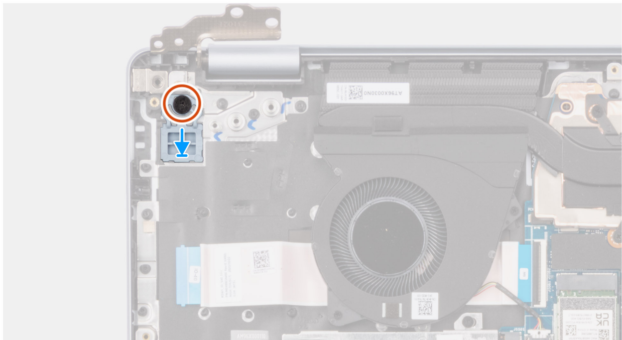
Figura 73. Installazione del pulsante di accensione
