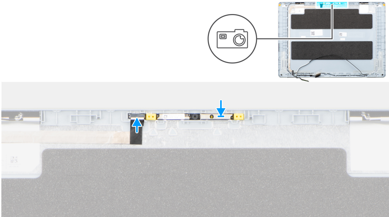
Figura 69. Installazione della fotocamera
