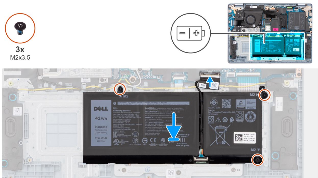
Figura 17. Installazione della batteria a 3 celle
