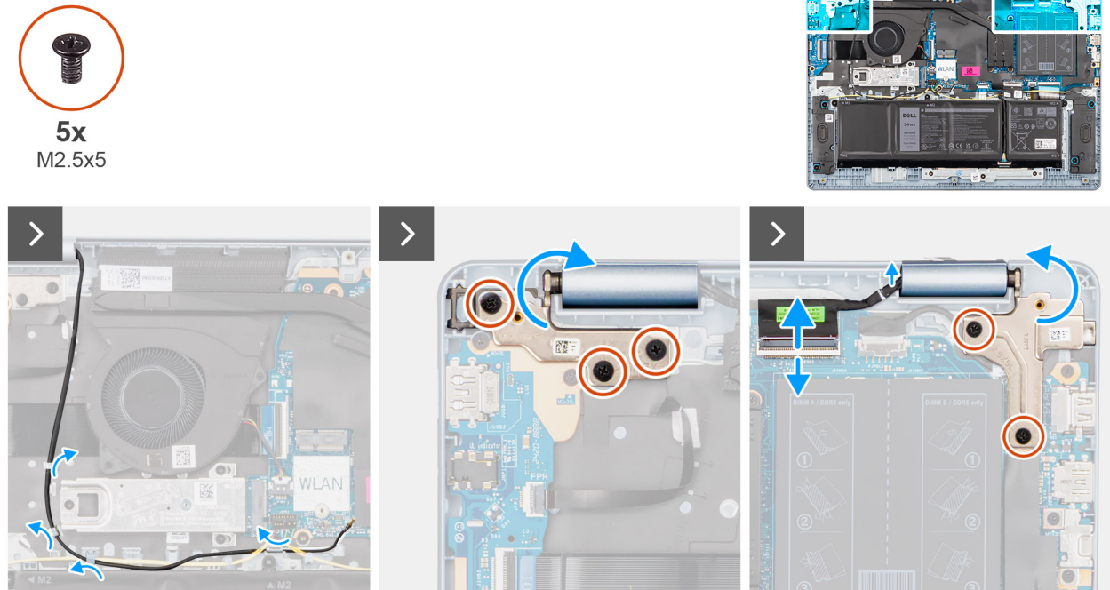
Figura 50. Rimozione del gruppo del display
