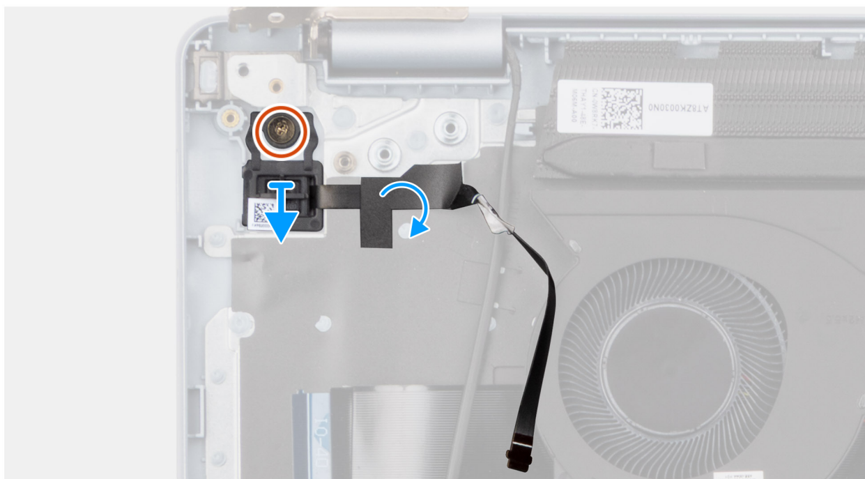
Figura 74. Rimozione del pulsante di accensione con lettore di impronte digitali
