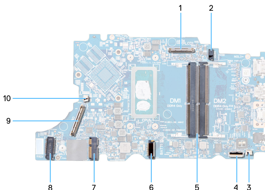
Figura 2. Connettori della scheda di sistema - parte anteriore
