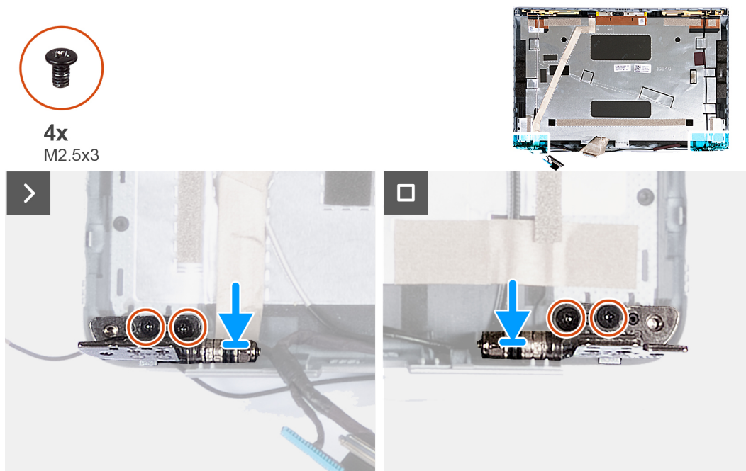
Figura 48. Installazione dei cardini del display
