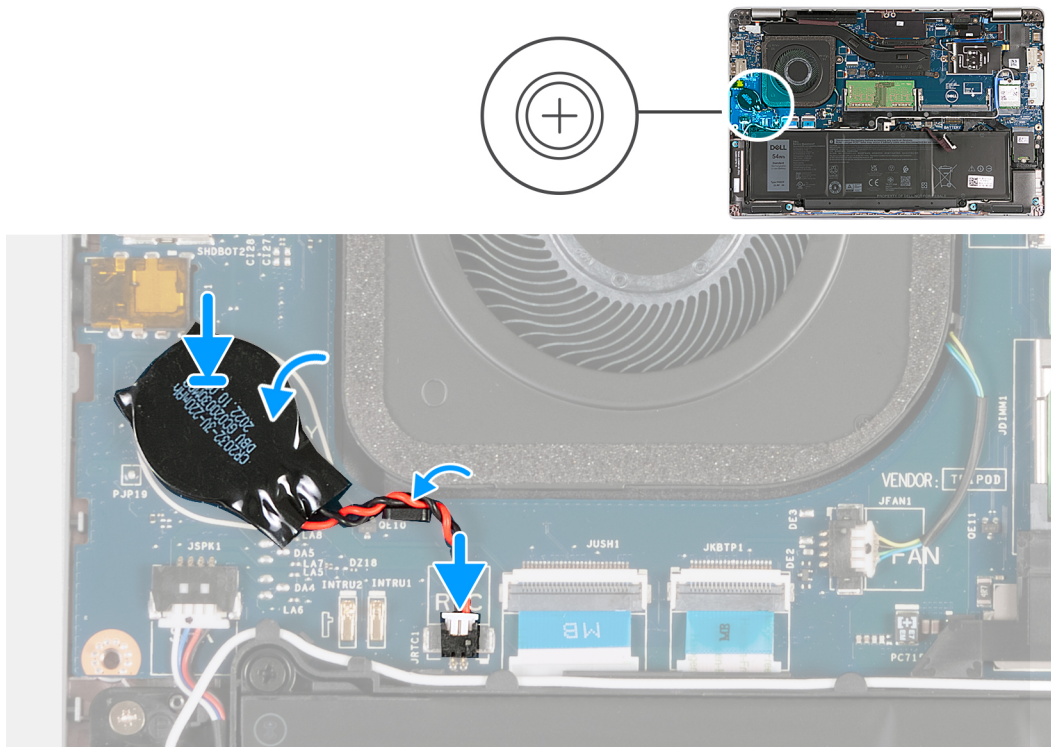
Figura 21. Installazione della batteria a bottone
