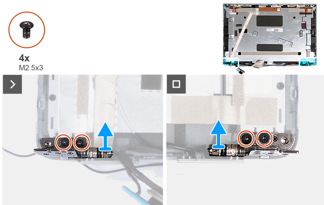
Figura 47. Rimozione dei cardini del display
