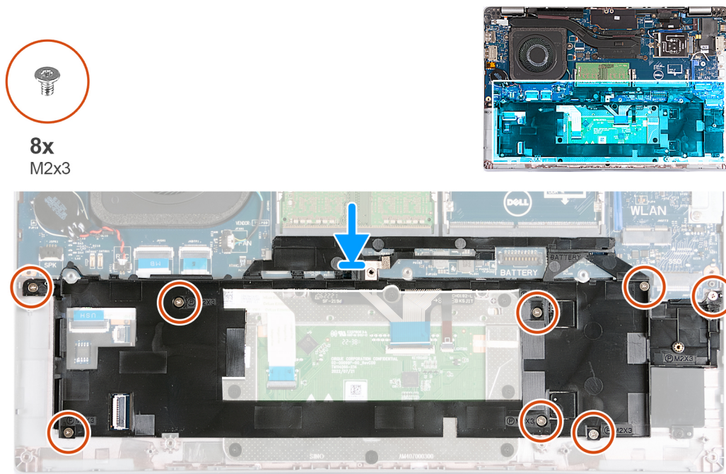
Figura 32. Installazione dell'intelaiatura interna del gruppo
