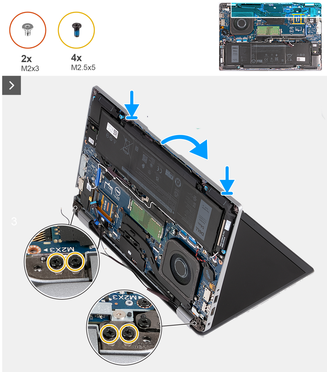
Figura 39. Installazione del gruppo del display - Per i computer forniti con scheda 5G
