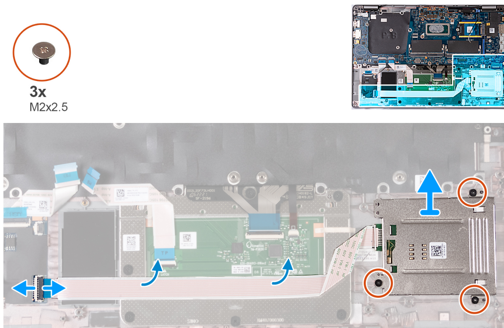
Figura 57. Rimozione del lettore di smart card
