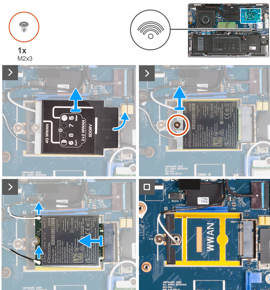
Figura 12. Rimozione della scheda WWAN - Per computer forniti con scheda 4G
