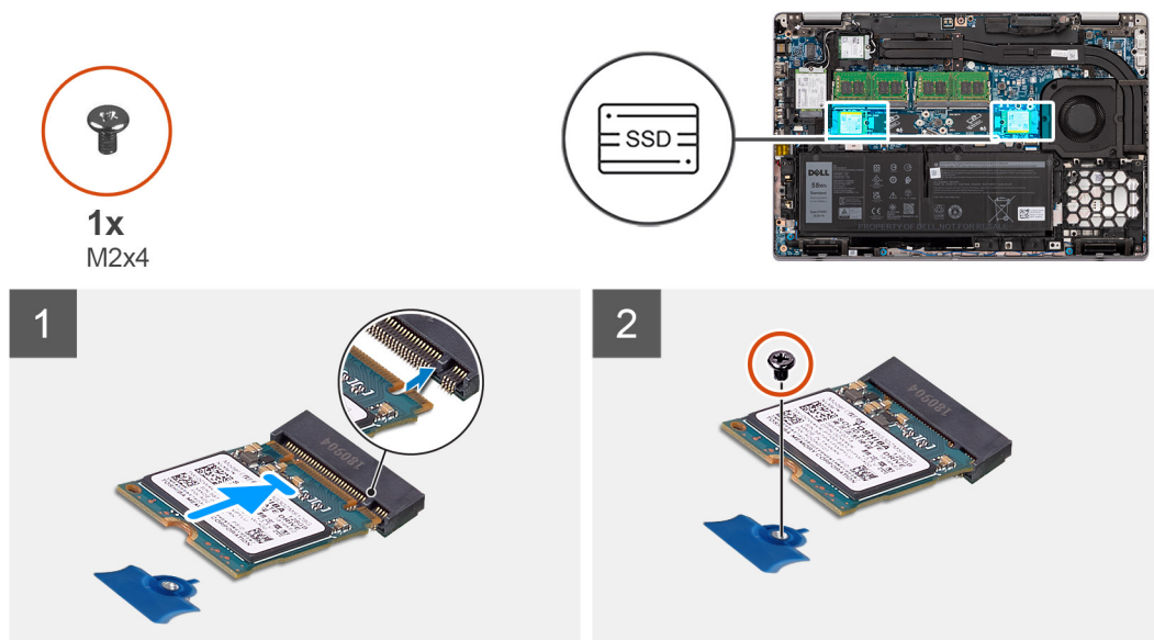
Figura 7. Unità SSD M.2 2230 senza staffa
