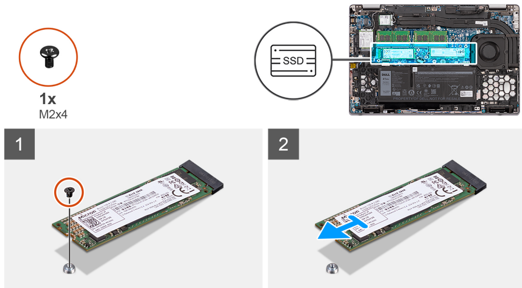
Figura 1. Unità SSD M.2 2280 senza staffa
