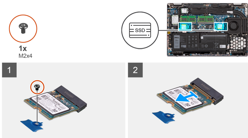
Figura 5. Unità SSD M.2 2230 senza staffa
