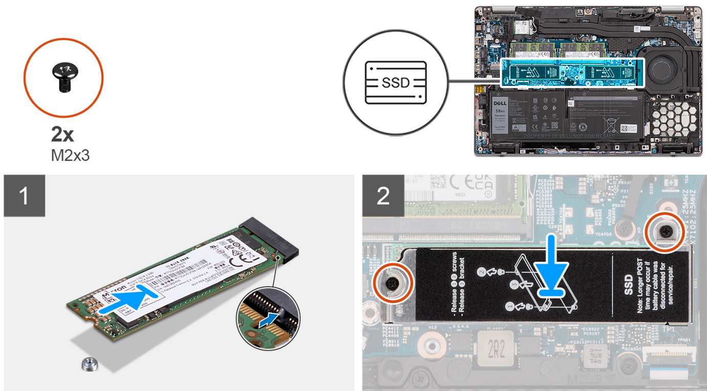
Figura 4. Unità SSD M.2 2280 con relativa staffa
