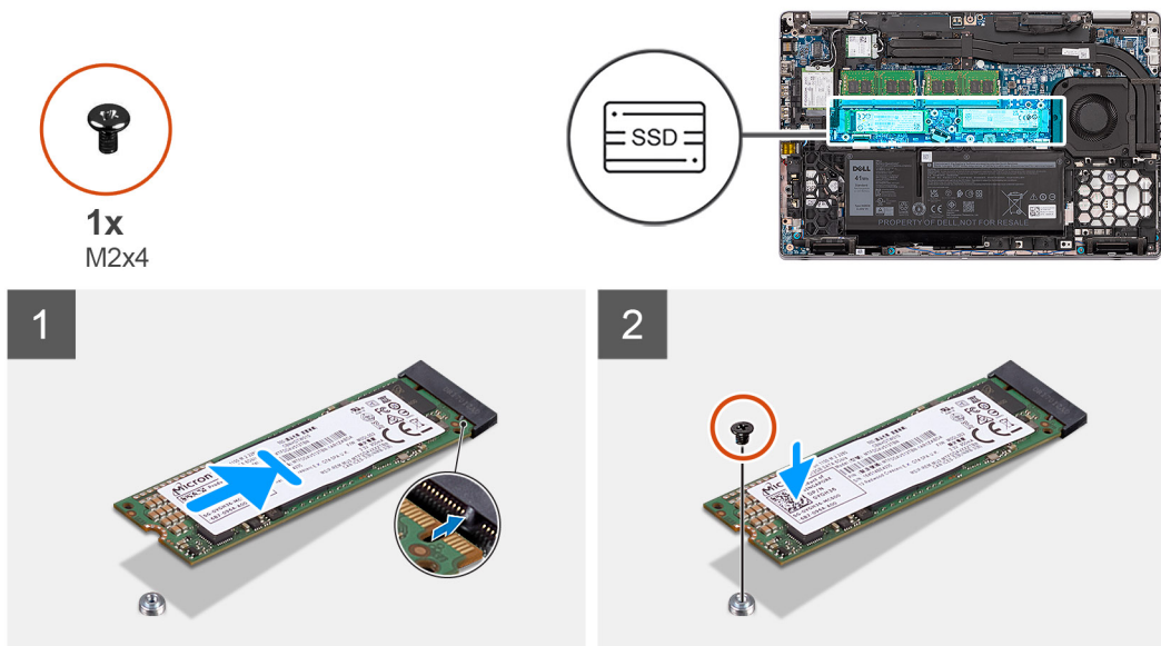
Figura 3. Unità SSD M.2 2280 senza staffa
