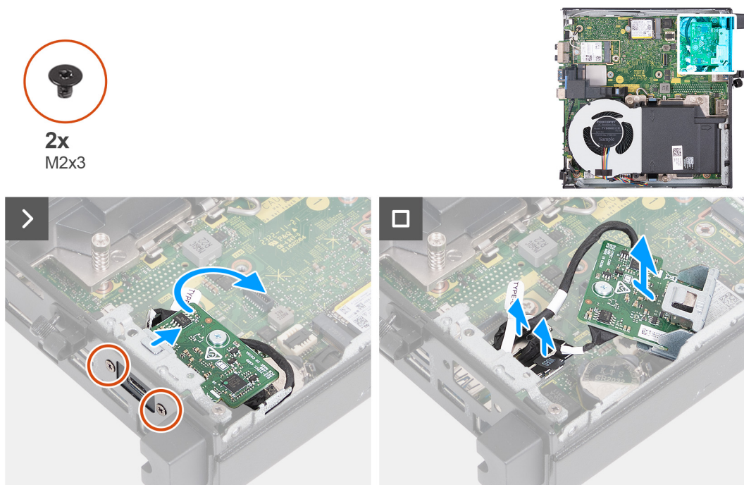
Figura 38. Rimozione del modulo Type-C opzionale
