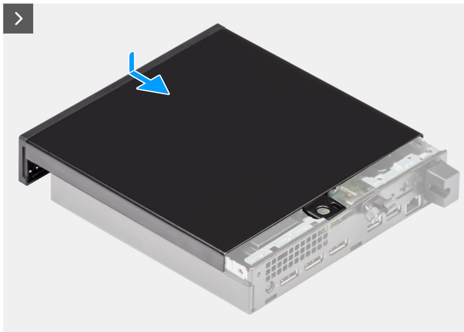
Figura 11. Installazione del coperchio laterale
