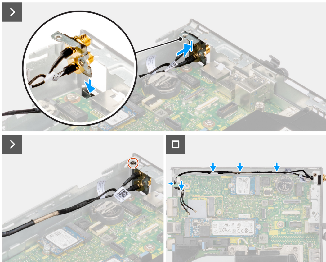
Figura 55. Installazione dell'antenna SMA (posizione 3)
