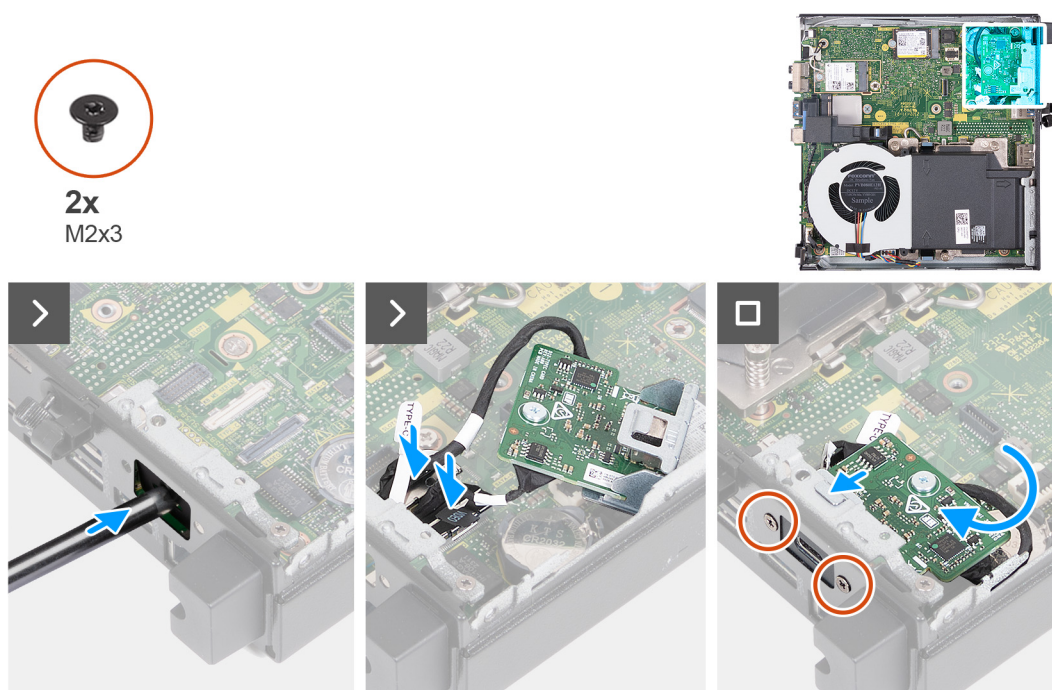
Figura 39. Installazione del modulo Type-C opzionale
