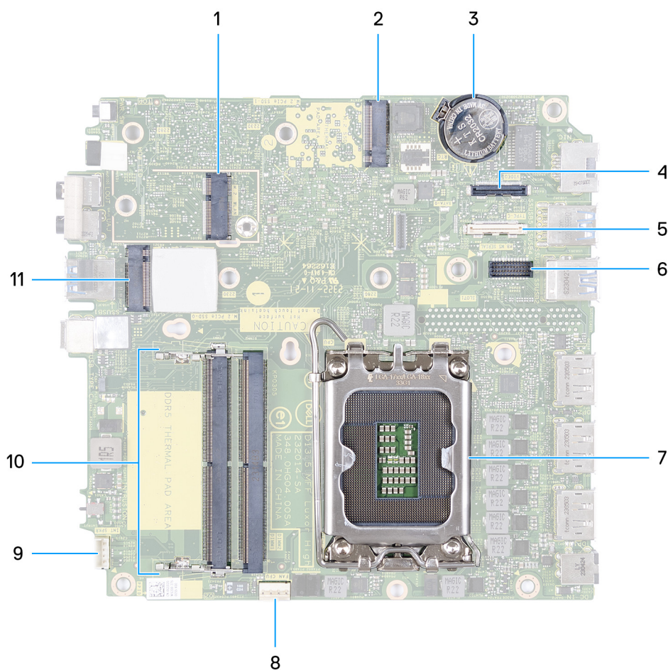
Figura 44. Connettori della scheda di sistema
