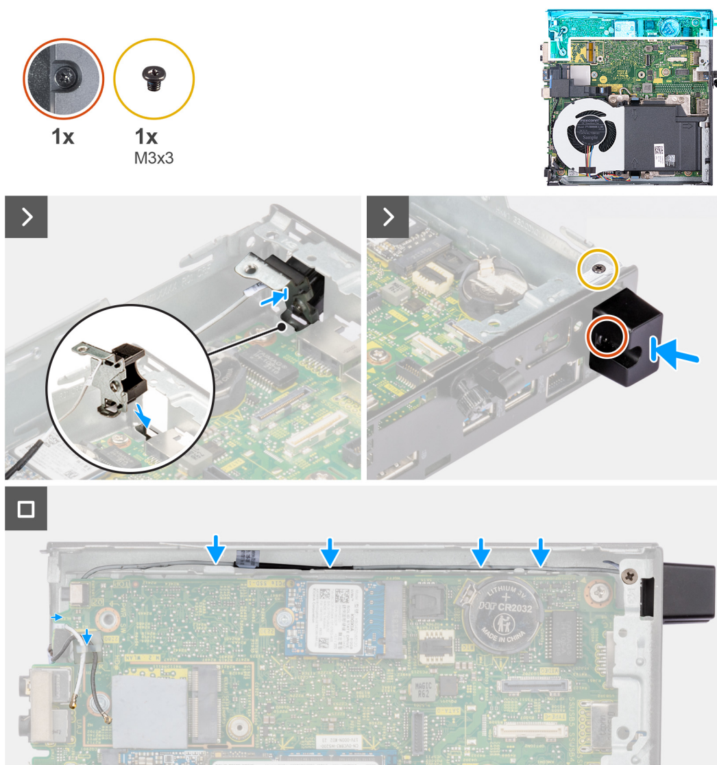
Figura 51. Installazione del modulo dell'antenna (cavo bianco)
