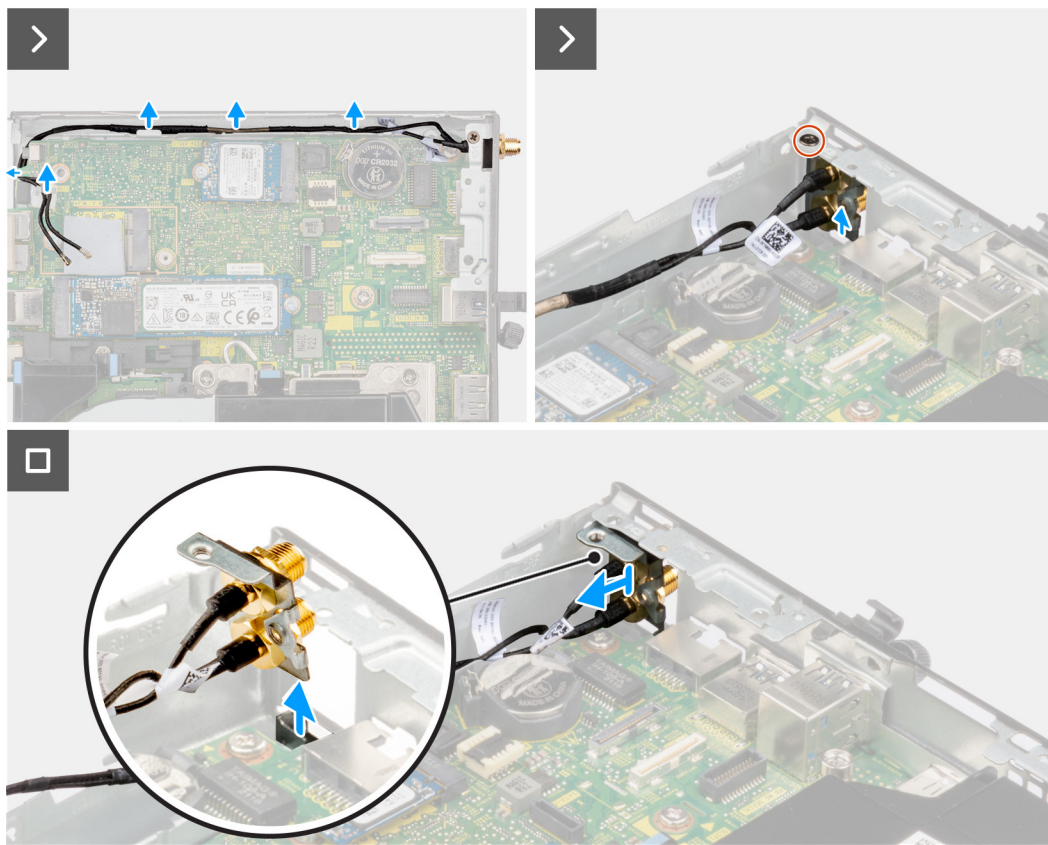
Figura 54. Rimozione dell'antenna SMA
