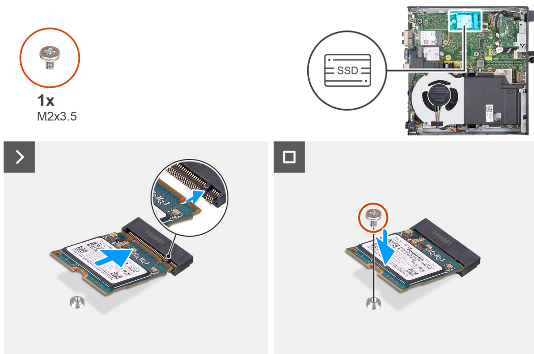
Figura 22. Installazione dell'unità SSD M.2 2230 nello slot 1
