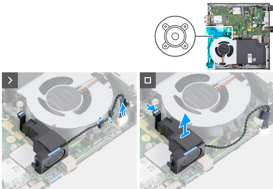
Figura 17. Rimozione degli altoparlanti
