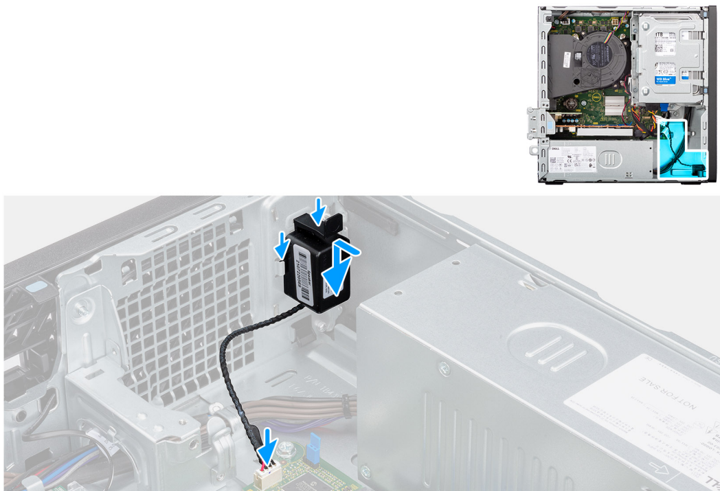
Figura 32. Installazione dell'altoparlante
