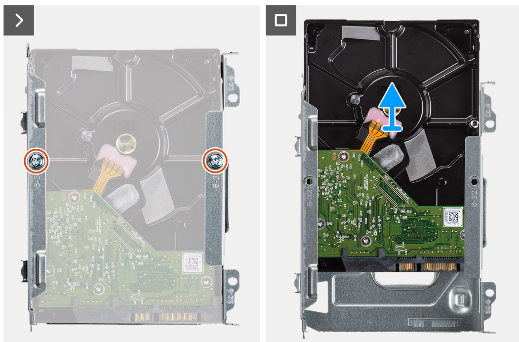
Figura 9. Rimozione del disco rigido da 3,5 pollici
