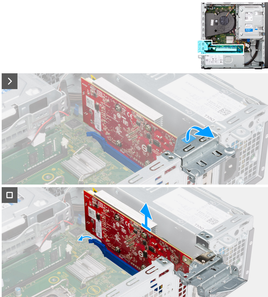
Figura 29. Rimozione della scheda grafica
