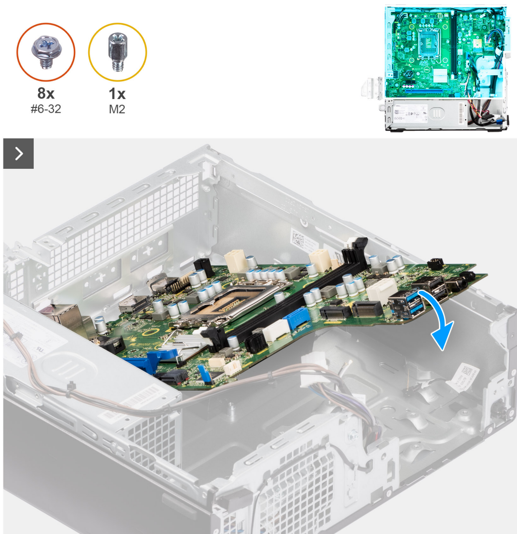
Figura 62. Installazione della scheda di sistema
