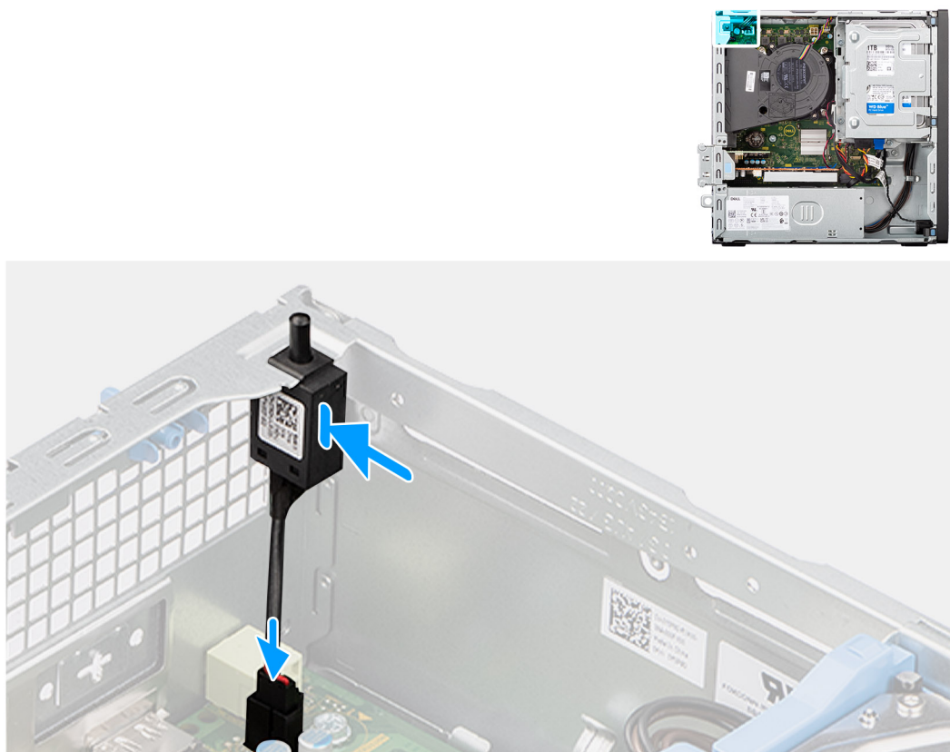
Figura 34. Installazione dello switch antintrusione
