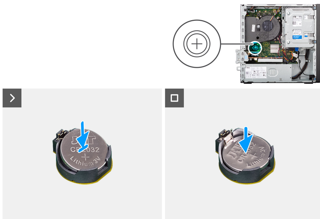
Figura 6. Installazione della batteria a bottone
