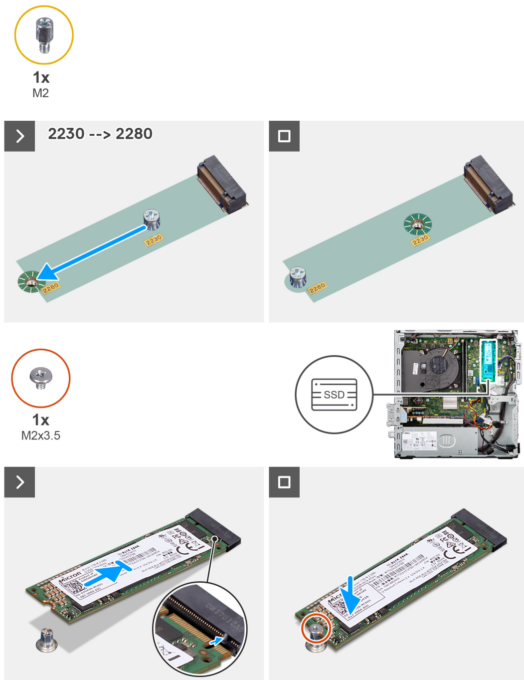
Figura 20. Installazione dell'unità SSD M.2 2280
