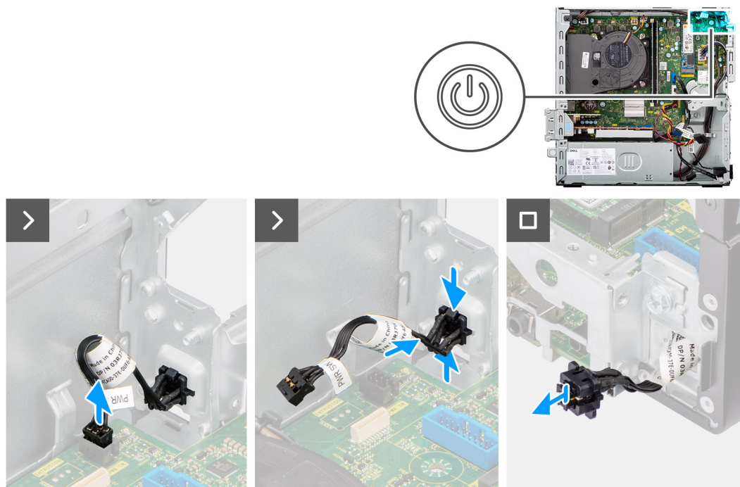
Figura 35. Rimozione del pulsante di accensione
