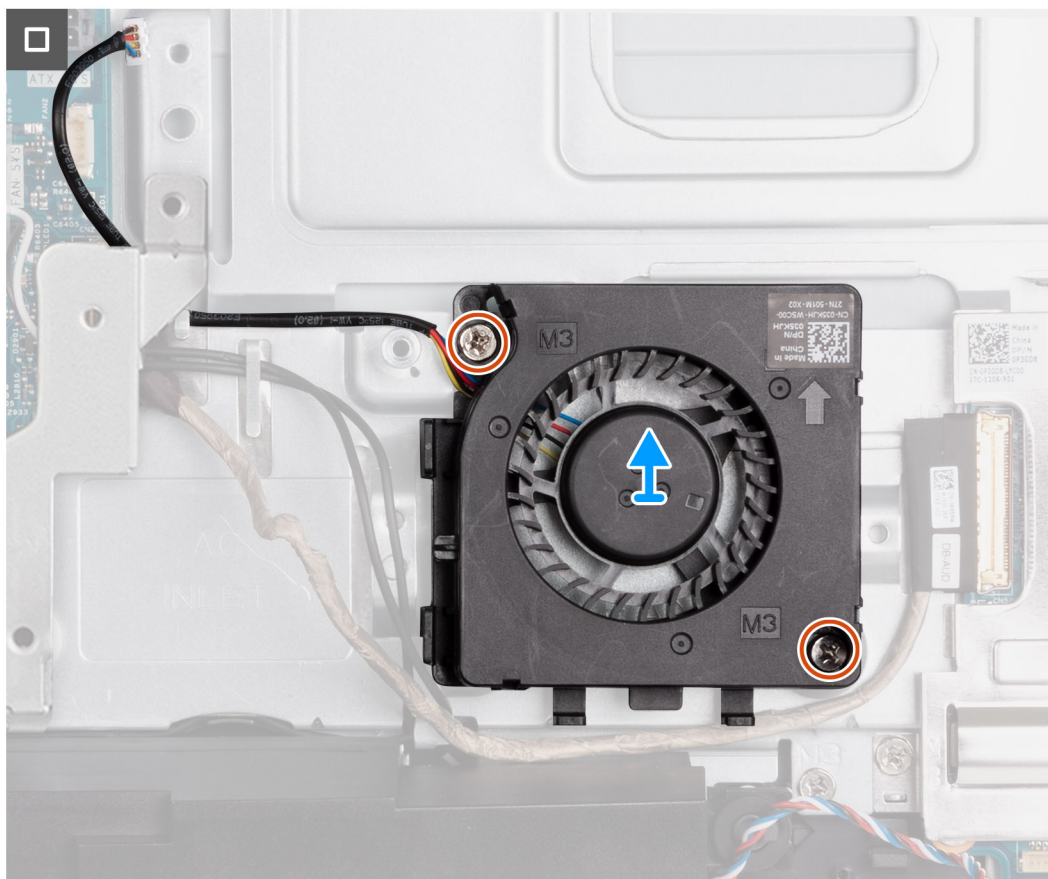
Figura 54. Rimozione della ventola di alimentazione
