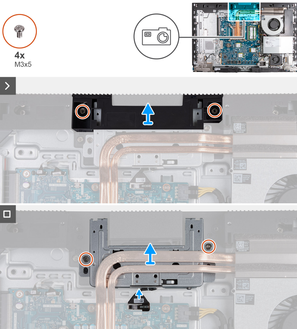
Figura 46. Rimozione del gruppo della fotocamera retraibile
