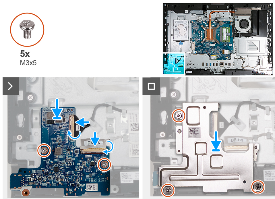
Figura 120. Installazione della scheda del pulsante di accensione e di I/O
