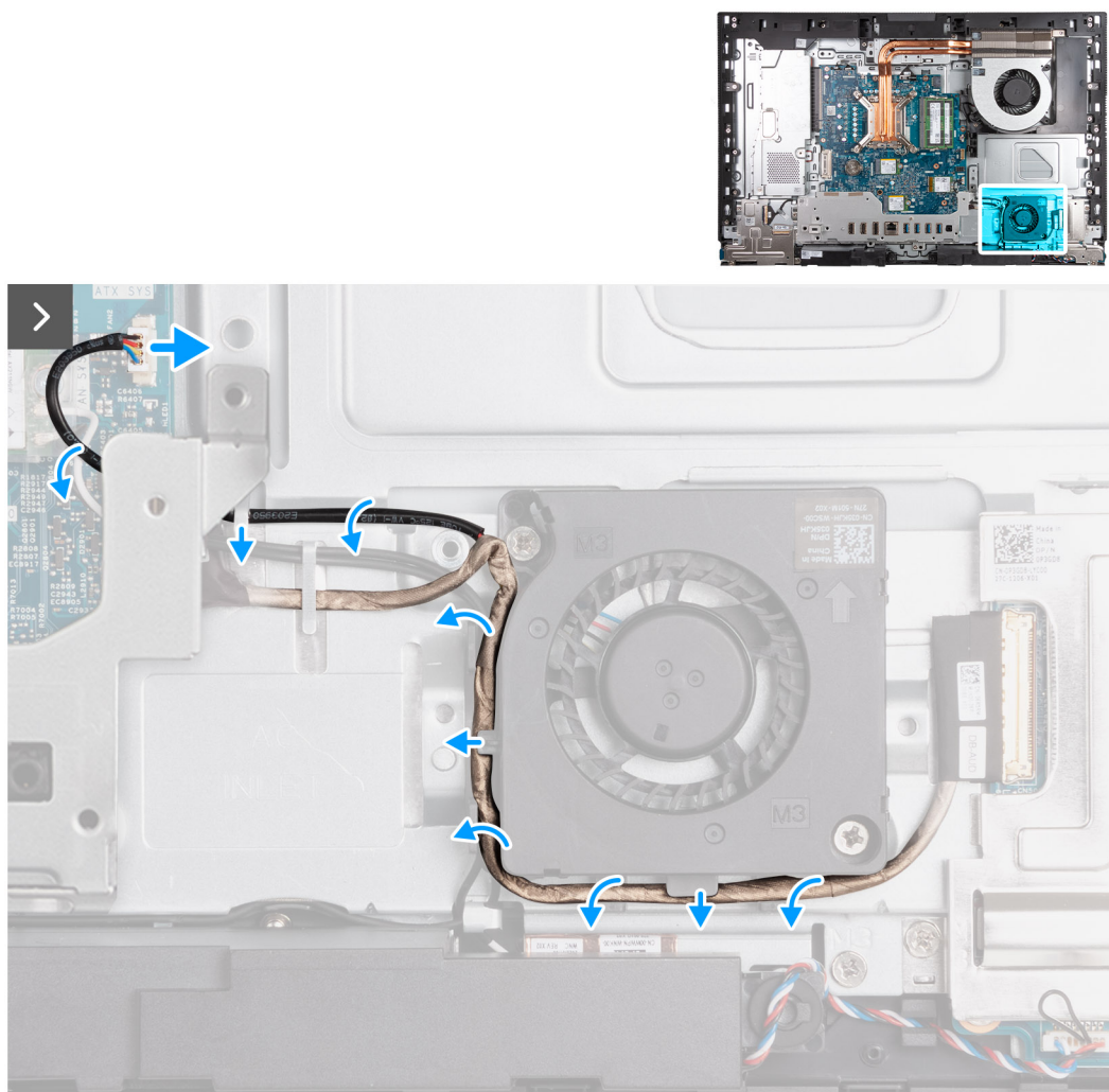
Figura 52. Rimozione della ventola di alimentazione
