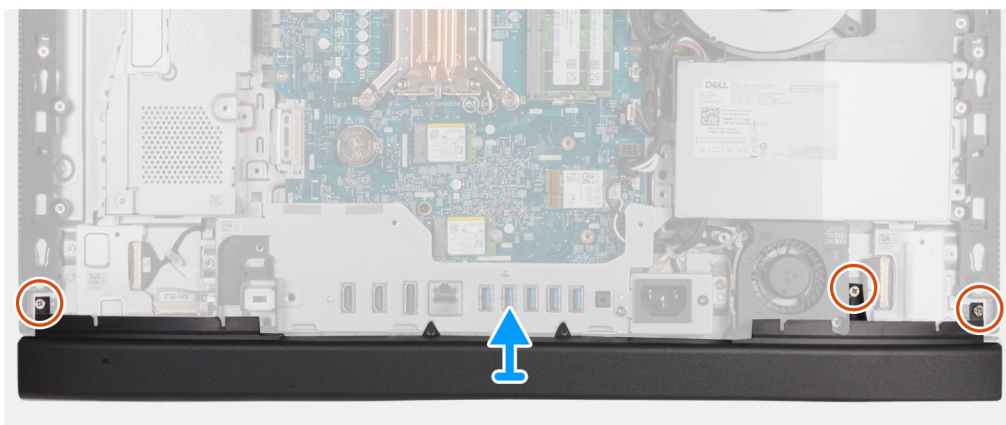
Figura 44. Rimozione del coperchio inferiore
