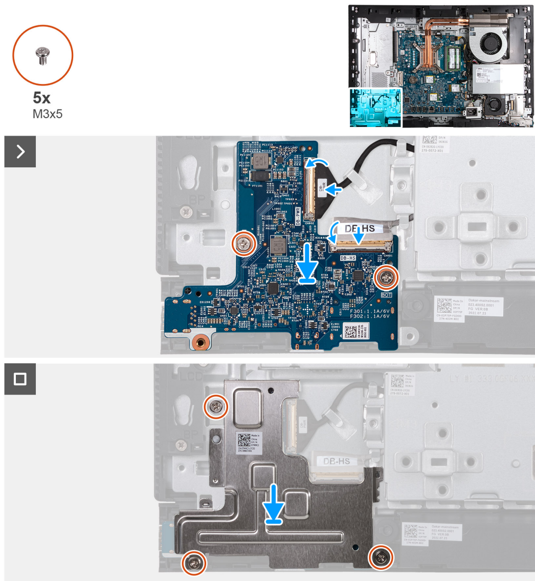
Figura 73. Installazione della scheda del pulsante di accensione e di I/O
