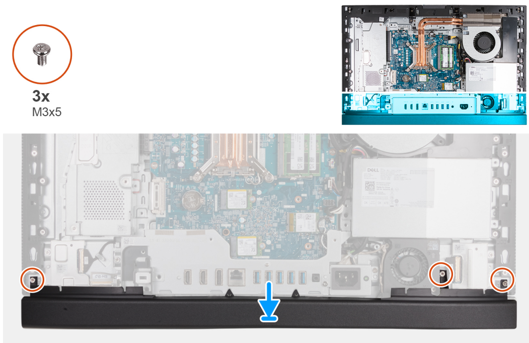
Figura 45. Installazione del coperchio inferiore
