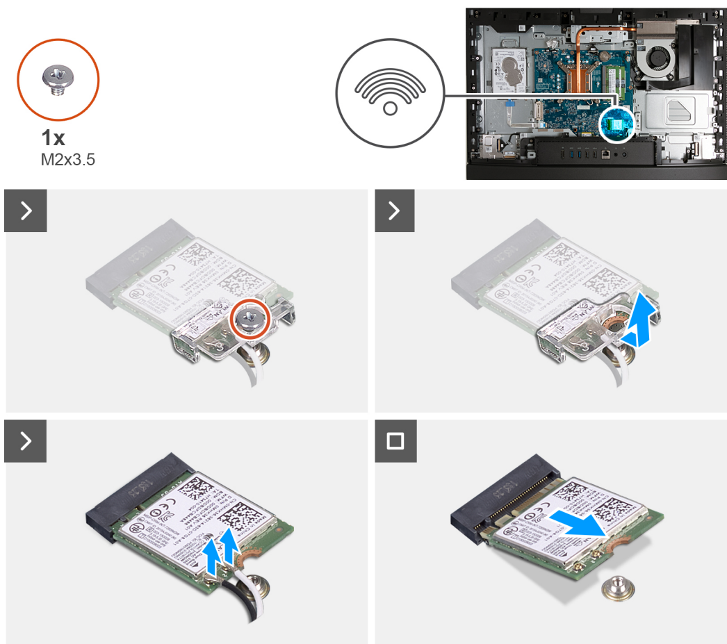
Figura 88. Rimozione della scheda wireless
