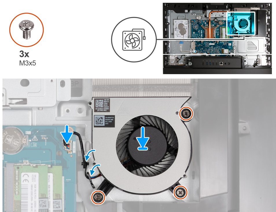
Figura 104. Installazione della ventola
