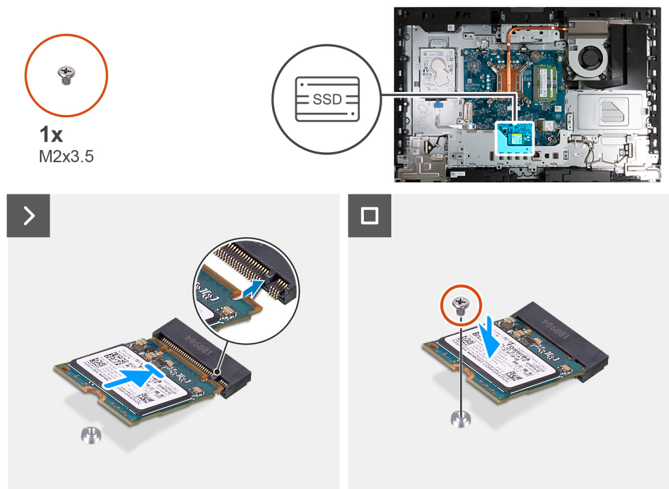
Figura 91. Installazione dell'unità SSD M.2 2230
