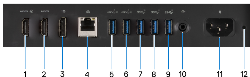
Figura 8. Vista del pannello posteriore di OptiPlex All-in-One 7420 con processore a prestazioni elevate
