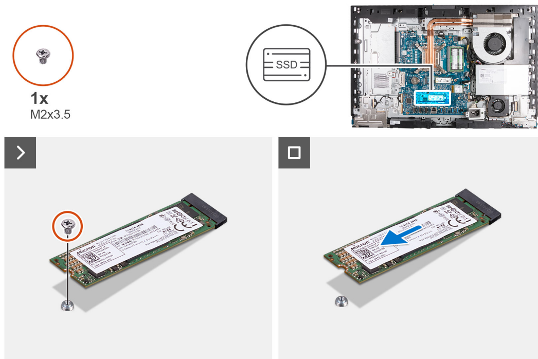
Figura 37. Rimozione dell'unità SSD M.2 2280 dallo slot M.2 1
