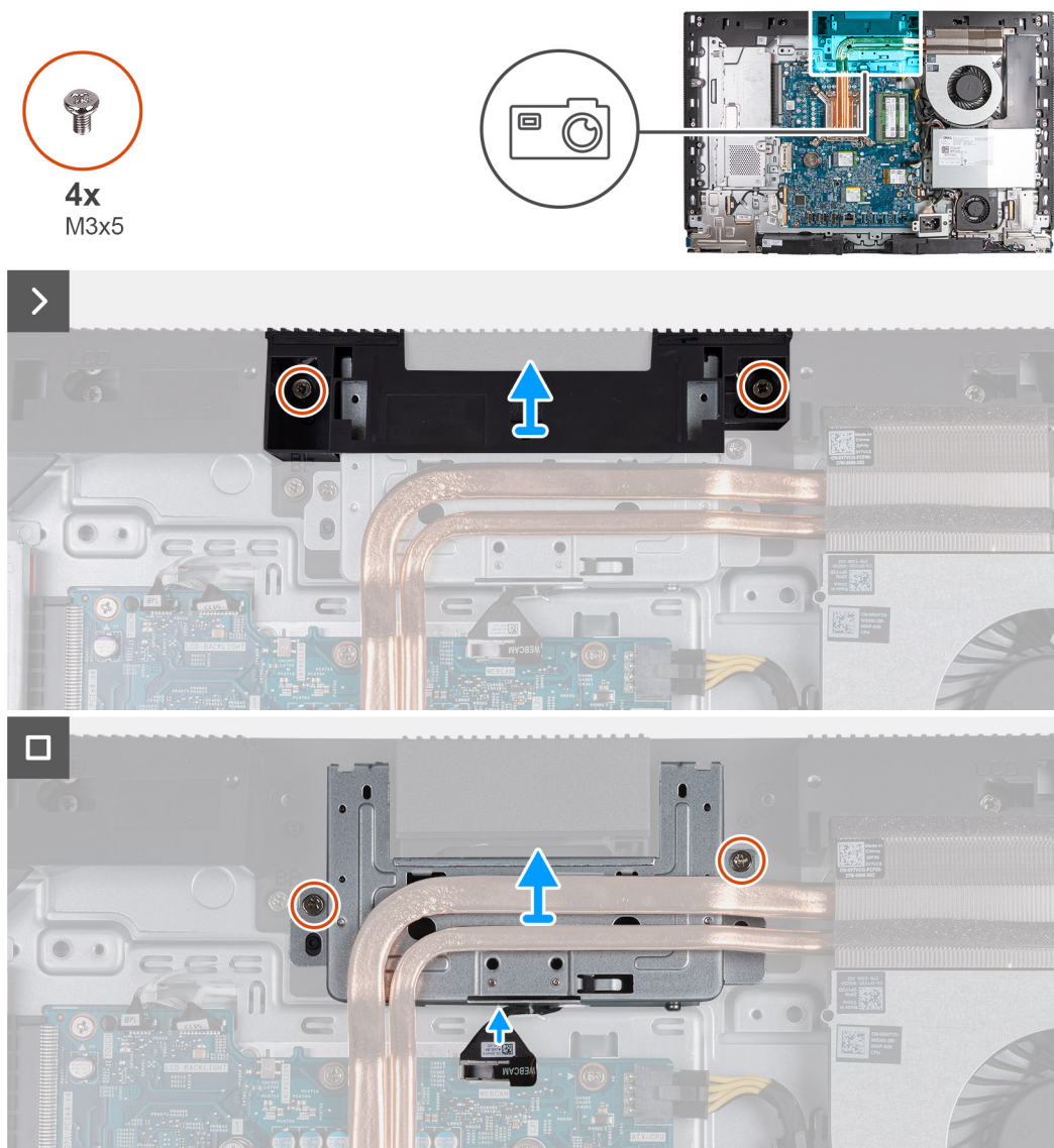
Figura 46. Rimozione del gruppo della fotocamera retraibile
