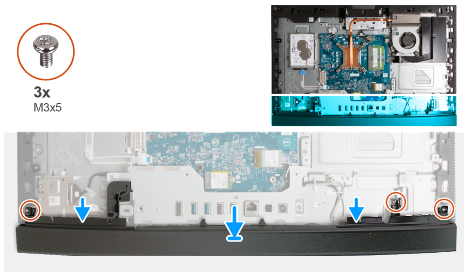
Figura 100. Installazione del coperchio inferiore
