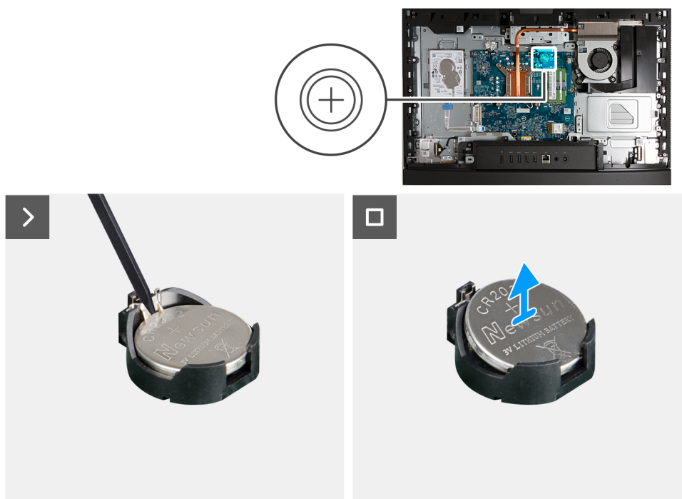
Figura 95. Rimozione della batteria a bottone
