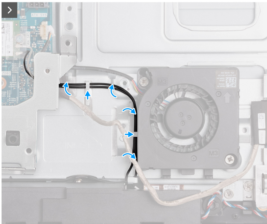
Figura 56. Installazione della ventola dell'alimentatore
