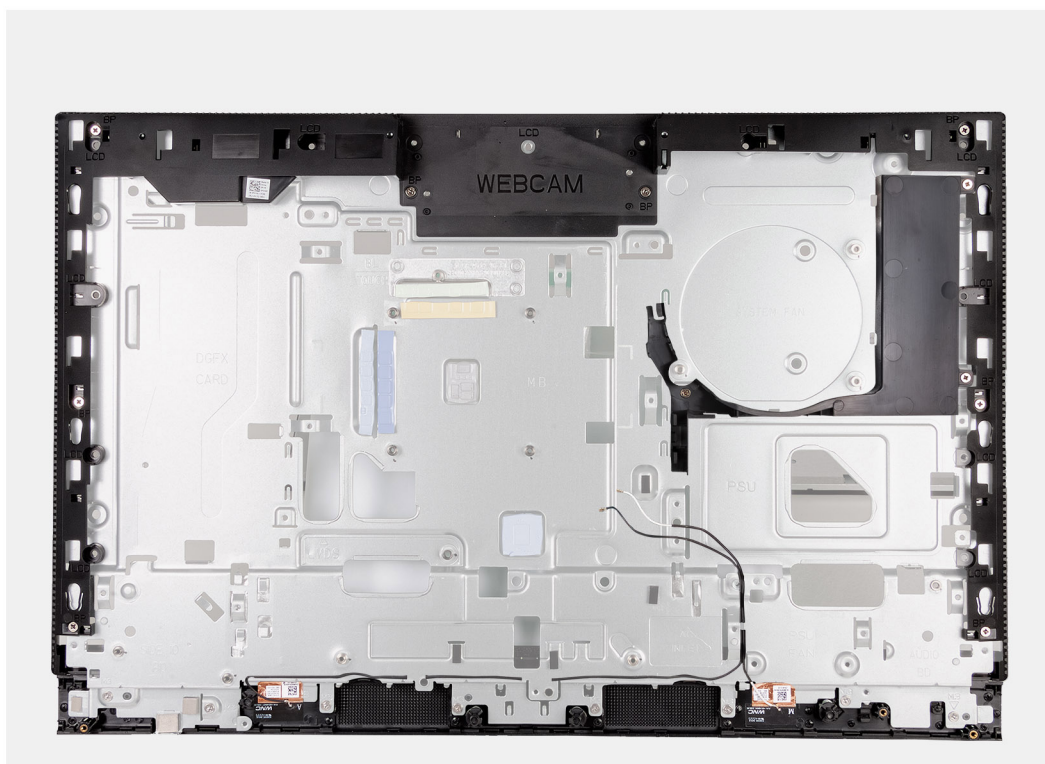
Figura 77. Installazione della base del gruppo del display
