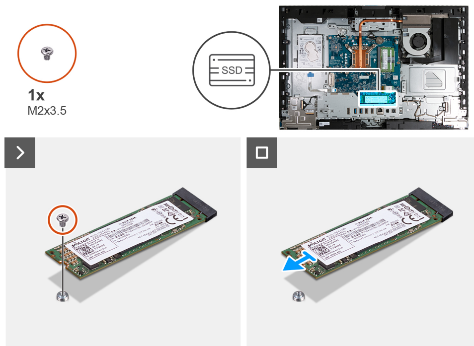
Figura 92. Rimozione dell'unità SSD M.2 2280
