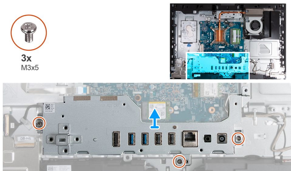
Figura 105. Rimozione della staffa di I/O
