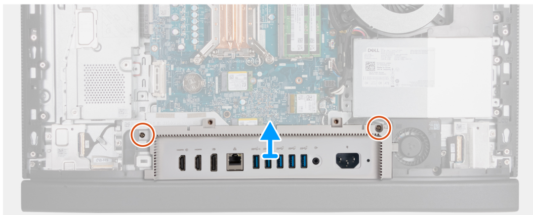
Figura 42. Rimozione del coperchio di I/O
