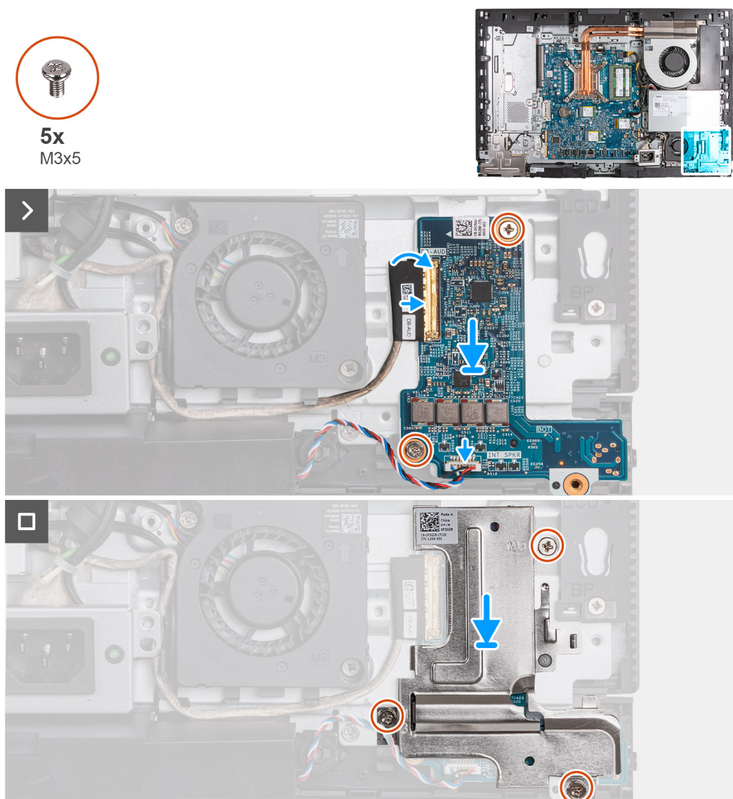
Figura 75. Installazione della scheda audio
