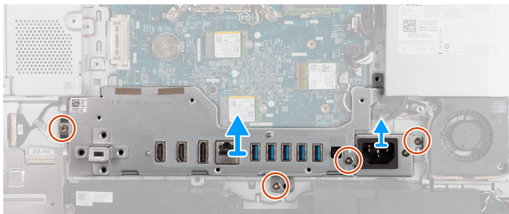
Figura 58. Rimozione della staffa di I/O
