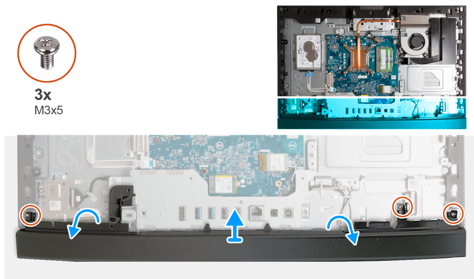
Figura 99. Rimozione del coperchio inferiore
