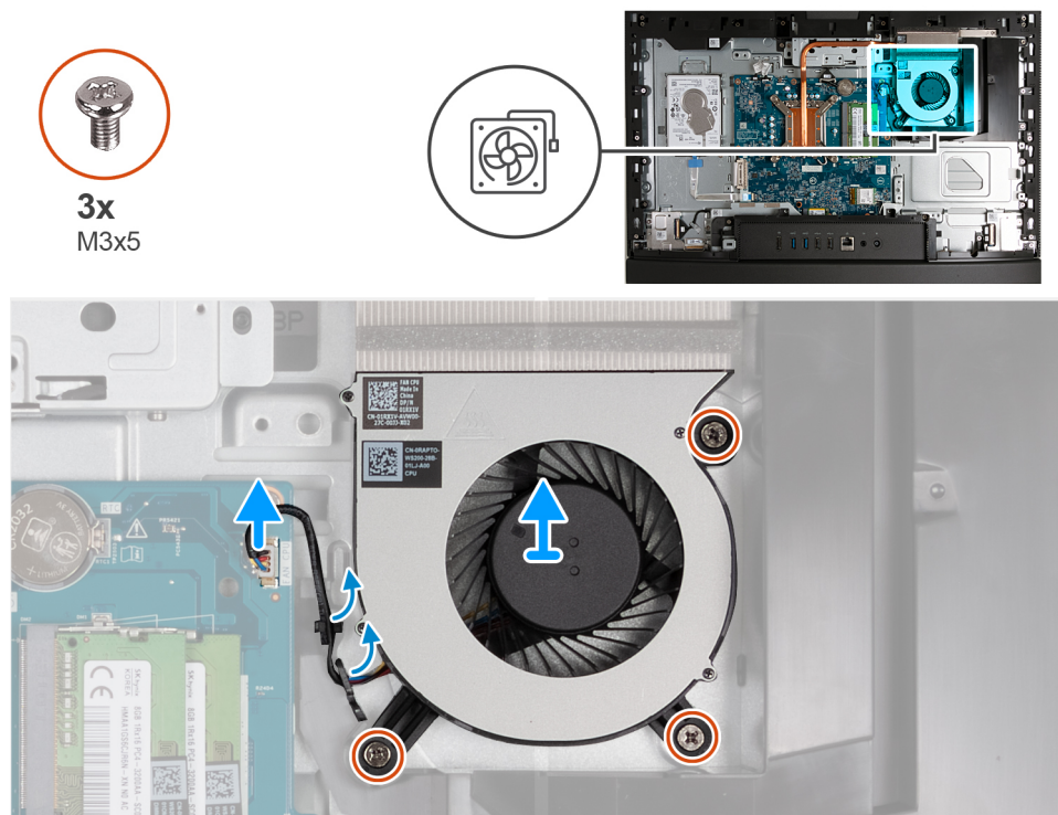
Figura 103. Rimozione della ventola
