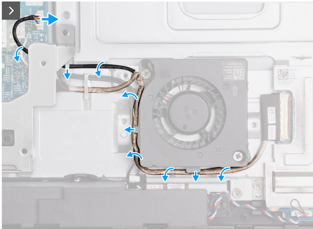
Figura 52. Rimozione della ventola di alimentazione
