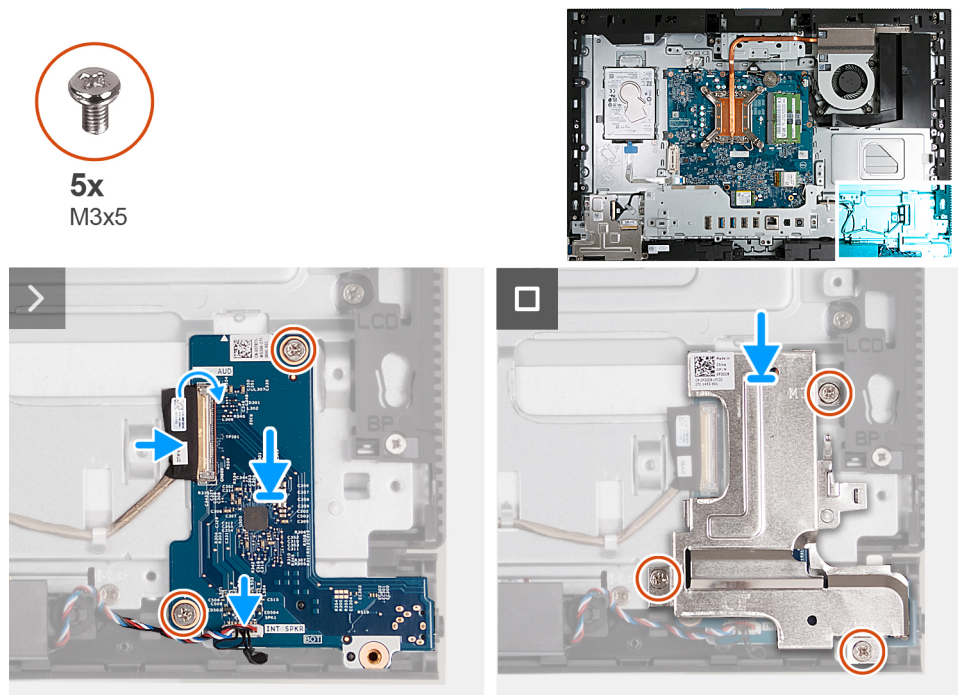
Figura 122. Installazione della scheda audio
