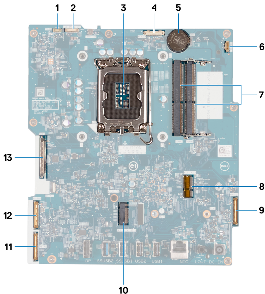
Figura 113. Callout della scheda di sistema
