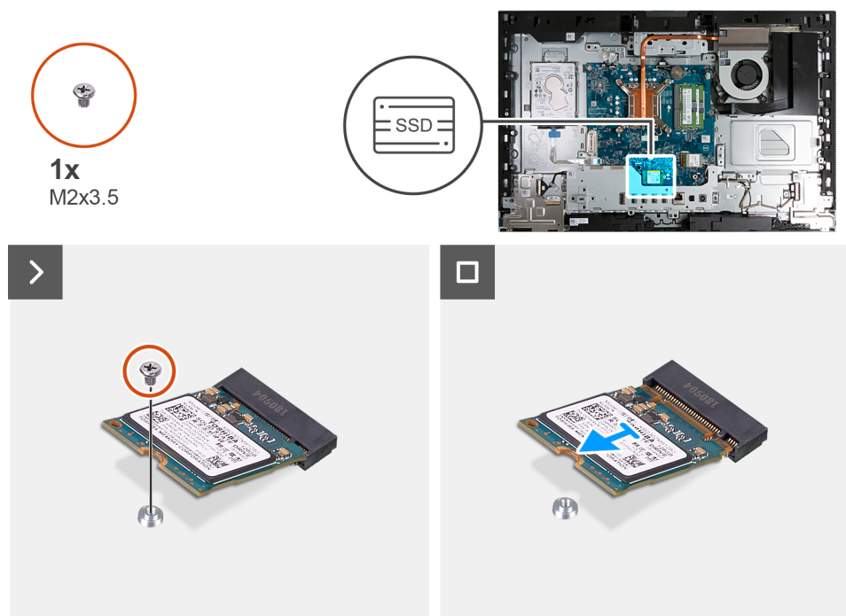
Figura 90. Rimozione dell'unità SSD M.2 2230
