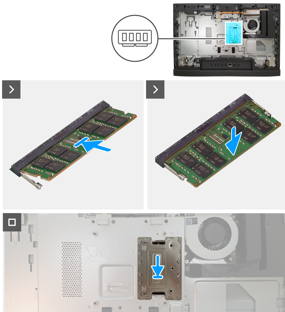
Figura 85. Installazione della memoria
