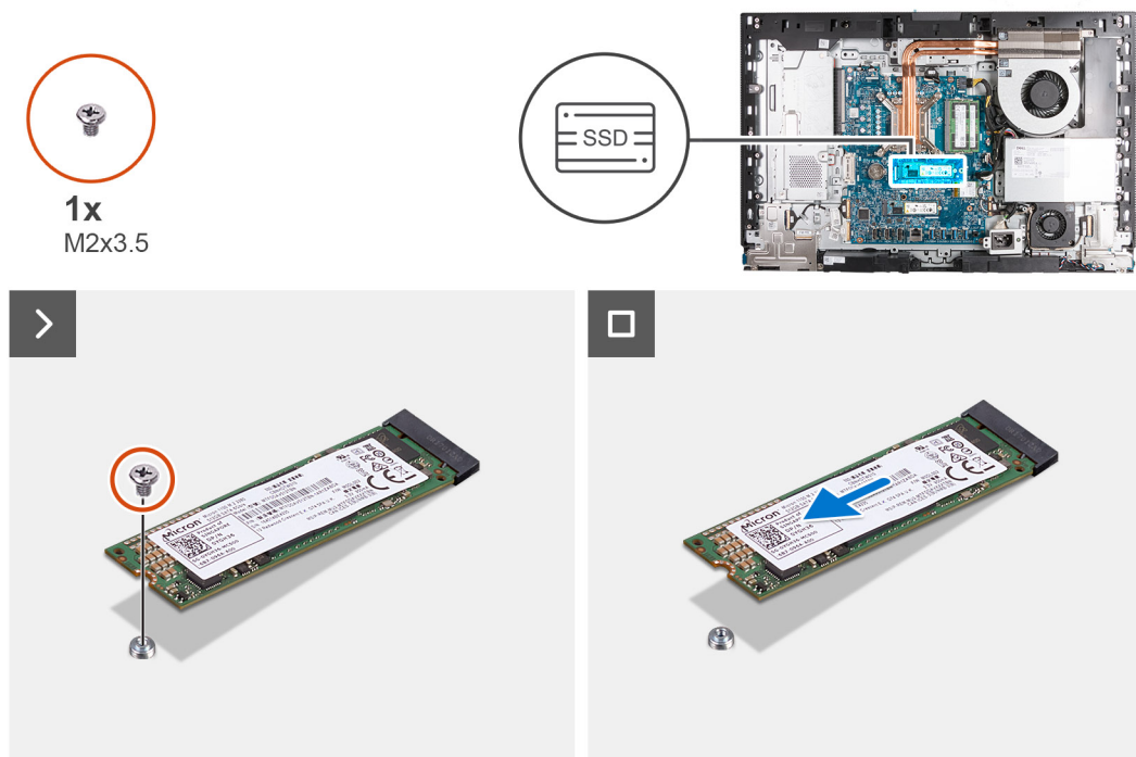
Figura 32. Rimozione dell'unità SSD M.2 2280 dallo slot M.2 0
