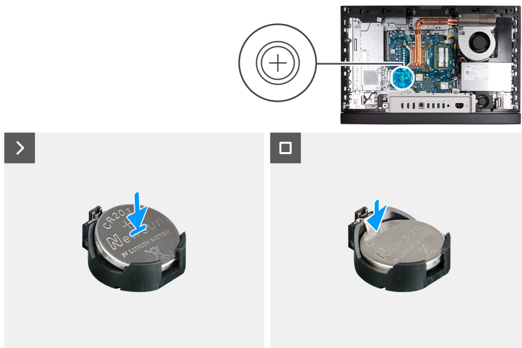
Figura 41. Installazione della batteria a bottone
