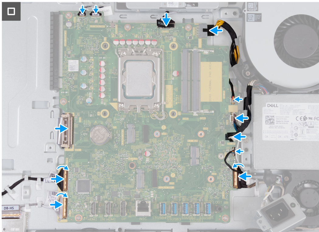
Figura 71. Installazione della scheda di sistema
