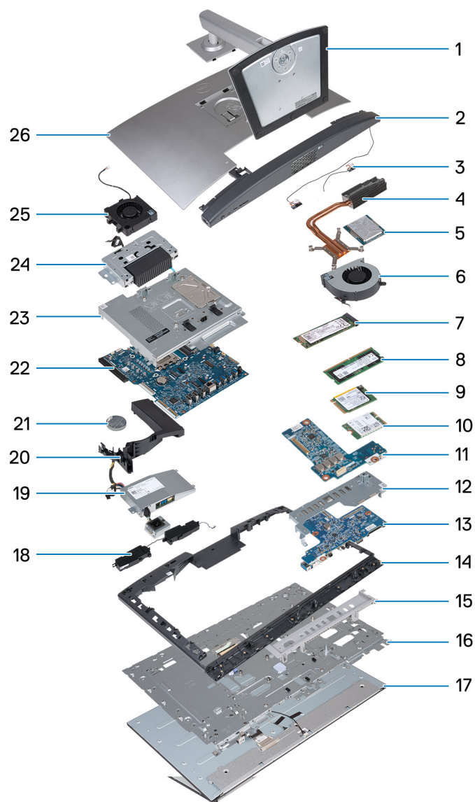
Figura 16. Componenti principali di OptiPlex All-in-One 7420 con processore a prestazioni elevate
