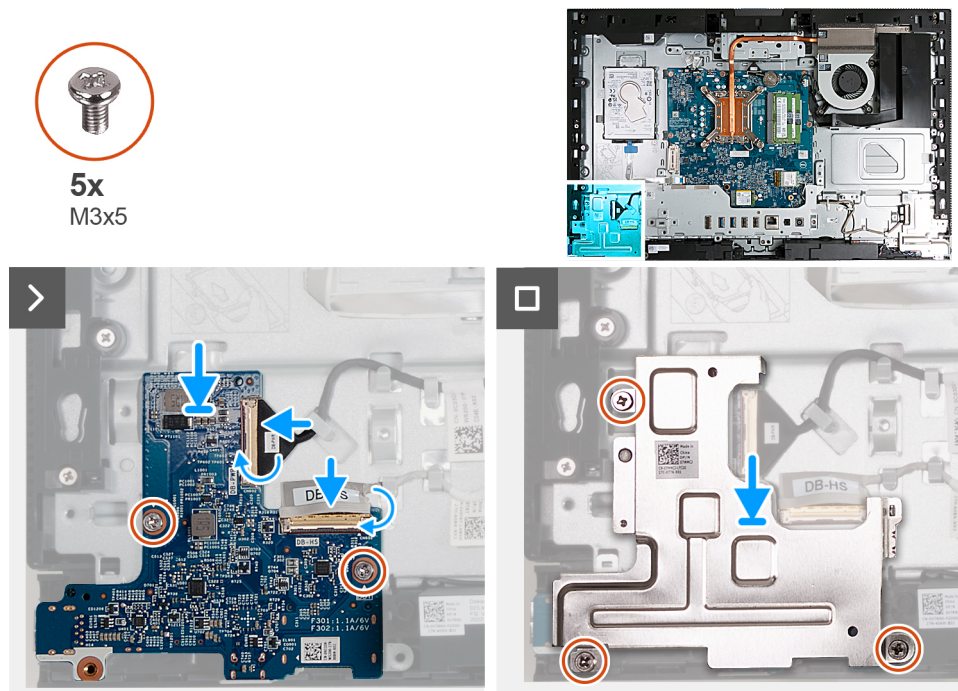
Figura 120. Installazione della scheda del pulsante di accensione e di I/O
