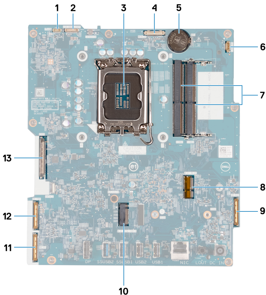
Figura 116. Callout della scheda di sistema
