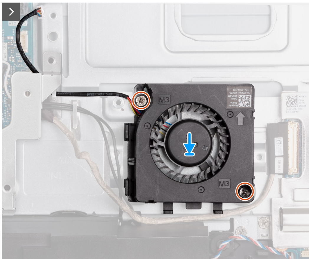
Figura 55. Installazione della ventola dell'alimentatore
