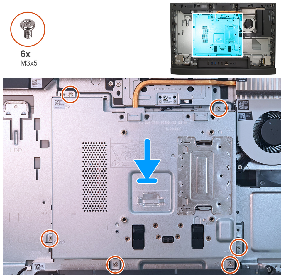
Figura 87. Installazione della protezione della scheda di sistema
