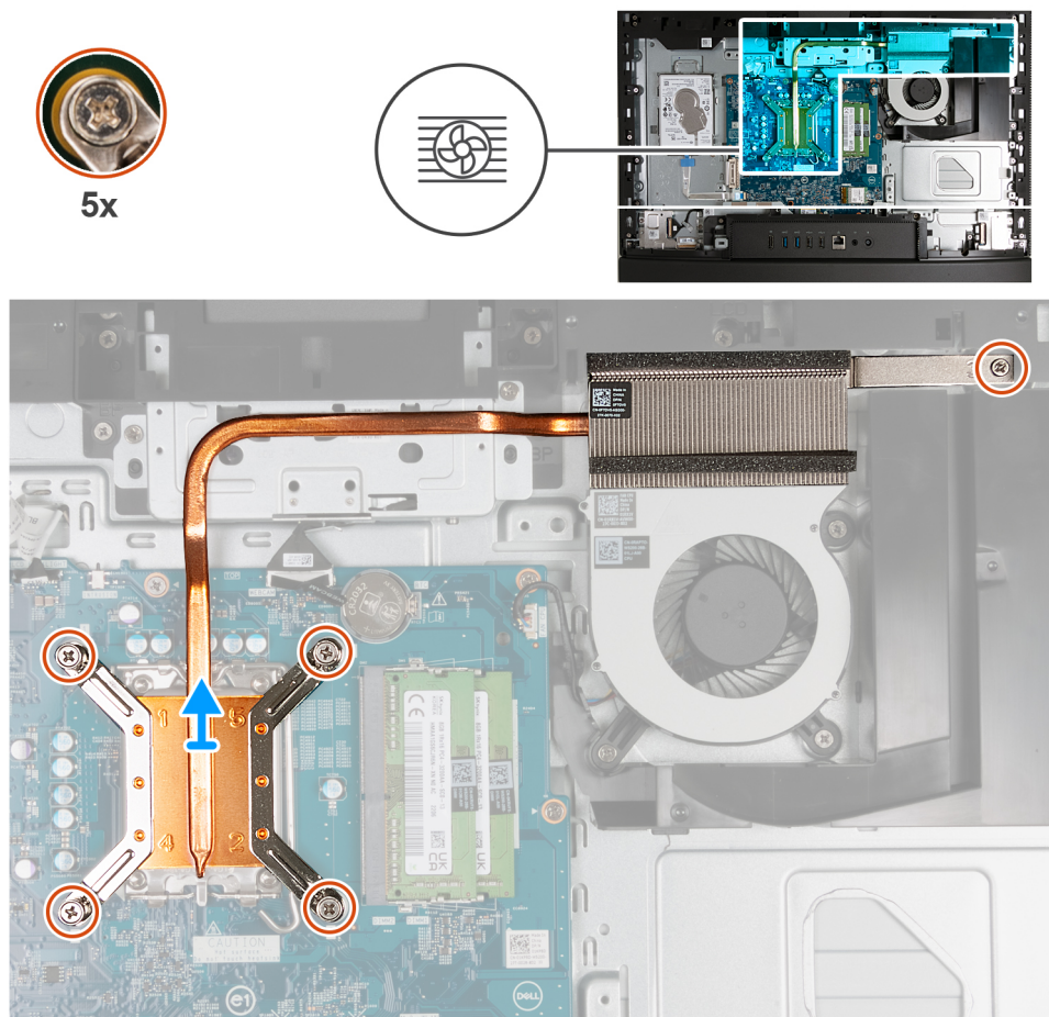
Figura 109. Rimozione del dissipatore di calore
