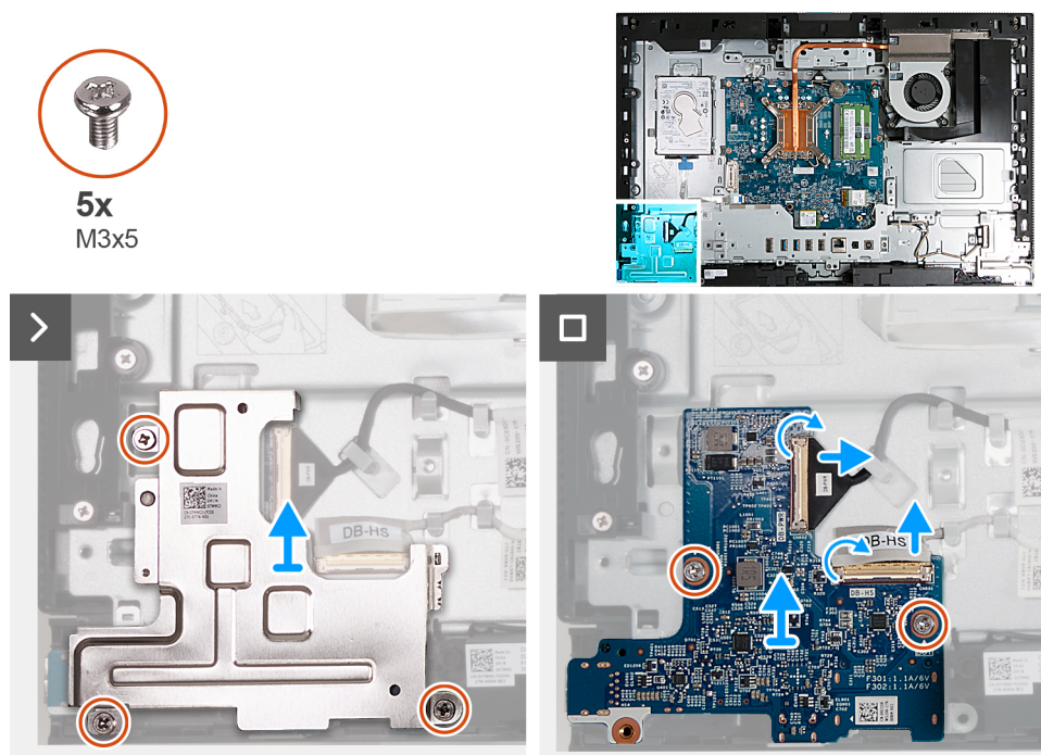
Figura 119. Rimozione della scheda del pulsante di accensione e di I/O
