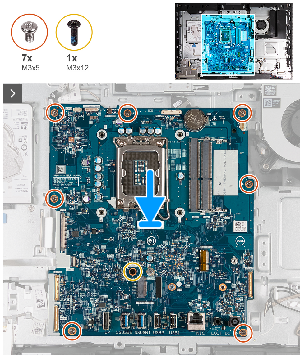
Figura 117. Installazione della scheda di sistema
