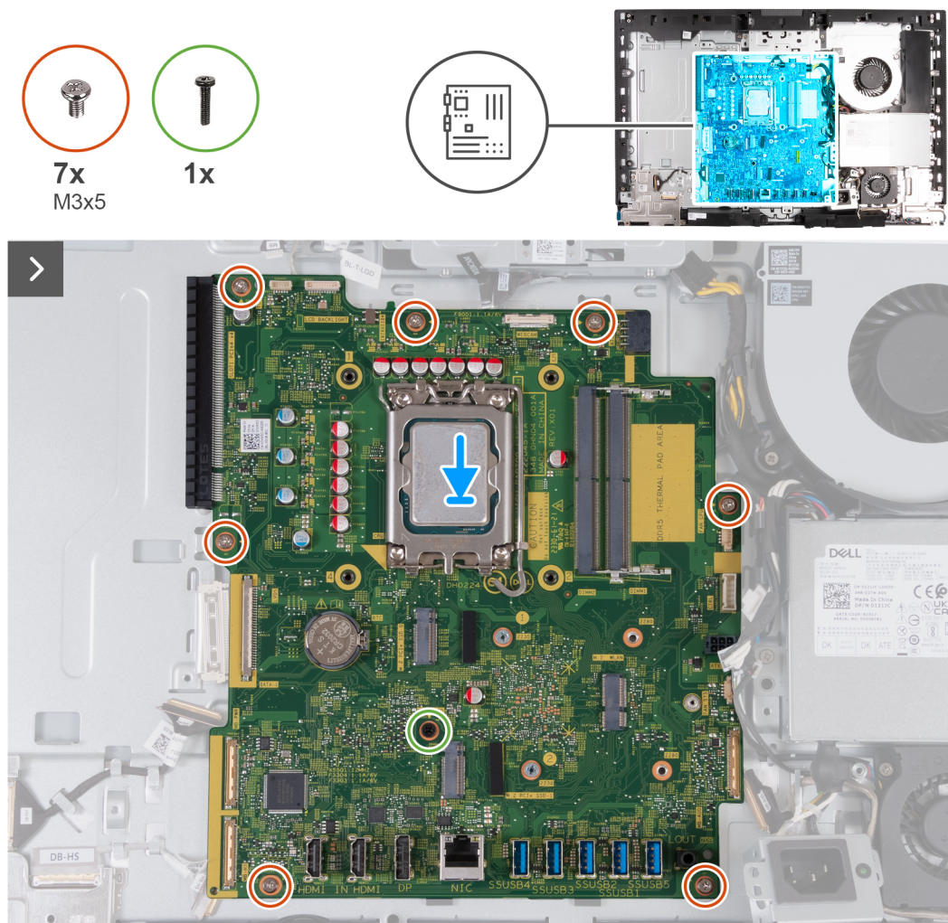
Figura 70. Installazione della scheda di sistema
