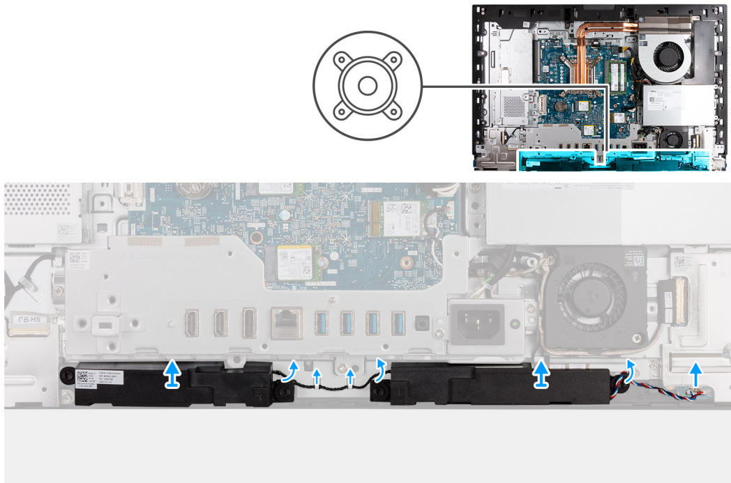
Figura 60. Rimozione degli altoparlanti
