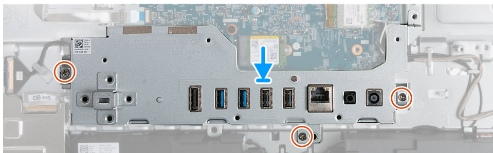
Figura 106. Installazione della staffa di I/O
