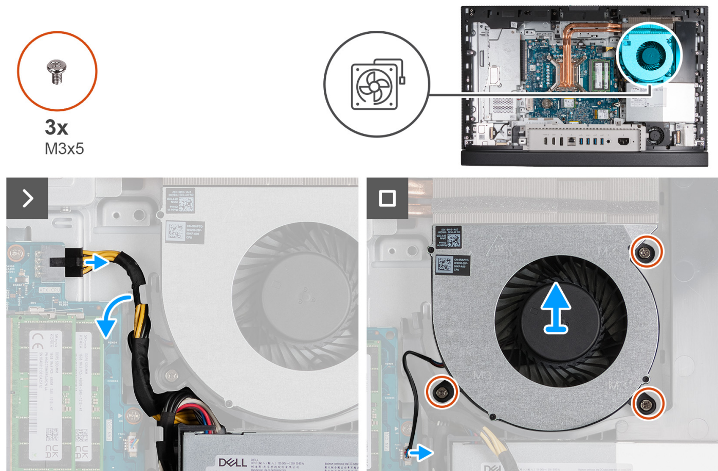
Figura 48. Rimozione della ventola
