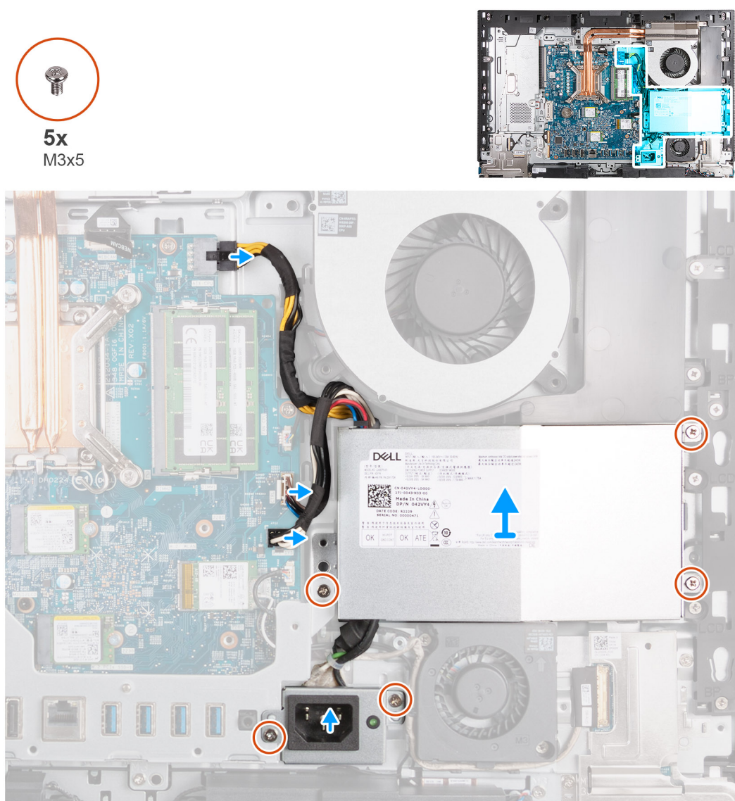
Figura 50. Rimozione dell'unità di alimentazione
