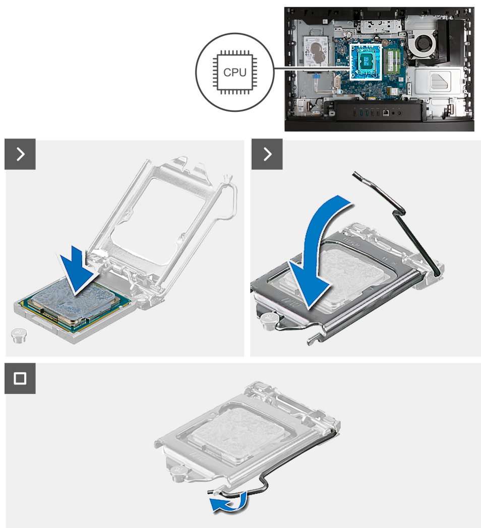
Figura 112. Installazione del processore
