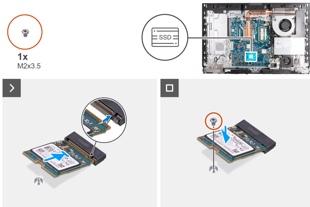
Figura 36. Installare l'unità SSD M.2 2230 nello slot M.2 1
