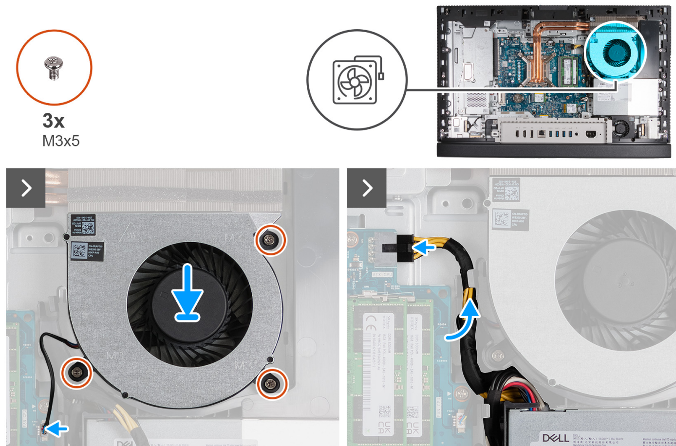
Figura 49. Installazione della ventola
