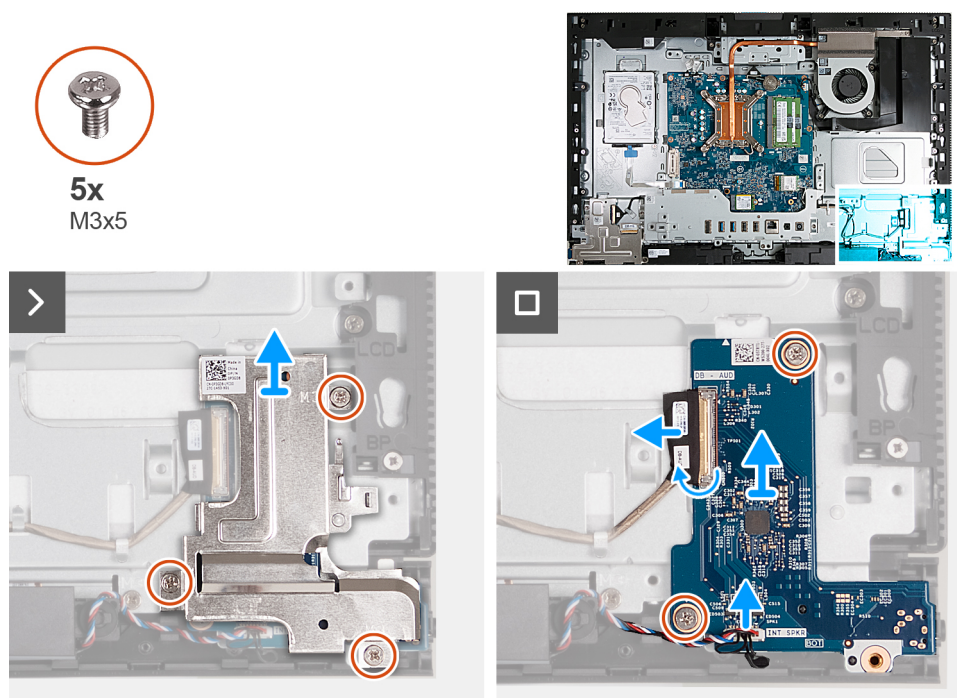
Figura 121. Rimozione della scheda audio
