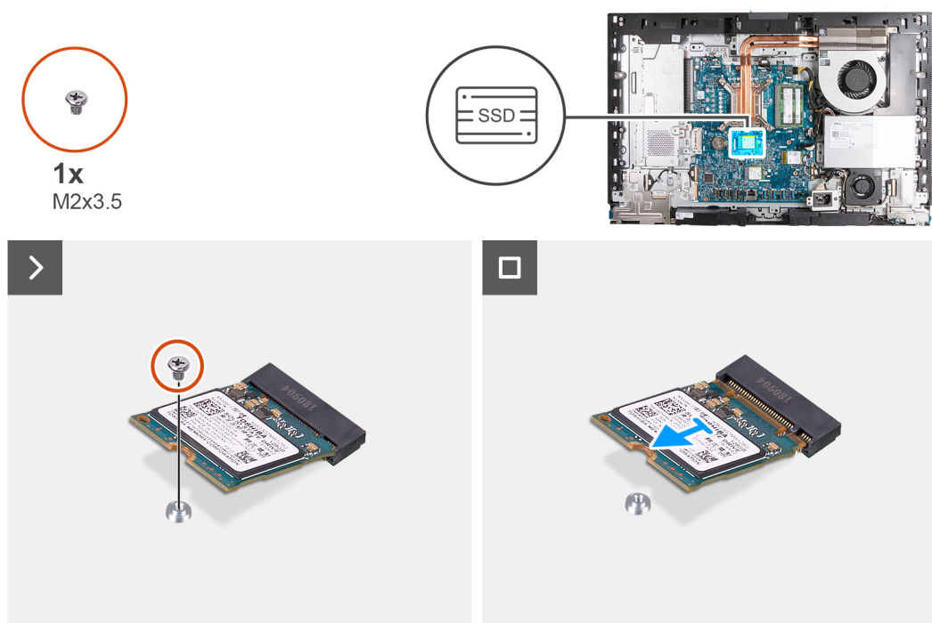
Figura 30. Rimozione dell'unità SSD M.2 2230 dallo slot M.2 0
