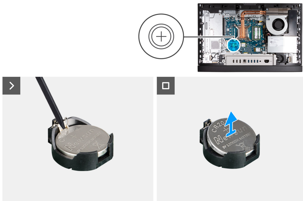
Figura 40. Rimozione della batteria a bottone
