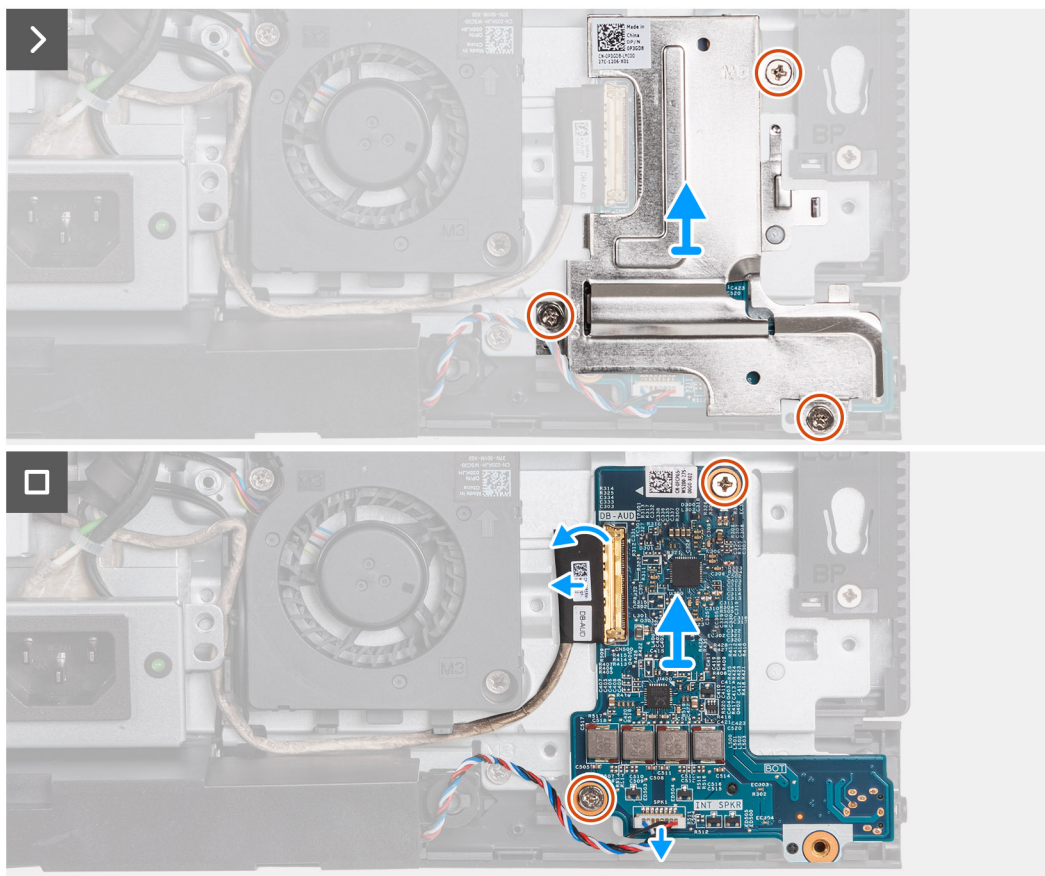
Figura 74. Rimozione della scheda audio
