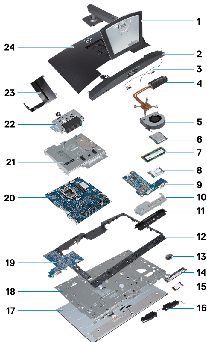
Figura 17. Componenti principali di OptiPlex All-in-One 7420 con processore con risparmio energetico
