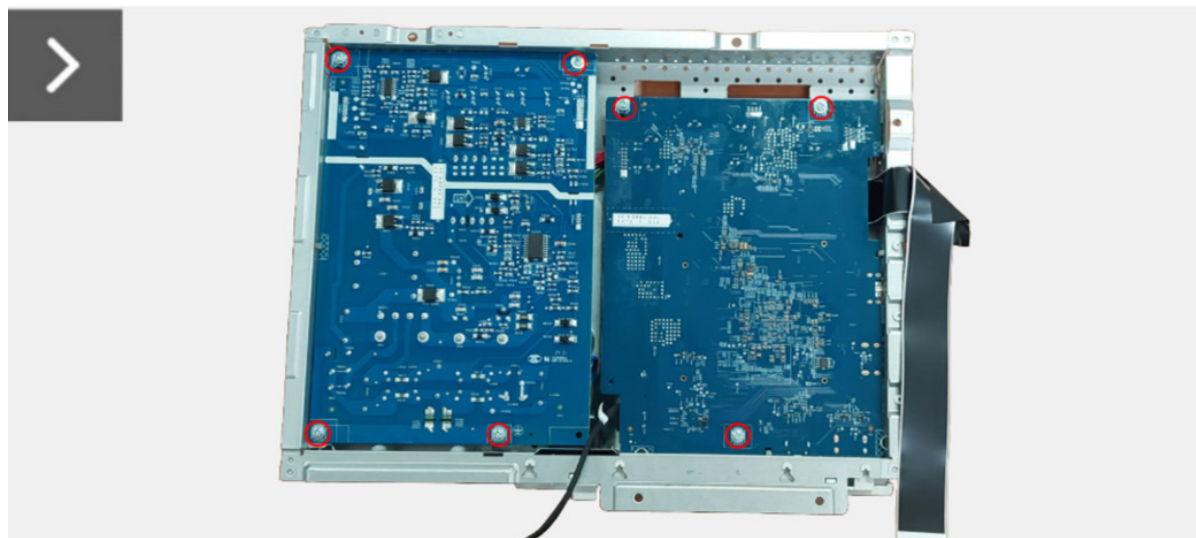
Immagine 22. Installazione della scheda interfaccia
