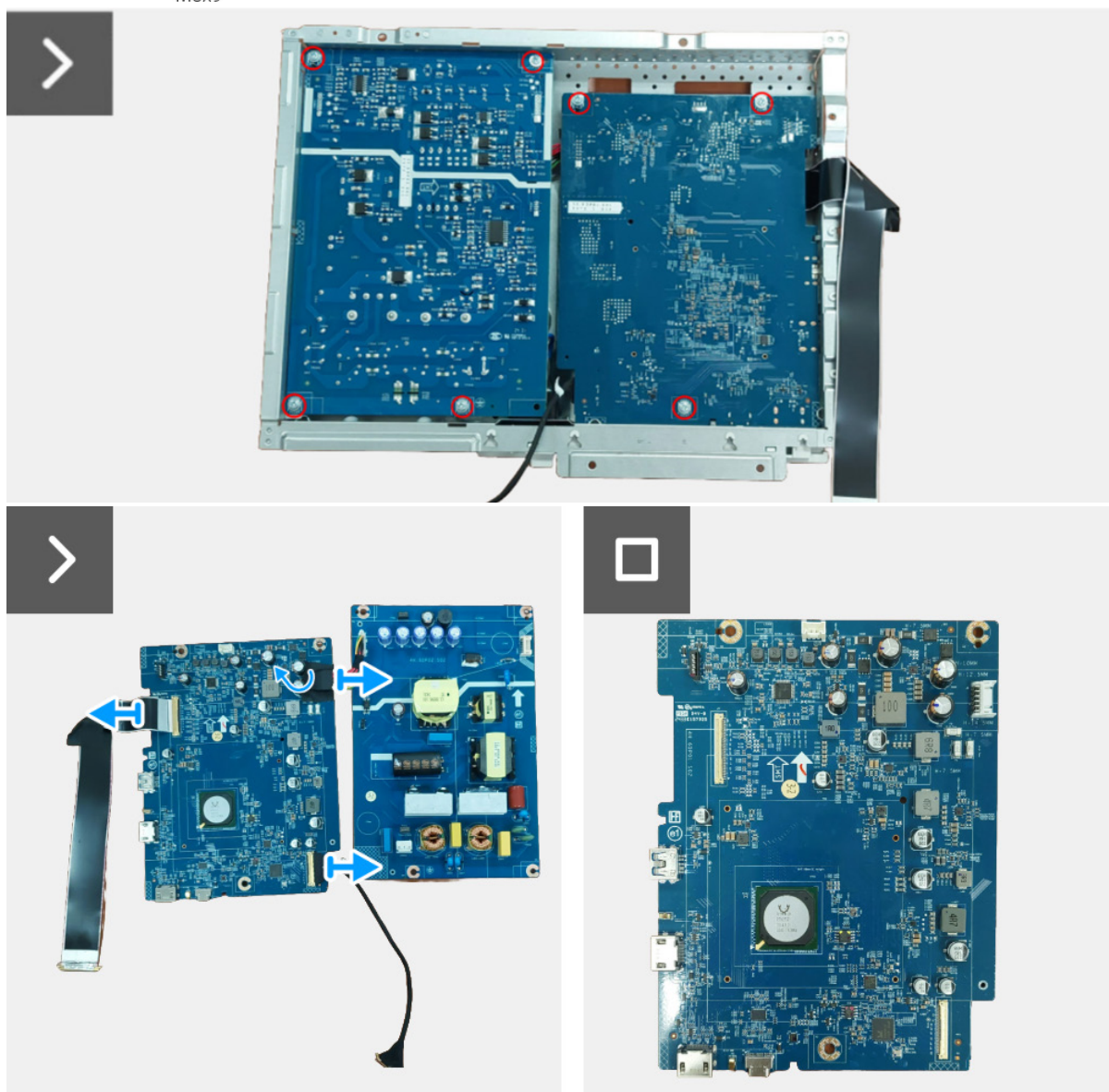
Immagine 21. Rimozione della scheda interfaccia
