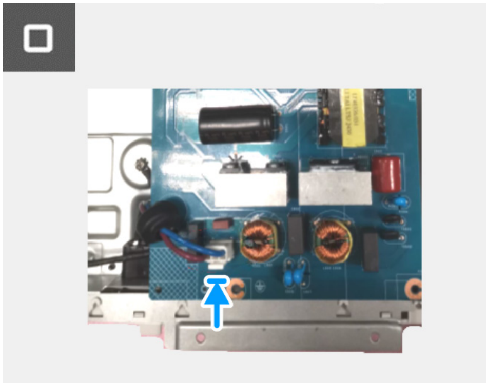
Immagine 25. Installazione della scheda alimentazione
