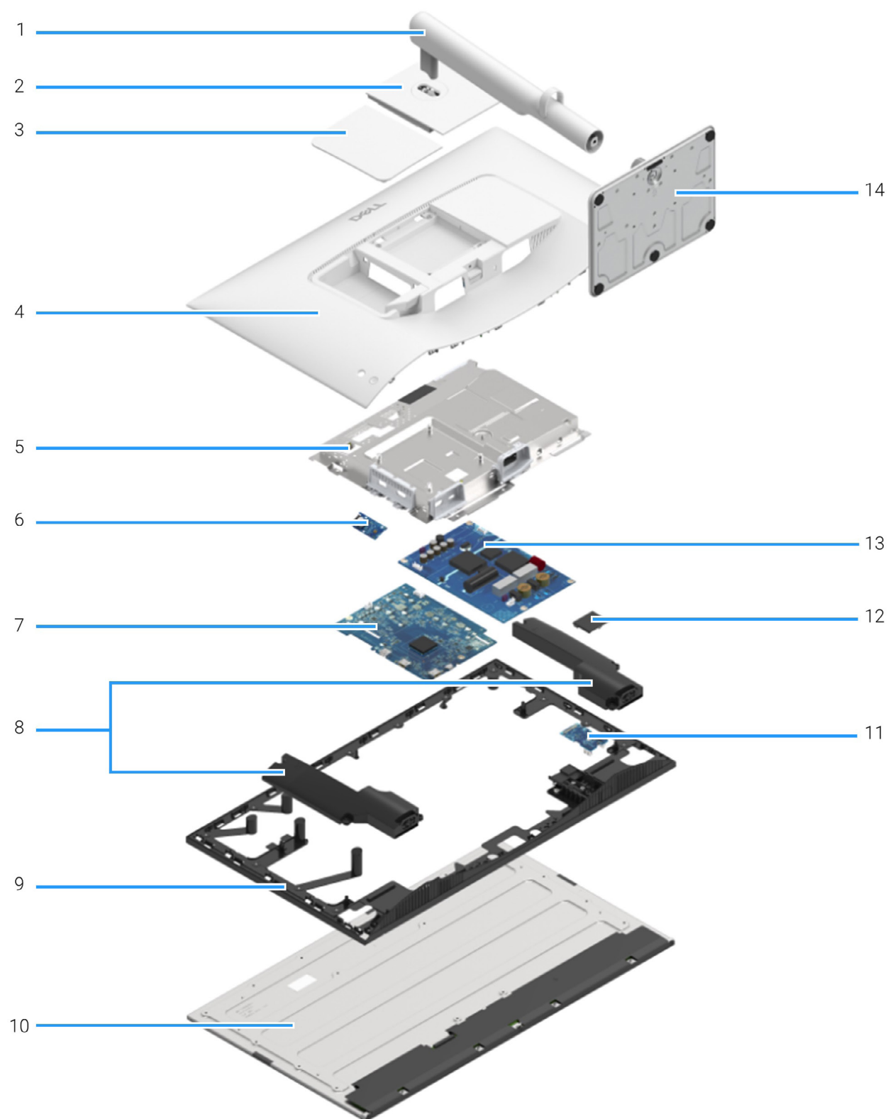
Immagine 6. Principali componenti
