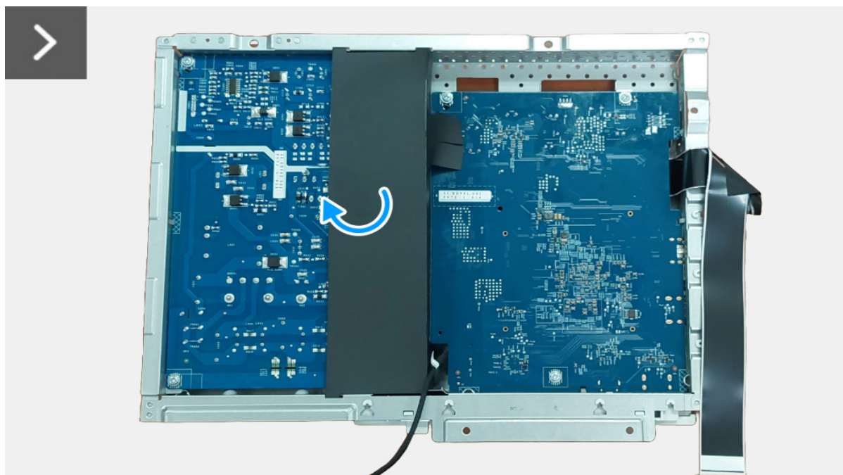
Immagine 20. Rimozione della scheda interfaccia
