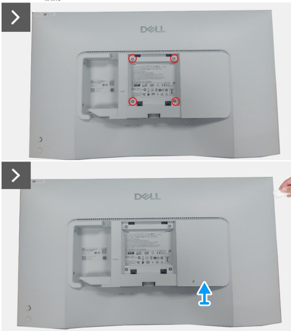
Immagine 12. Rimozione del coperchio posteriore
