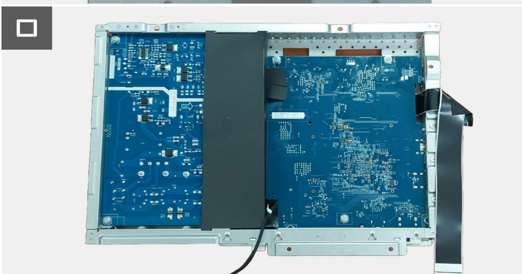
Immagine 17. Rimozione del gruppo scheda interfaccia
