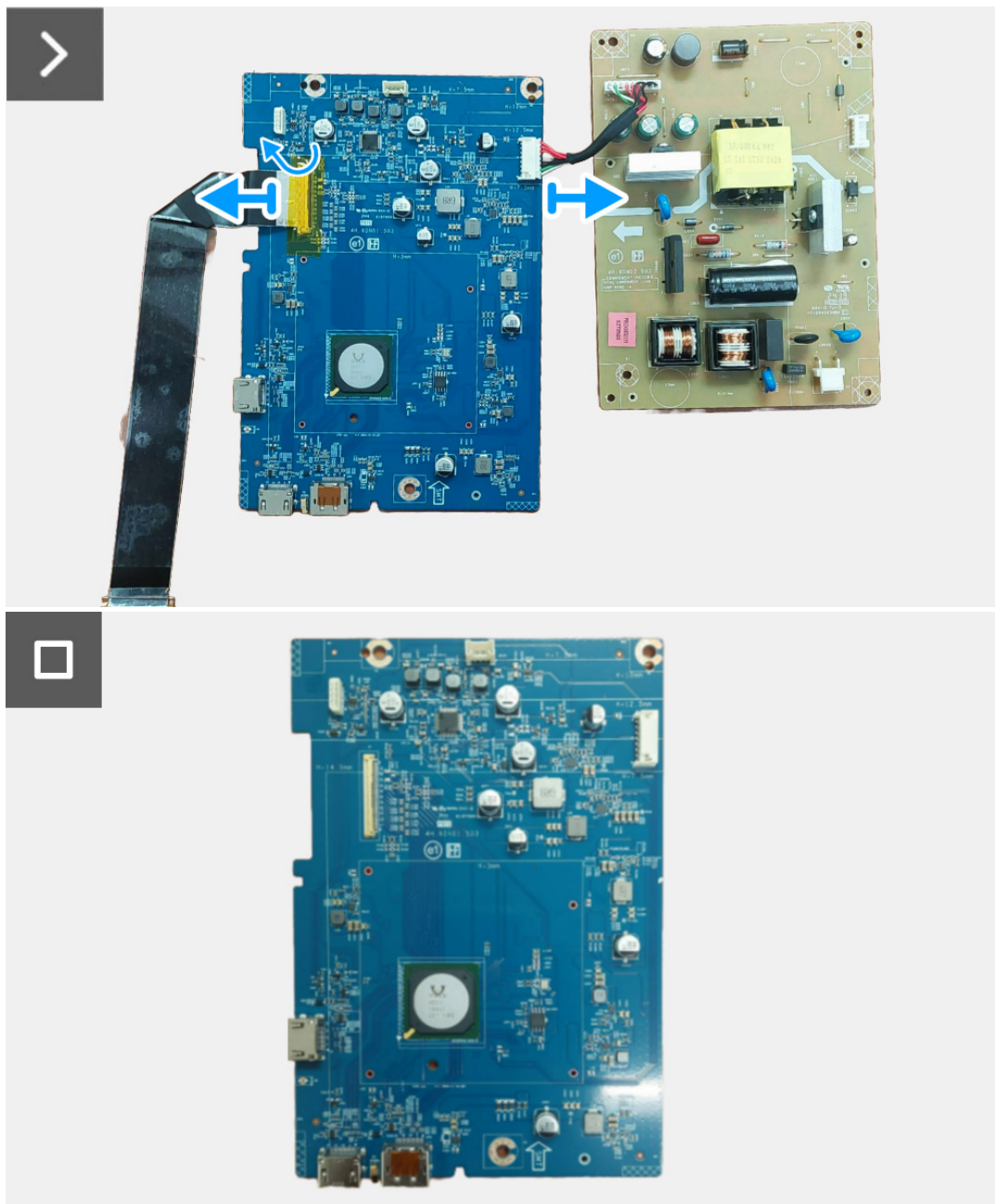
Immagine 20. Rimozione della scheda interfaccia
