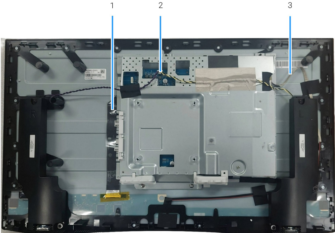
Immagine 6. Diagramma della connettività del cablaggio
