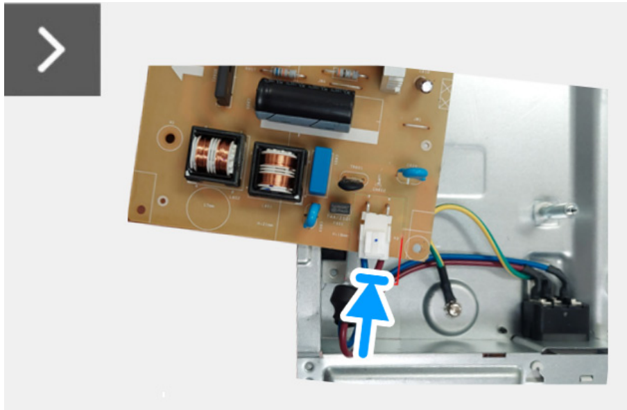
Immagine 24. Installazione della scheda alimentazione
