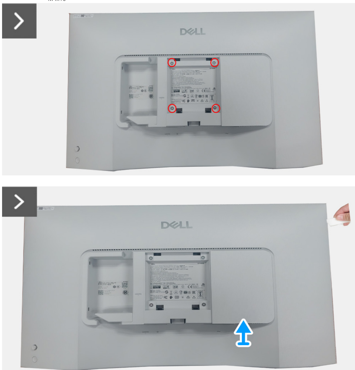
Immagine 11. Rimozione del coperchio posteriore
