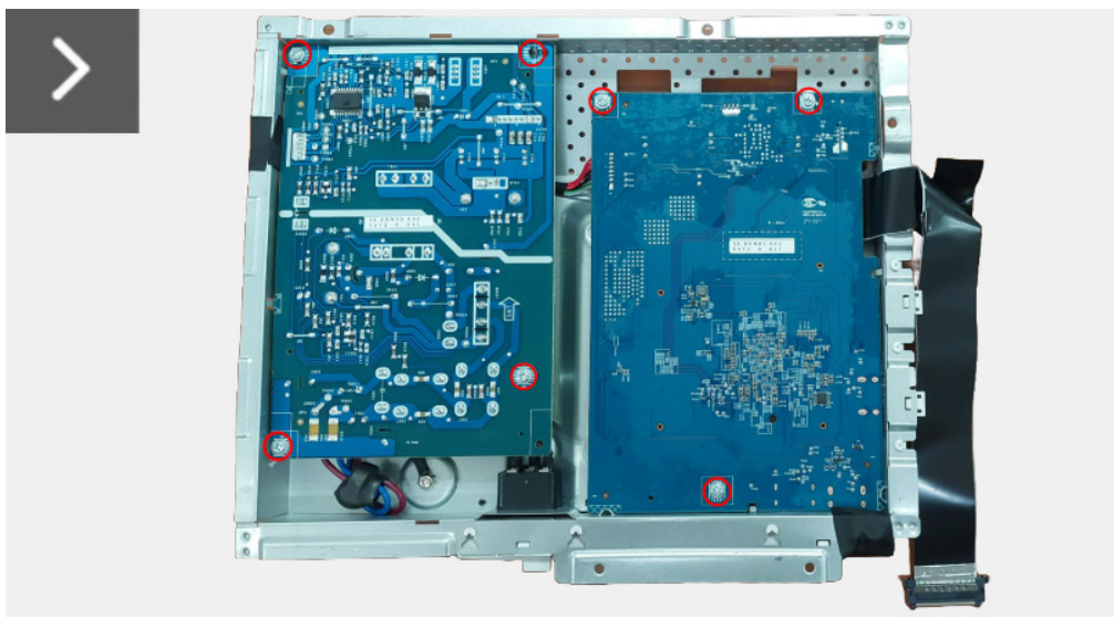
Immagine 21. Installazione della scheda interfaccia
