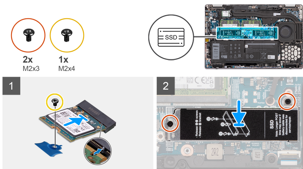
Figura 8. Unità SSD M.2 2230 con relativa staffa
