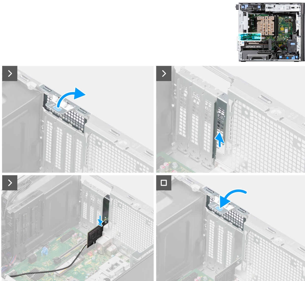
Figura 37. Installazione dell'antenna PCIe esterna
