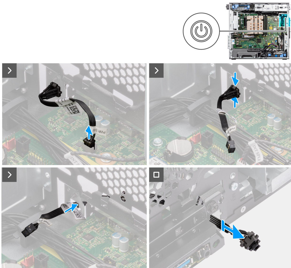
Figura 68. Rimozione del pulsante di accensione
