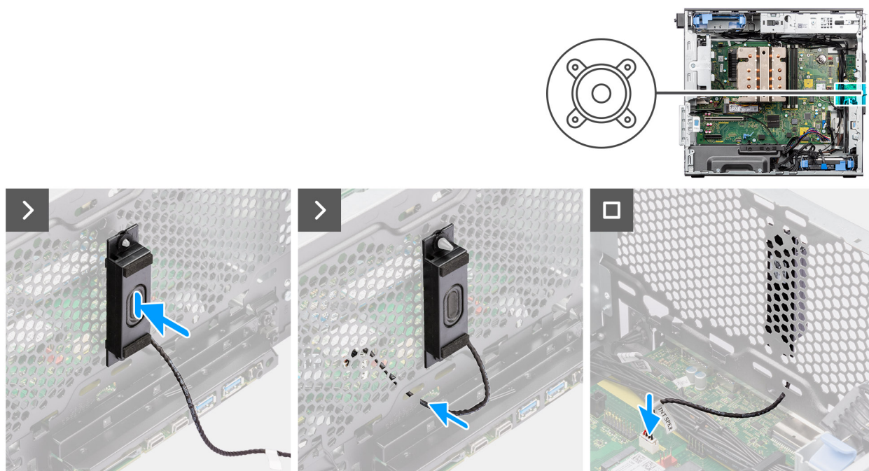
Figura 73. Installazione dell'altoparlante interno
