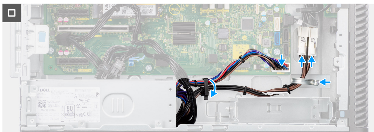
Figura 50. Installazione dell'unità di alimentazione da 1.000 W
