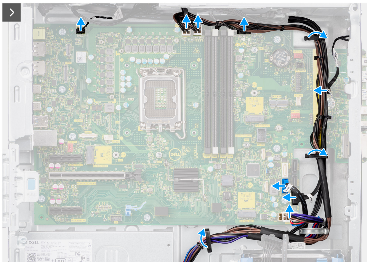
Figura 76. Rimozione della scheda di sistema
