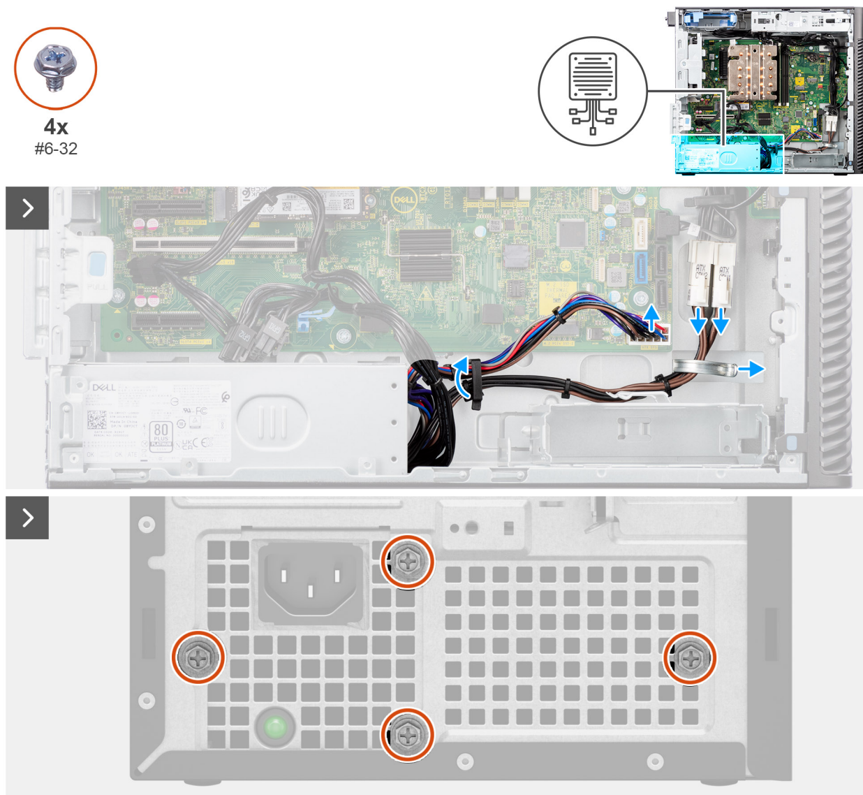
Figura 48. Rimozione dell'unità di alimentazione da 1.000 W
