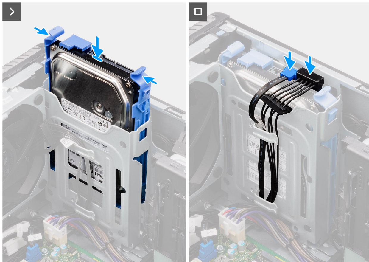
Figura 20. Installazione del gruppo del disco rigido da 3,5 pollici (Bay-2)
