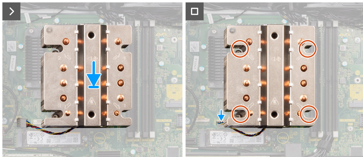
Figura 53. Installazione del gruppo della ventola del processore e del dissipatore di calore a 125 W
