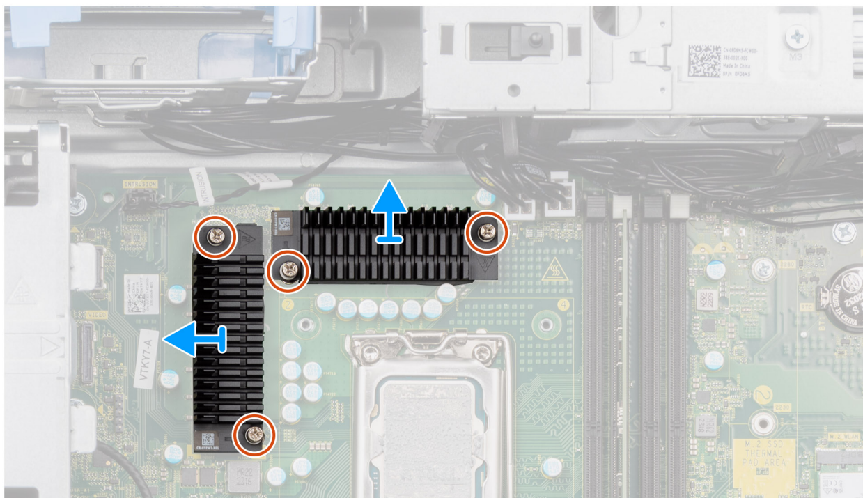
Figura 58. Rimozione del dissipatore di calore VR
