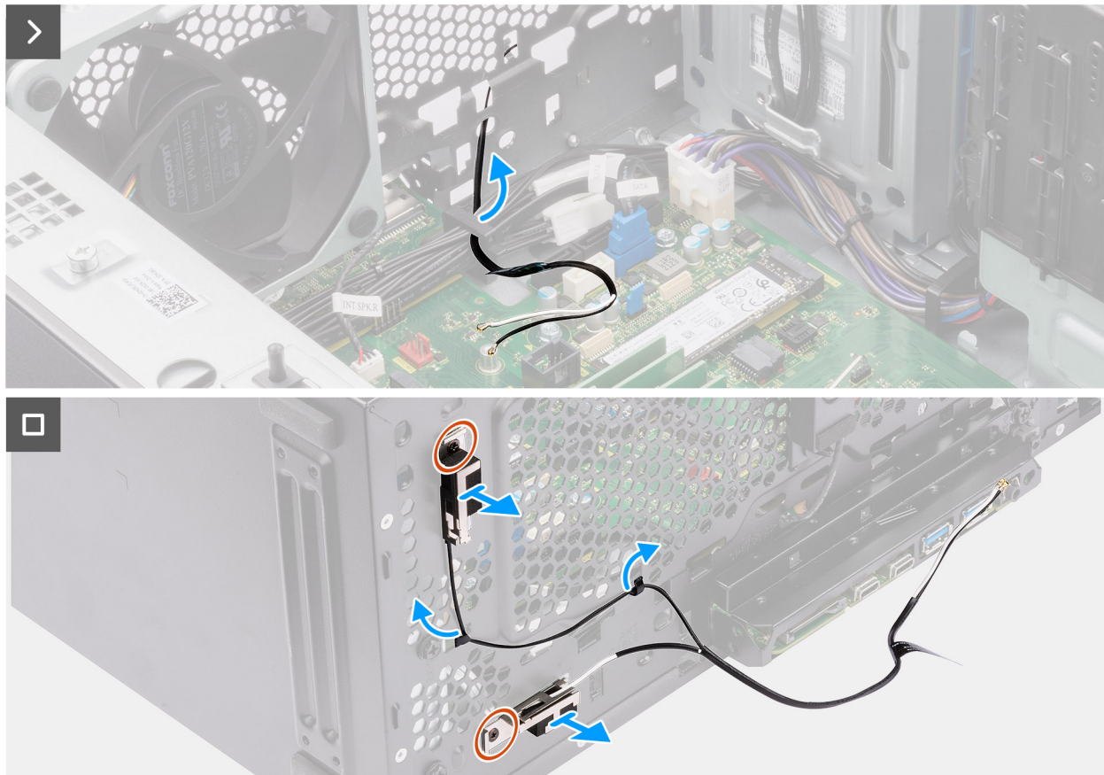
Figura 28. Rimozione dell'antenna WLAN interna
