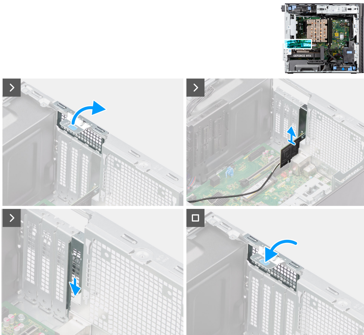
Figura 36. Rimozione dell'antenna PCIe esterna
