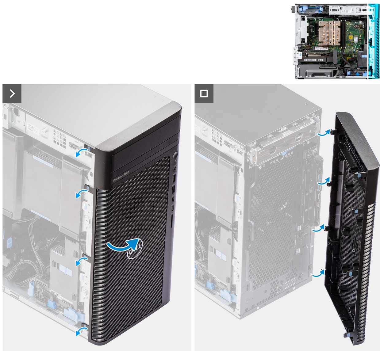
Figura 12. Rimozione del pannello anteriore
