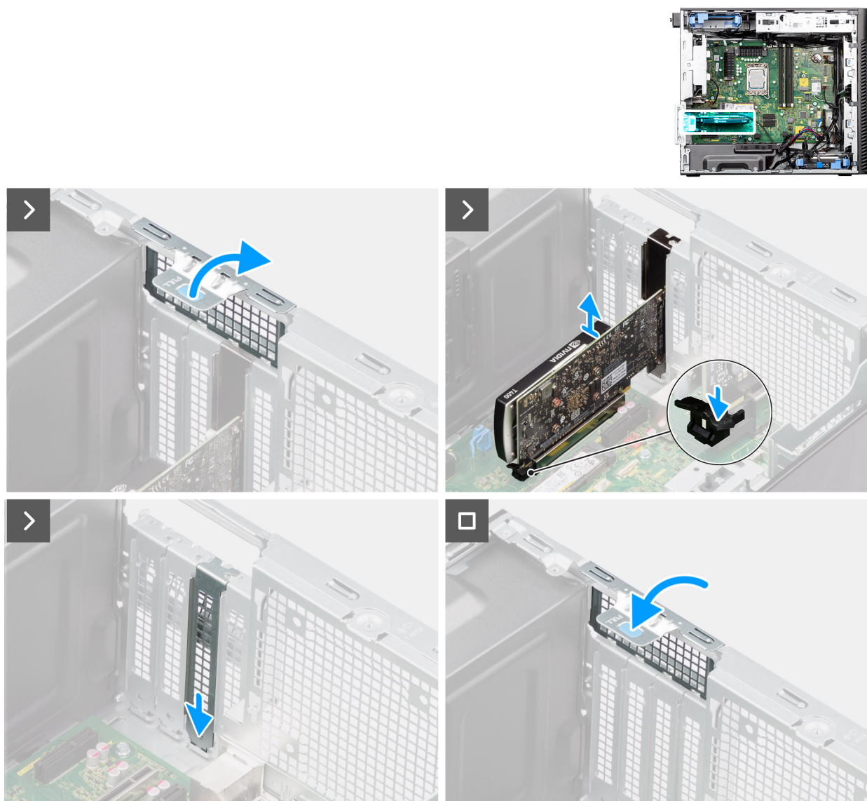
Figura 38. Rimozione della scheda grafica
