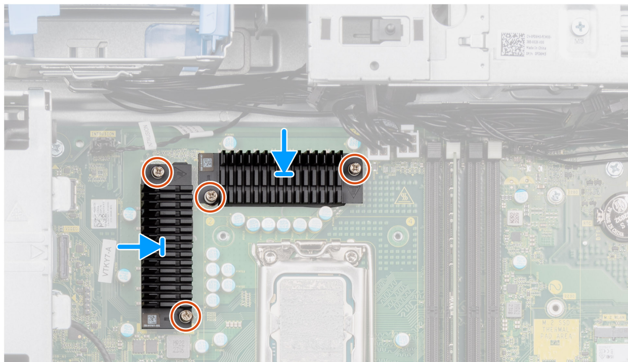
Figura 59. Installazione del dissipatore di calore VR
