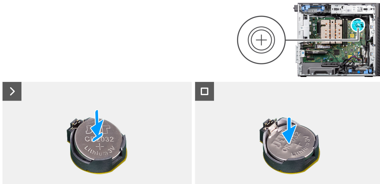
Figura 31. Installazione della batteria a bottone
