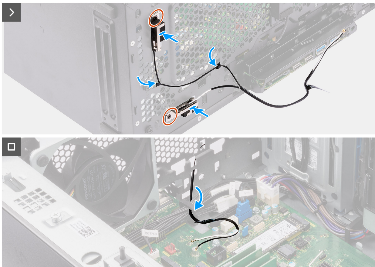
Figura 29. Installazione dell'antenna WLAN interna
