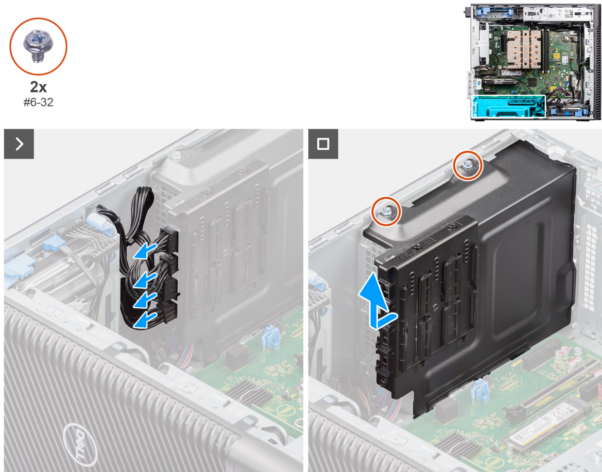
Figura 46. Rimozione del coperchio dell'unità di alimentazione
