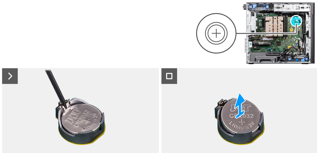
Figura 30. Rimozione della batteria a bottone
