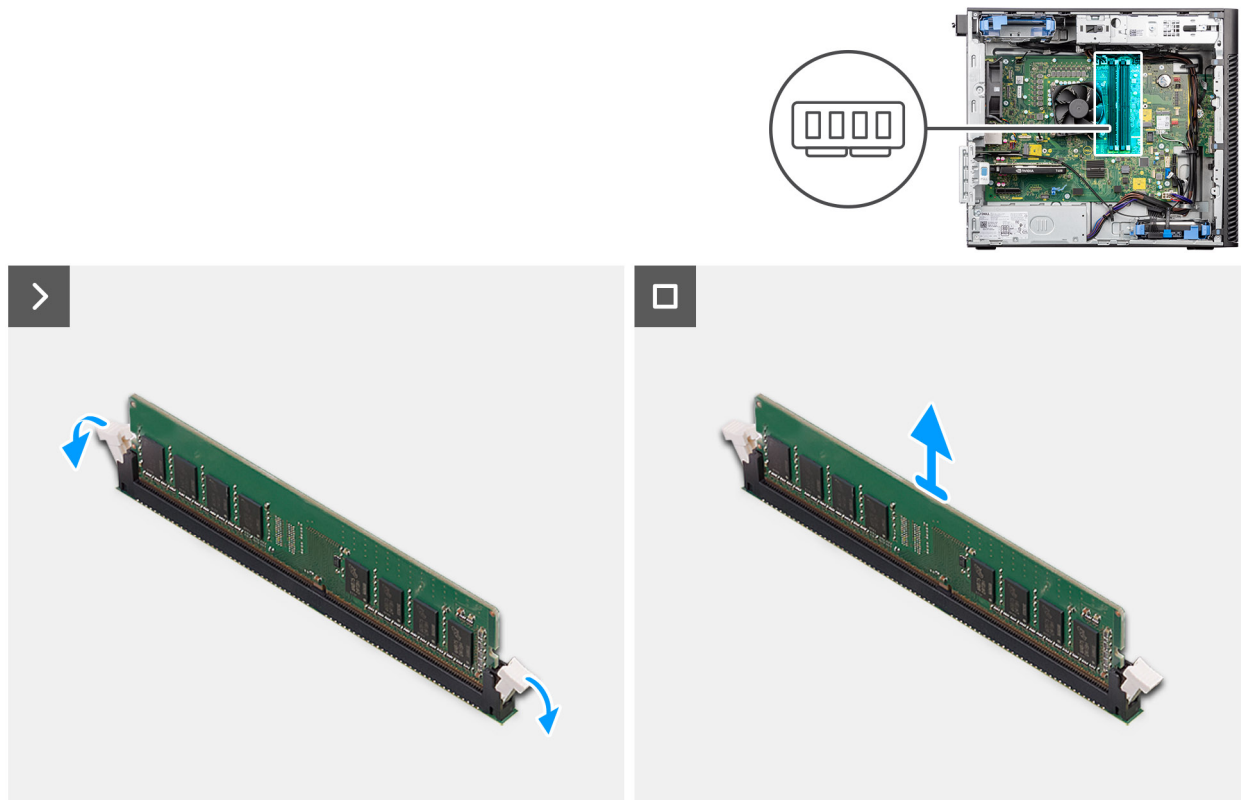
Figura 32. Rimozione del modulo di memoria
