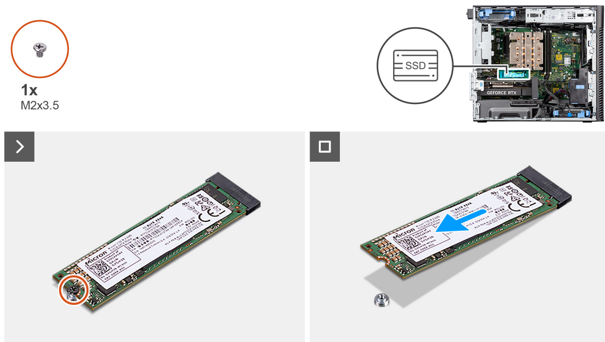
Figura 24. Rimozione dell'unità SSD M.2 2280 PCIe
