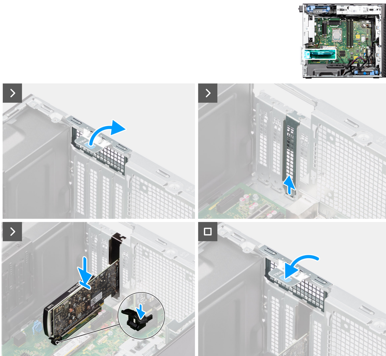
Figura 39. Installazione della scheda grafica
