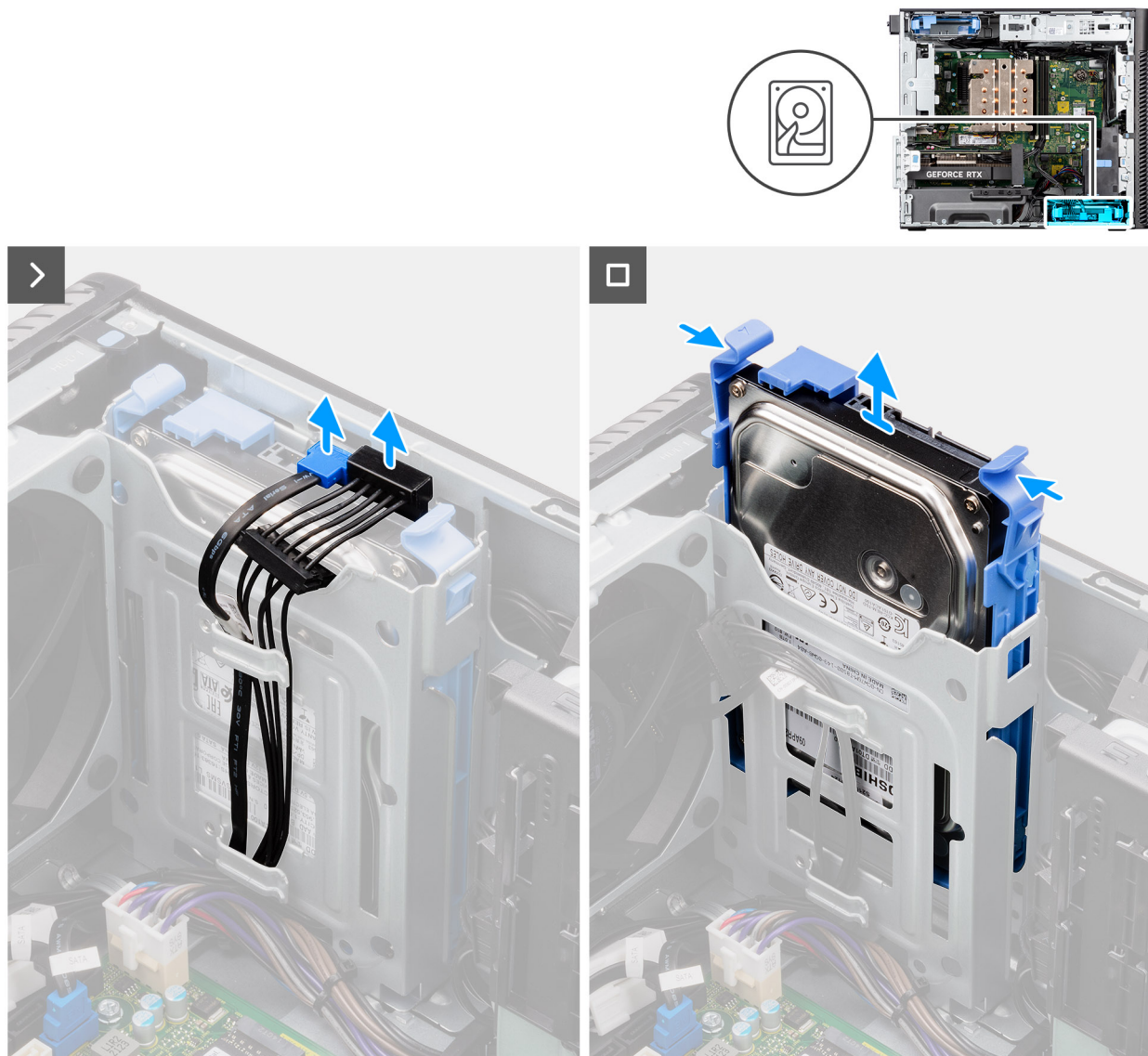
Figura 16. Rimozione del gruppo del disco rigido da 3,5 pollici dall'alloggiamento 1
