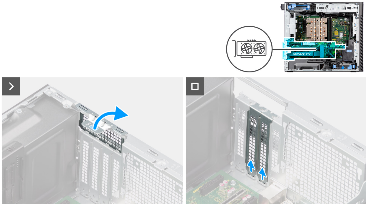
Figura 43. Installazione della GPU alimentata
