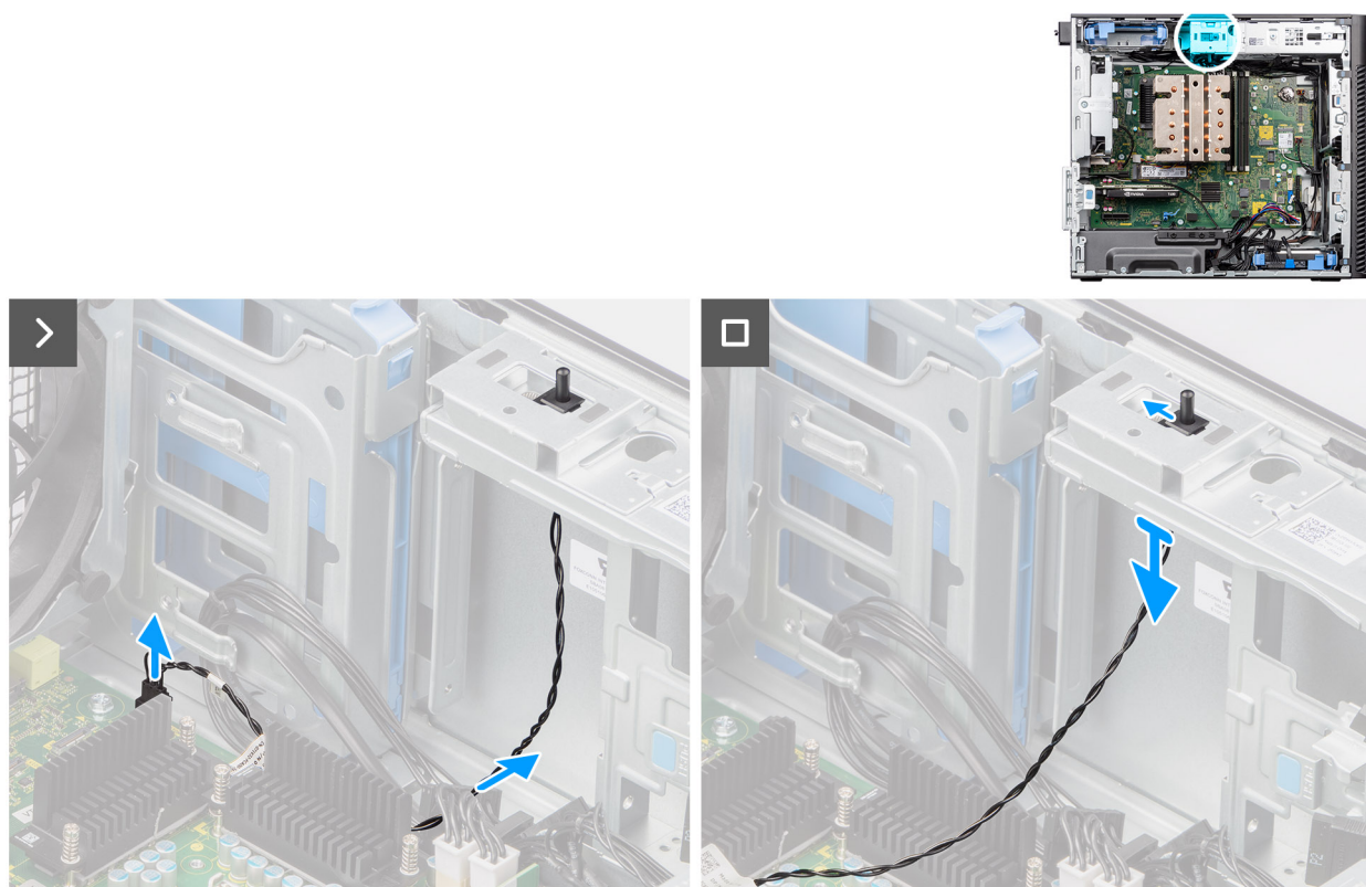
Figura 70. Rimozione dell'interruttore di intrusione
