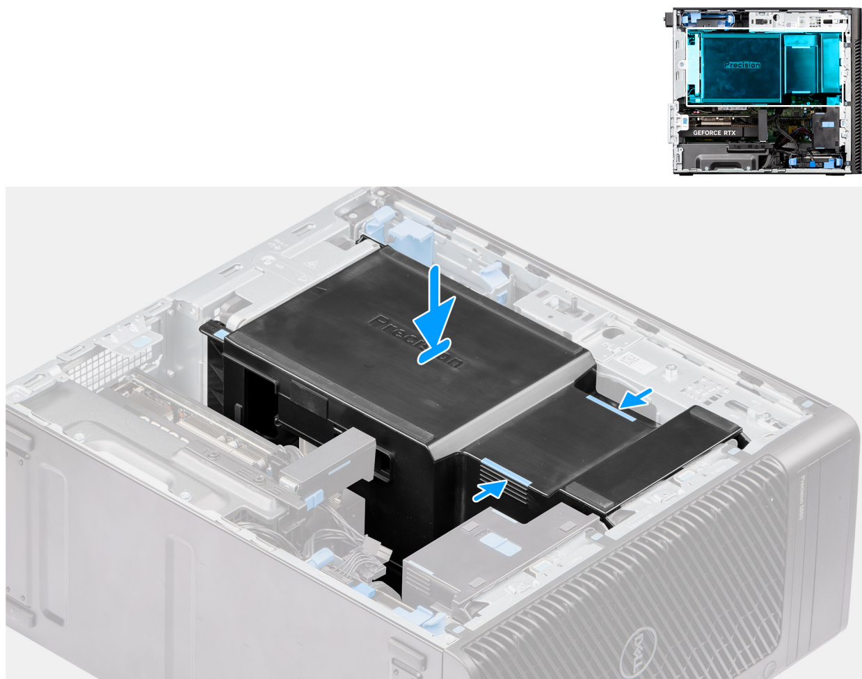
Figura 15. Installazione del manicotto dell'aria
