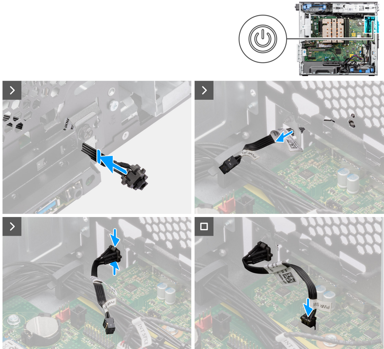
Figura 69. Installazione del pulsante di accensione
