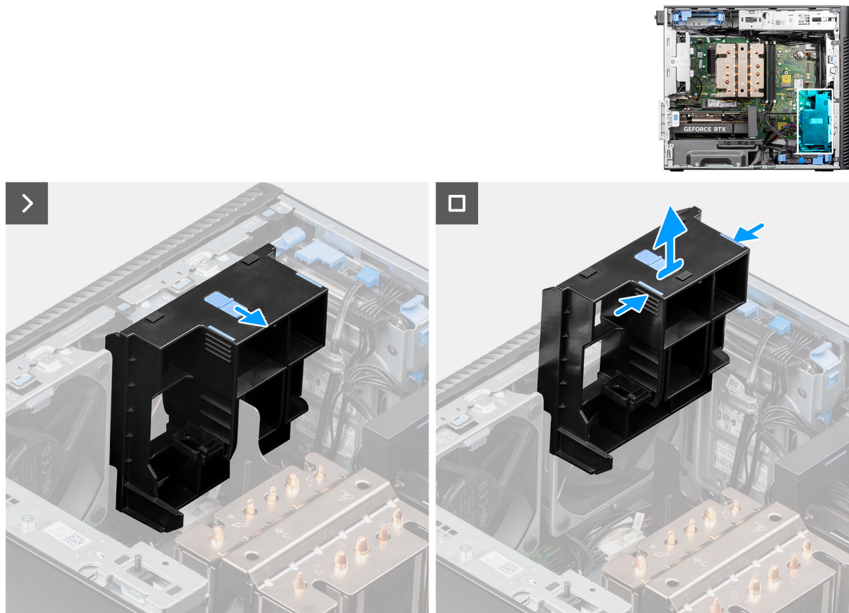
Figura 34. Rimozione del supporto terminale della GPU
