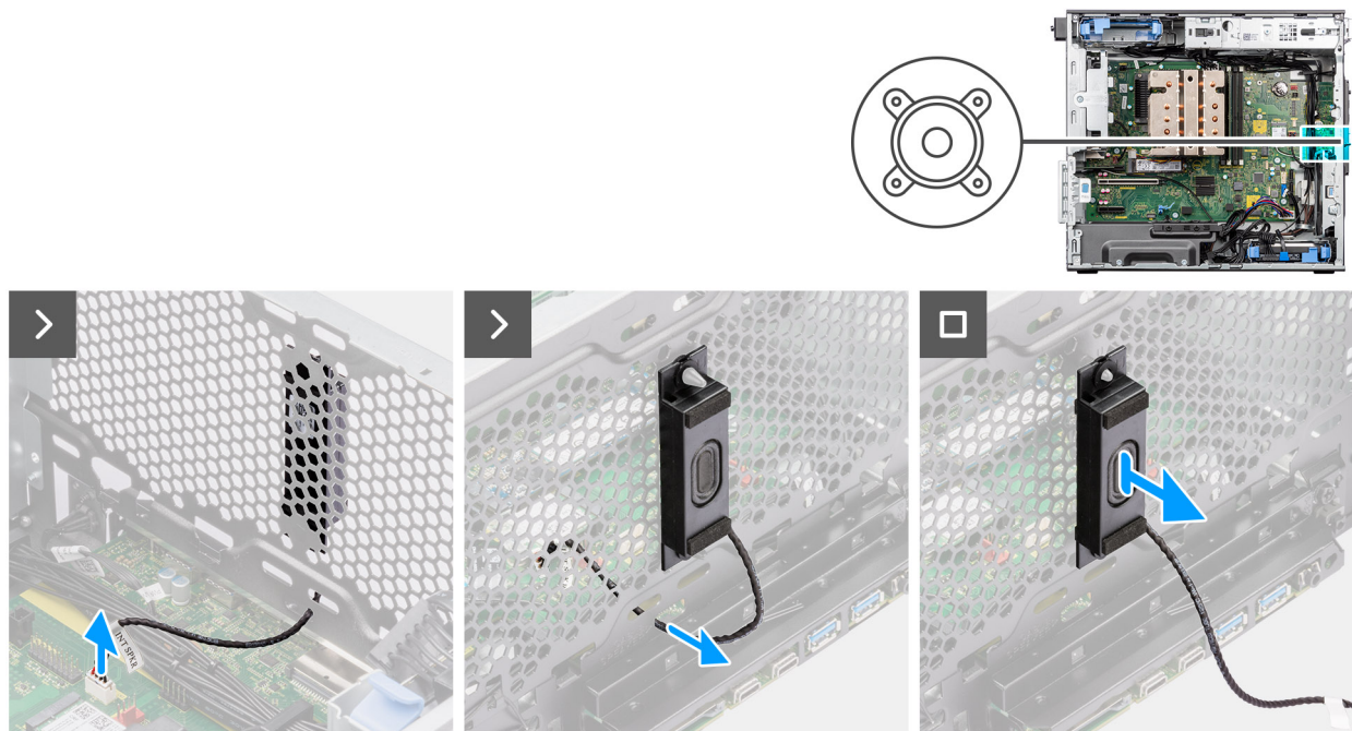
Figura 72. Rimozione dell'altoparlante interno
