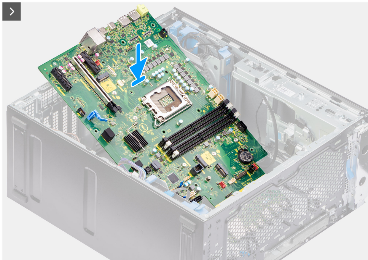
Figura 80. Installazione della scheda di sistema
