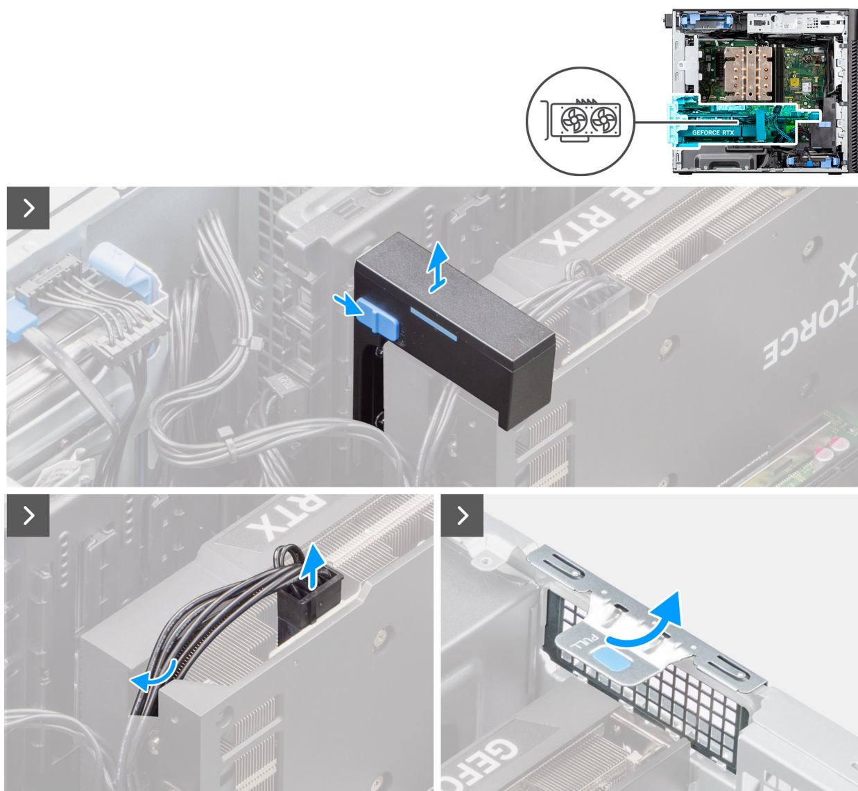
Figura 40. Rimozione della GPU alimentata
