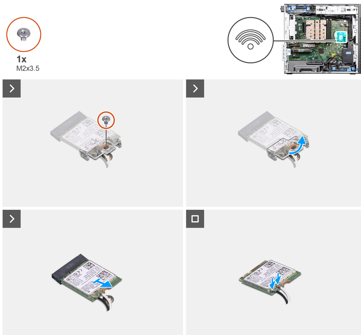
Figura 26. Rimozione della scheda WLAN
