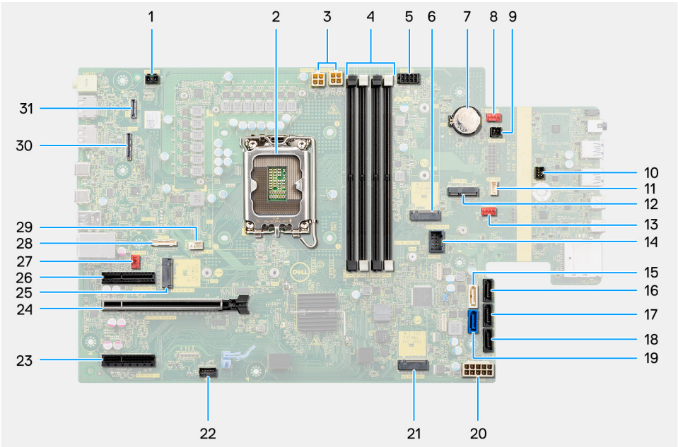
Figura 74. Callout della scheda di sistema
