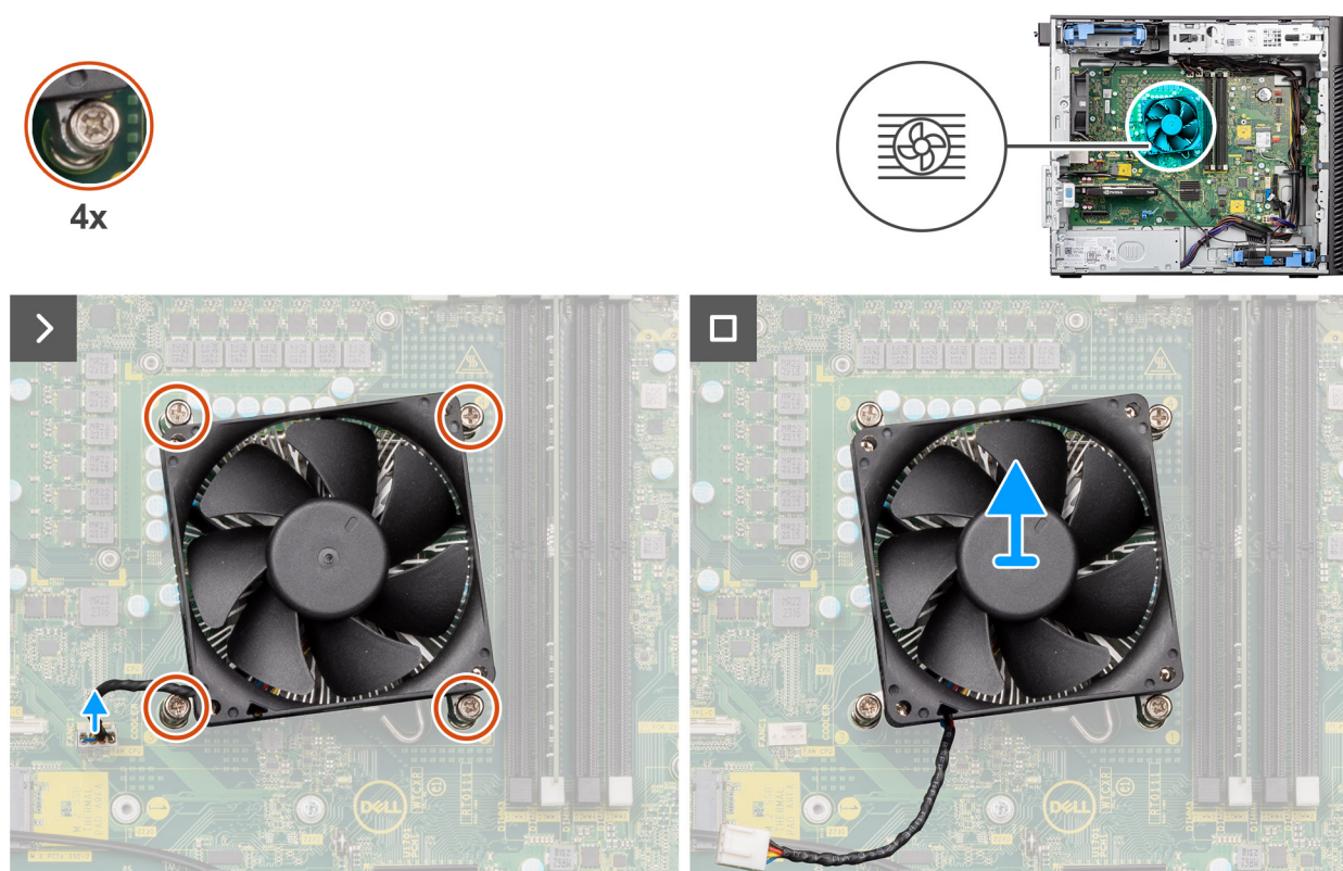
Figura 54. Rimozione del gruppo della ventola del processore e del dissipatore di calore a 65 W
