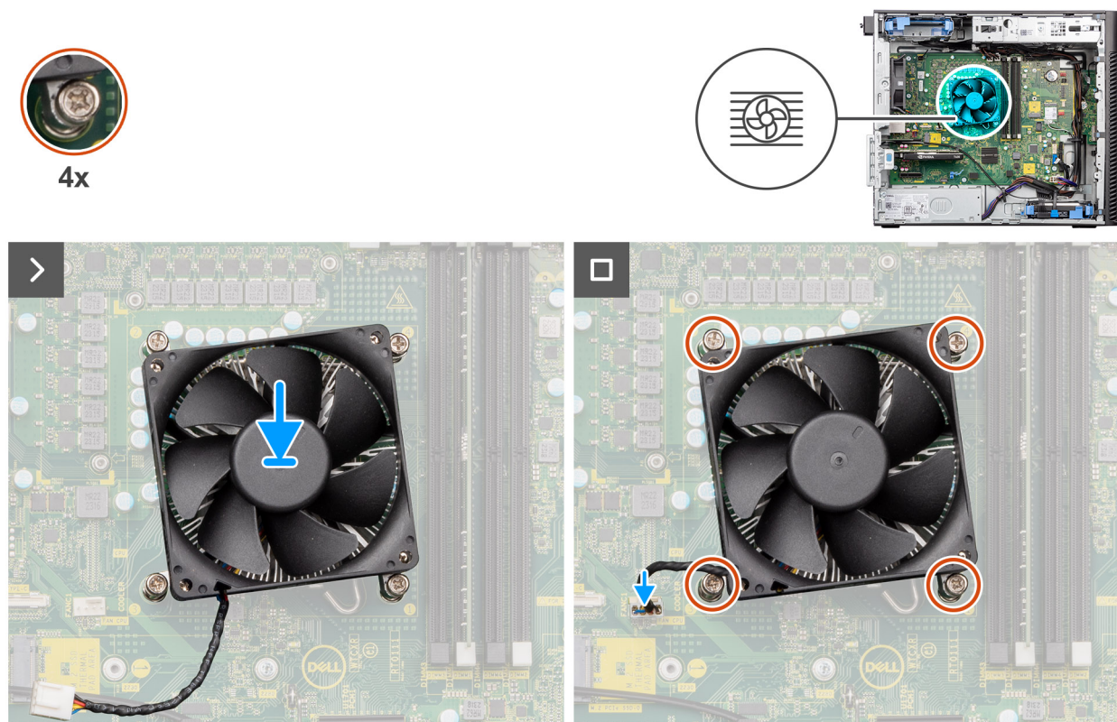
Figura 55. Installazione del gruppo della ventola del processore e del dissipatore di calore a 65 W
