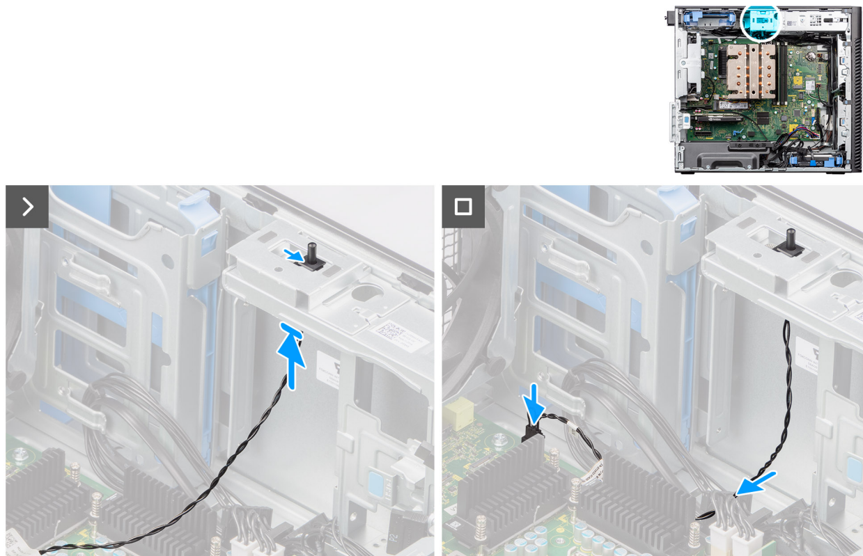
Figura 71. Installazione dell'interruttore di apertura
