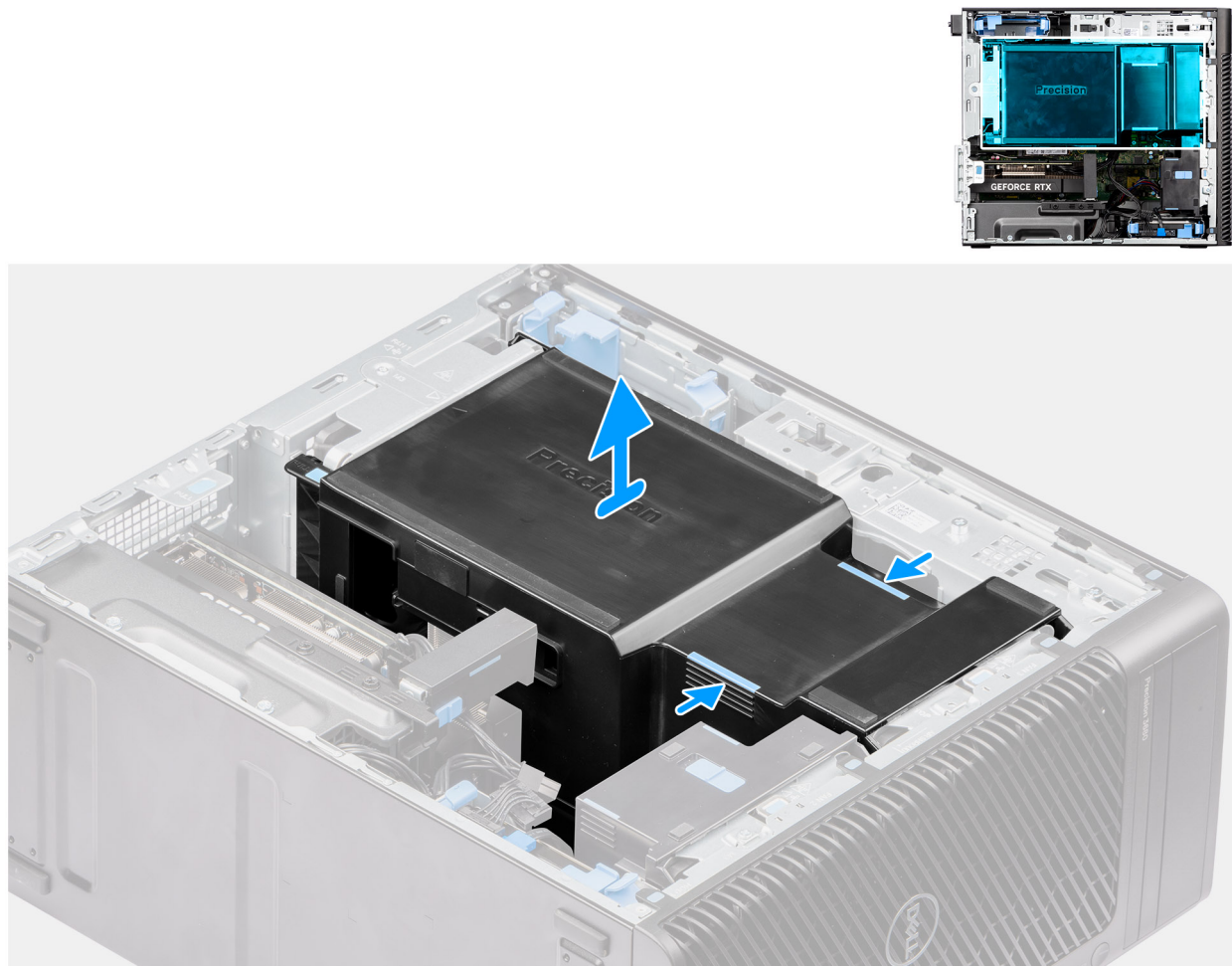
Figura 14. Rimozione del manicotto dell'aria
