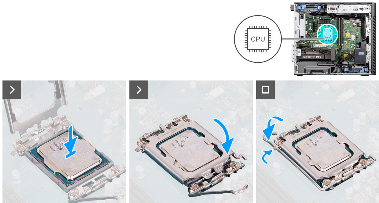
Figura 57. Installazione del processore
