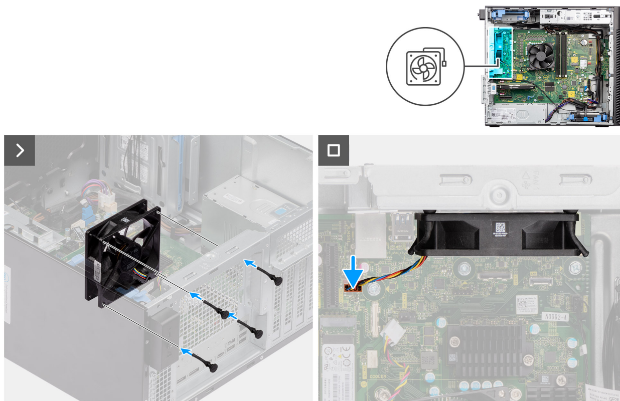
Figura 65. Installazione della ventola posteriore per sistemi PSU da 300 W
