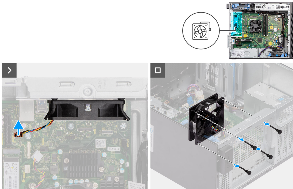
Figura 64. Rimozione della ventola posteriore per sistemi PSU da 300 W
