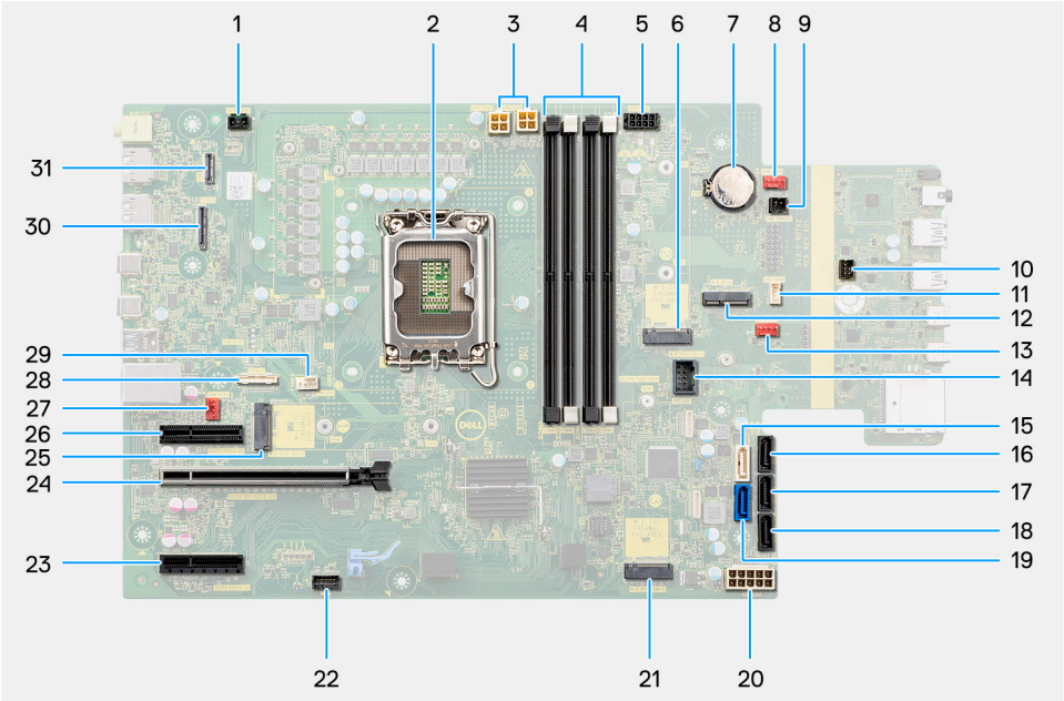
Figura 79. Callout della scheda di sistema
