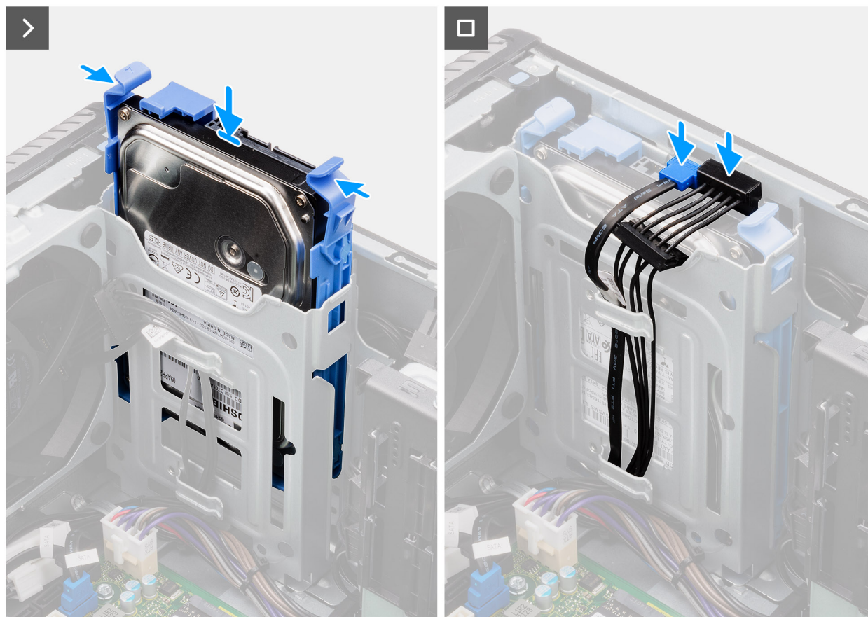
Figura 21. Installazione del gruppo del disco rigido da 3,5 pollici dall'alloggiamento 1
