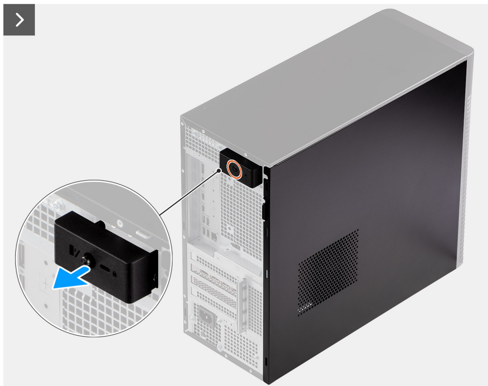
Figura 8. Rimozione del coperchio laterale
