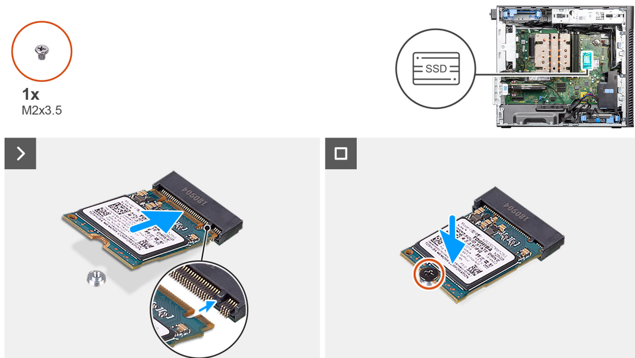
Figura 23. Installazione dell'unità SSD PCIe M.2 2230
