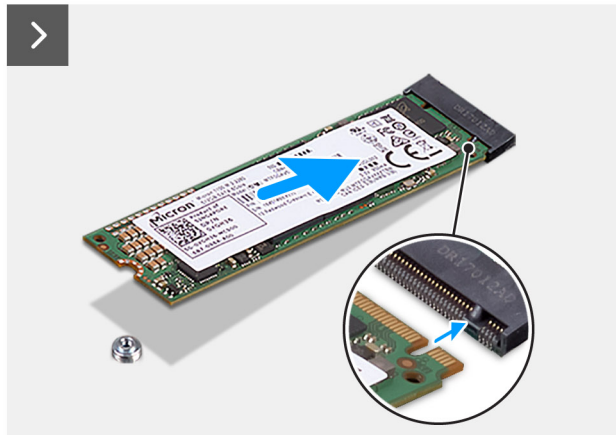
Figura 25. Installazione dell'unità SSD PCIe M.2 2280
