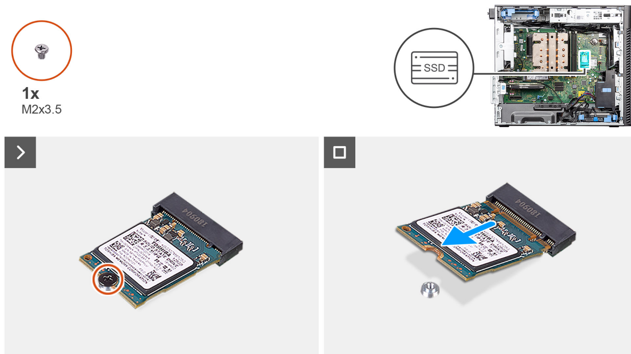
Figura 22. Rimozione dell'unità SSD M.2 2230 PCIe
