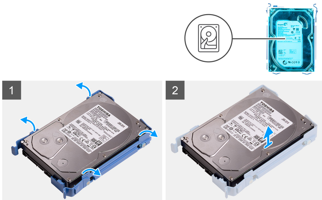
Figura 18. Rimozione della staffa dell'unità del disco rigido da 3,5 pollici
