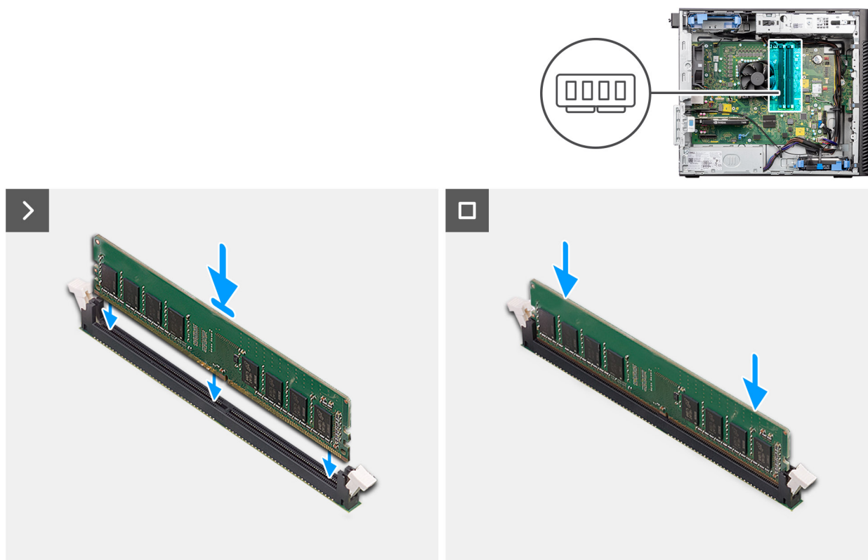
Figura 33. Installazione del modulo di memoria
