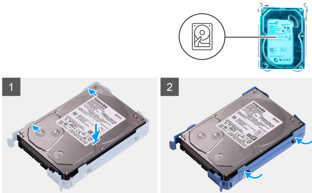
Figura 19. Installazione della staffa del disco rigido da 3,5 pollici
