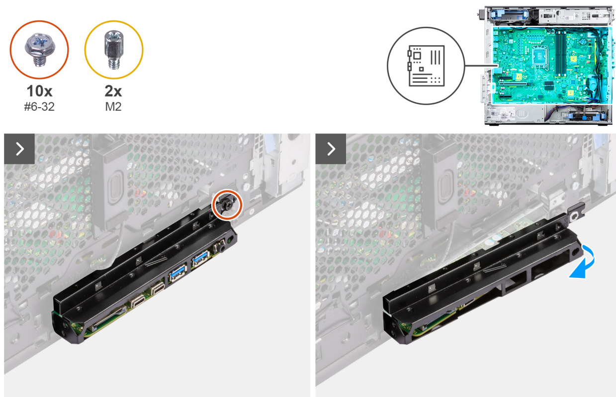
Figura 75. Rimozione della scheda di sistema
