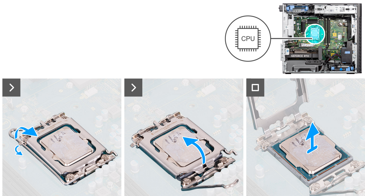
Figura 56. Rimozione del processore
