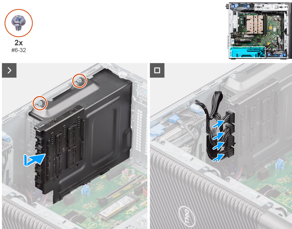
Figura 47. Installazione dell'unità di alimentazione (PSU)
