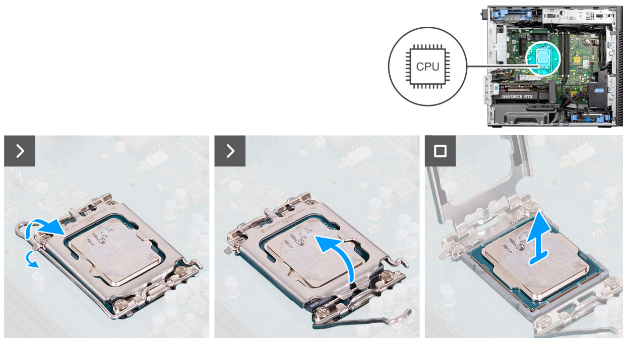
Figura 56. Rimozione del processore
