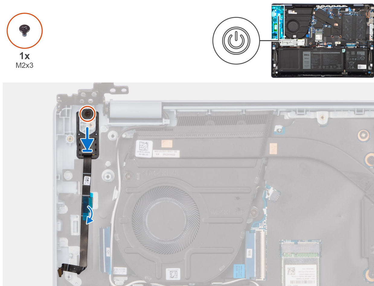
Figura 57. Installazione del pulsante di accensione con lettore di impronte digitali
