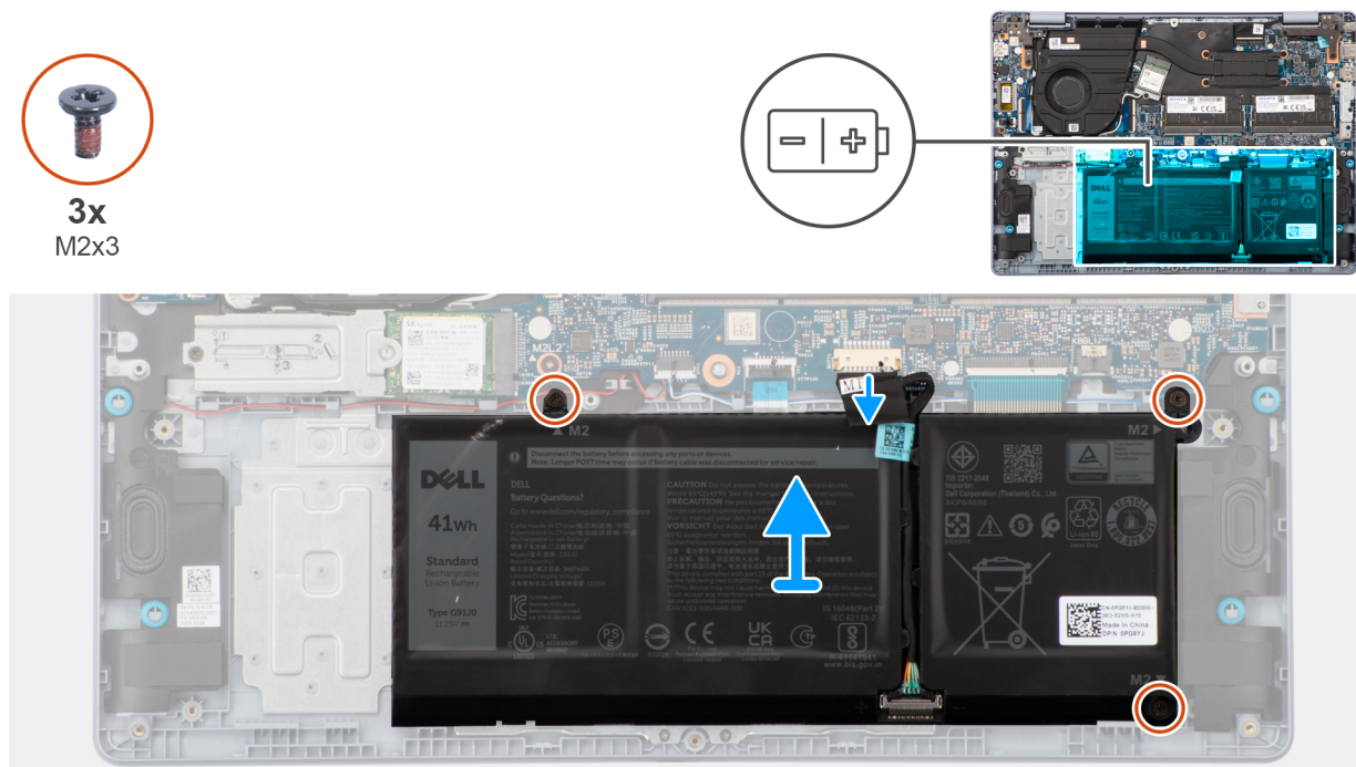
Figura 20. Rimozione della batteria
