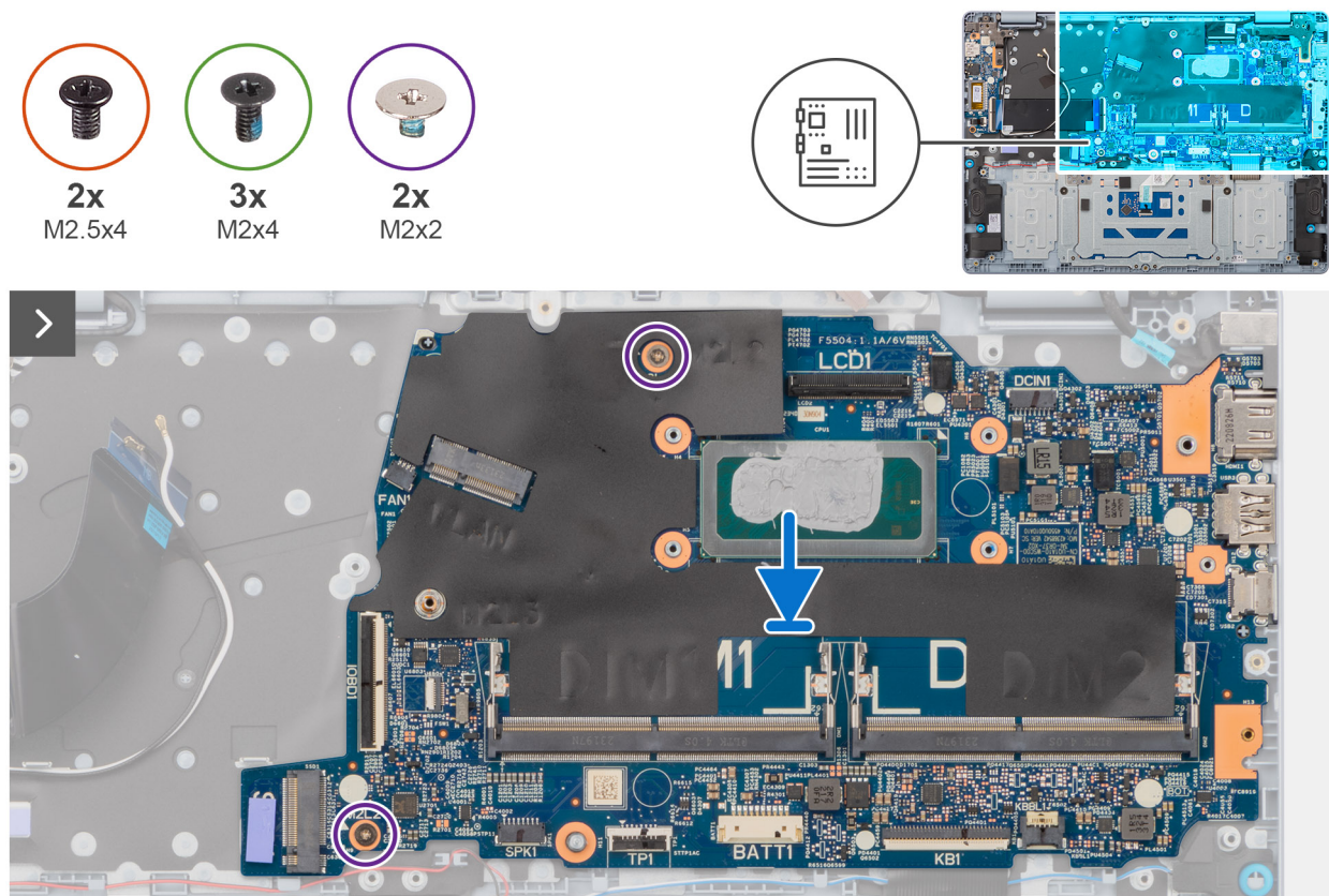
Figura 96. Installazione della scheda di sistema
