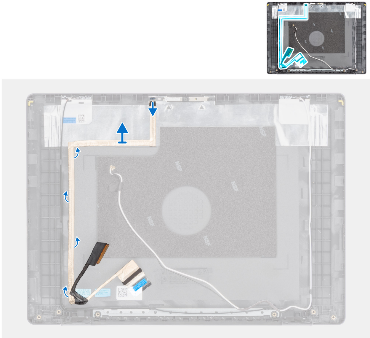
Figura 85. Rimozione del cavo del display
