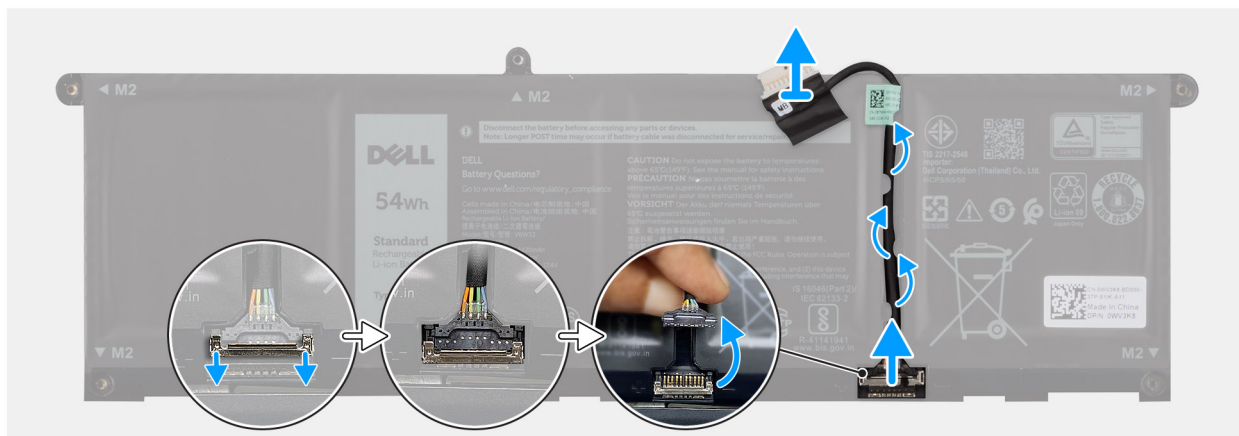
Figura 26. Scollegamento del cavo della batteria
