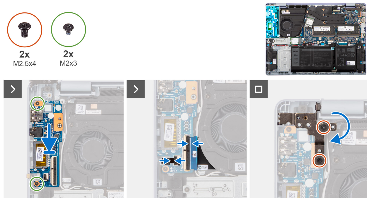
Figura 51. Installazione della scheda di I/O
