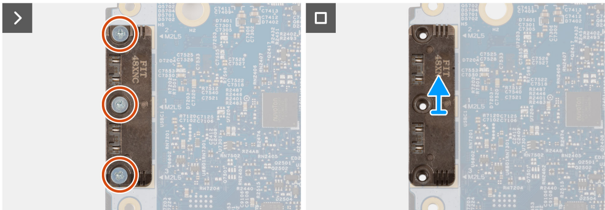
Figura 77. Rimozione del modulo USB Type-C
