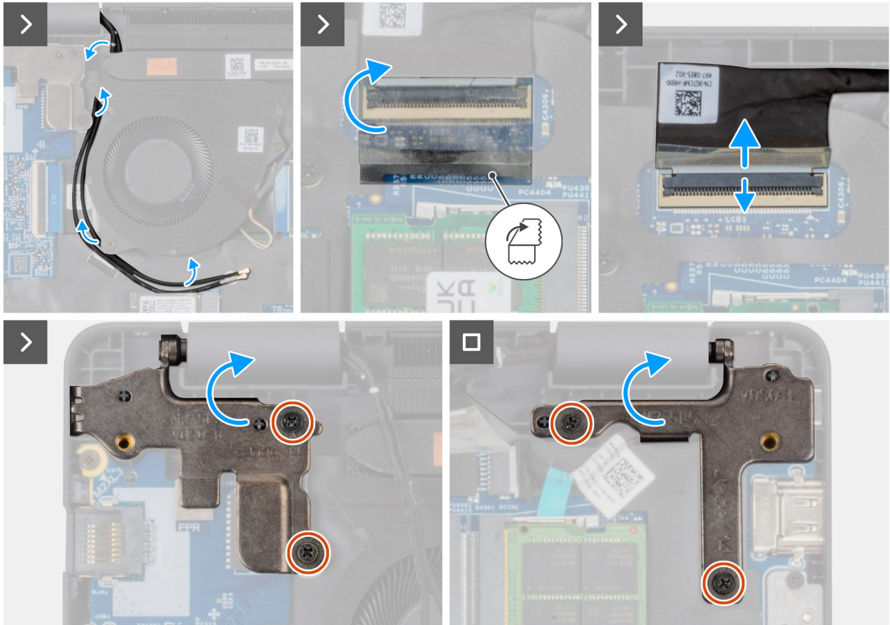
Figura 99. Rimozione del gruppo del display
