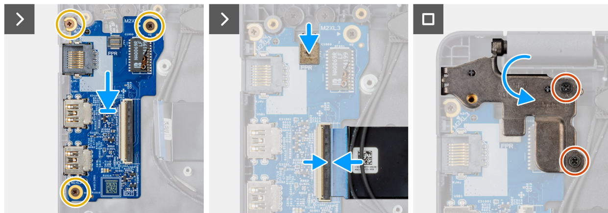
Figura 50. Installazione della scheda di I/O
