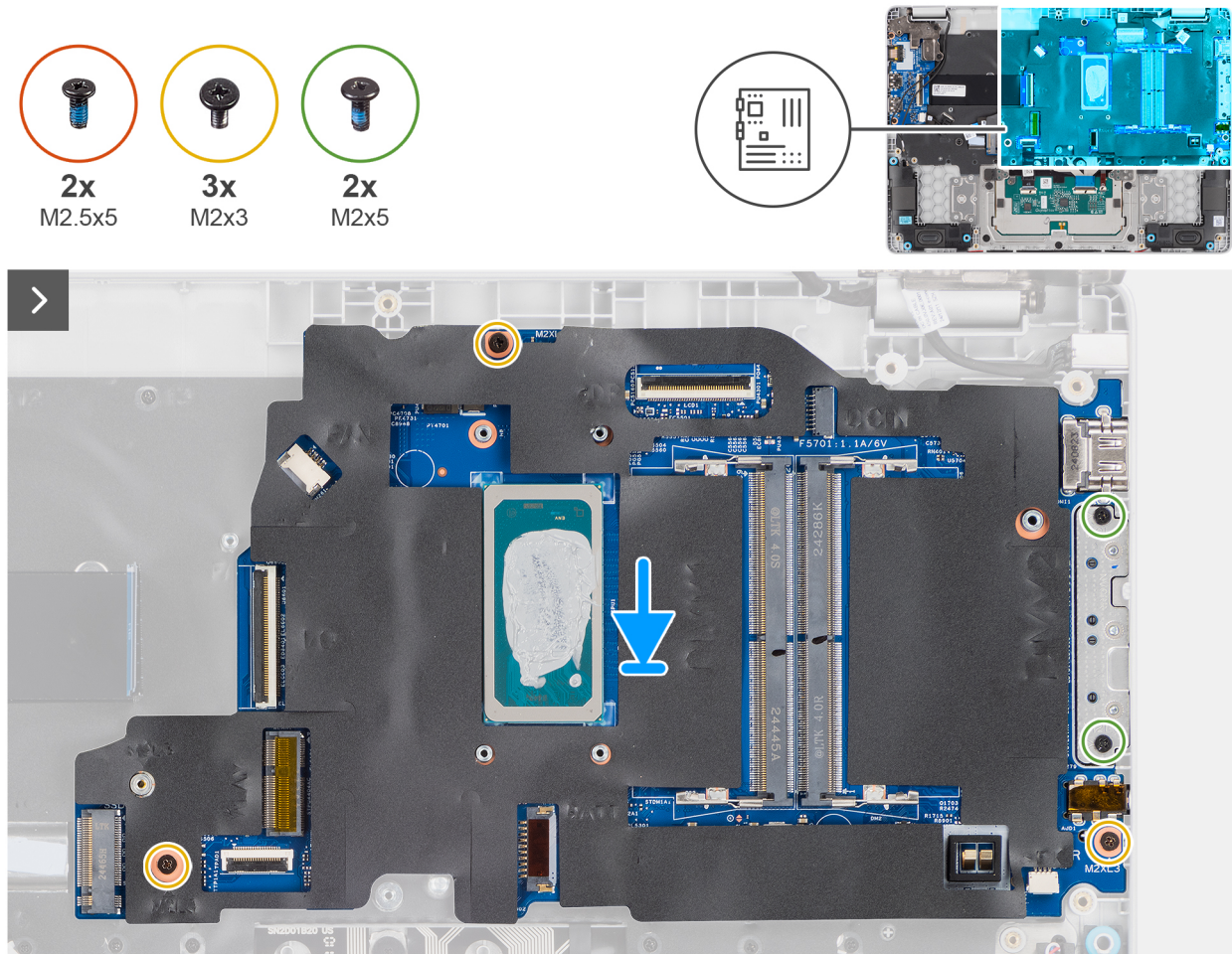
Figura 67. Installazione della scheda di sistema
