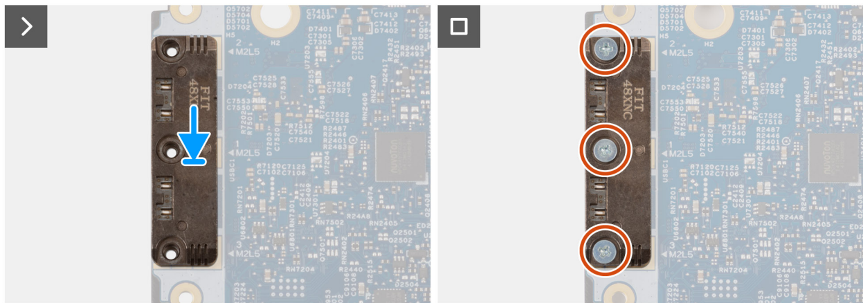
Figura 78. Installazione del modulo USB Type-C
