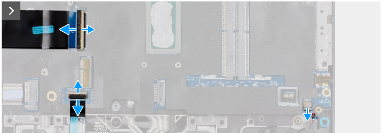
Figura 58. Rimozione della scheda di sistema
