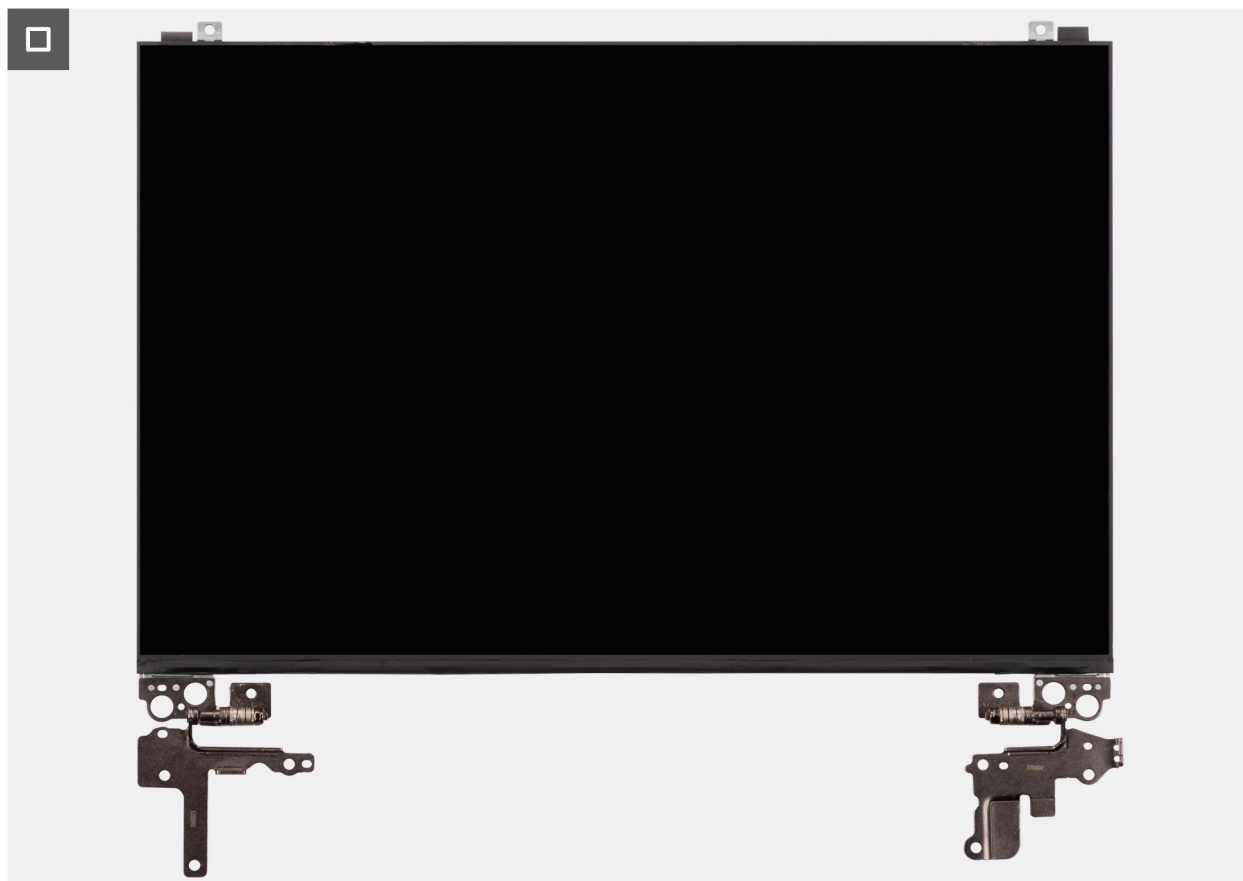
Figura 114. Rimozione del gruppo del pannello del display
