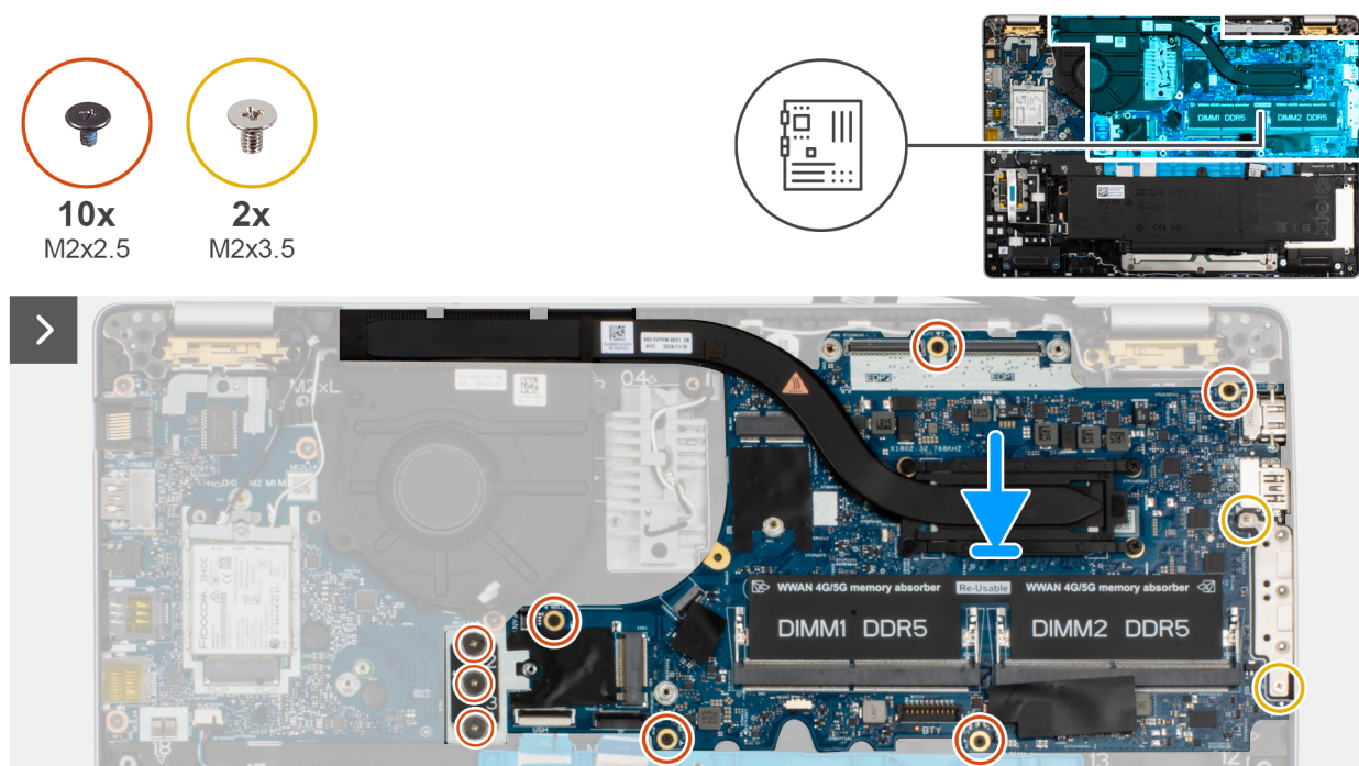
Figura 53. Installazione della scheda di sistema
