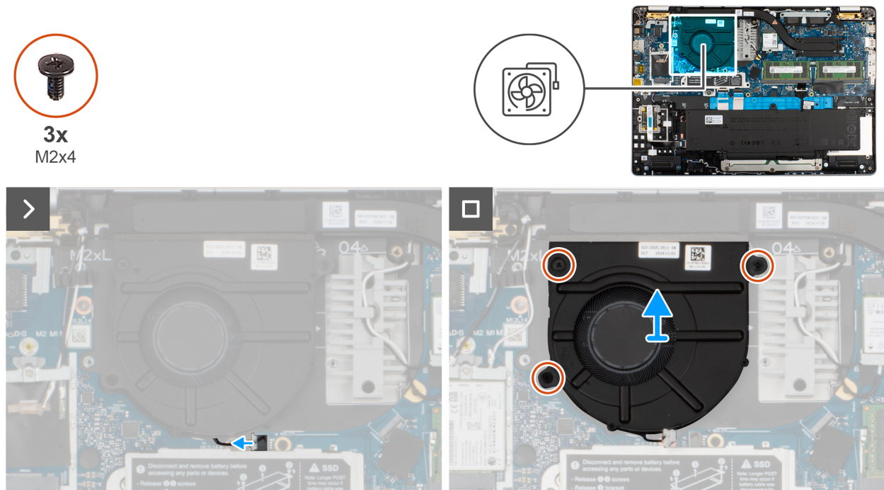
Figura 35. Rimozione della ventola
