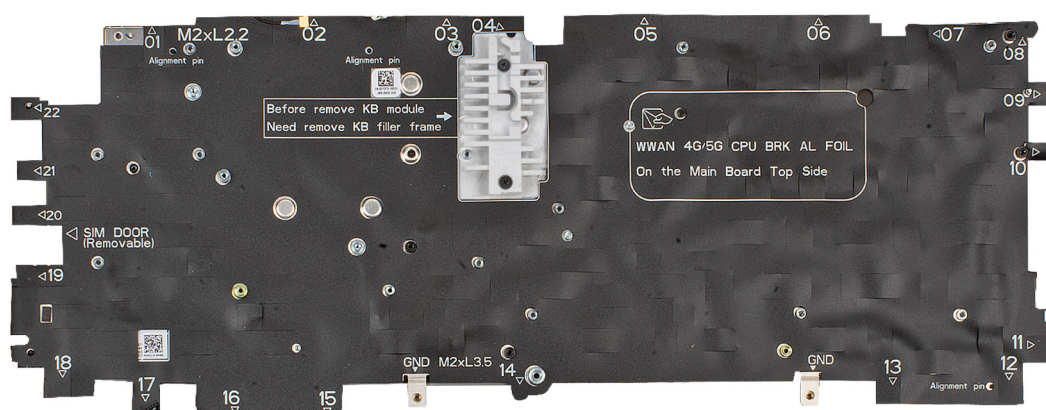
Figura 86. Installazione del riempimento della tastiera
