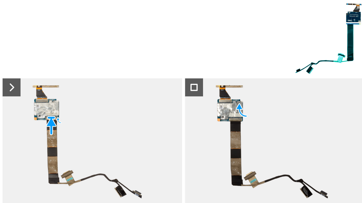
Figura 74. Installazione del cavo del display
