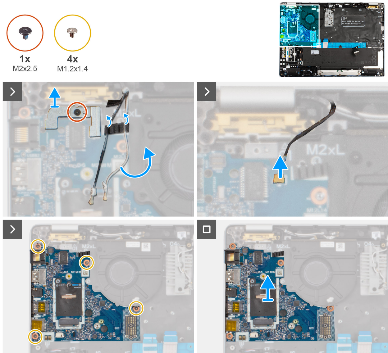
Figura 55. Rimozione della scheda di I/O
