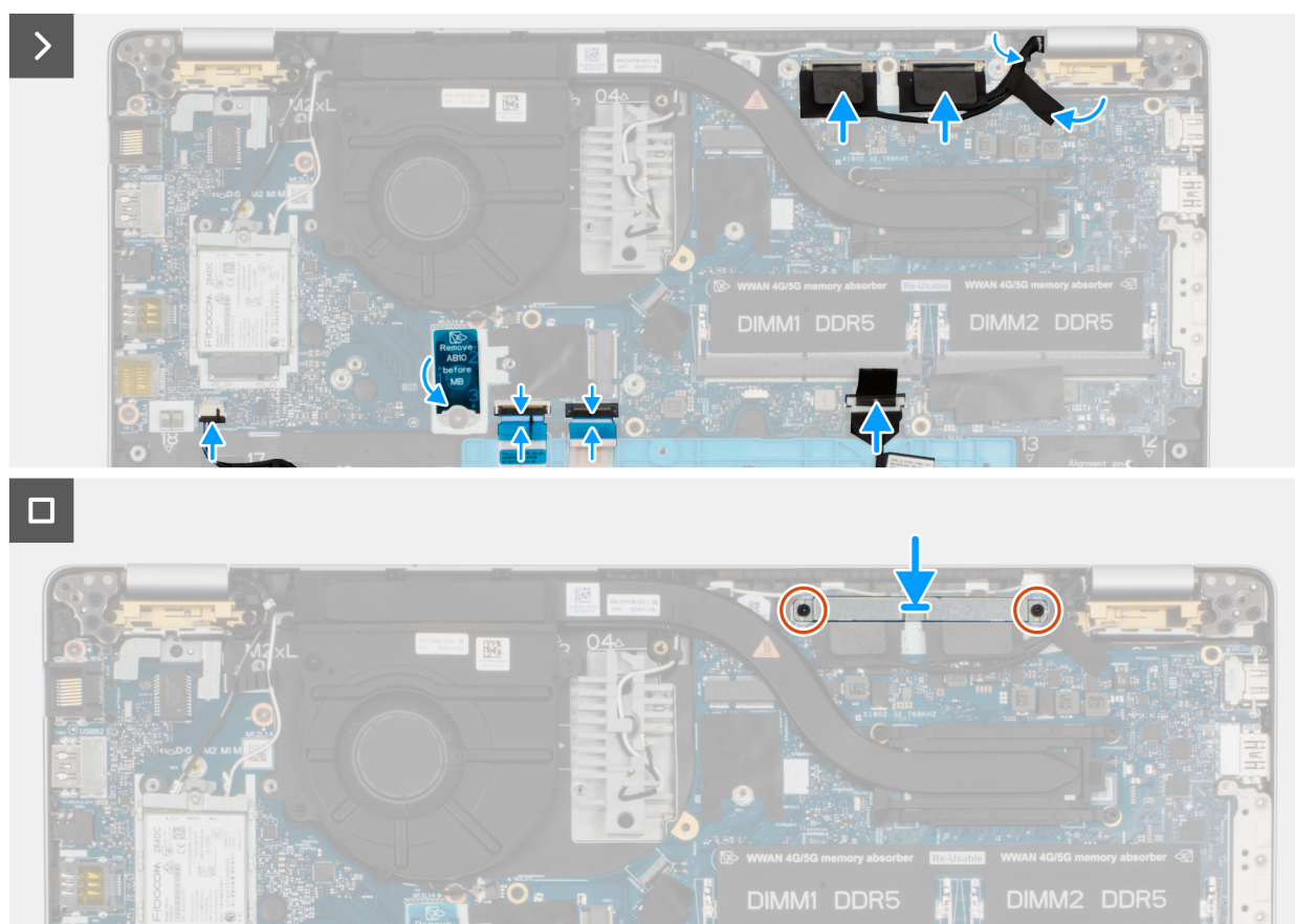
Figura 54. Installazione della scheda di sistema
