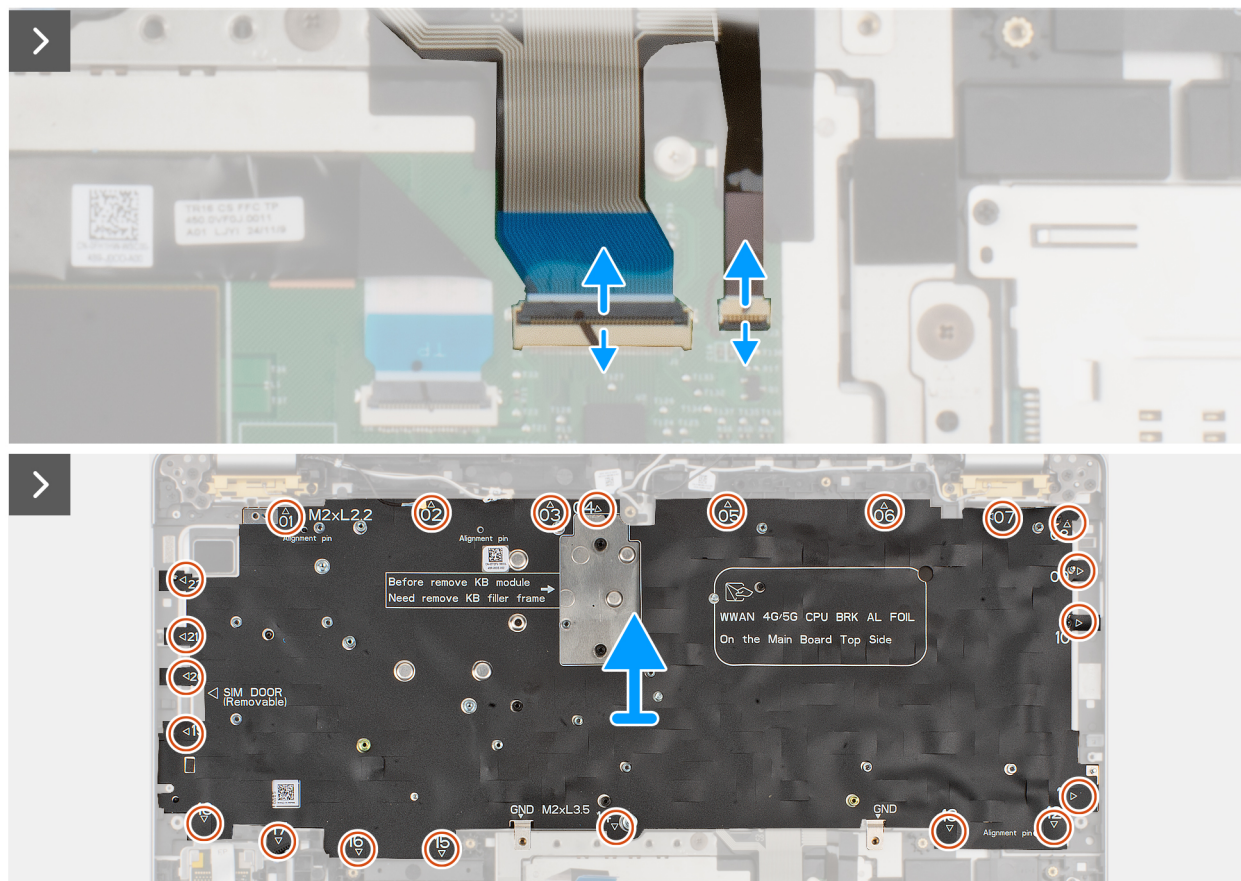
Figura 81. Rimozione della tastiera
