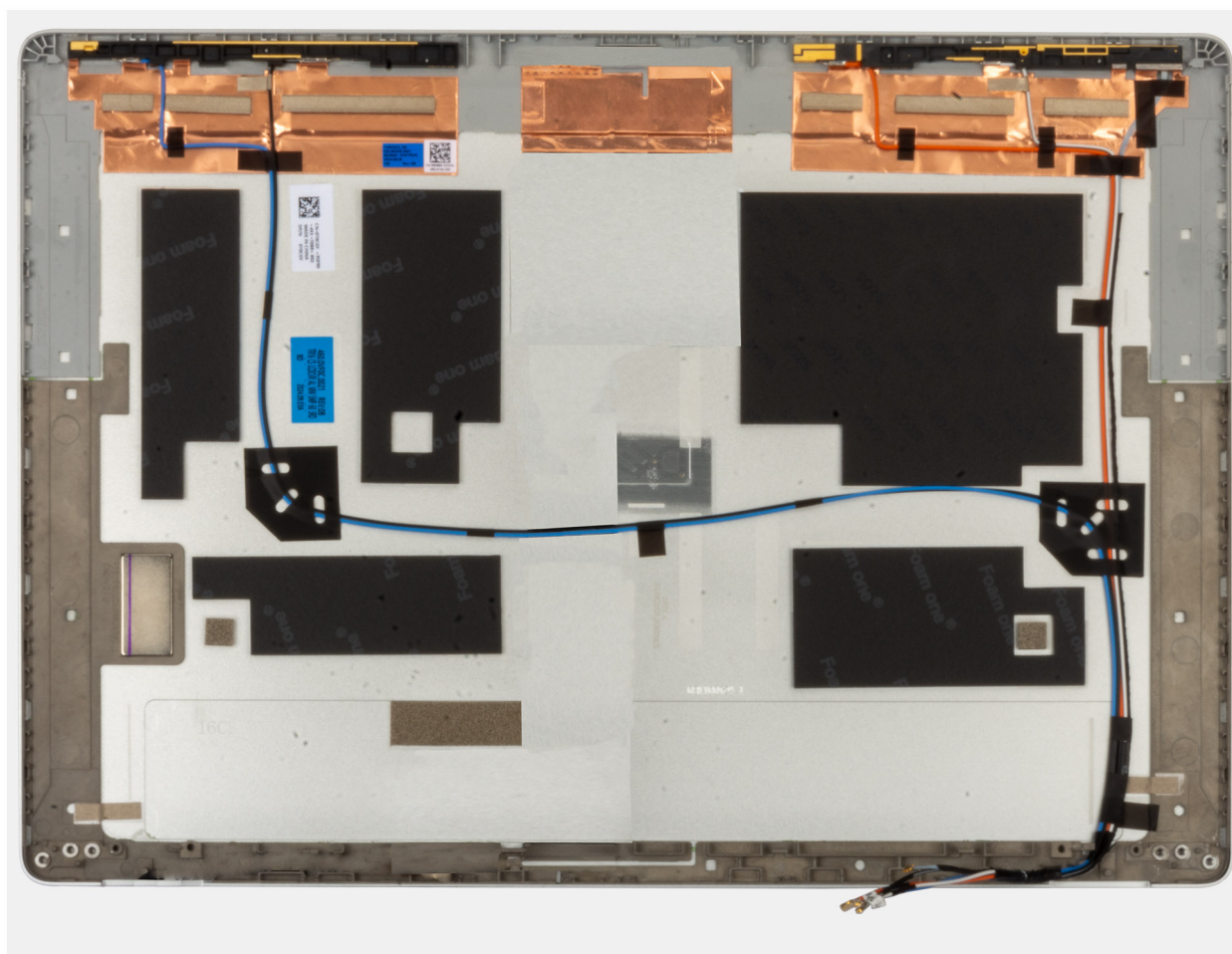
Figura 77. Rimozione del coperchio posteriore del display
