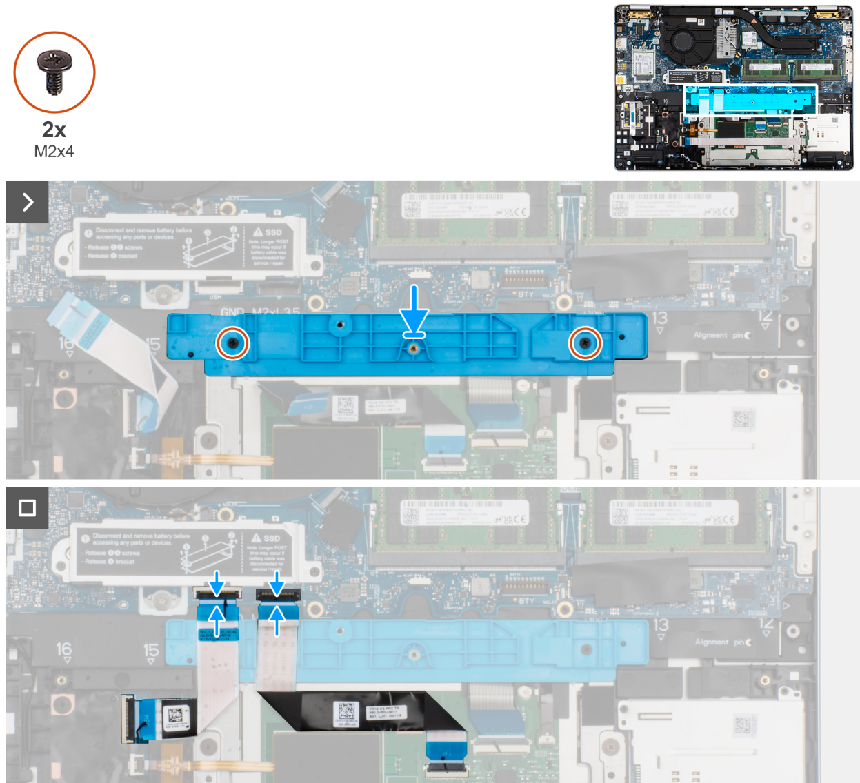
Figura 46. Installazione della staffa di supporto della batteria
