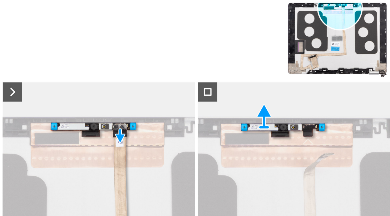
Figura 75. Rimozione del modulo della fotocamera
