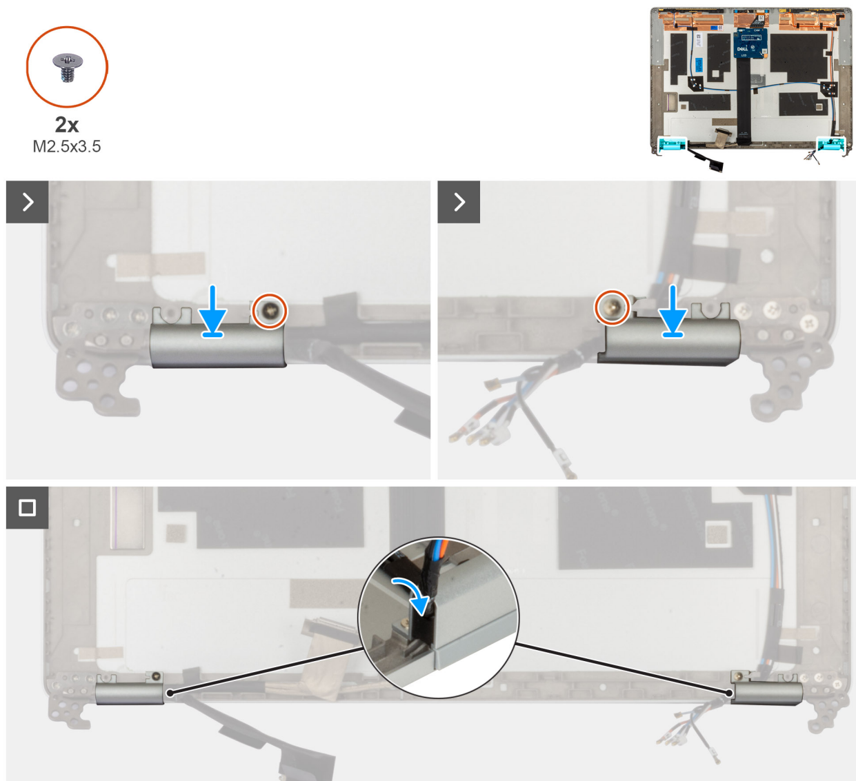
Figura 72. Installazione del tappo dei cardini del display
