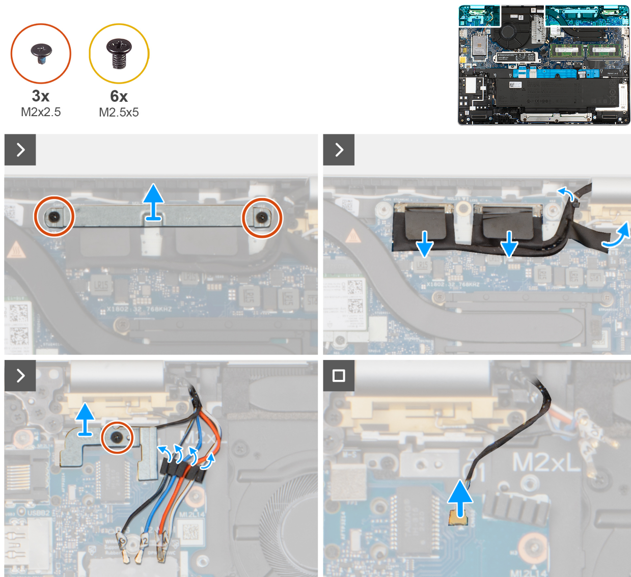
Figura 58. Rimozione del gruppo del display
