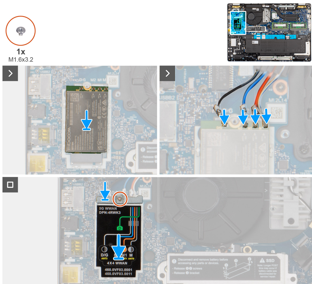
Figura 32. Installazione della scheda WWAN 5G
