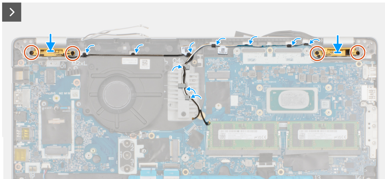
Figura 43. Installazione dell'antenna WLAN
