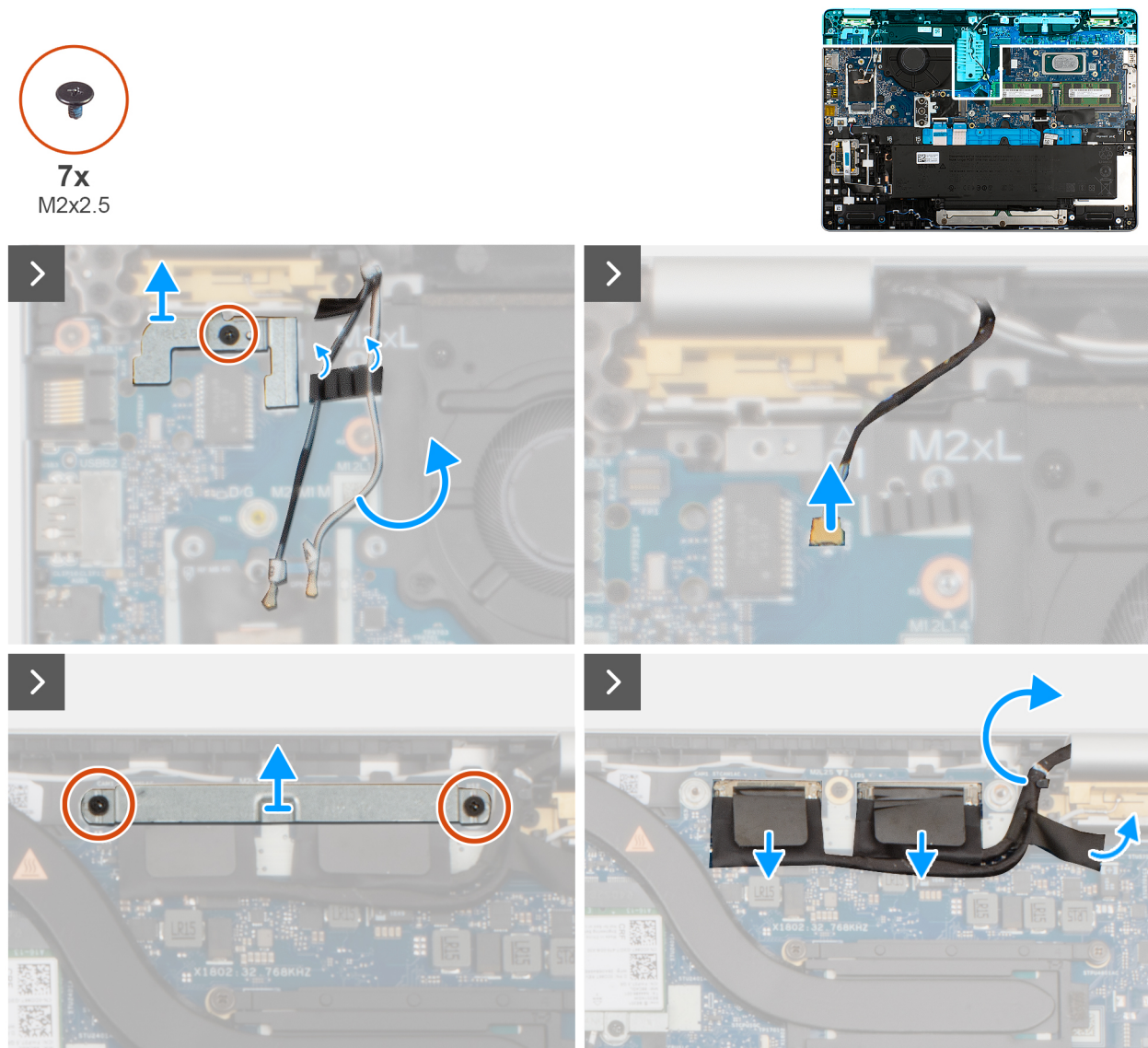
Figura 41. Rimozione dell'antenna WLAN
