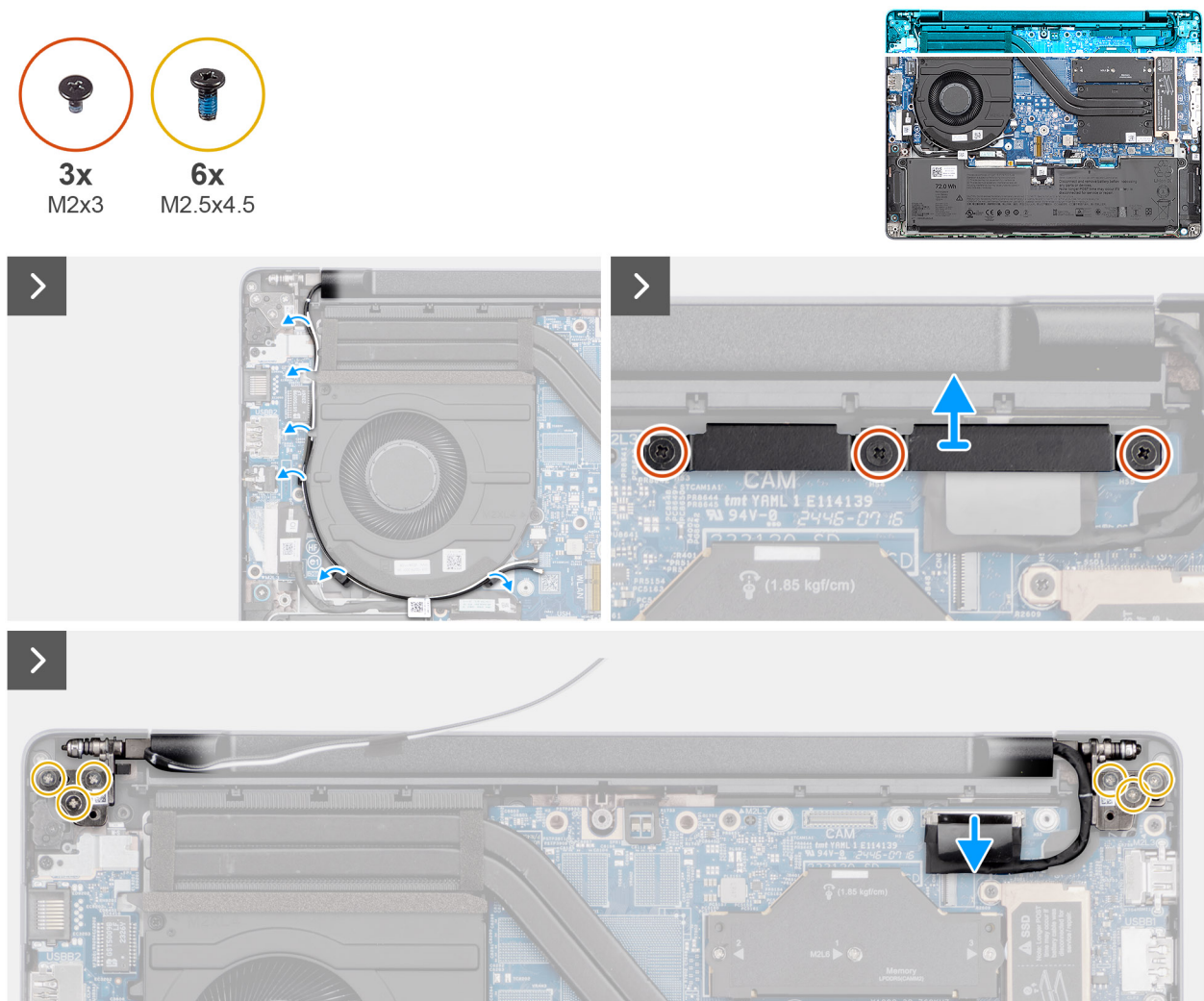
Figura 47. Rimozione del gruppo del display
