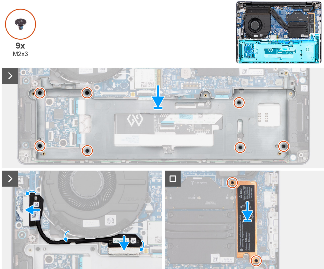
Figura 34. Installazione del telaio della batteria
