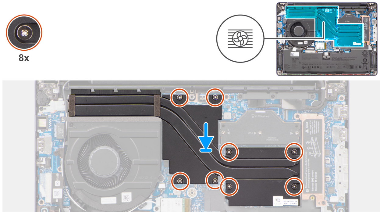
Figura 42. Installazione del dissipatore di calore
