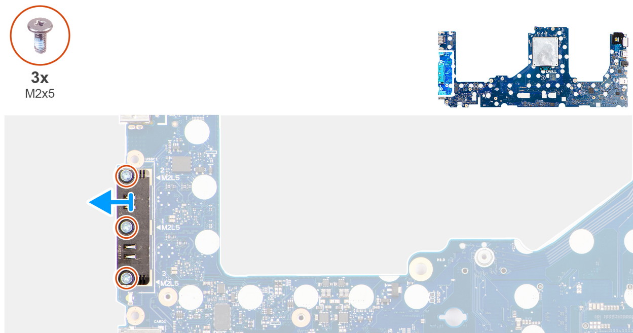
Figura 94. Rimozione del modulo USB Type-C
