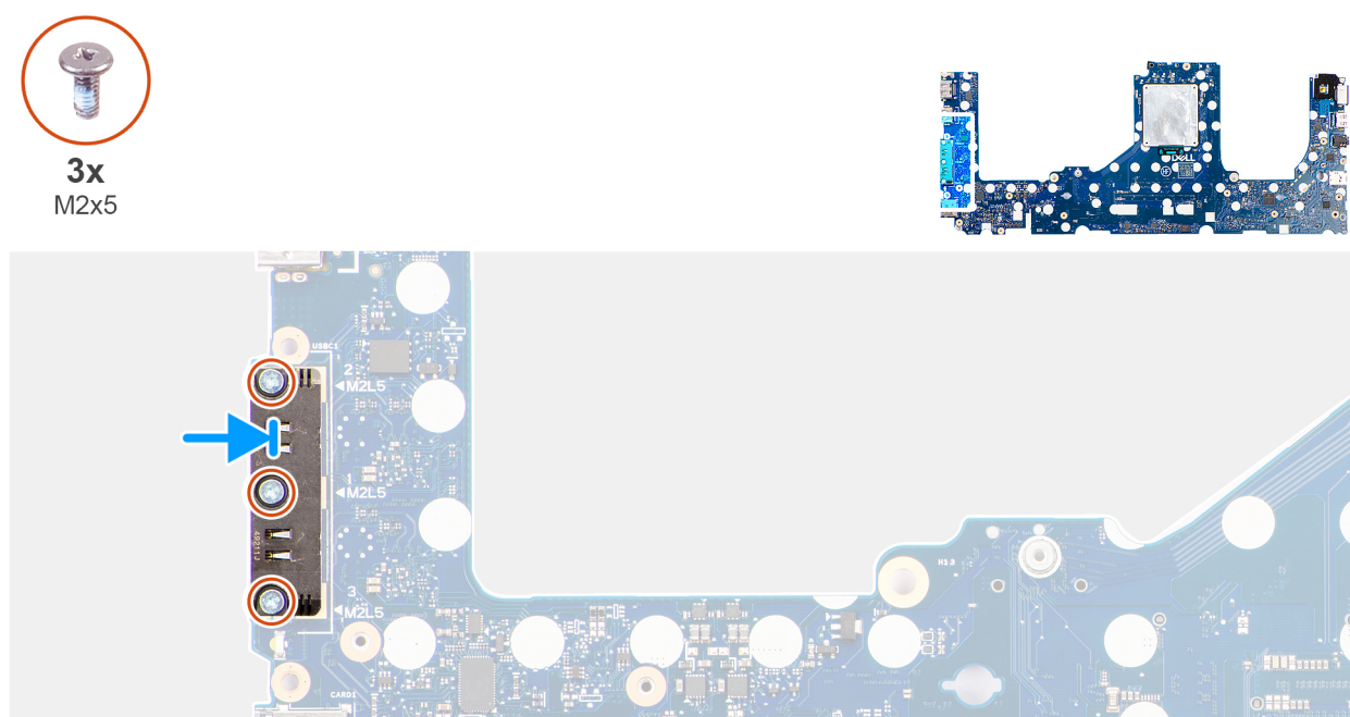
Figura 95. Installazione del modulo USB Type-C
