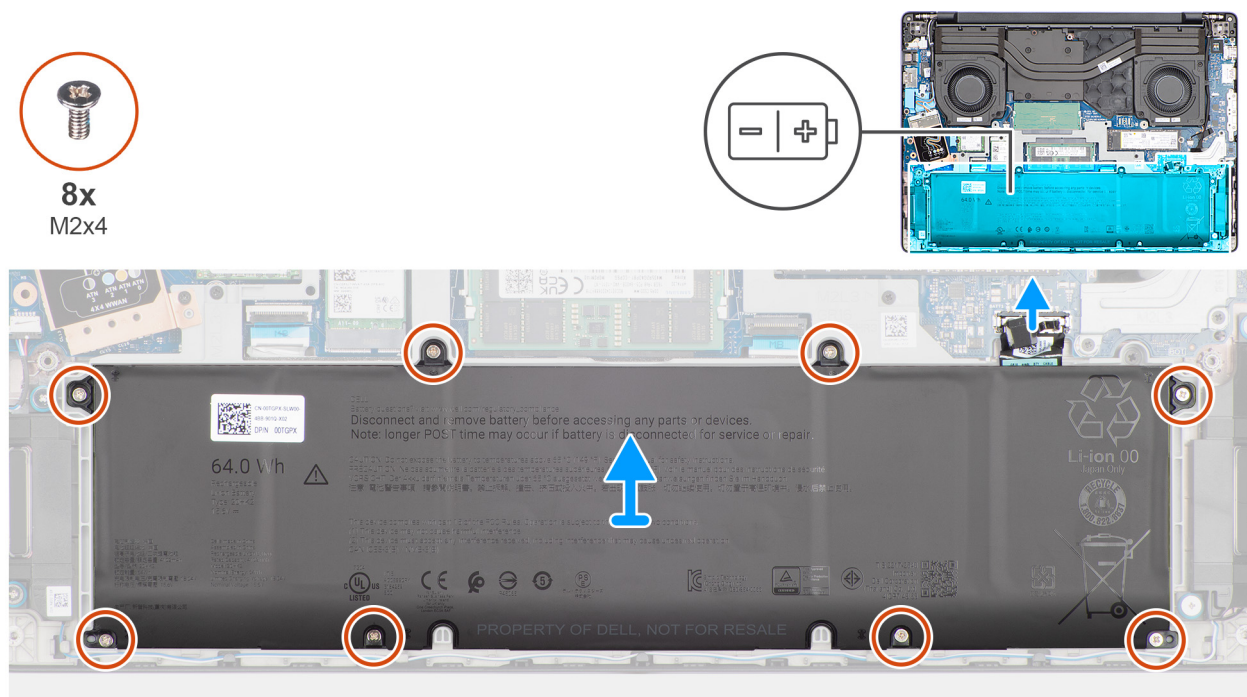
Figura 17. Rimozione della batteria
