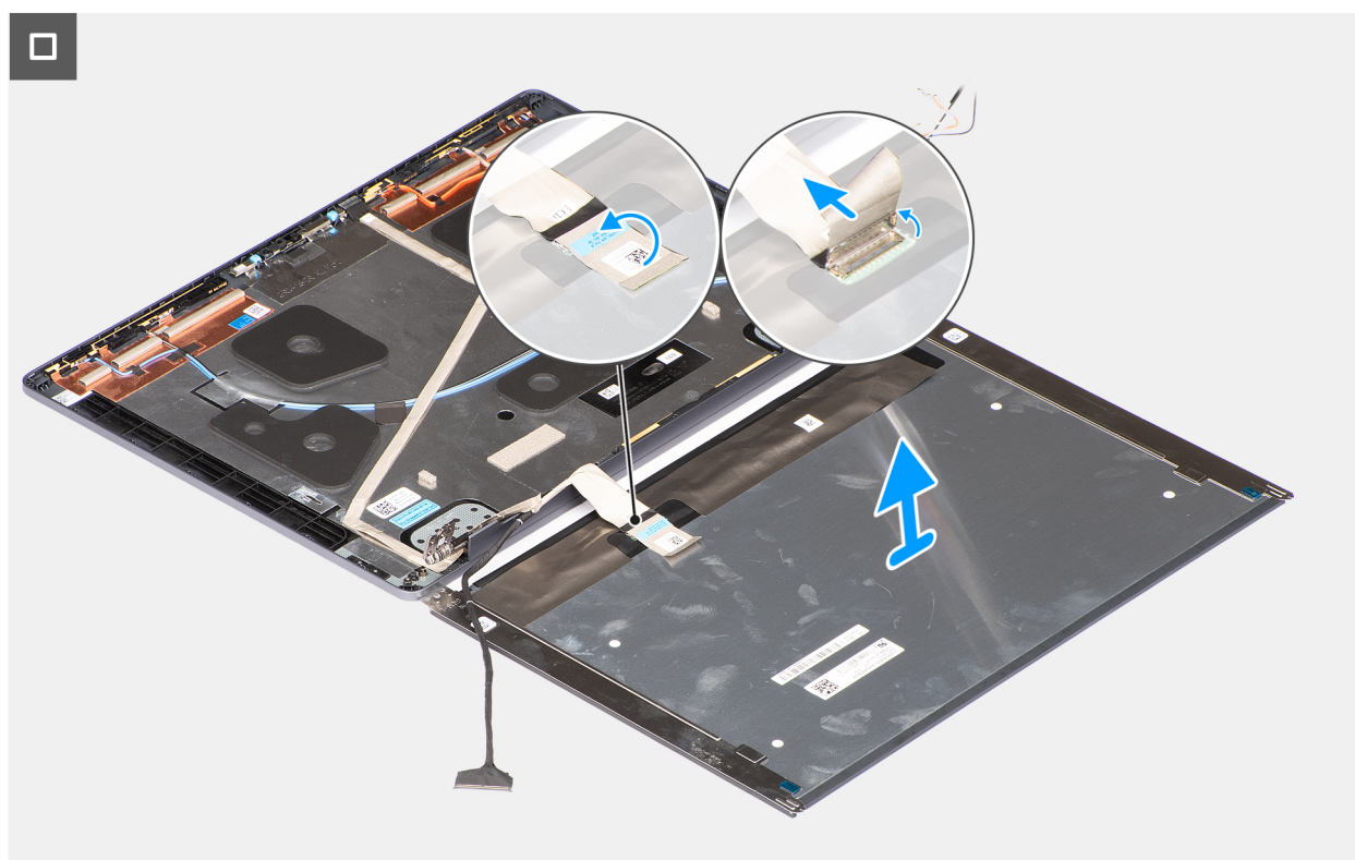
Figura 70. Rimozione del pannello del display
