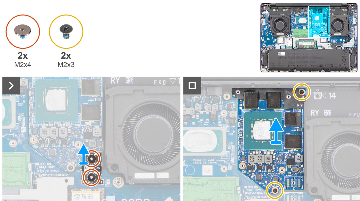
Figura 46. Rimozione dell'GPU
