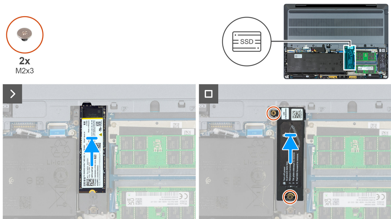
Figura 35. Installazione dell'SSD M.2 2280 nello slot 3 (SSD3)
