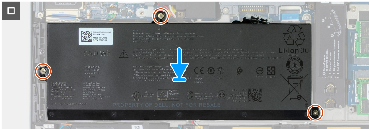
Figura 43. Ricollocamento della batteria
