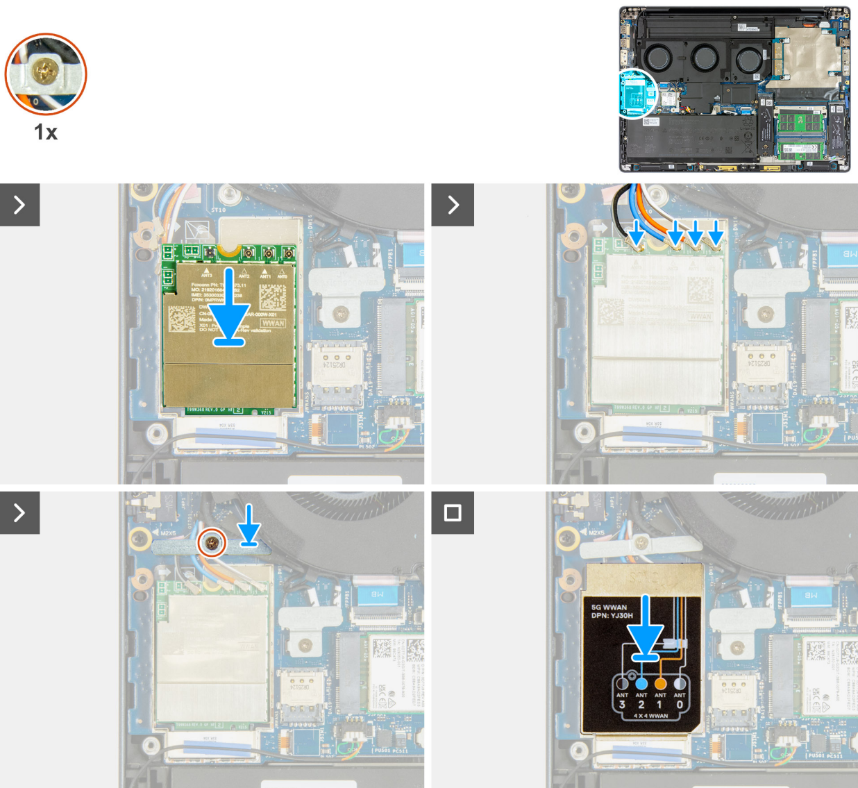
Figura 49. Installazione della scheda WWAN
