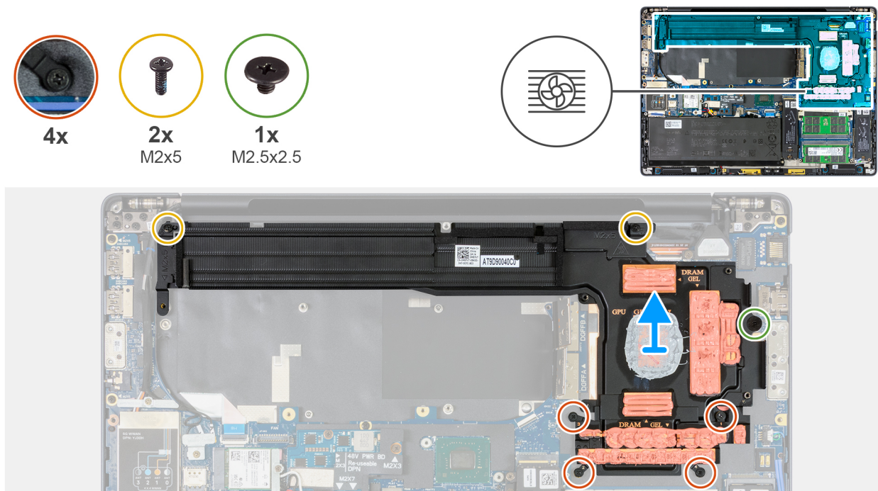
Figura 78. Rimozione del dissipatore di calore per computer forniti con scheda grafica dedicata
