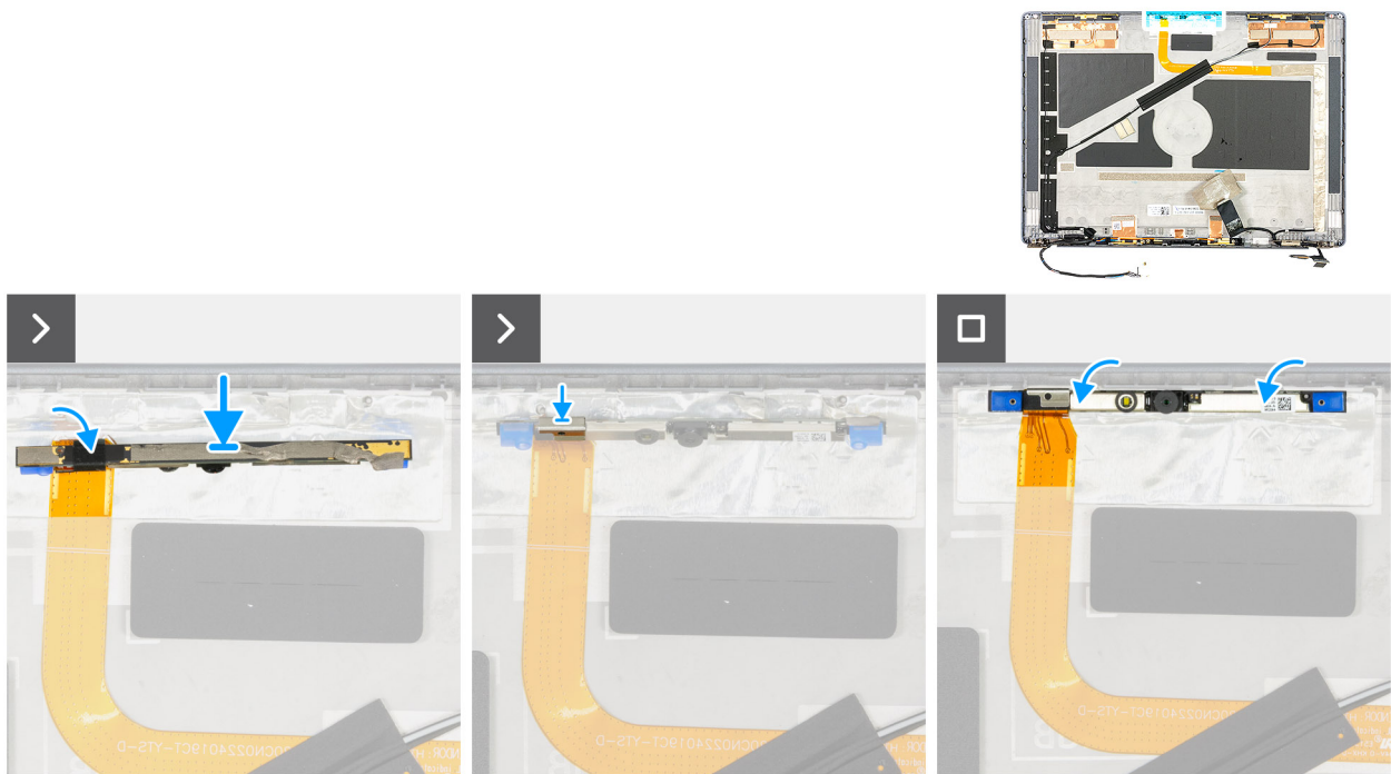
Figura 105. Installazione del modulo della fotocamera
