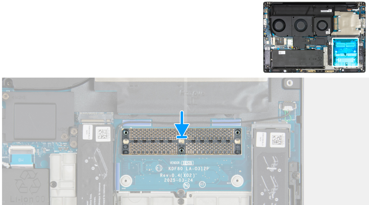
Figura 73. Installazione del connettore di memoria
