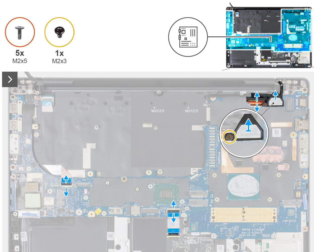
Figura 112. Rimozione della scheda di sistema
