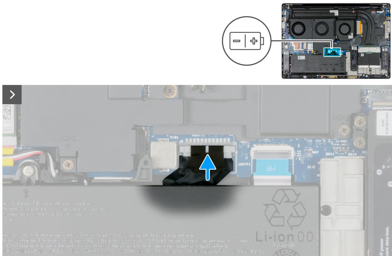
Figura 27. Collegamento del cavo della batteria
