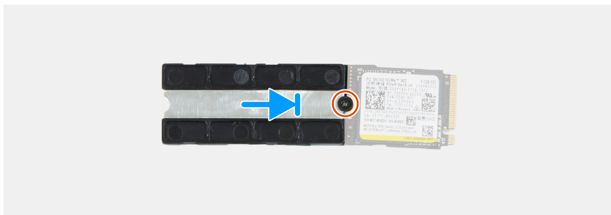
Figura 41. Installazione dell'SSD M.2 2230
