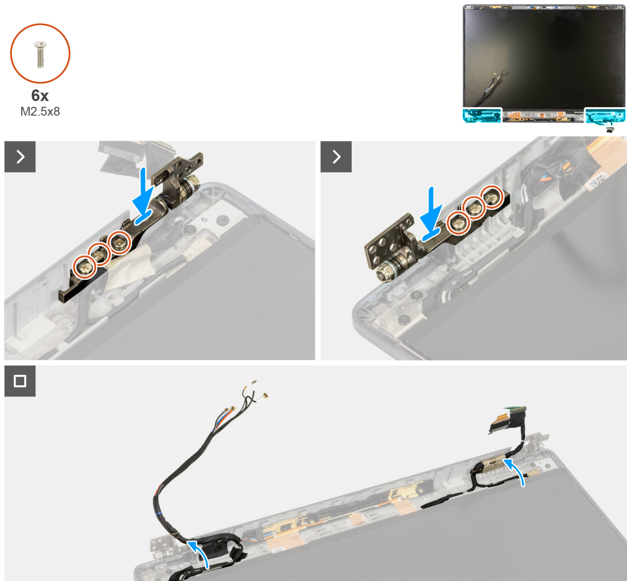
Figura 100. Installazione delle cerniere del display
