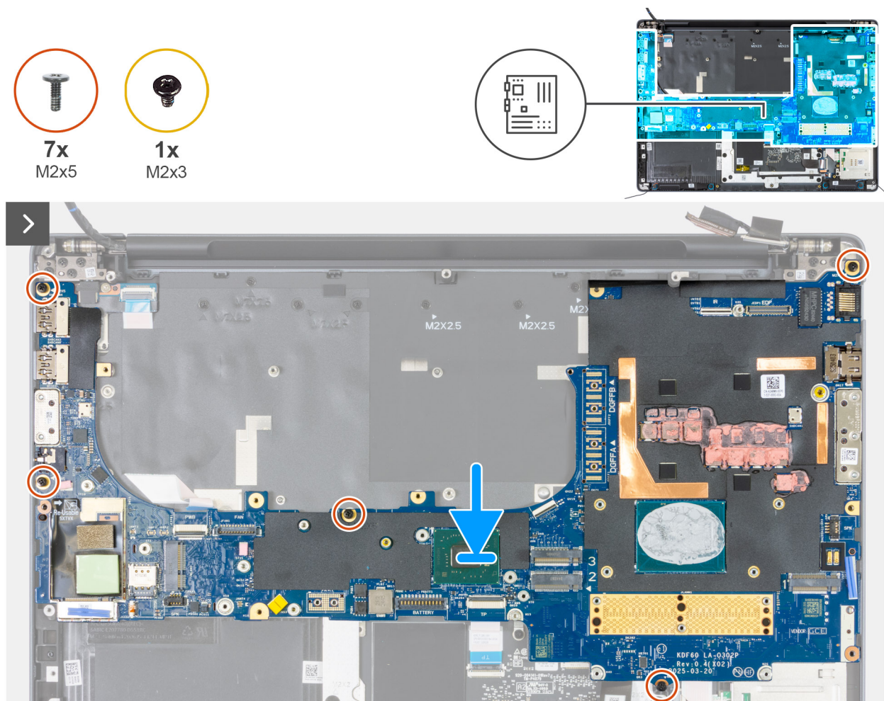
Figura 115. Installazione della scheda di sistema
