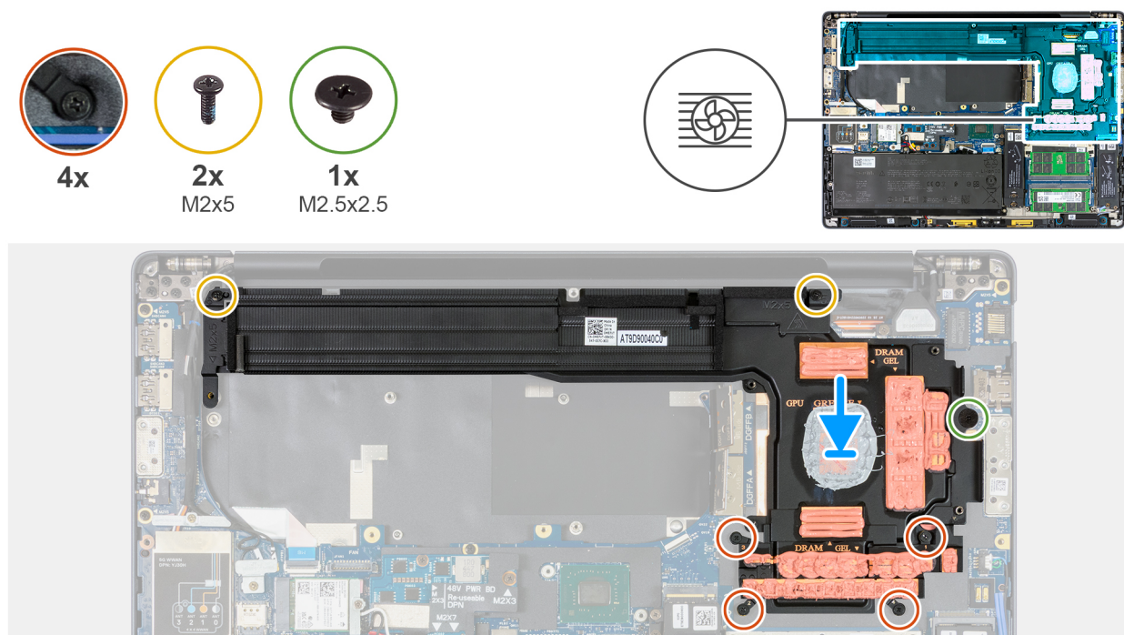
Figura 76. Installazione del dissipatore di calore per computer forniti con scheda grafica dedicata
