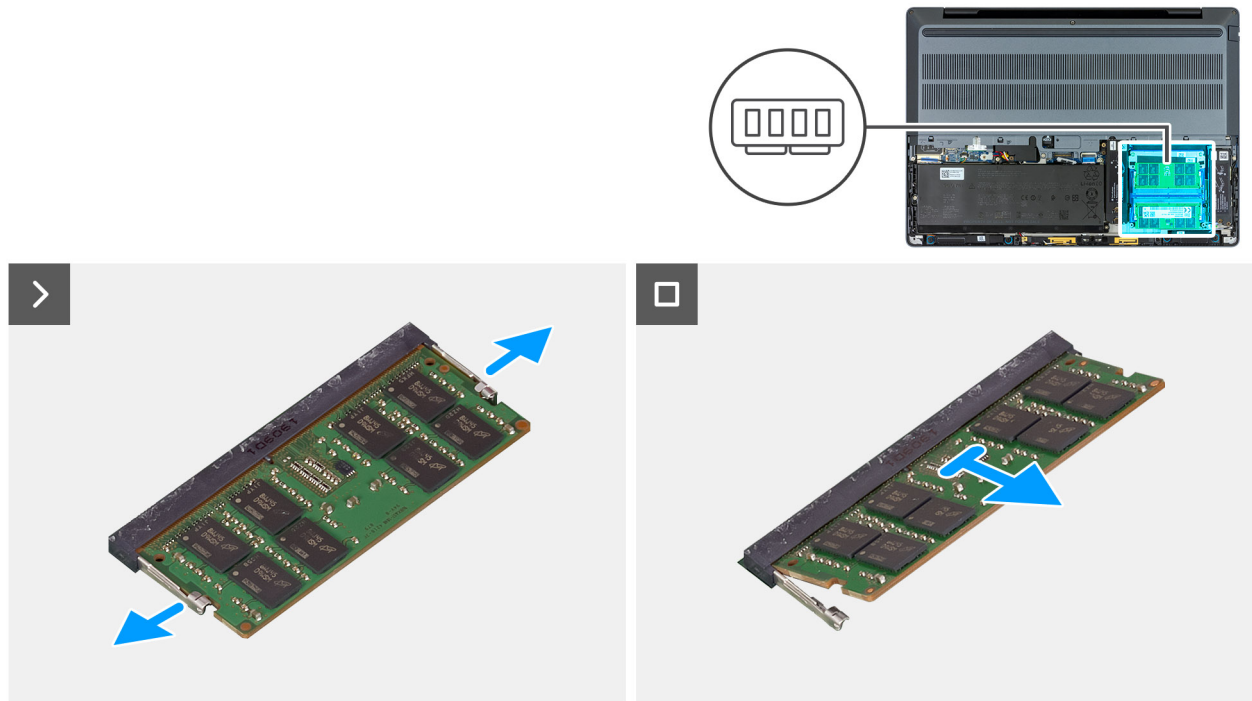
Figura 30. Rimozione del modulo di memoria
