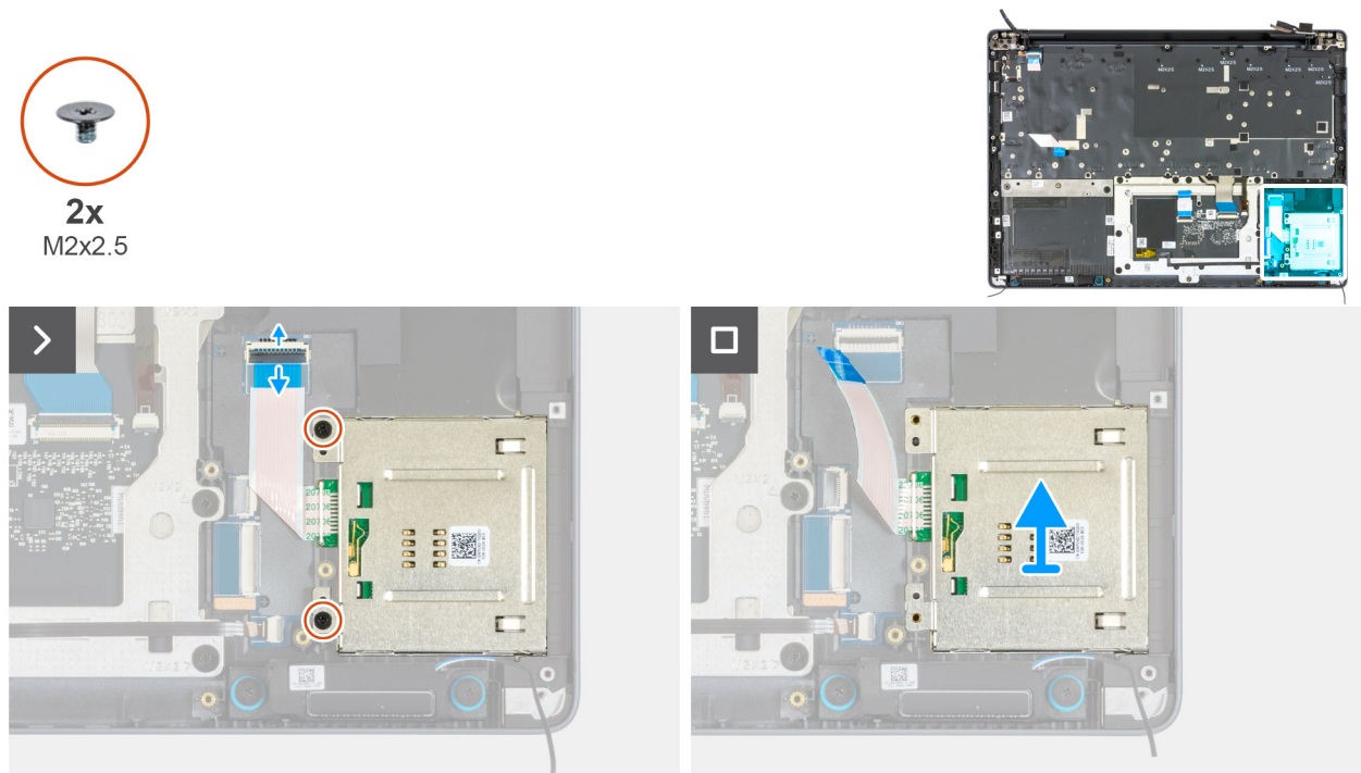
Figura 123. Rimozione del lettore di smart card
