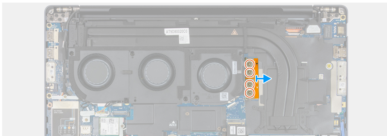
Figura 55. Rimozione del connettore del laser FPC integrato
