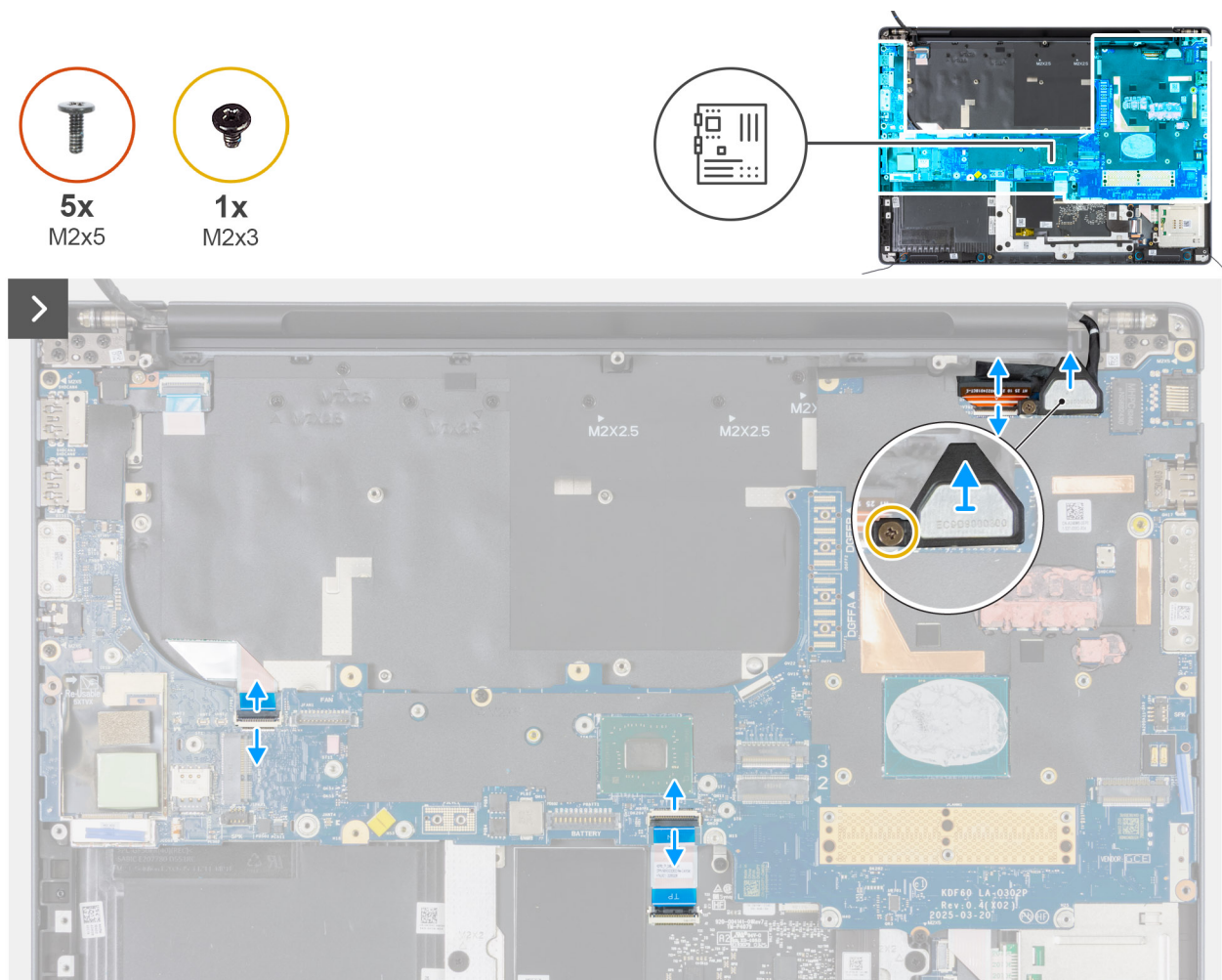
Figura 111. Rimozione della scheda di sistema
