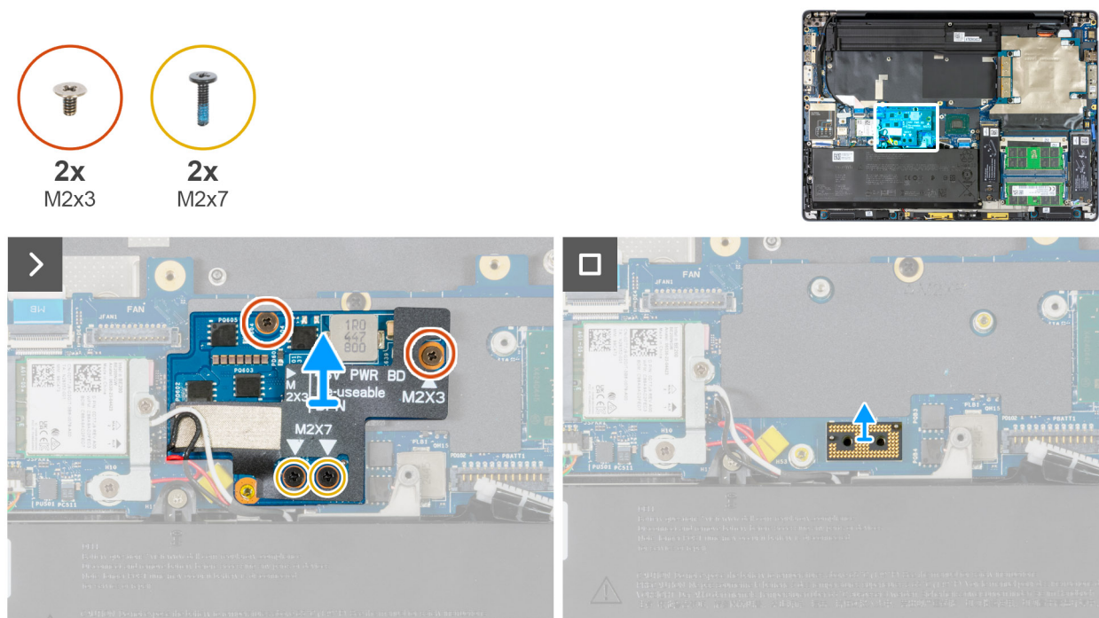
Figura 71. Rimozione della scheda di alimentazione
