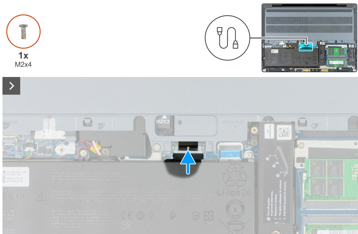
Figura 21. Collegamento del cavo della batteria
