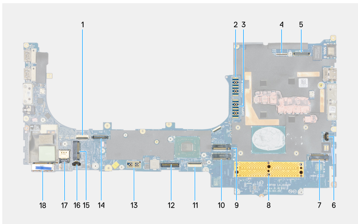
Figura 110. Componenti della scheda di sistema
