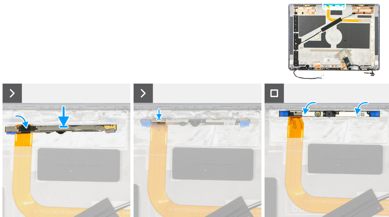
Figura 104. Installazione del modulo della fotocamera
