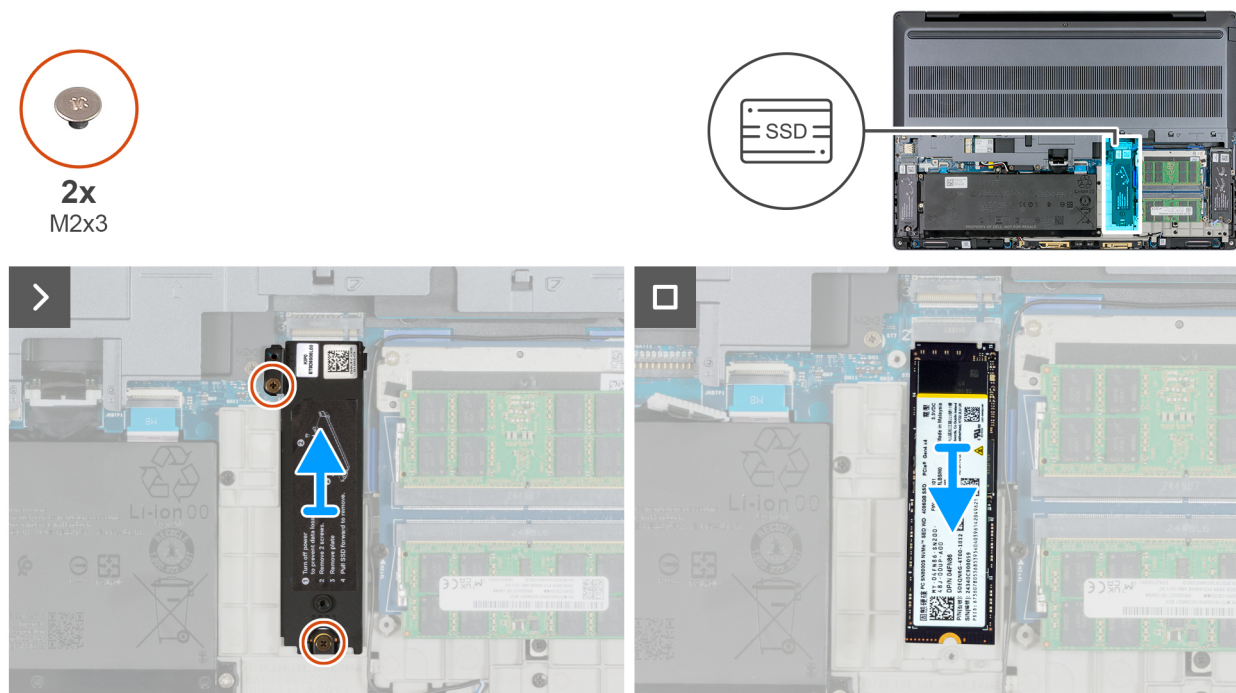
Figura 36. Rimozione dell'SSD M.2 2280 dallo slot 3 (SSD3)
