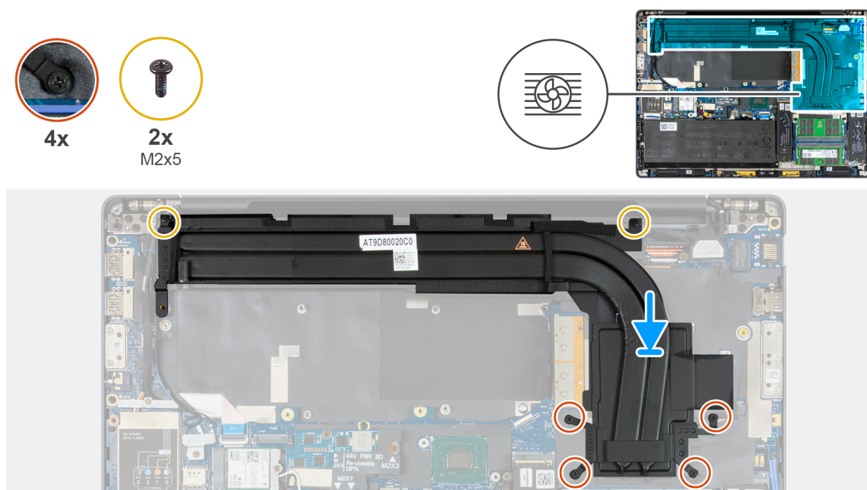
Figura 74. Installazione del dissipatore di calore per computer forniti con scheda grafica integrata
