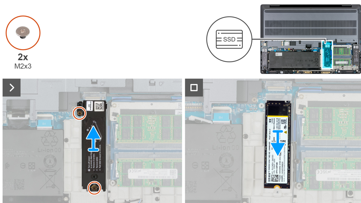
Figura 38. Rimozione dell'SSD M.2 2280 dallo slot 2 (SSD2)
