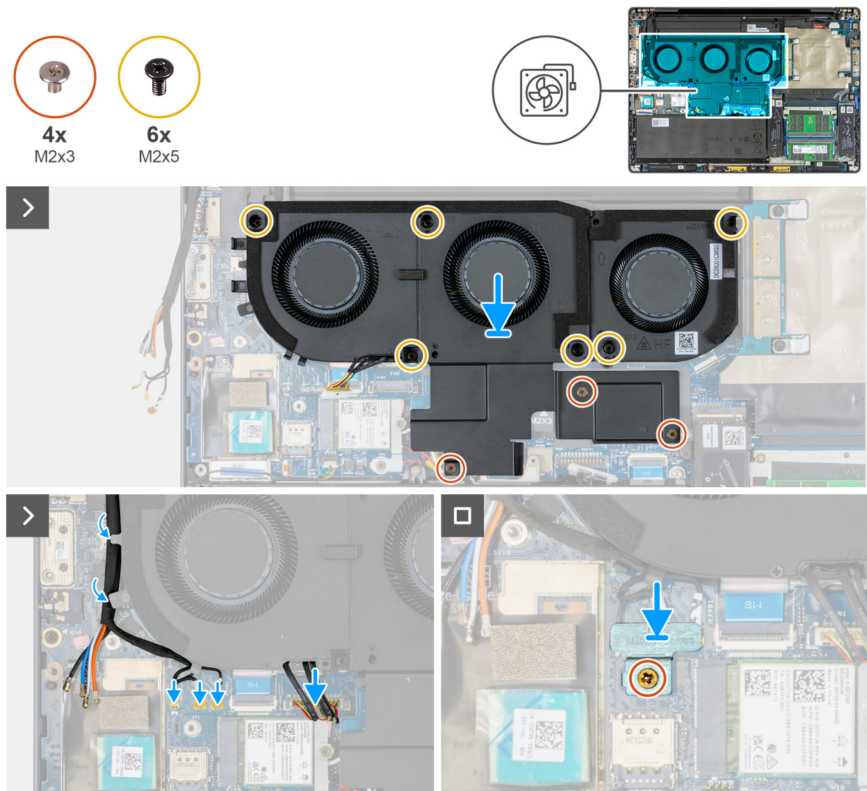
Figura 62. Installazione del gruppo ventola
