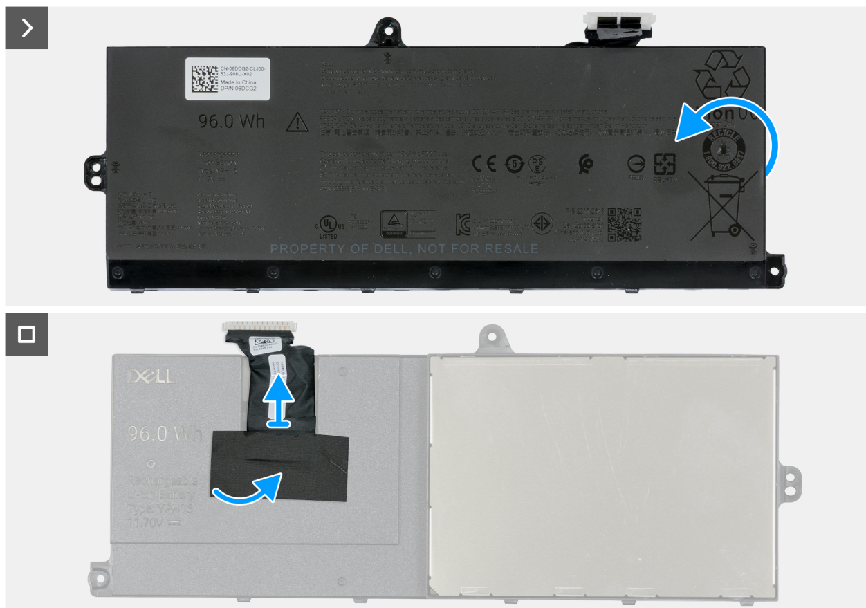
Figura 43. Rimozione del cavo della batteria dalla batteria
