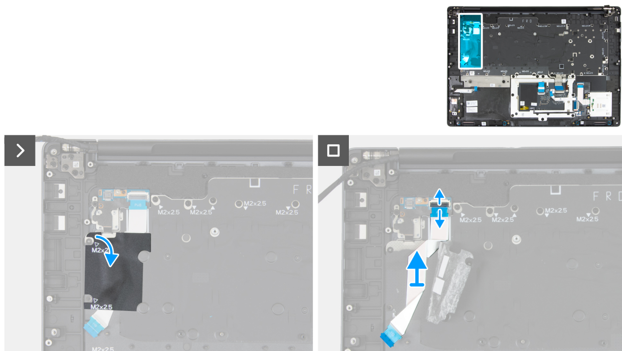
Figura 125. Rimozione del cavo della scheda del pulsante di alimentazione
