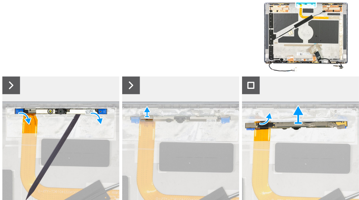
Figura 103. Rimozione del modulo della fotocamera
