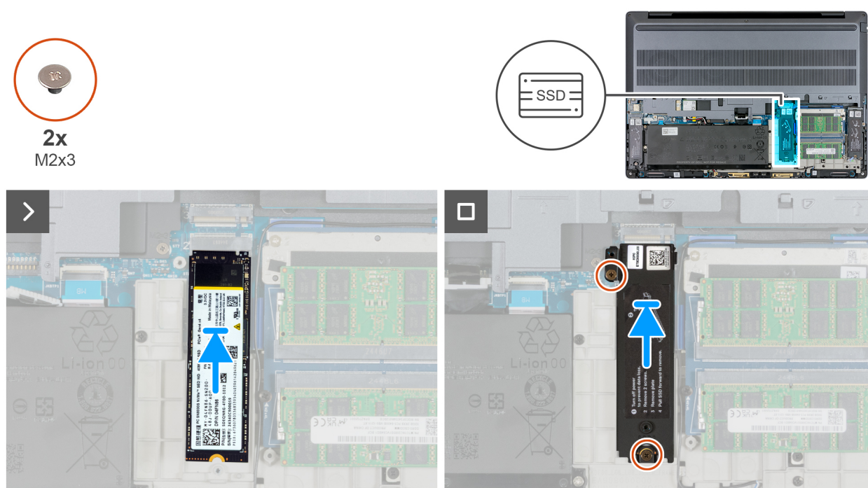
Figura 39. Installazione dell'SSD M.2 2280 nello slot 2 (SSD2)
