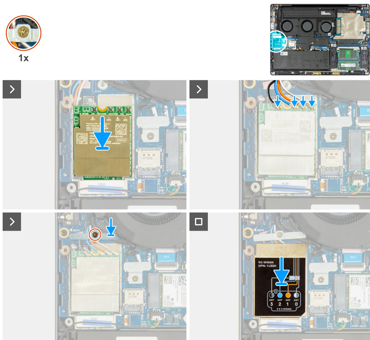
Figura 51. Installazione della scheda WWAN
