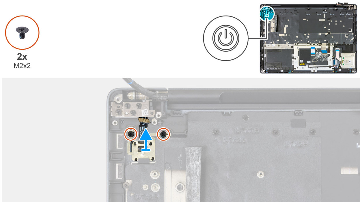
Figura 129. Rimozione del pulsante di accensione
