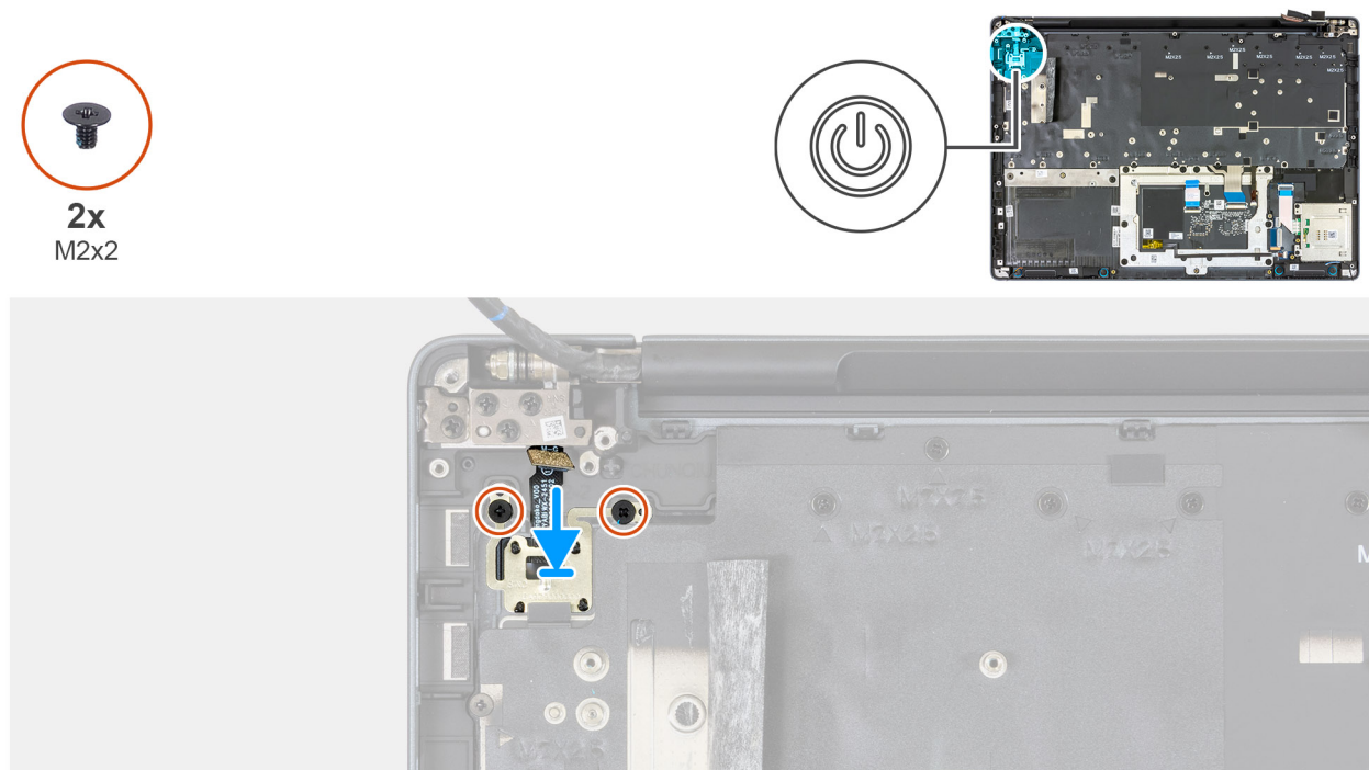
Figura 130. Installazione del pulsante di accensione
