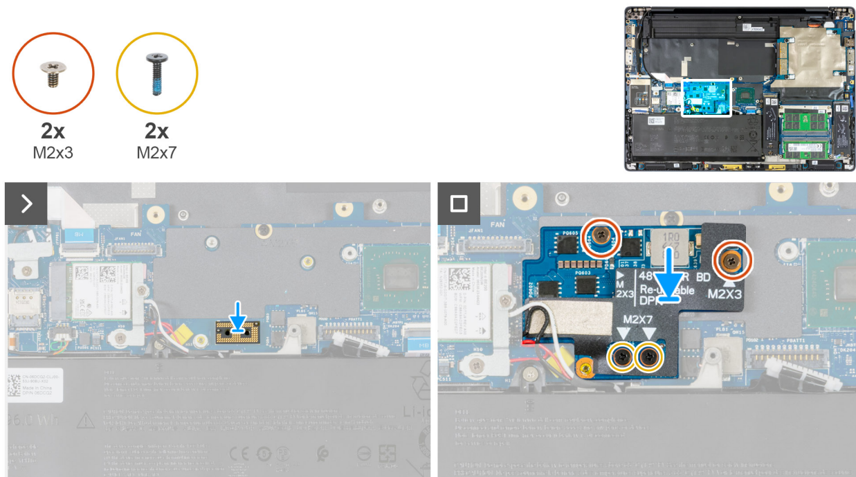
Figura 72. Installazione della scheda di alimentazione
