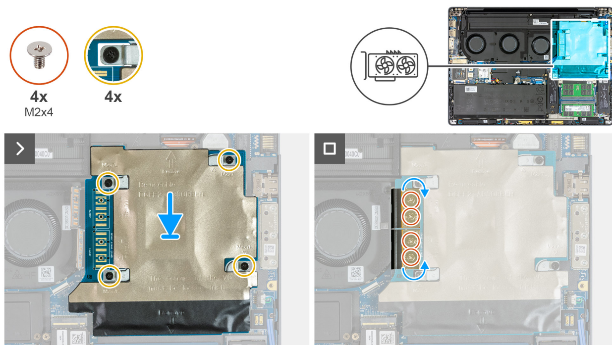
Figura 54. Installazione della scheda GPU
