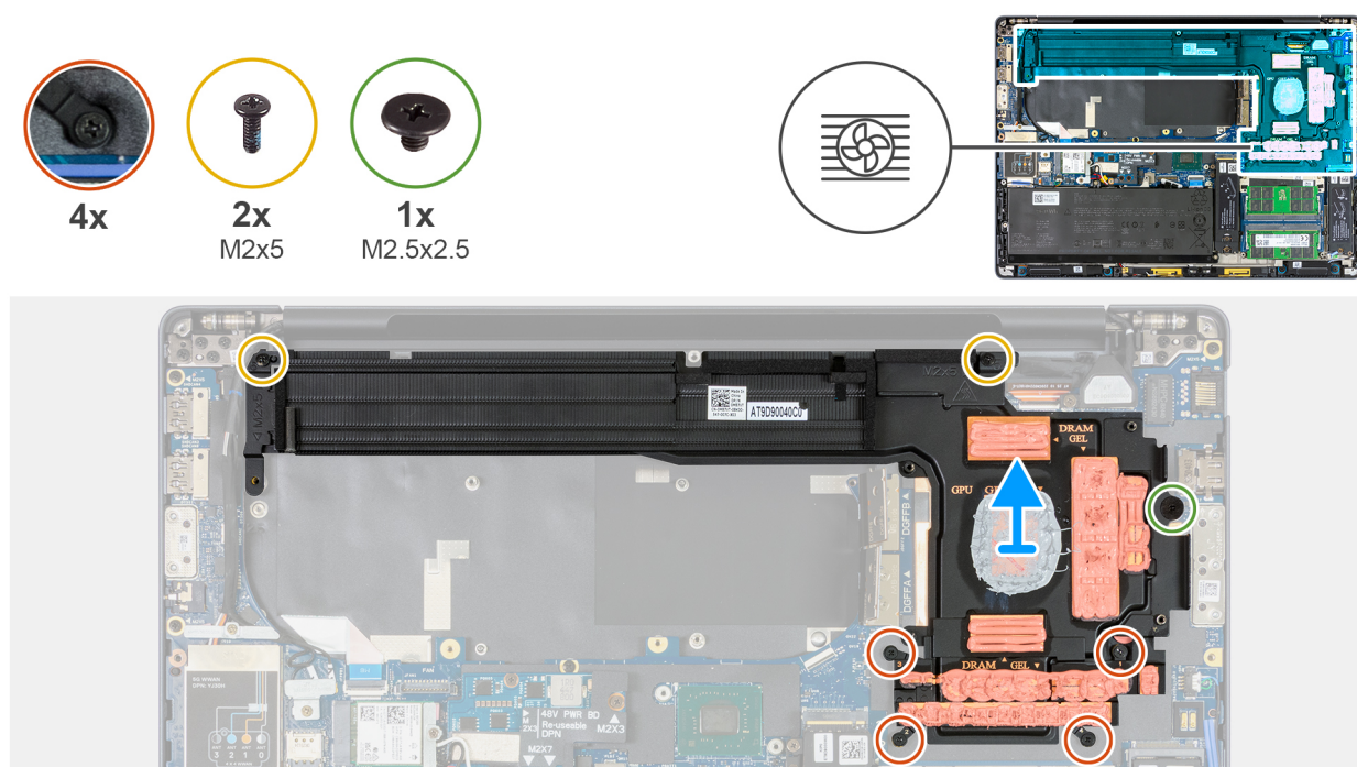
Figura 75. Rimozione del dissipatore di calore per computer forniti con scheda grafica dedicata
