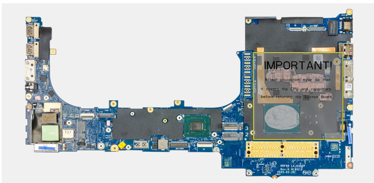
Figura 113. Preparazione della scheda di sistema difettosa per la restituzione
