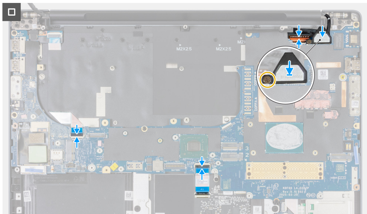
Figura 116. Installazione della scheda di sistema
