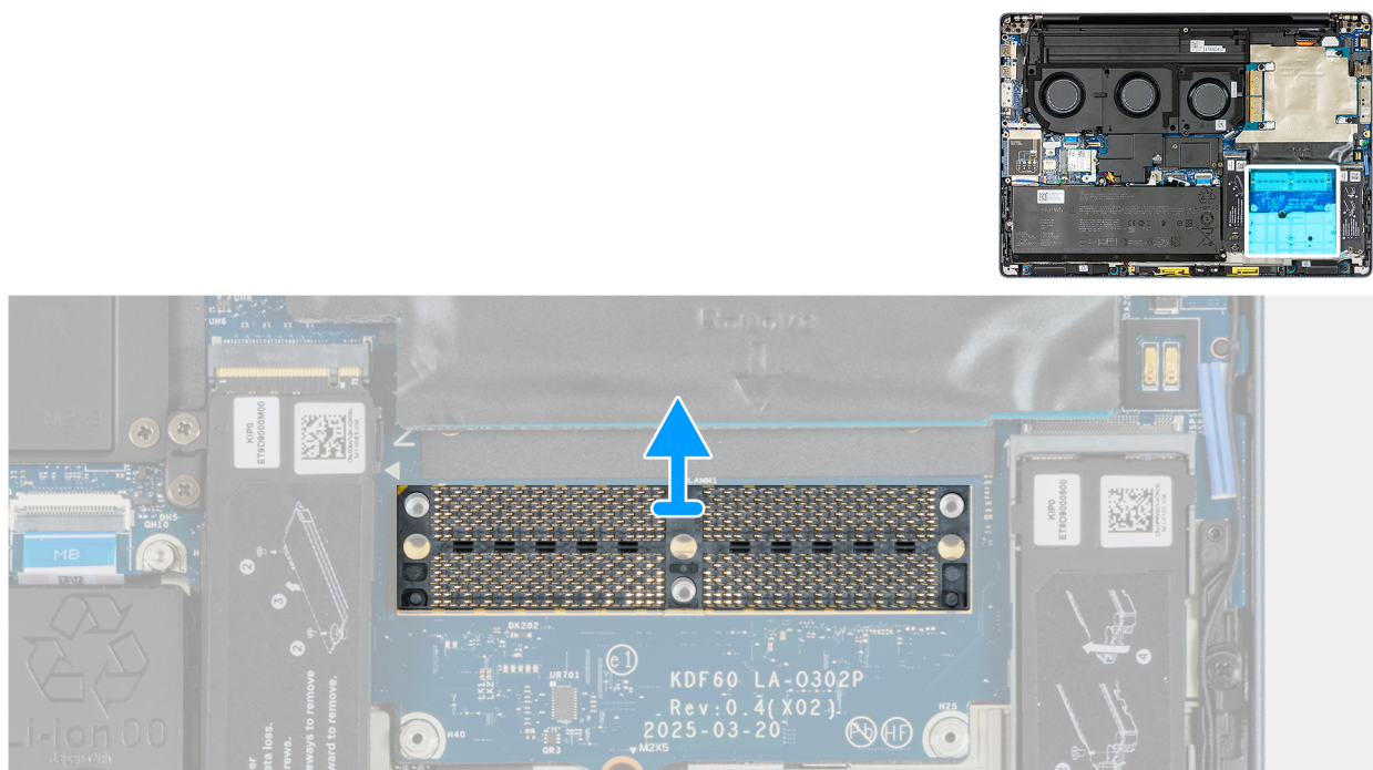
Figura 69. Rimozione del connettore della memoria
