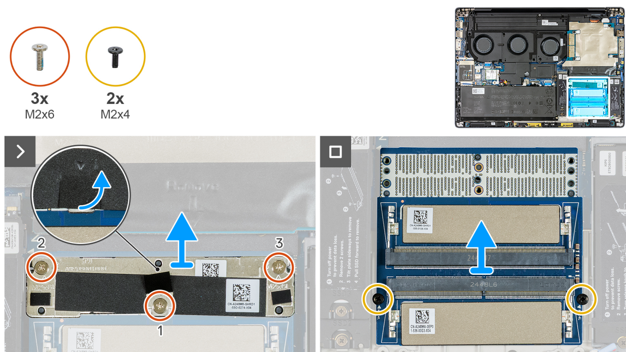
Figura 67. Rimozione della scheda interposer della memoria
