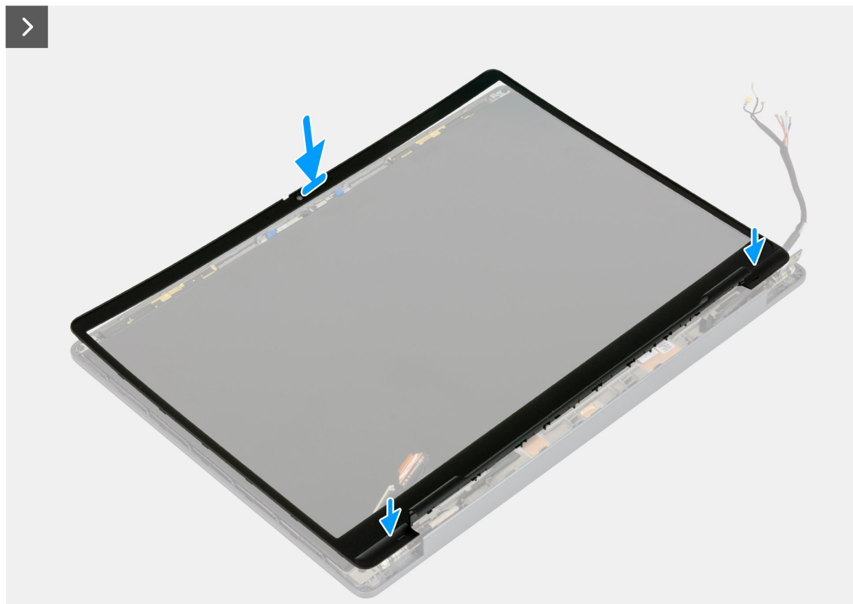
Figura 89. Installazione della cornice del display
