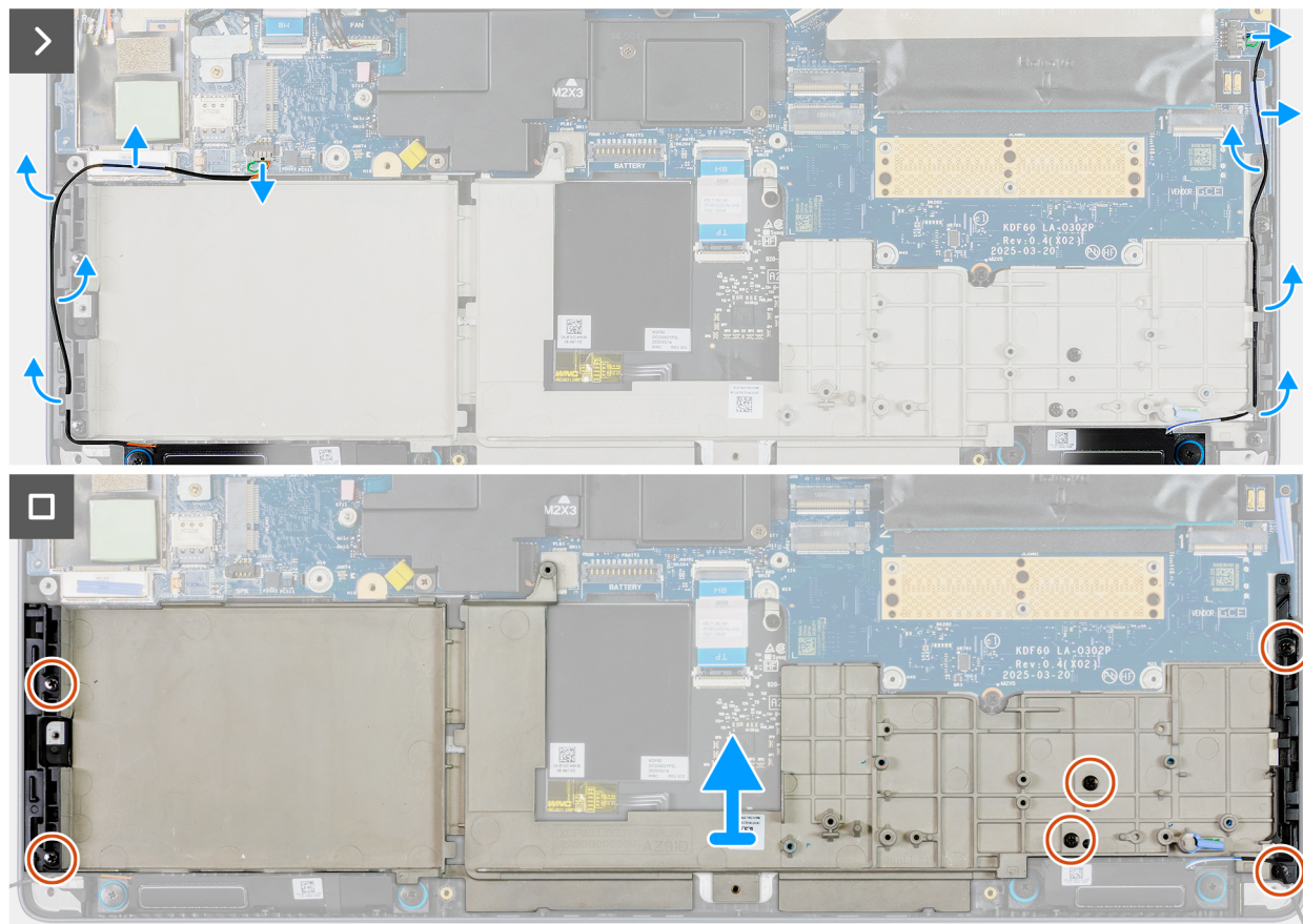
Figura 79. Rimozione dell'intelaiatura interna
