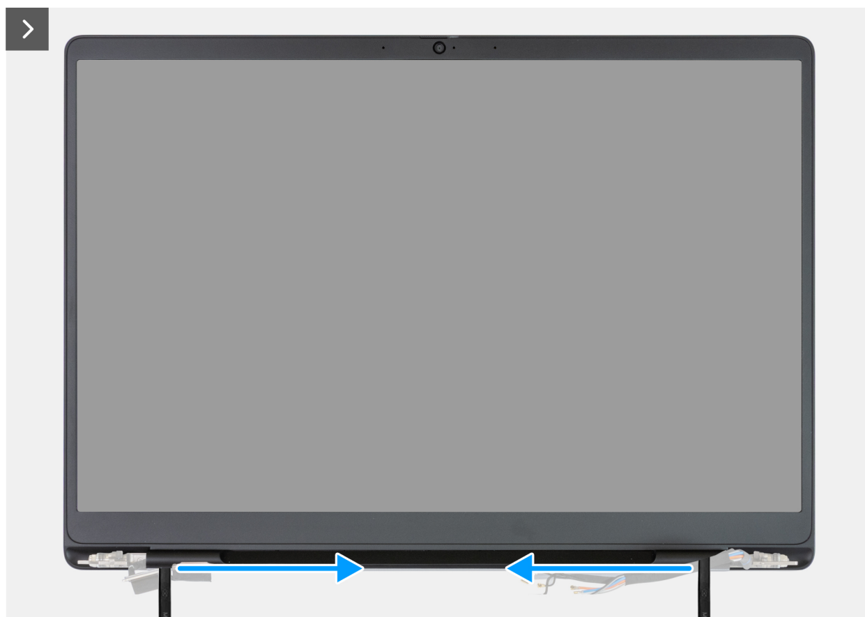
Figura 86. Rimozione della cornice del display
