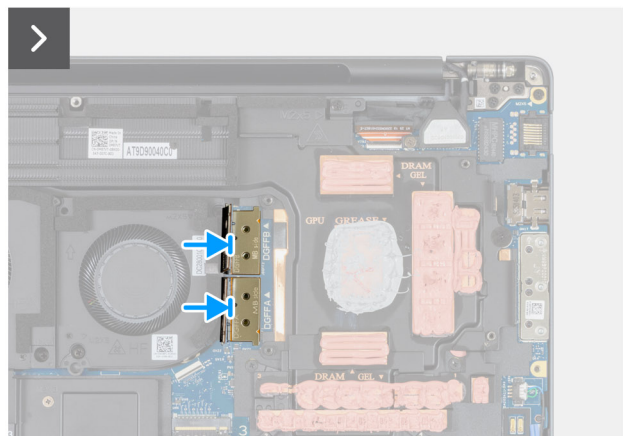
Figura 58. Installazione del connettore del laser FPC dedicato
