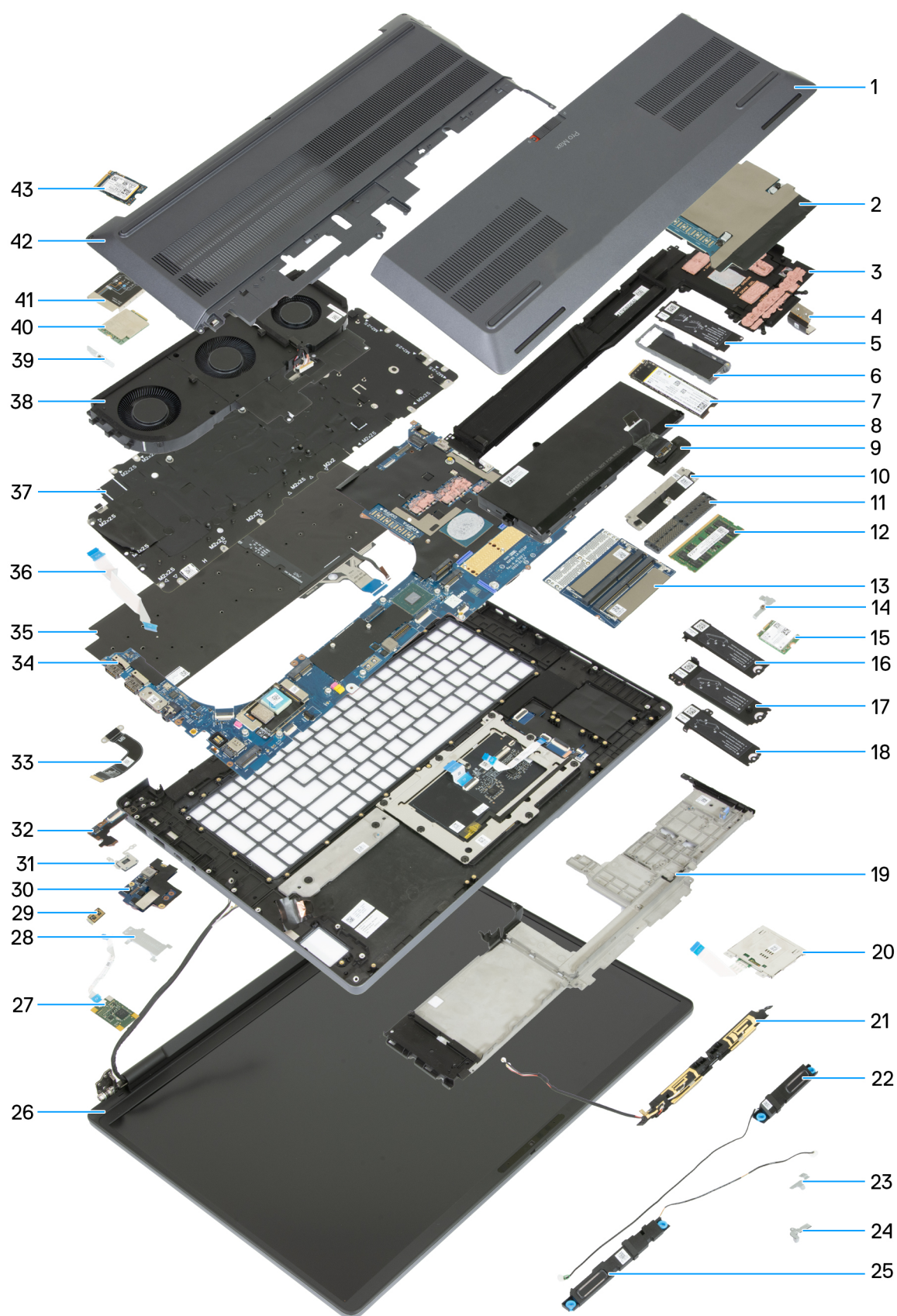
Figura 9. Componenti principali di Dell Pro Max 18 Plus MB18250
