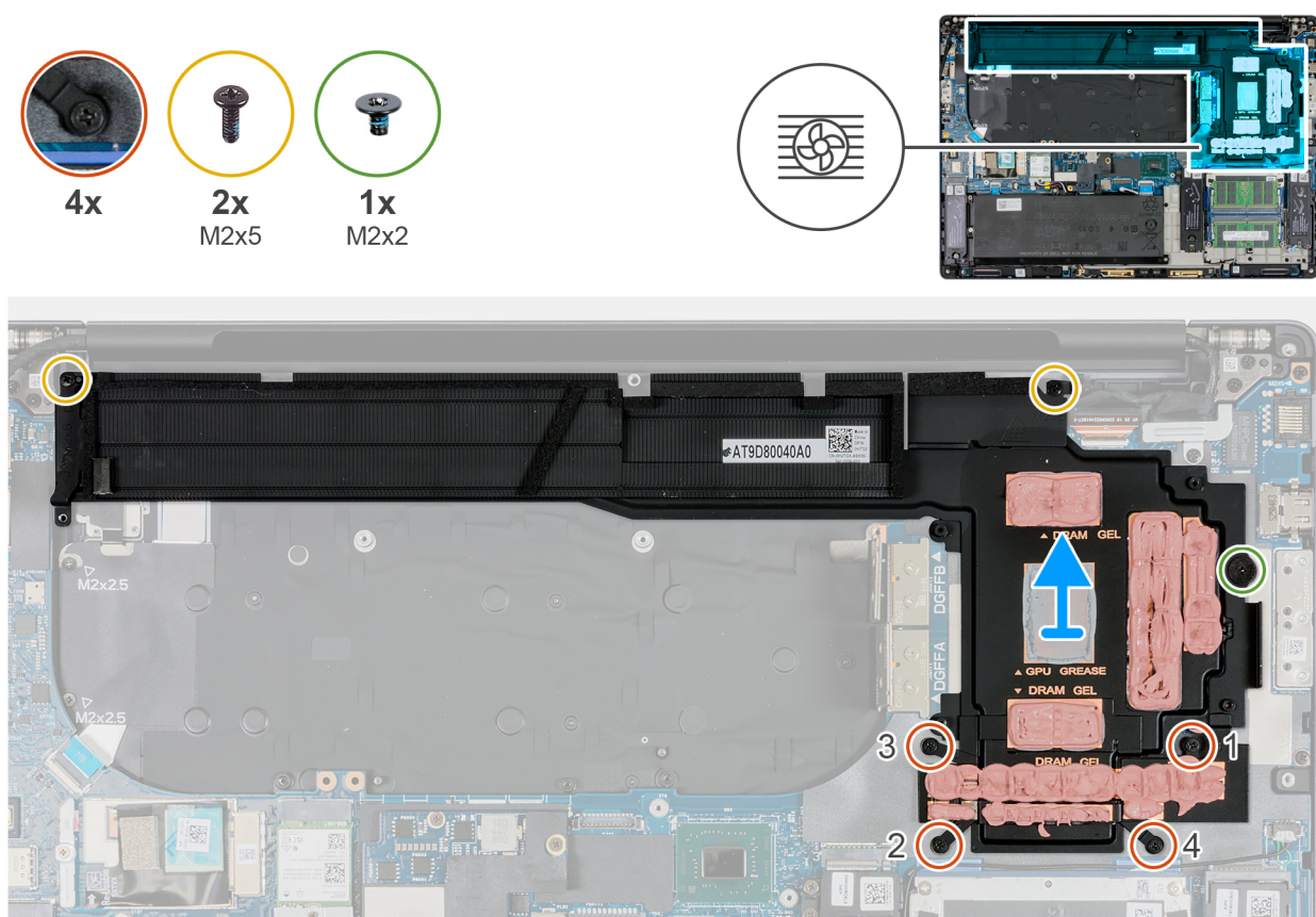
Figura 75. Rimozione del dissipatore di calore per computer forniti con scheda grafica dedicata
