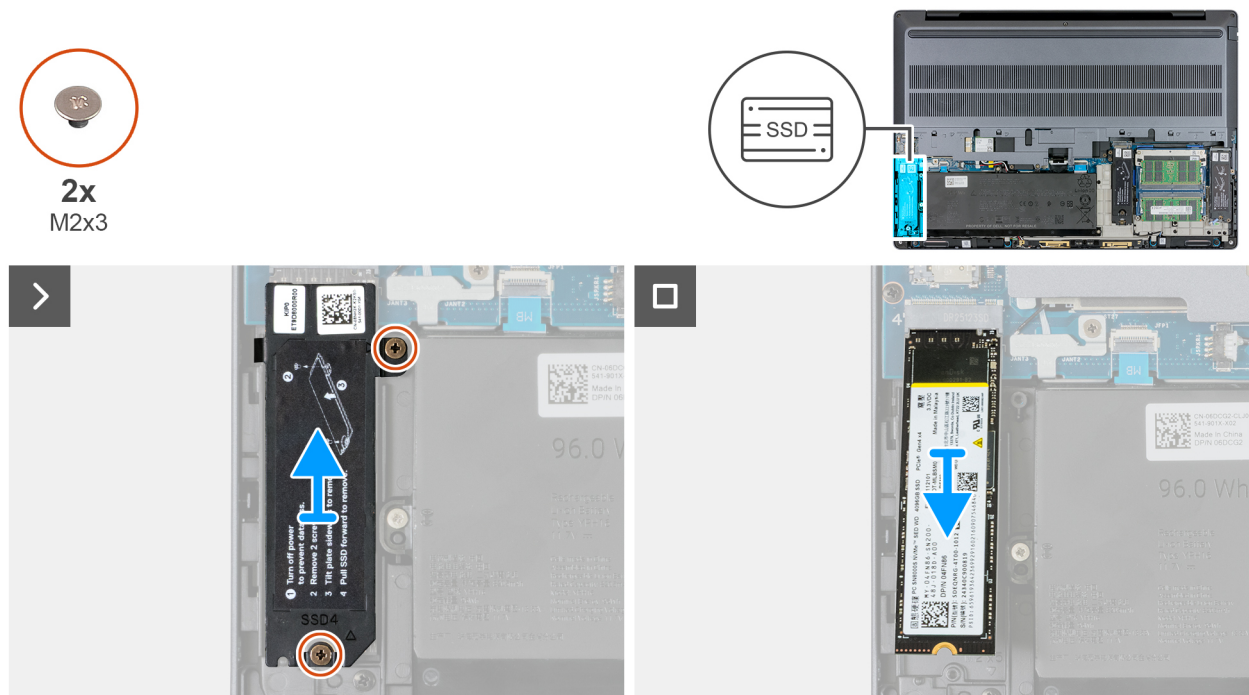
Figura 40. Rimozione dell'SSD M.2 2280 dallo slot 4 (SSD4)
