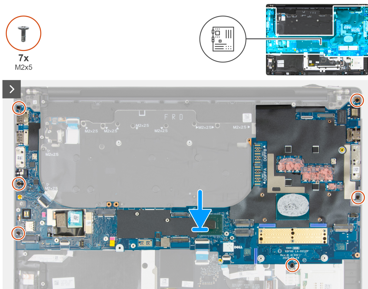
Figura 111. Installazione della scheda di sistema
