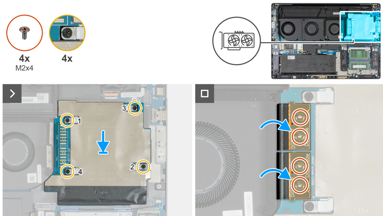
Figura 56. Installazione della scheda GPU
