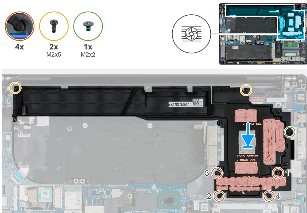
Figura 76. Installazione del dissipatore di calore per computer forniti con scheda grafica dedicata
