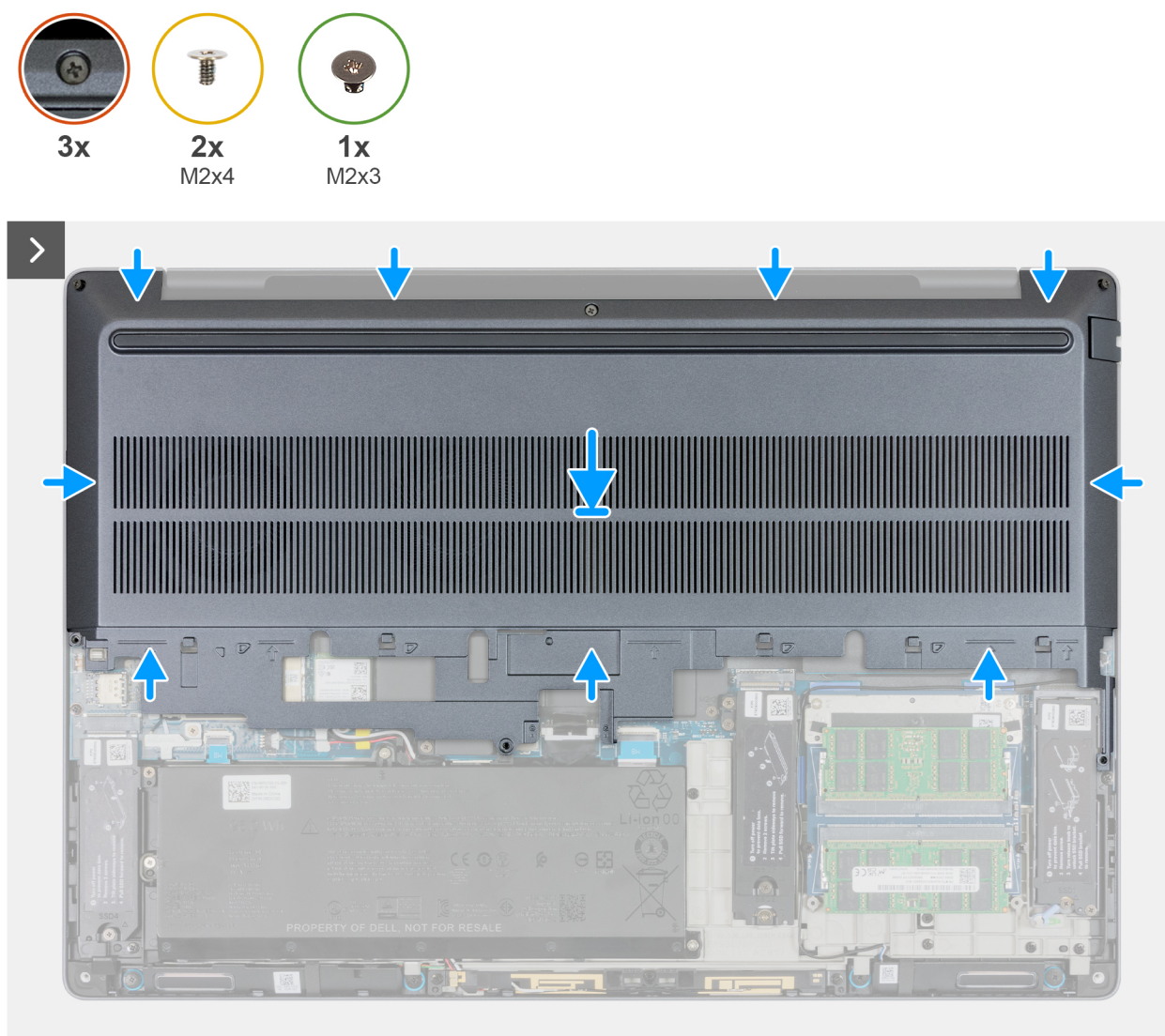
Figura 22. Allineamento dei fori delle viti sul coperchio della base ai fori sul gruppo del poggiapolsi e tastiera
