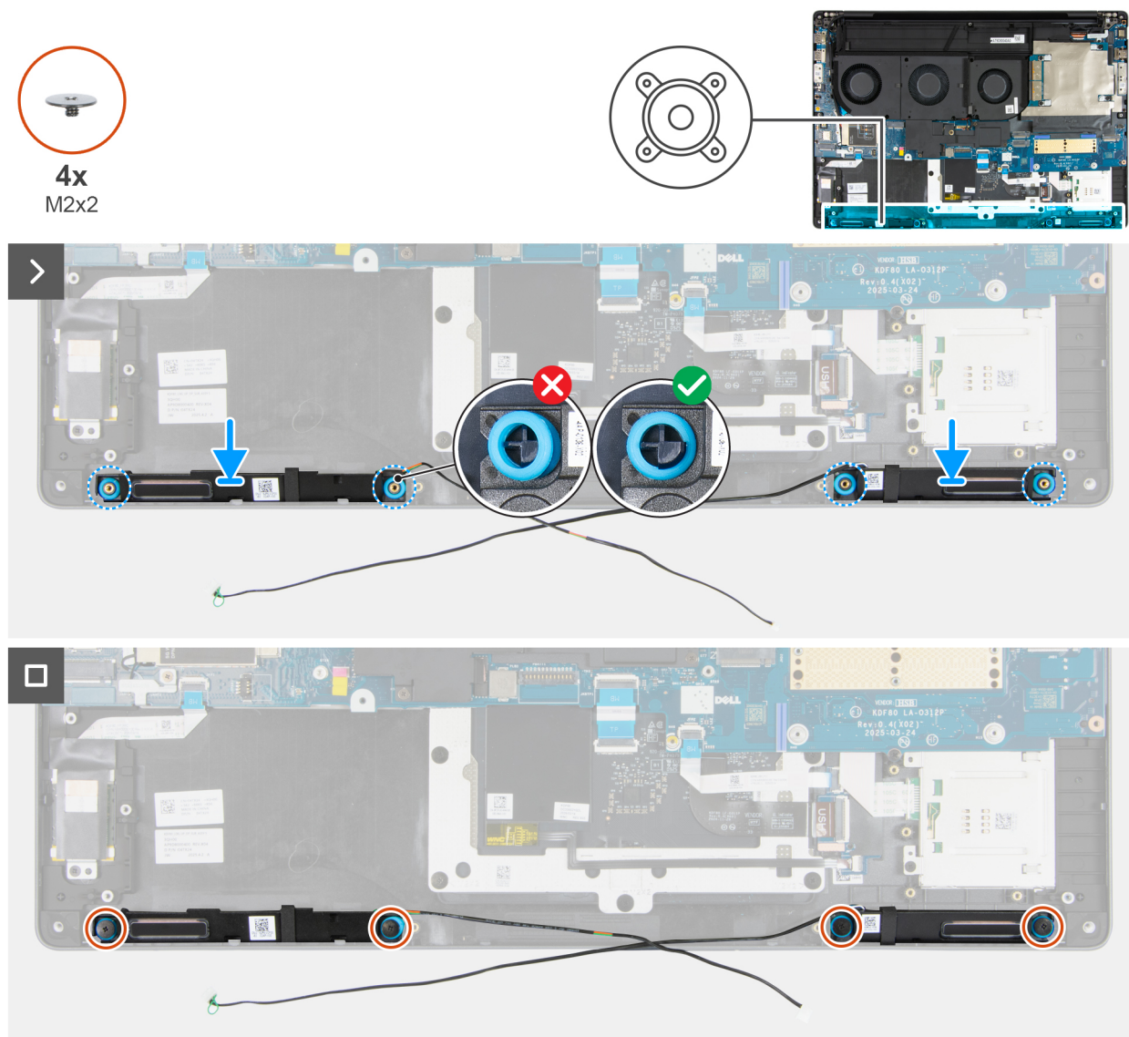
Figura 82. Installazione degli altoparlanti
