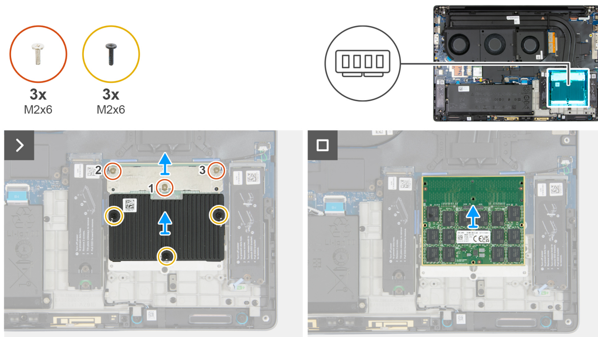
Figura 32. Rimozione del modulo CAMM
