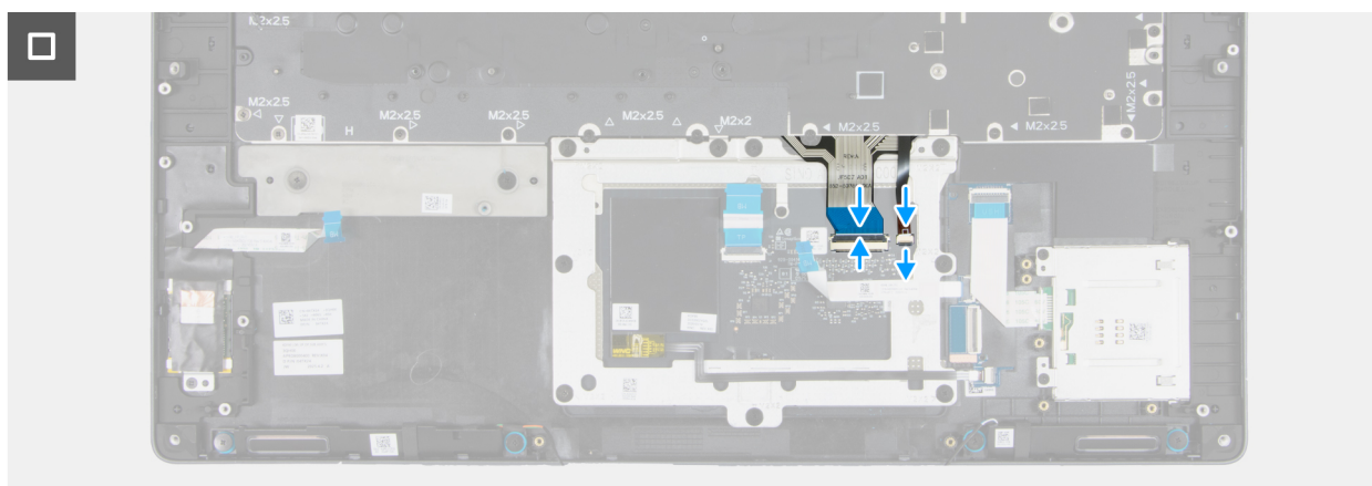
Figura 120. Installazione della tastiera
