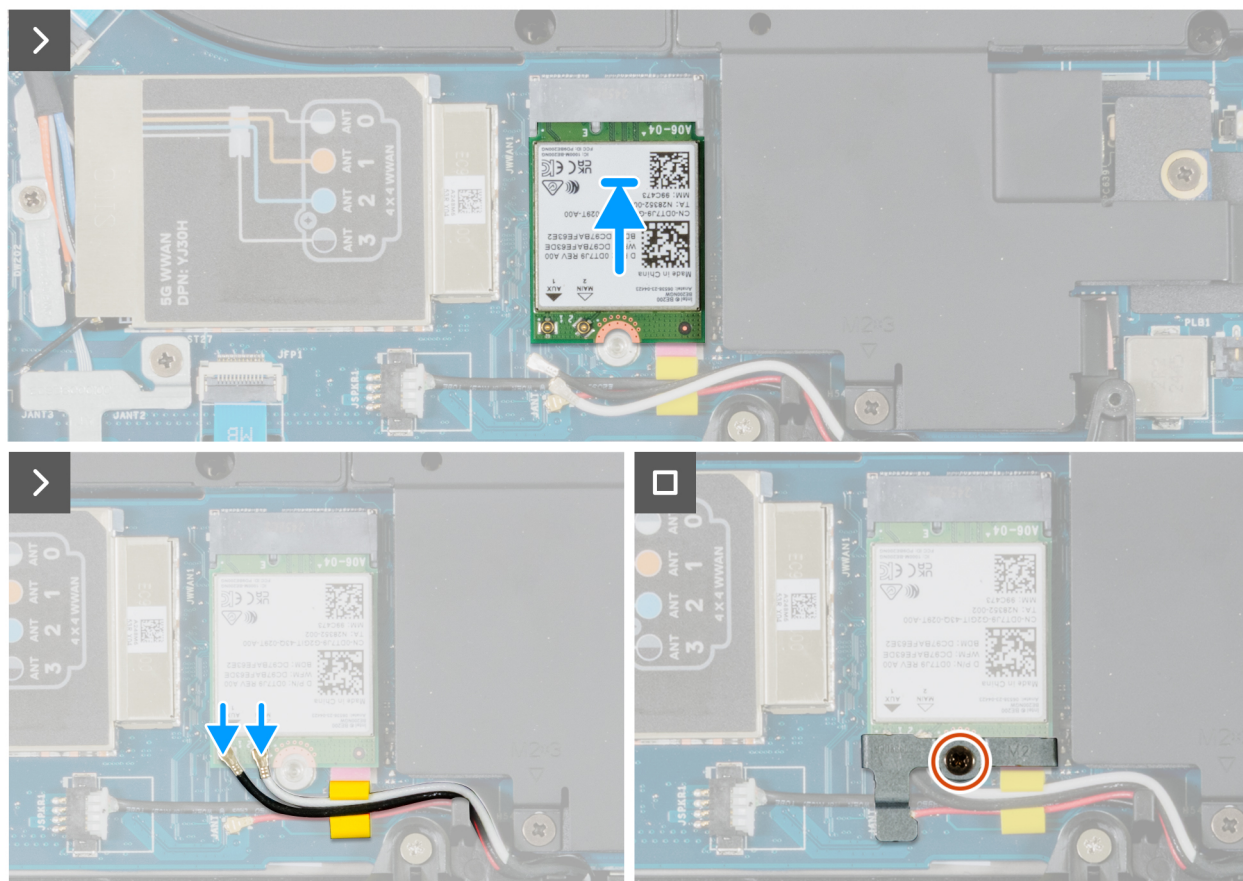
Figura 49. Installazione della scheda WLAN
