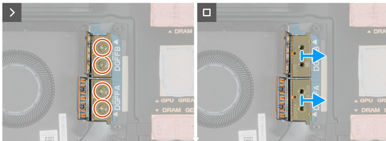
Figura 59. Rimozione del connettore del laser FPC dedicato
