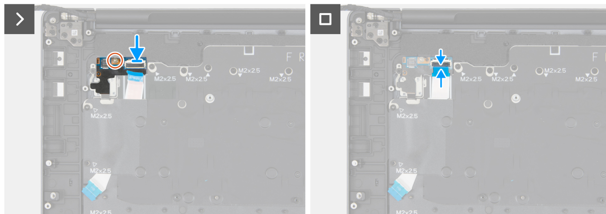
Figura 126. Installazione della scheda del pulsante di alimentazione
