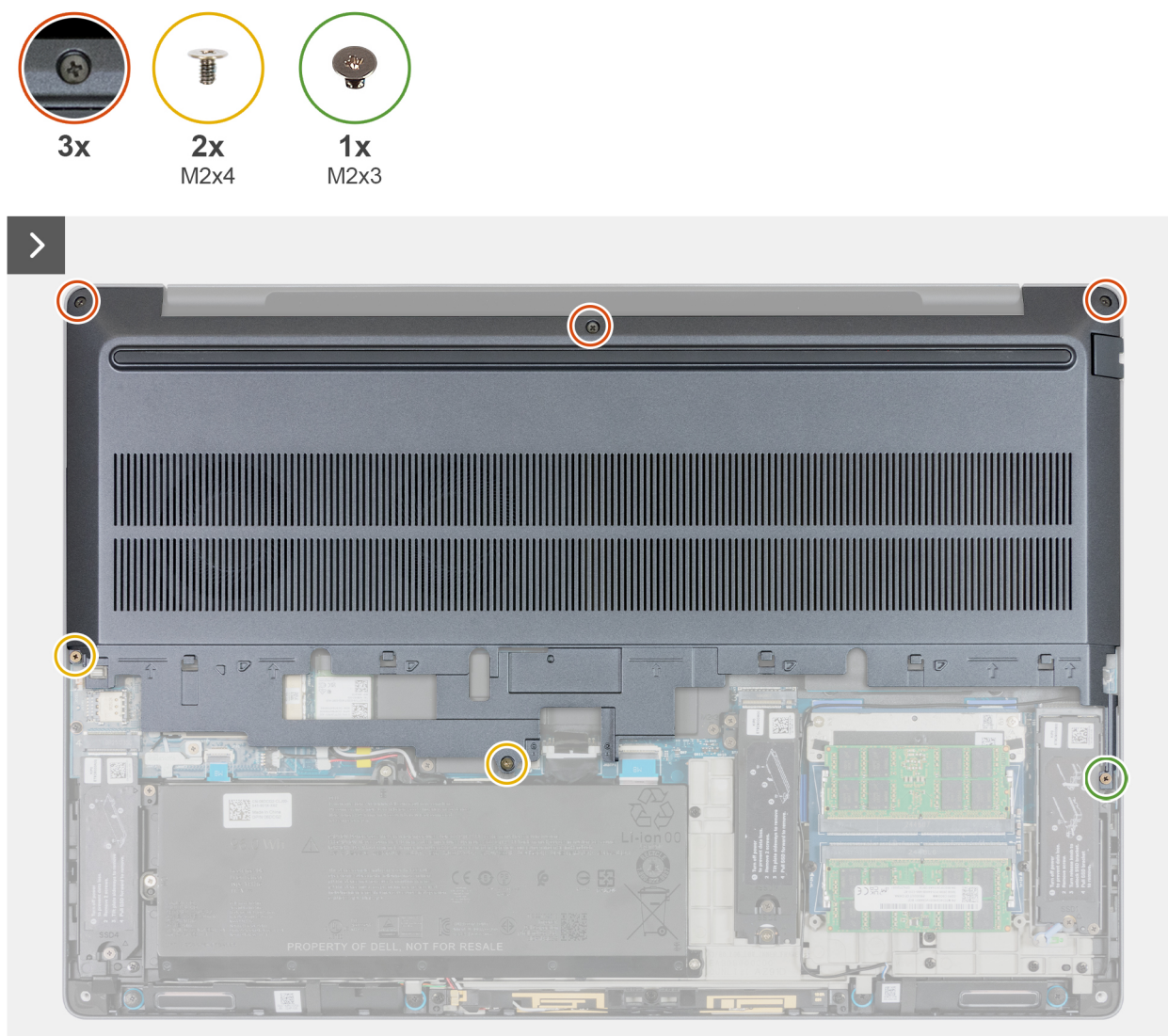
Figura 18. Allentamento delle tre viti di fissaggio e rimozione delle tre viti
