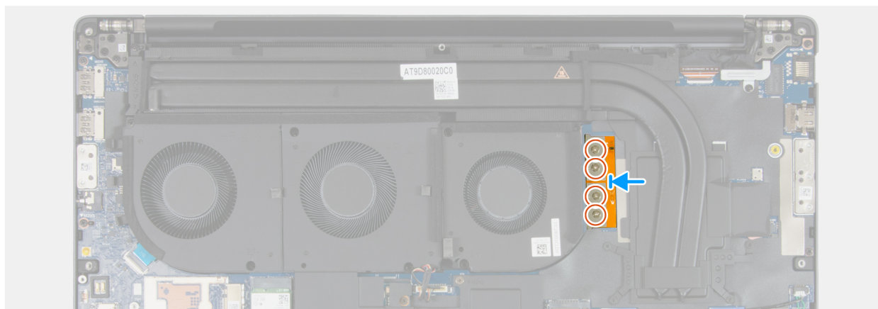
Figura 58. Installazione del connettore del laser FPC integrato
