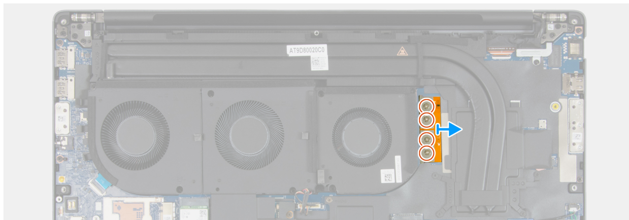
Figura 57. Rimozione del connettore del laser FPC integrato
