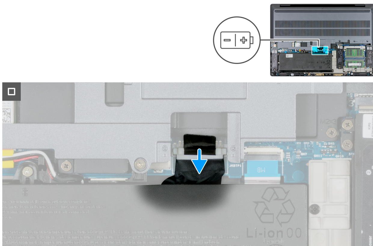
Figura 14. Scollegamento del cavo della batteria
