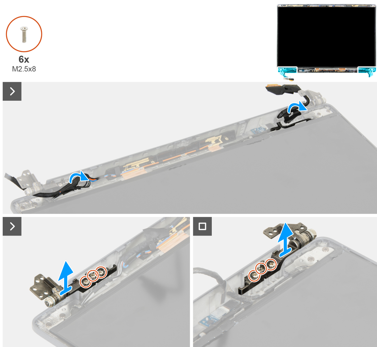
Figura 99. Rimozione delle cerniere del display
