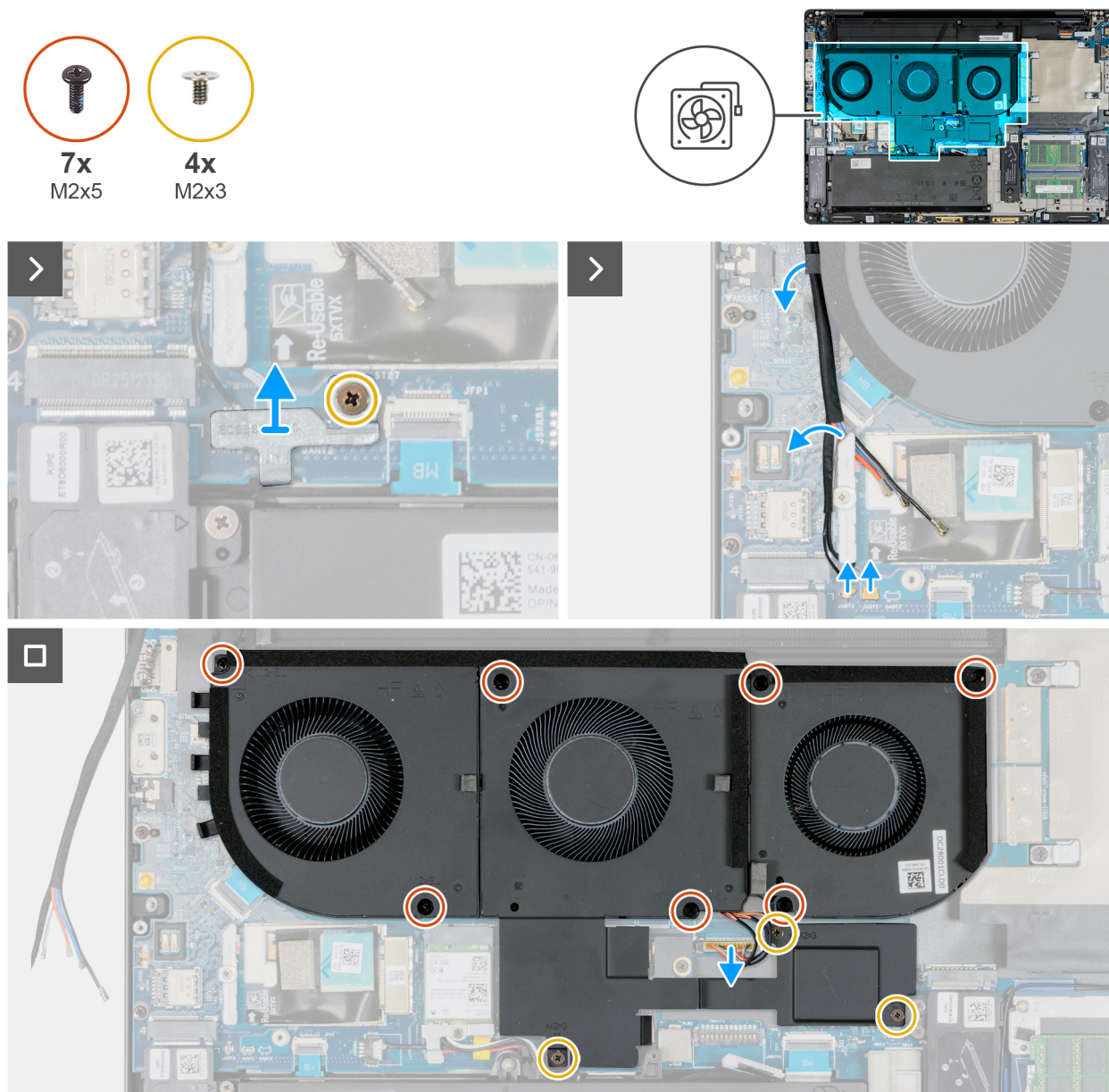
Figura 61. Rimozione del gruppo ventola
