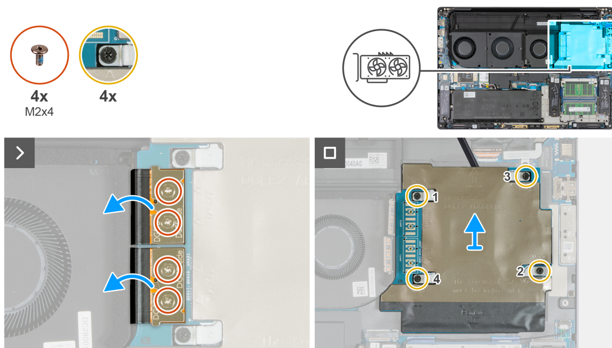
Figura 54. Rimozione della scheda GPU
