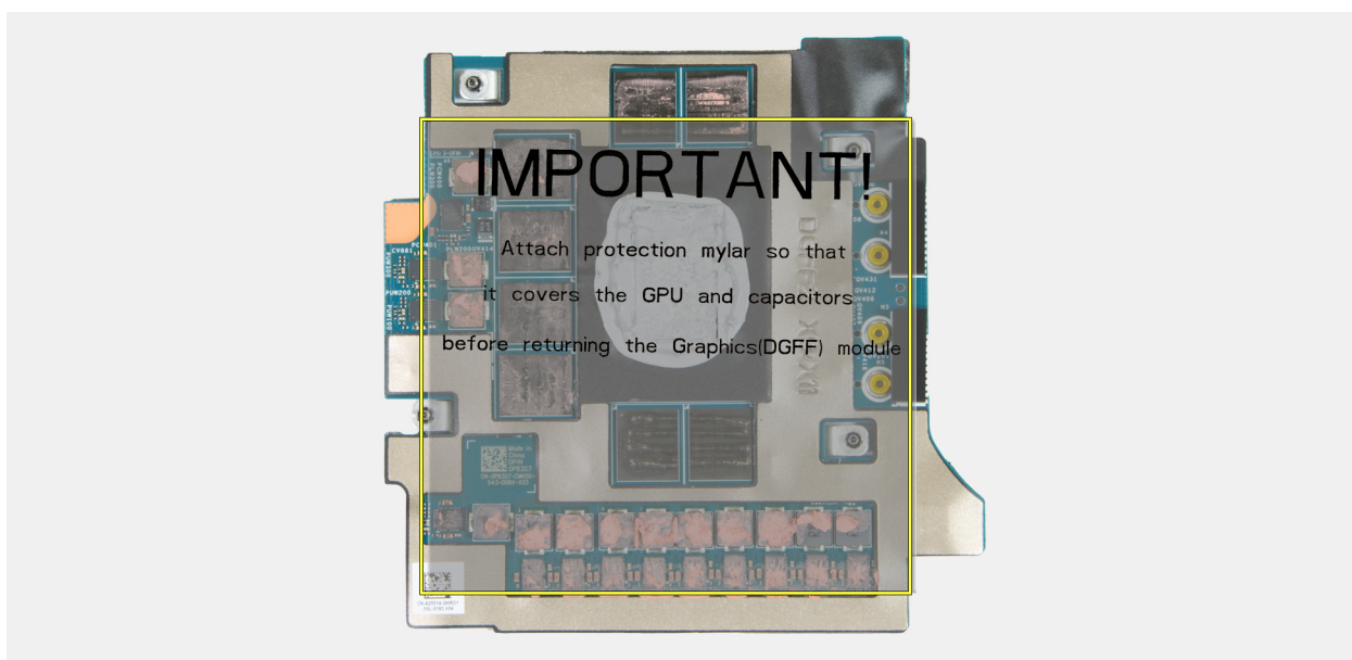
Figura 55. Preparazione della scheda GPU difettosa per la restituzione
