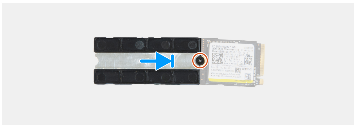
Figura 43. Installazione dell'SSD M.2 2230
