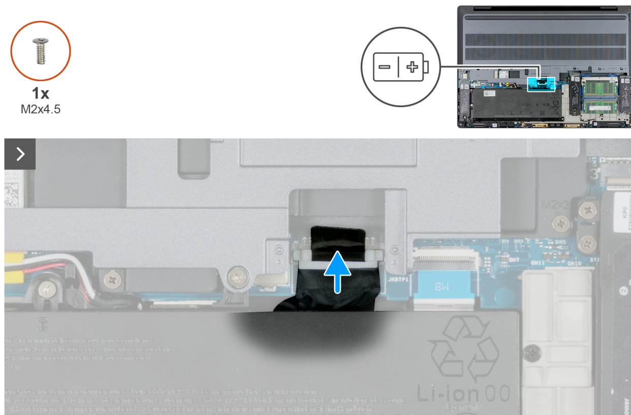
Figura 15. Collegamento del cavo della batteria
