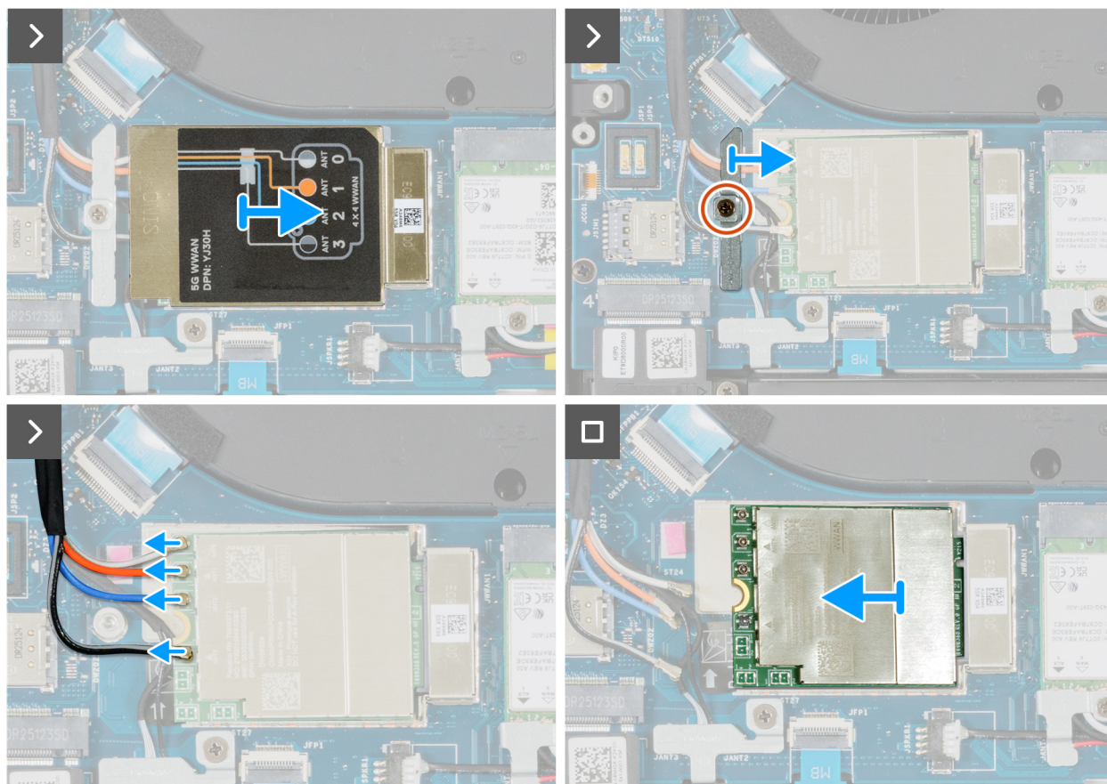
Figura 52. Rimozione della scheda WWAN
