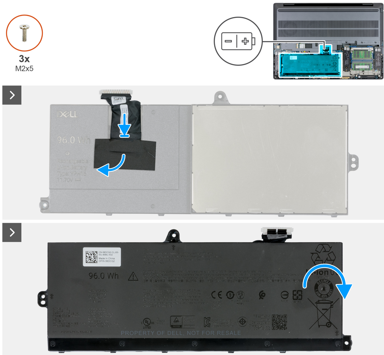
Figura 46. Ricollocamento del cavo della batteria
