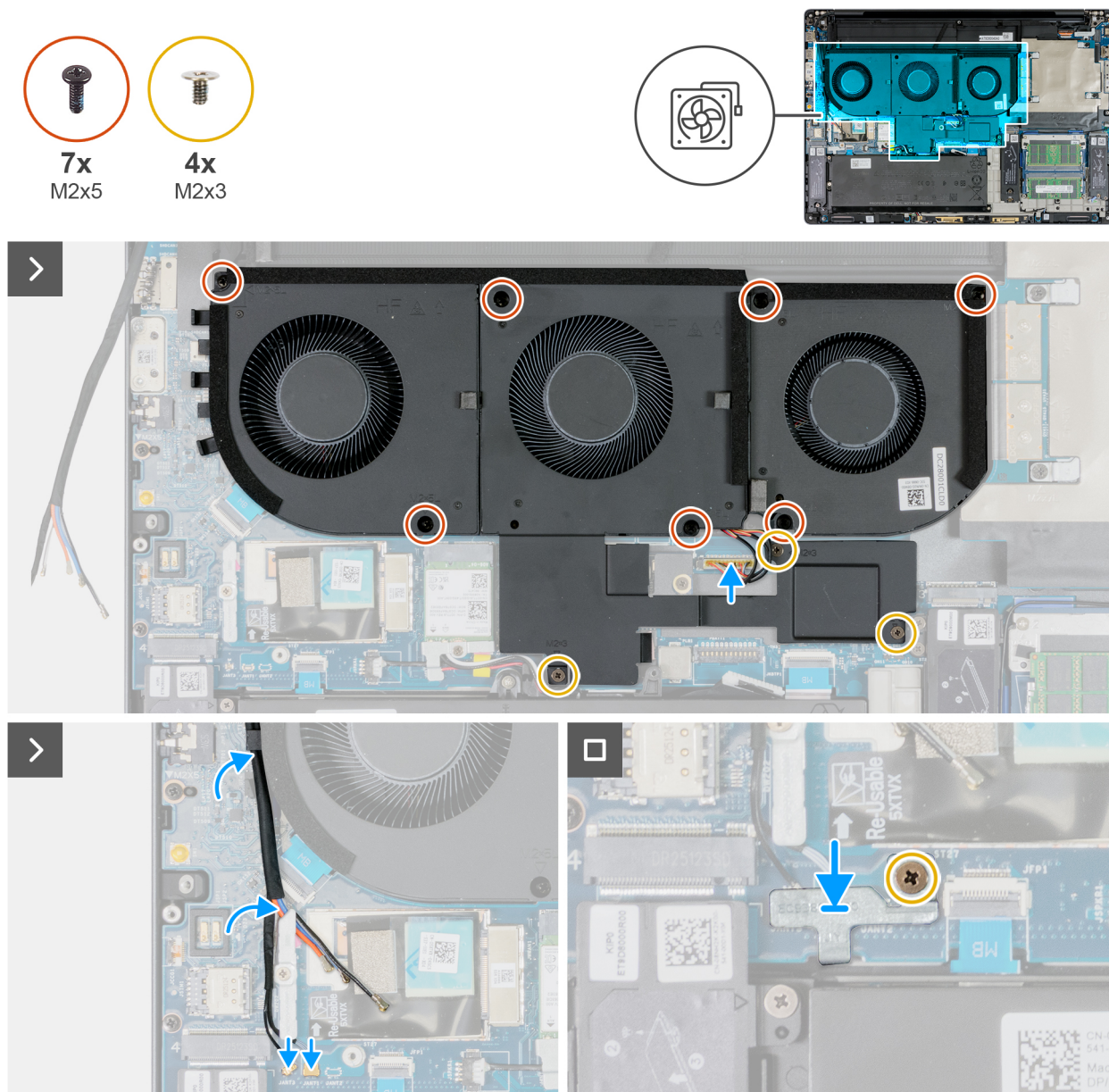
Figura 62. Installazione del gruppo ventola
