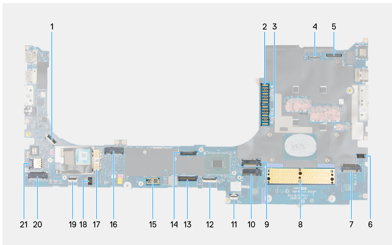
Figura 110. Connettori scheda di sistema
