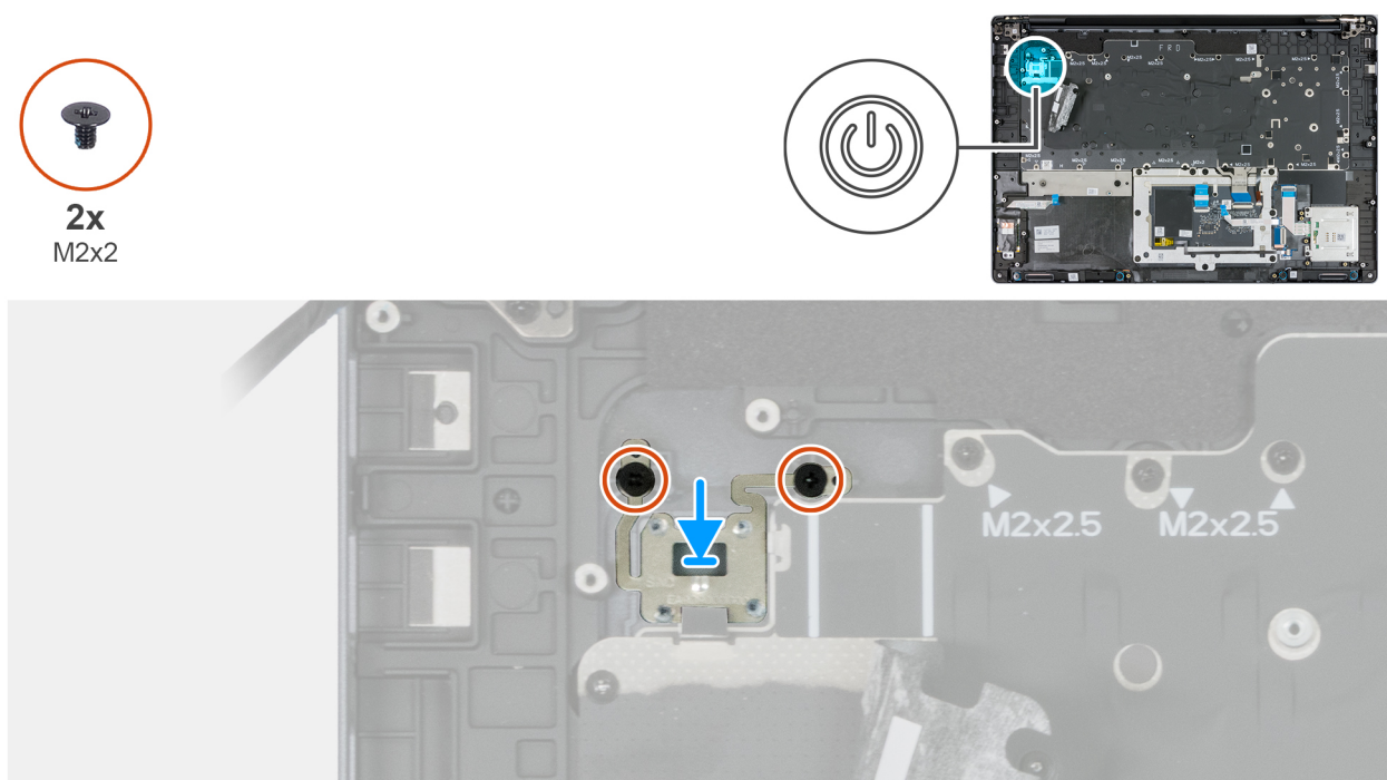
Figura 128. Installazione del pulsante di accensione
