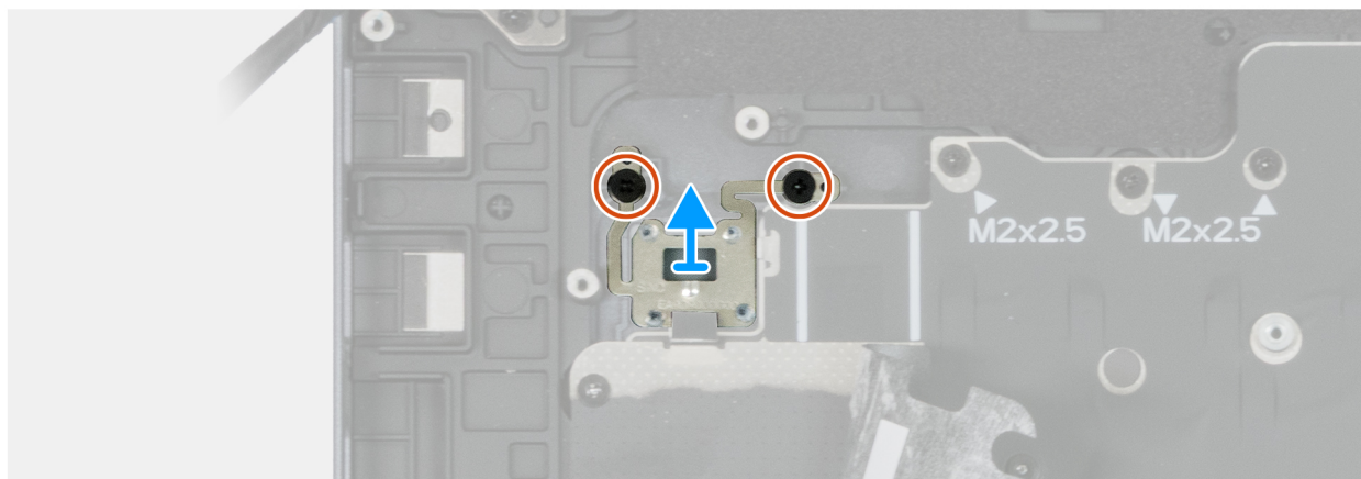
Figura 127. Rimozione del pulsante di accensione
