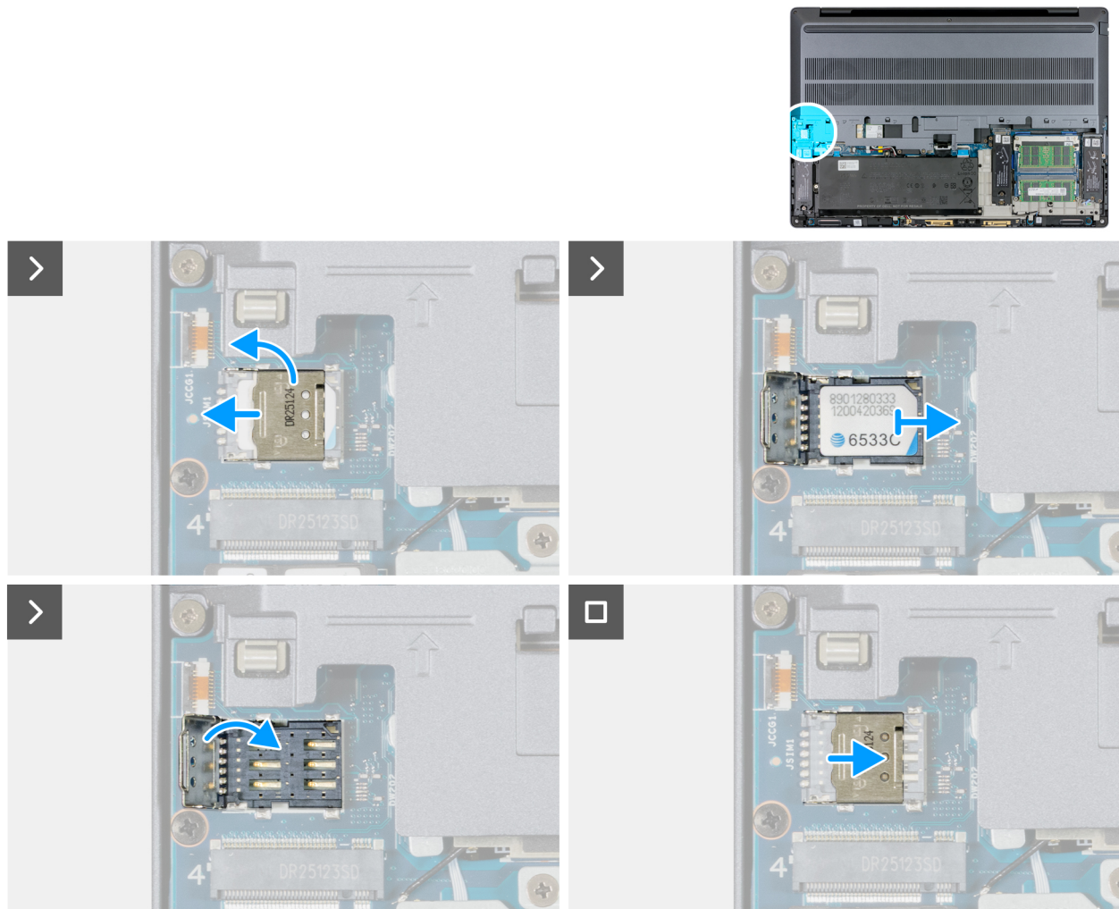
Figura 50. Rimozione della scheda SIM
