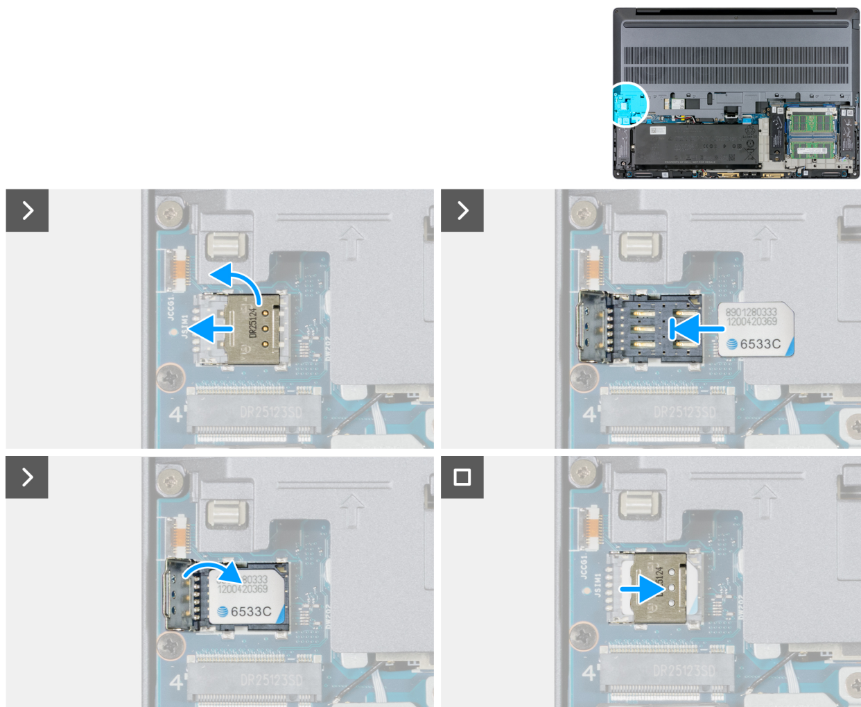
Figura 51. Installazione della scheda SIM
