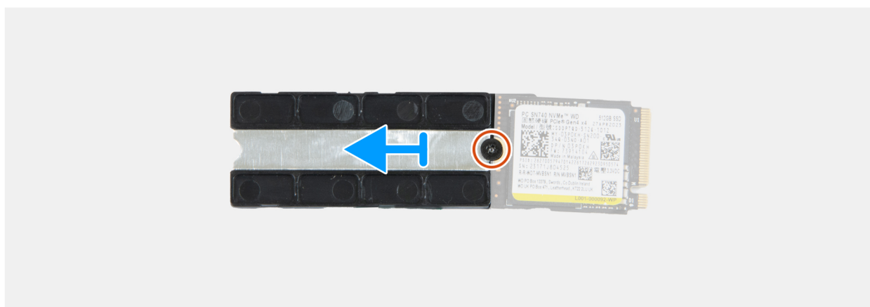
Figura 42. Rimozione dell'SSD M.2 2230
