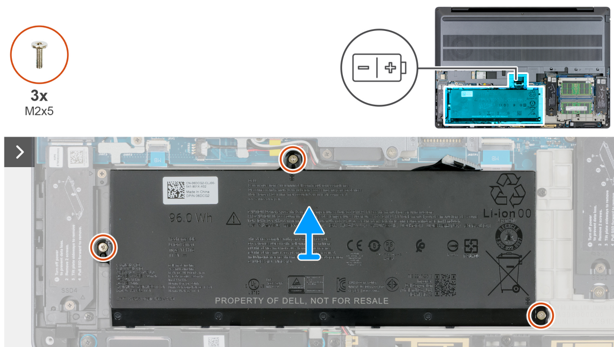
Figura 44. Rimozione della batteria
