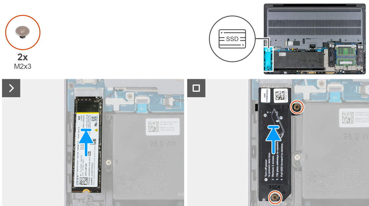
Figura 41. Installazione dell'SSD M.2 2280 nello slot 4 (SSD4)
