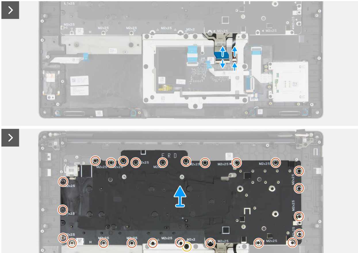
Figura 117. Rimozione della tastiera
