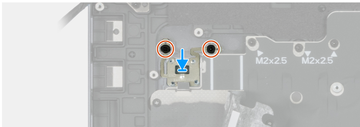
Figura 128. Installazione del pulsante di accensione
