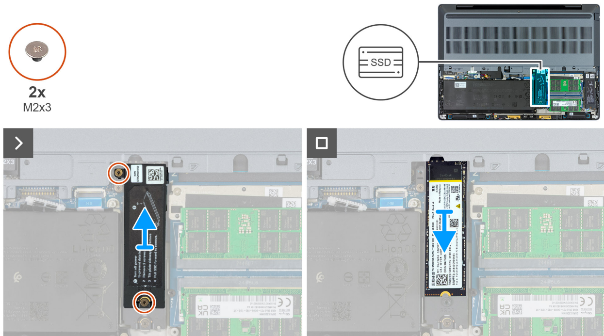
Figura 36. Rimozione dell'SSD M.2 2280 dallo slot 3 (SSD3)
