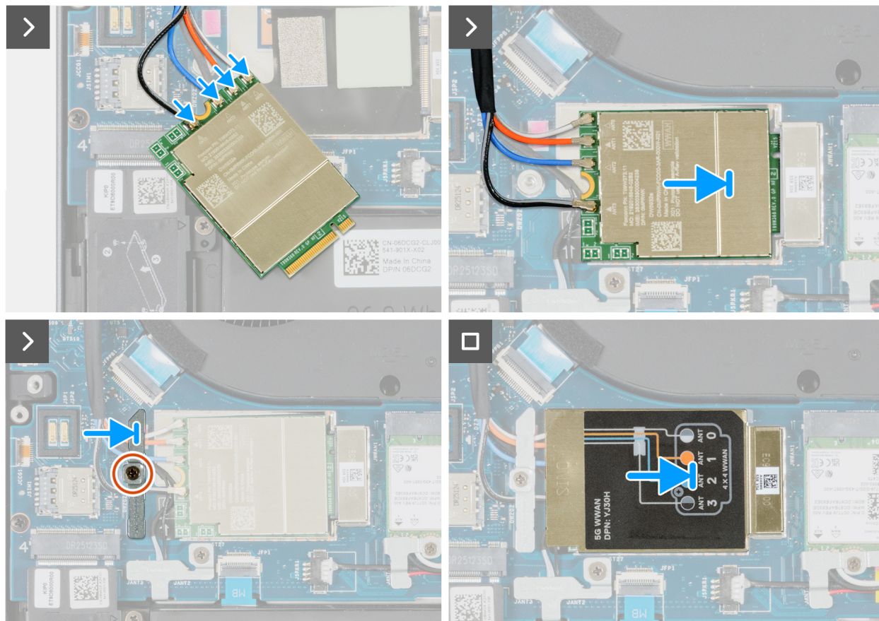
Figura 53. Installazione della scheda WWAN
