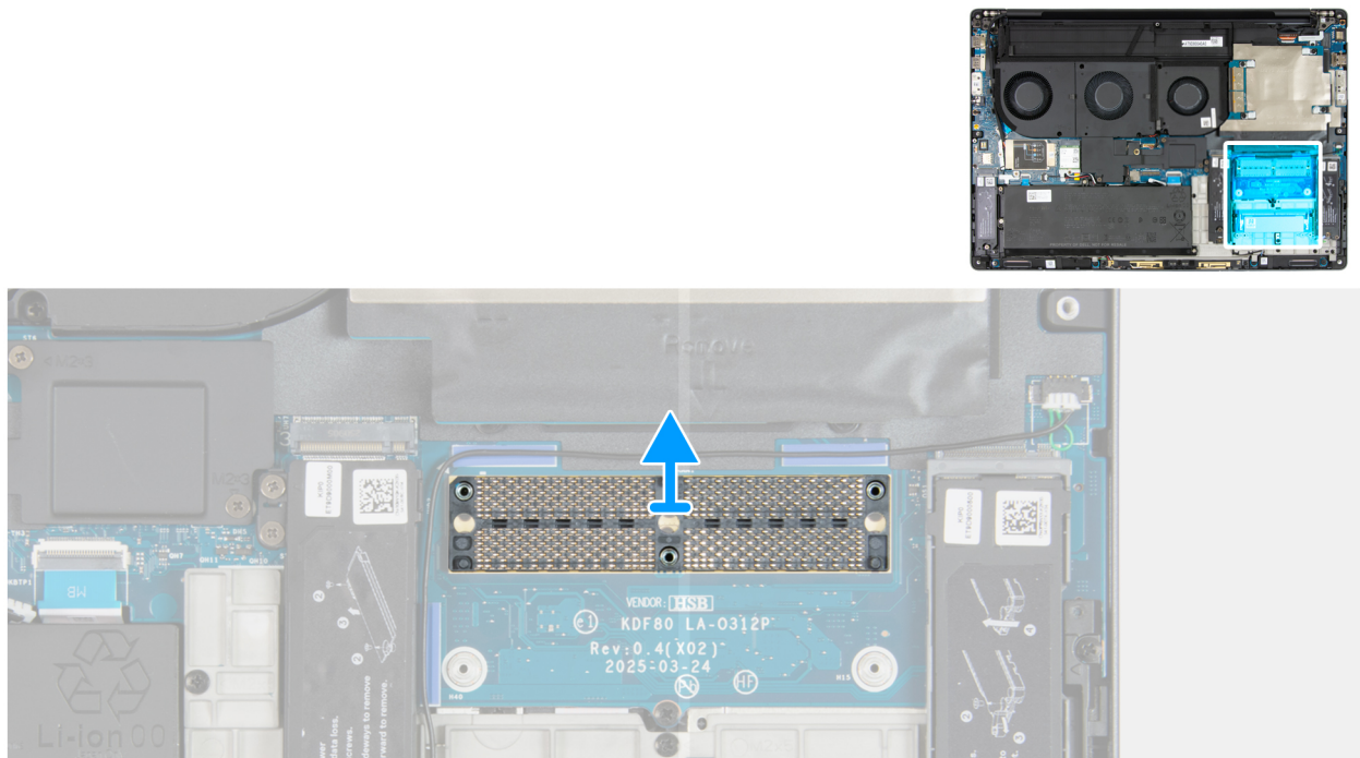
Figura 69. Rimozione del connettore della memoria
