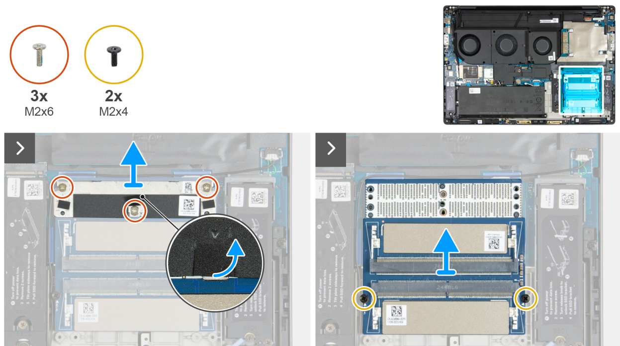
Figura 67. Rimozione della scheda interposer della memoria
