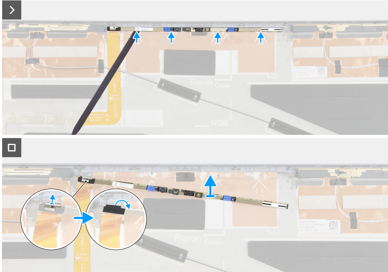
Figura 101. Rimozione del modulo della fotocamera
