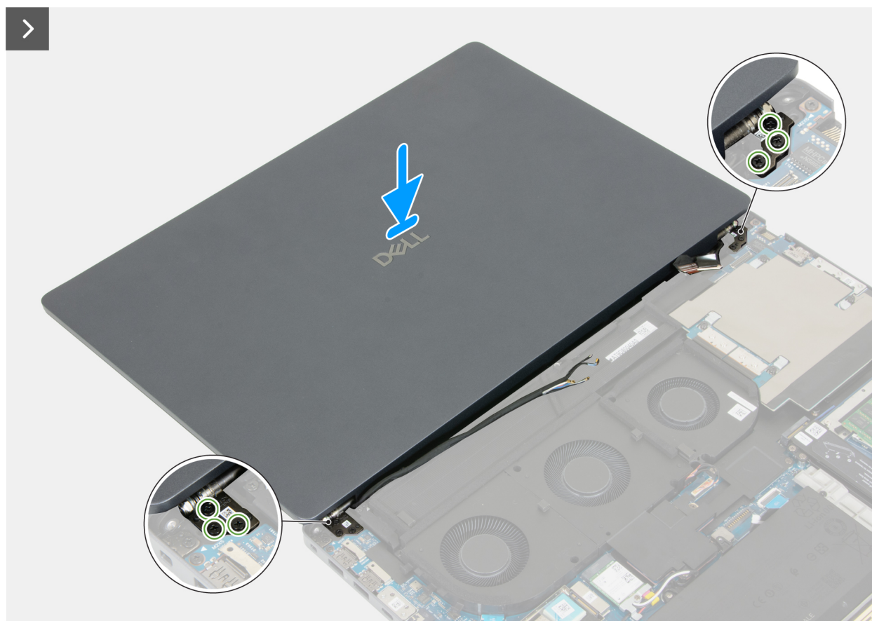
Figura 65. Installazione del gruppo del display
