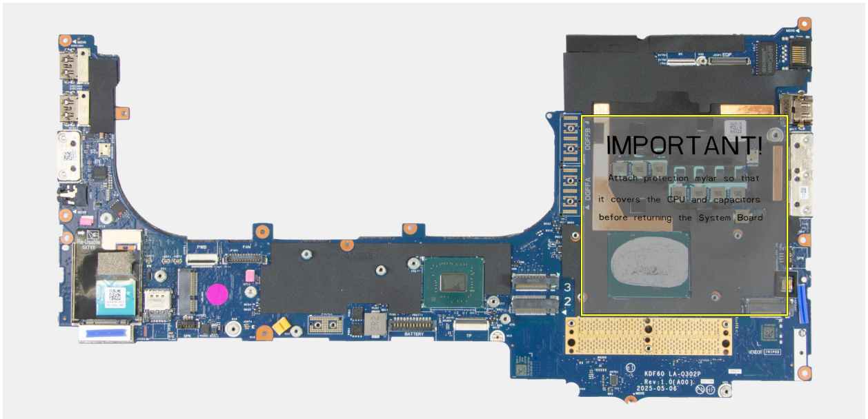
Figura 109. Preparazione della scheda di sistema difettosa per la restituzione
