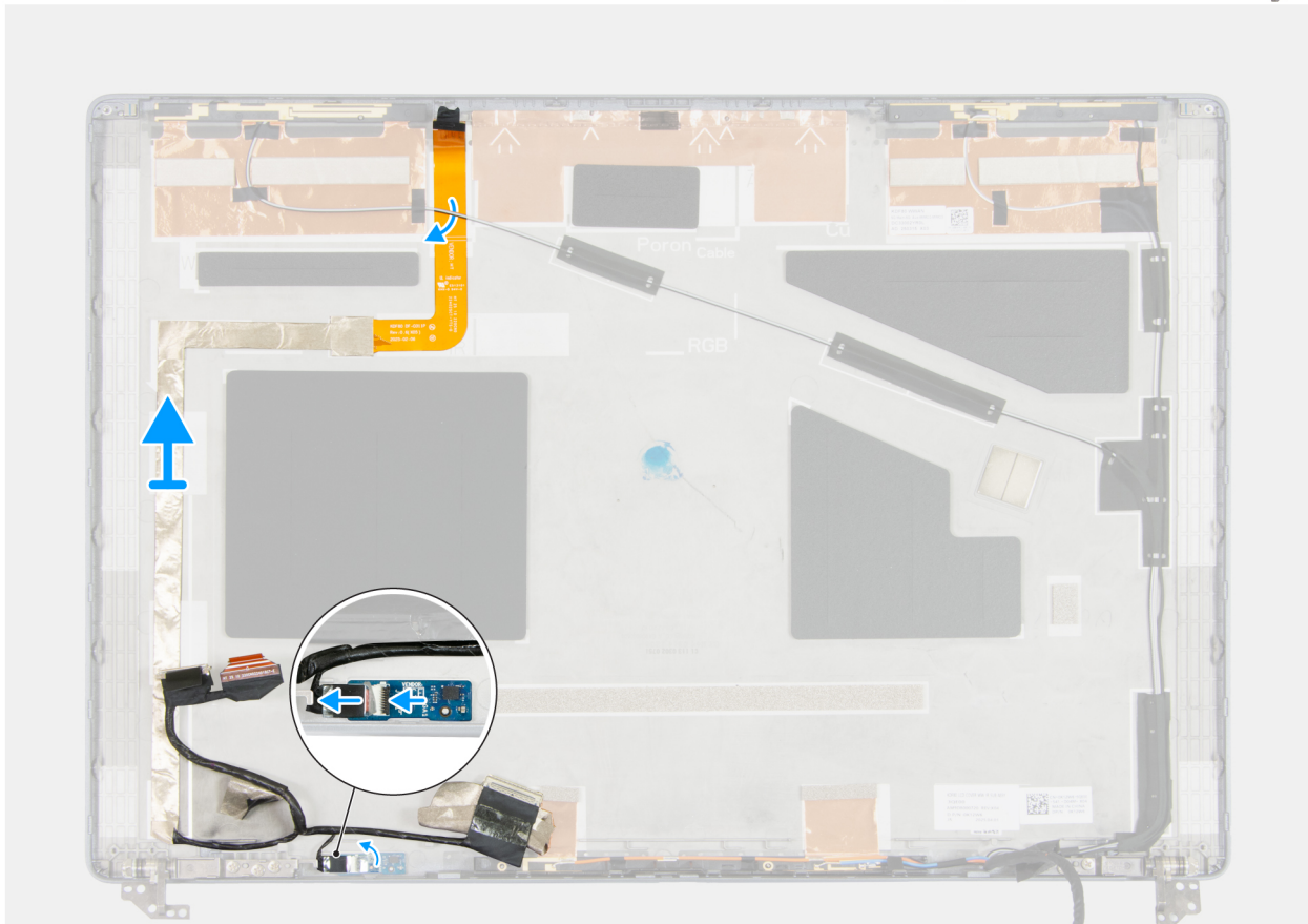
Figura 102. Rimozione del cavo del display
