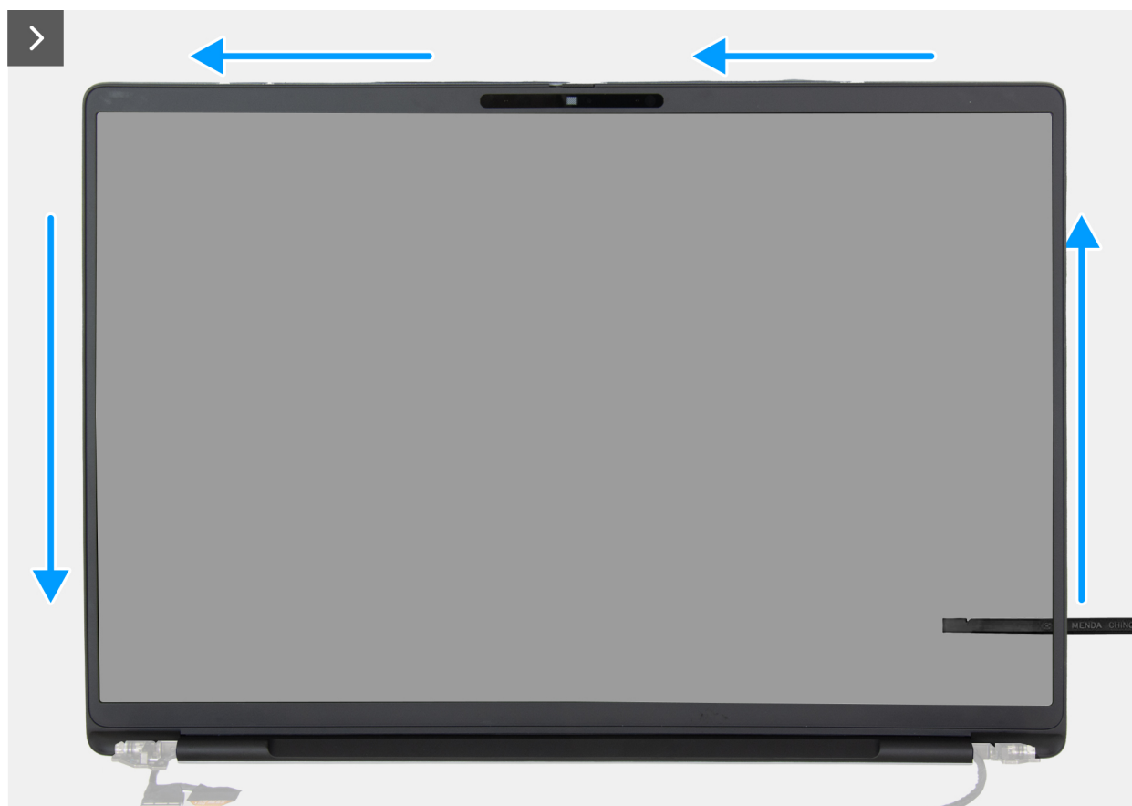
Figura 85. Rimozione della cornice del display
