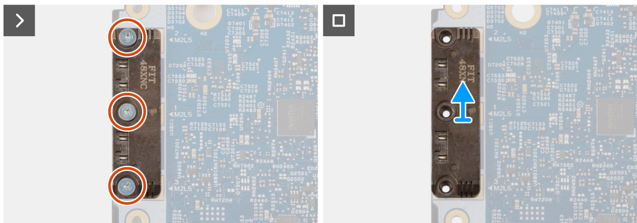
Figura 75. Rimozione del modulo USB Type-C
