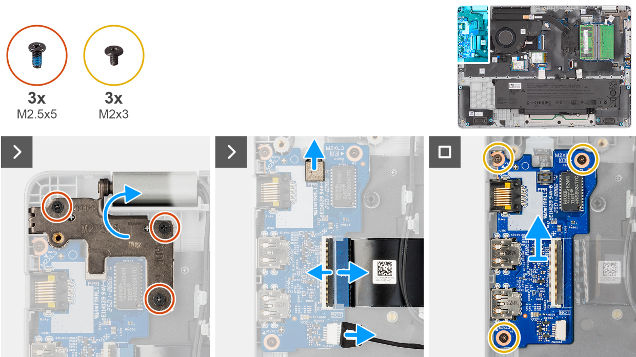
Figura 51. Rimozione della scheda di I/O
