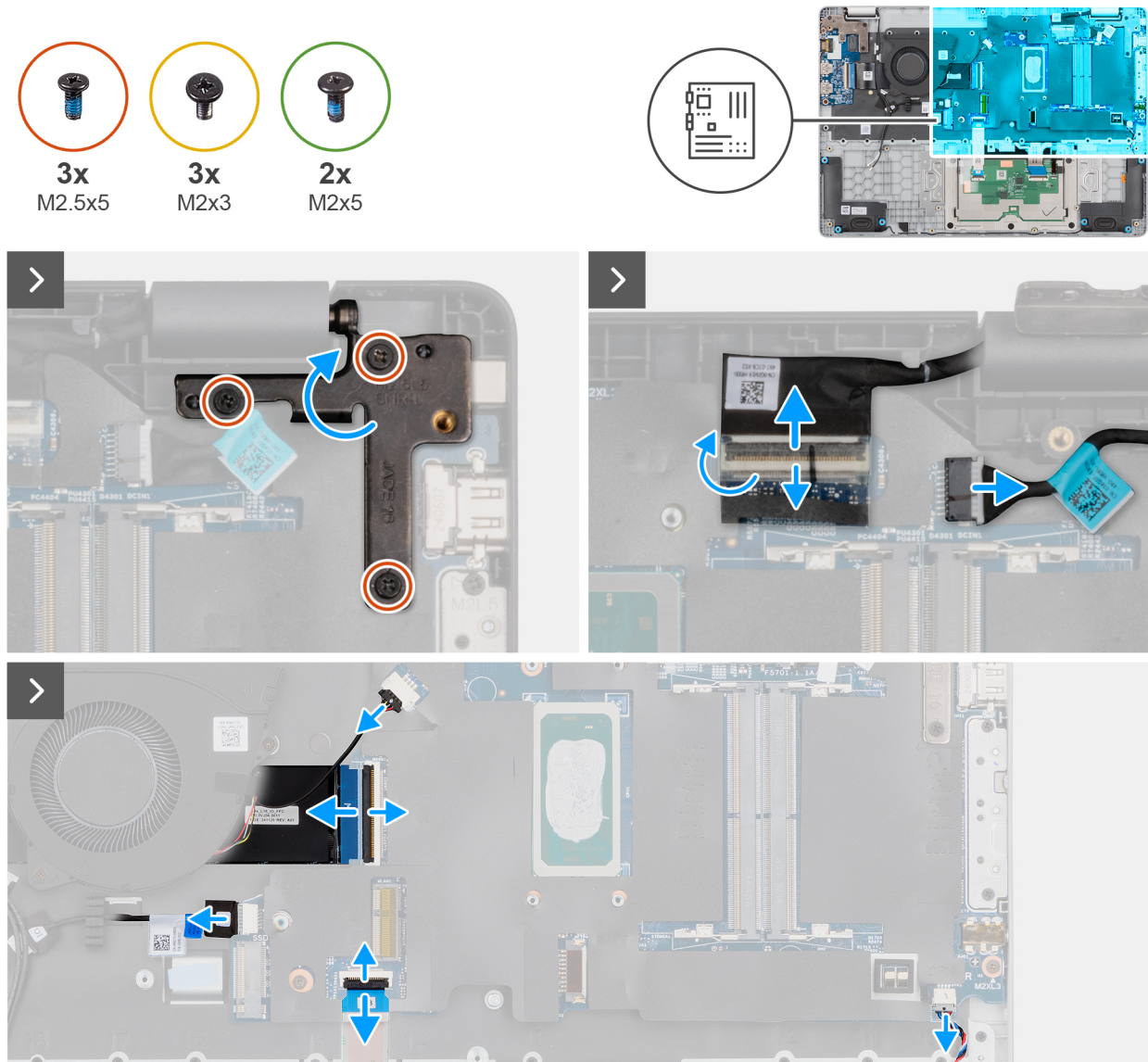
Figura 64. Rimozione della scheda di sistema
