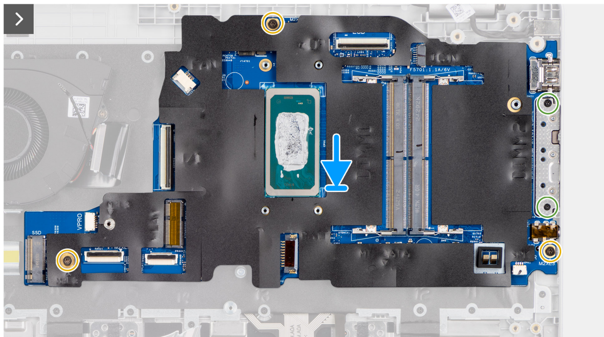
Figura 73. Installazione della scheda di sistema
