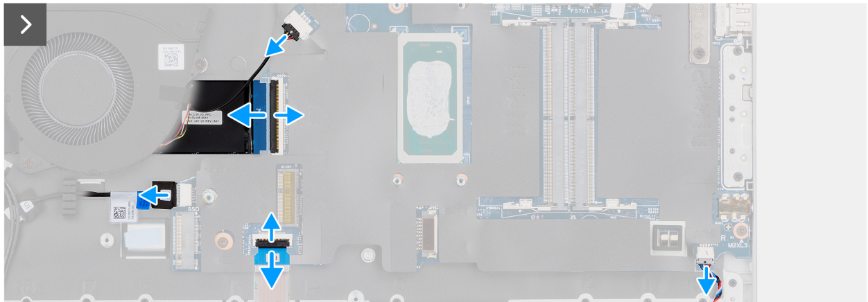
Figura 64. Rimozione della scheda di sistema
