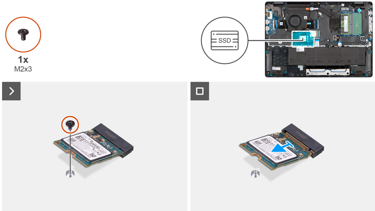
Figura 23. Rimozione dell'SSD
