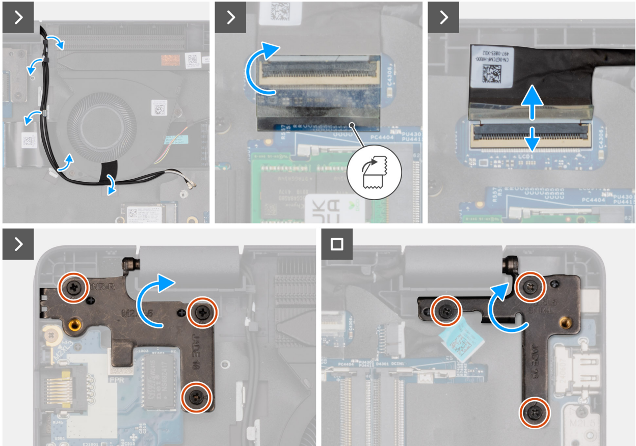
Figura 93. Rimozione del gruppo del display
