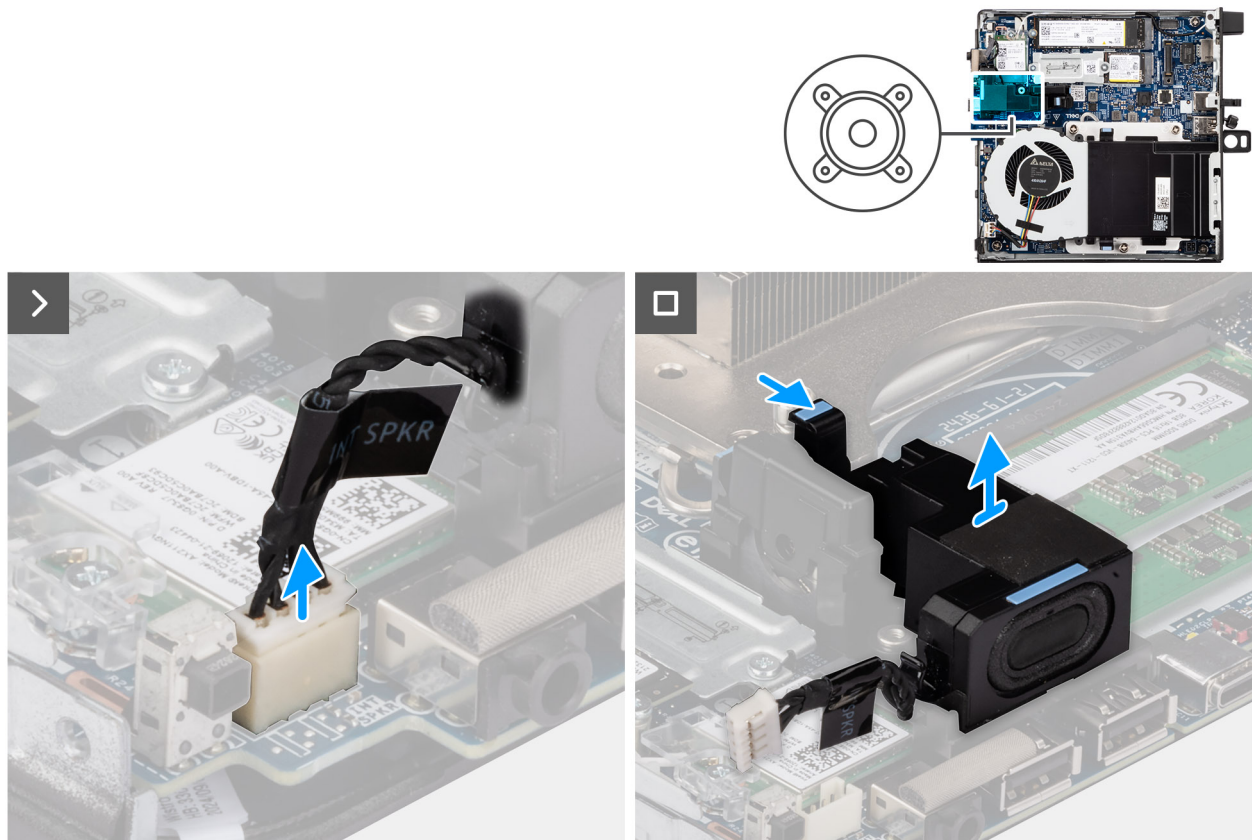
Figura 14. Rimozione dell'altoparlante
