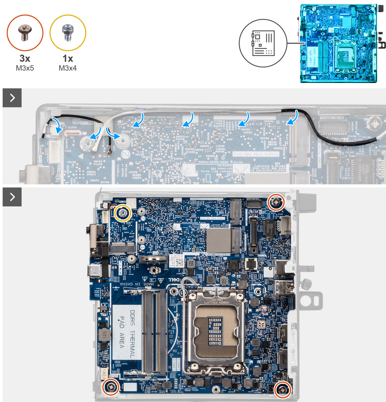
Figura 75. Rimozione della scheda di sistema
