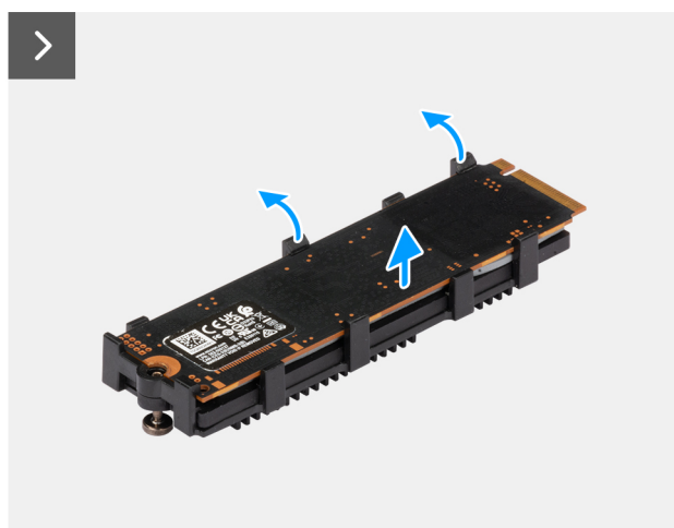
Figura 24. Rimozione dell'unità SSD M.2 2280 PCIe
