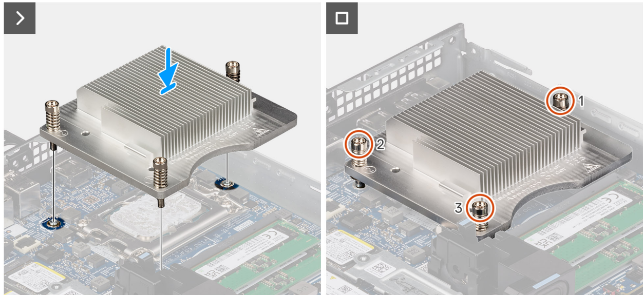
Figura 63. Installazione del dissipatore di calore
