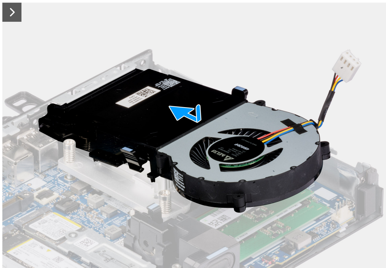
Figura 31. Installazione della ventola
