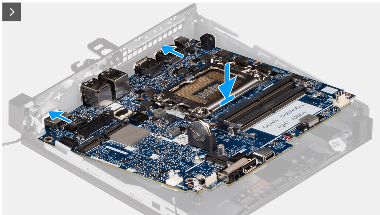
Figura 78. Installazione della scheda di sistema
