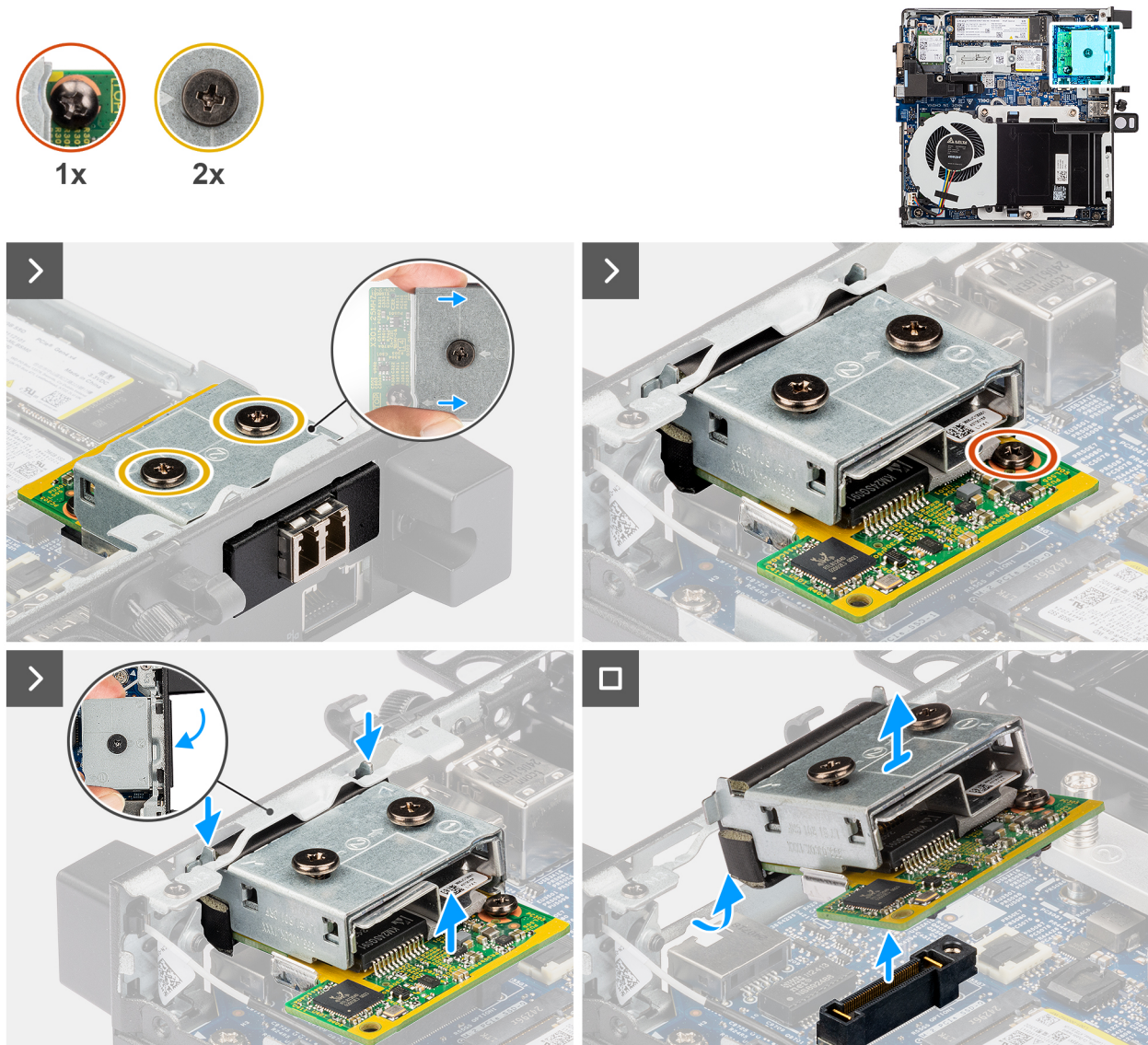
Figura 59. Rimozione del modulo della porta in fibra ottica
