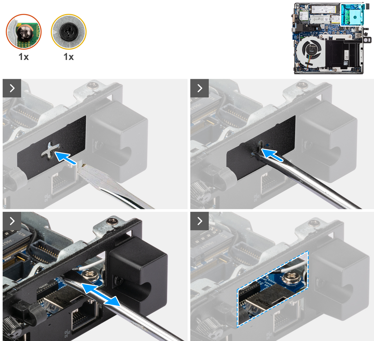
Figura 51. Installazione del modulo della porta VGA
