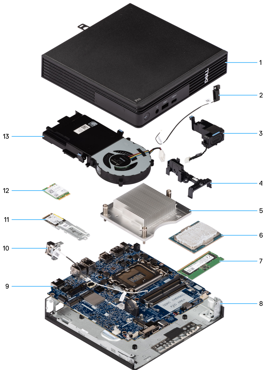
Figura 9. Componenti principali di Dell Pro con fattore di forma micro GCM1250
