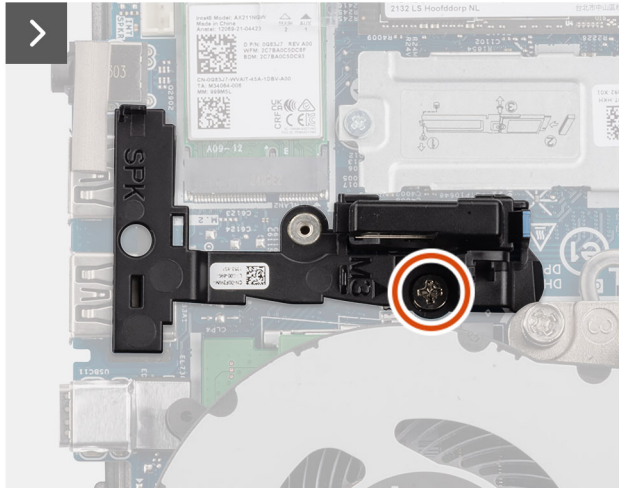
Figura 72. Rimozione del supporto degli altoparlanti
