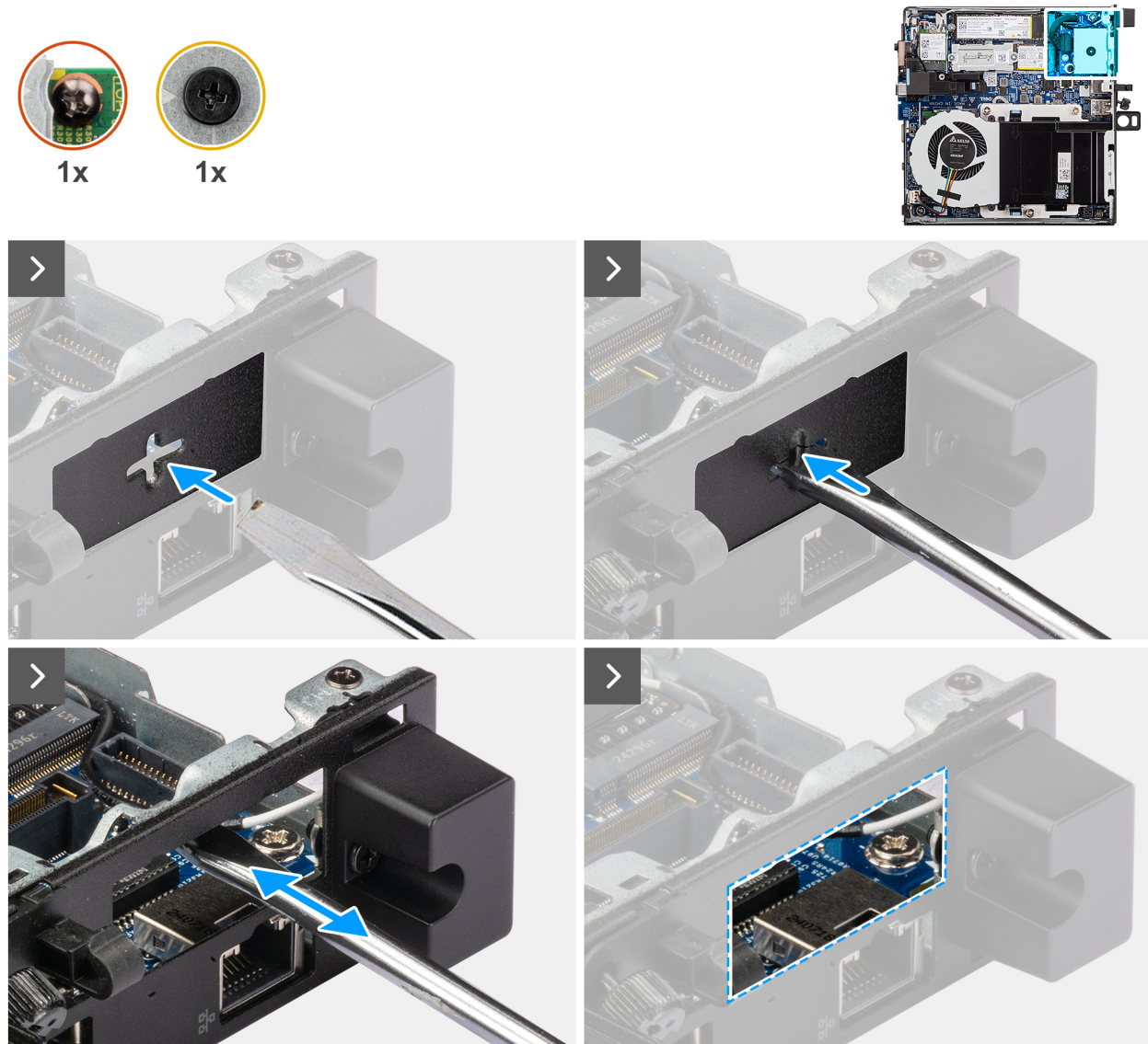
Figura 57. Installazione del modulo della porta seriale
