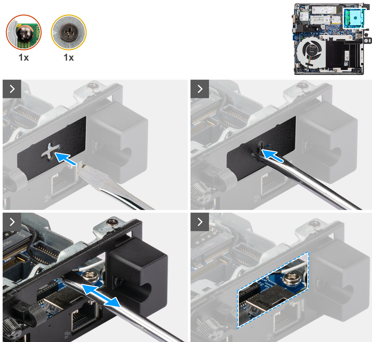
Figura 45. Installazione del modulo DisplayPort
