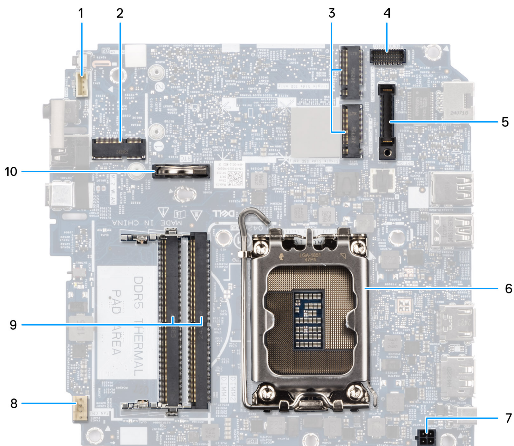
Figura 74. Connettori della scheda di sistema
