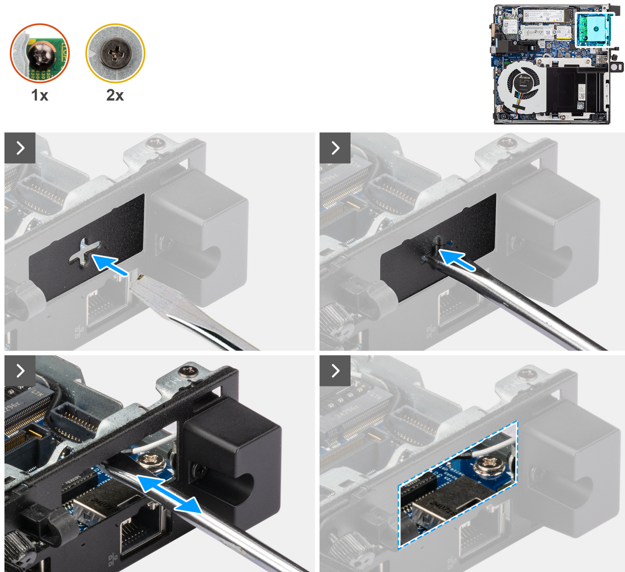
Figura 60. Installazione del modulo della porta in fibra ottica
