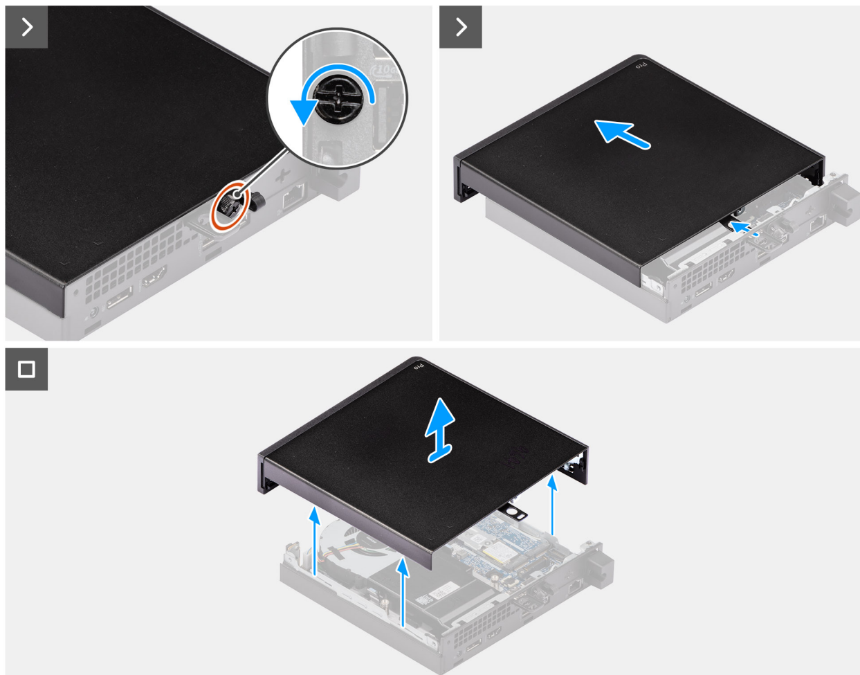
Figura 10. Rimozione del coperchio laterale
