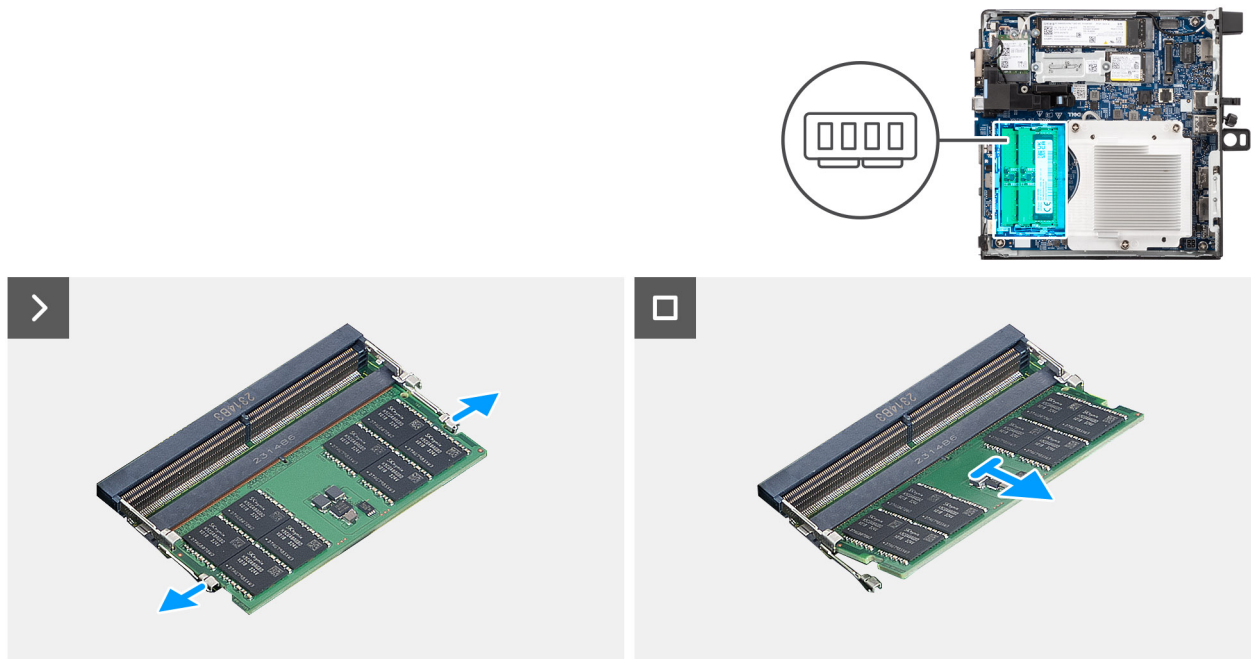
Figura 32. Rimozione del modulo di memoria
