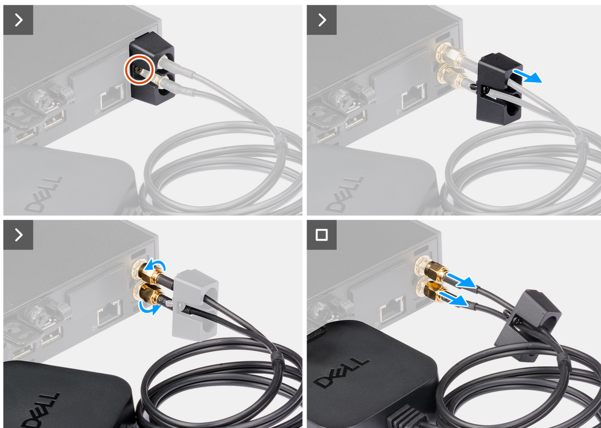
Figura 34. Rimozione dell'antenna a disco esterna
