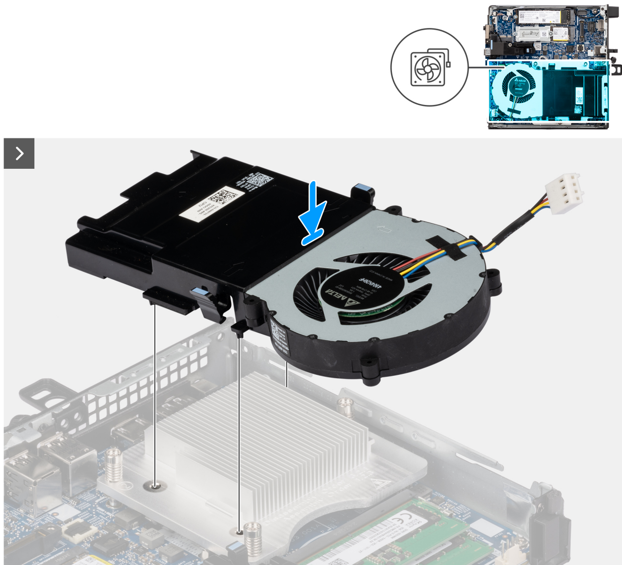
Figura 30. Installazione della ventola
