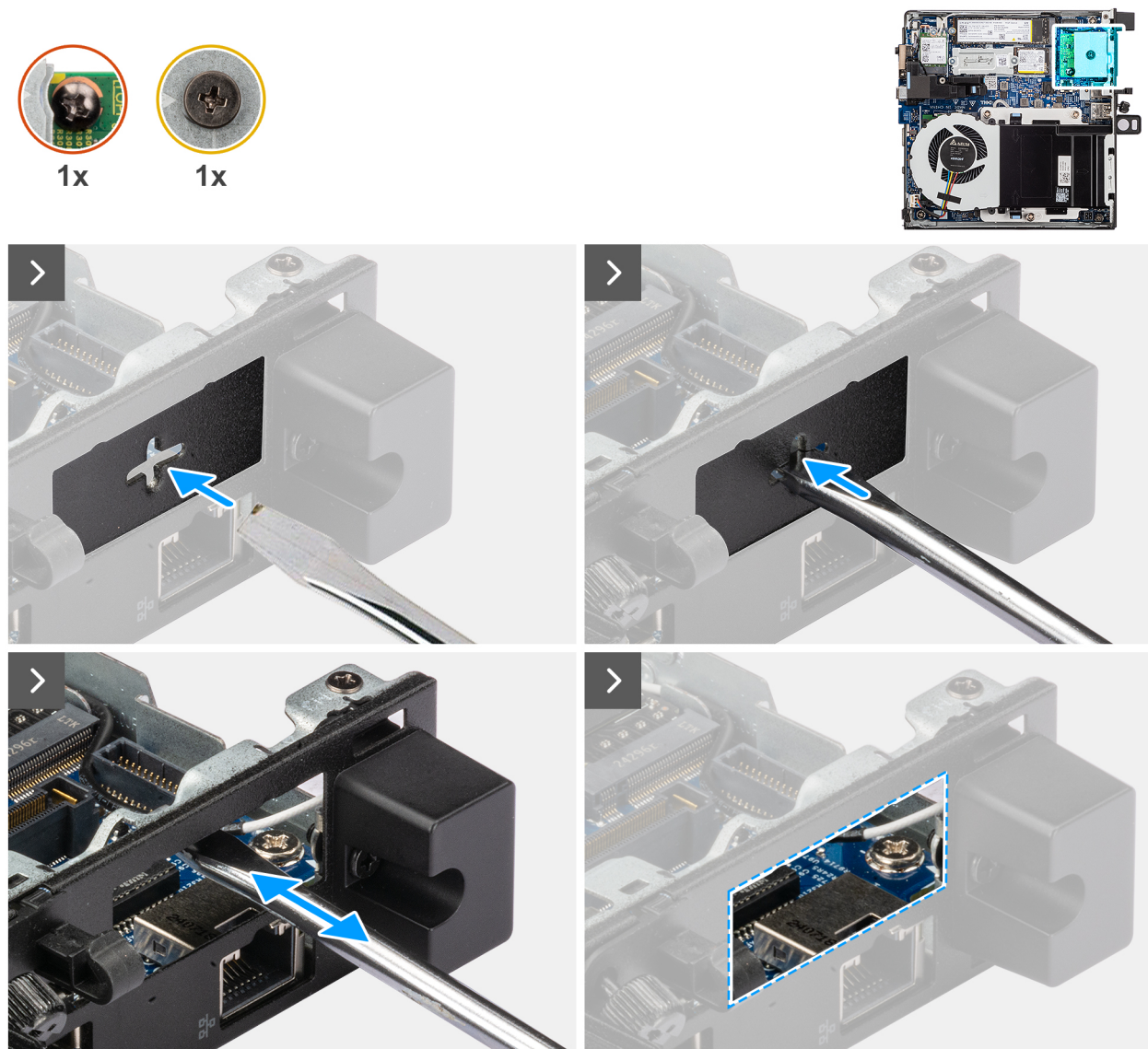
Figura 42. Installazione del modulo della porta USB Type-C
