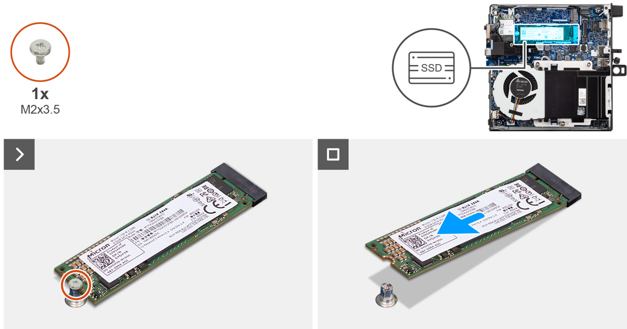
Figura 19. Rimozione dell'unità SSD M.2 2280
