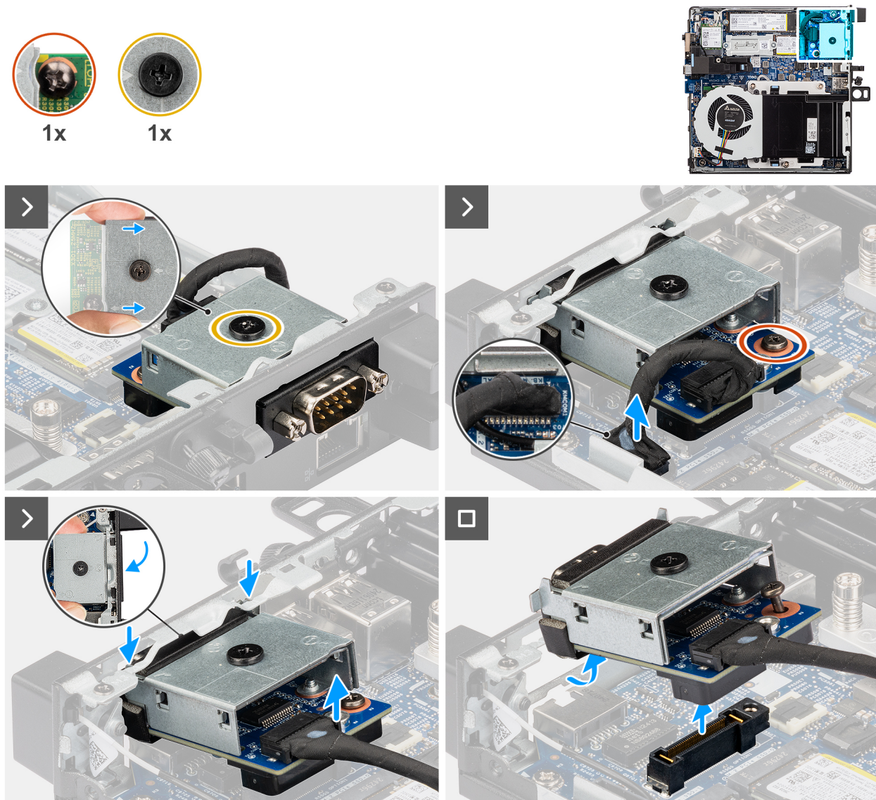
Figura 56. Rimozione del modulo della porta seriale
