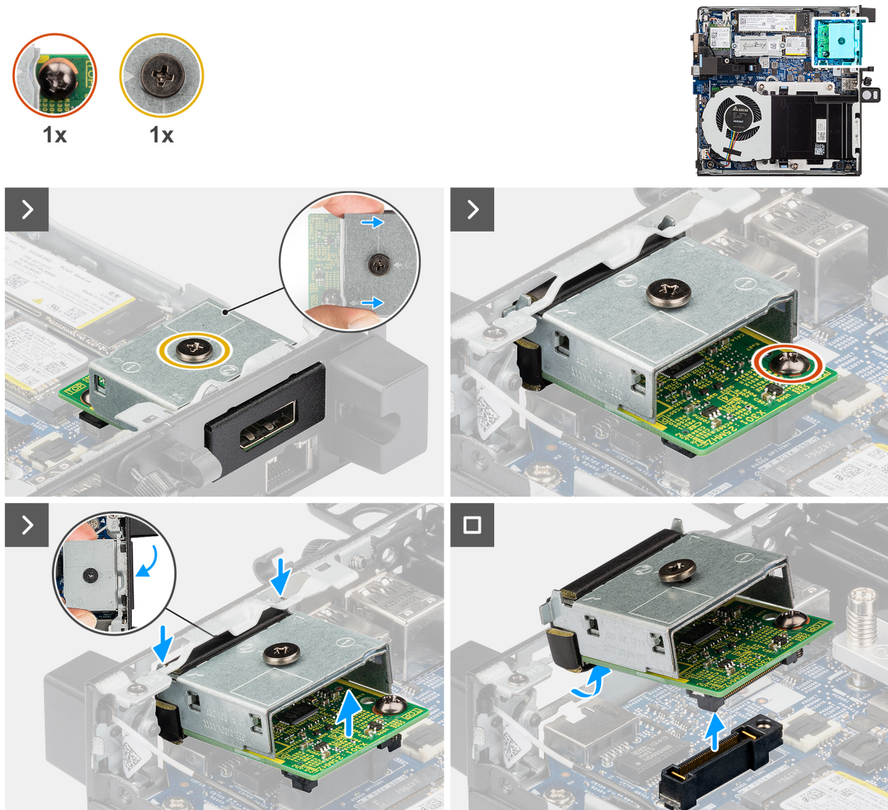
Figura 44. Rimozione del modulo DisplayPort
