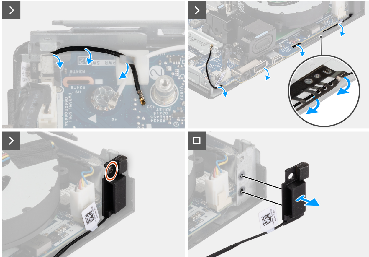
Figura 64. Rimozione del modulo dell'antenna (cavo nero)
