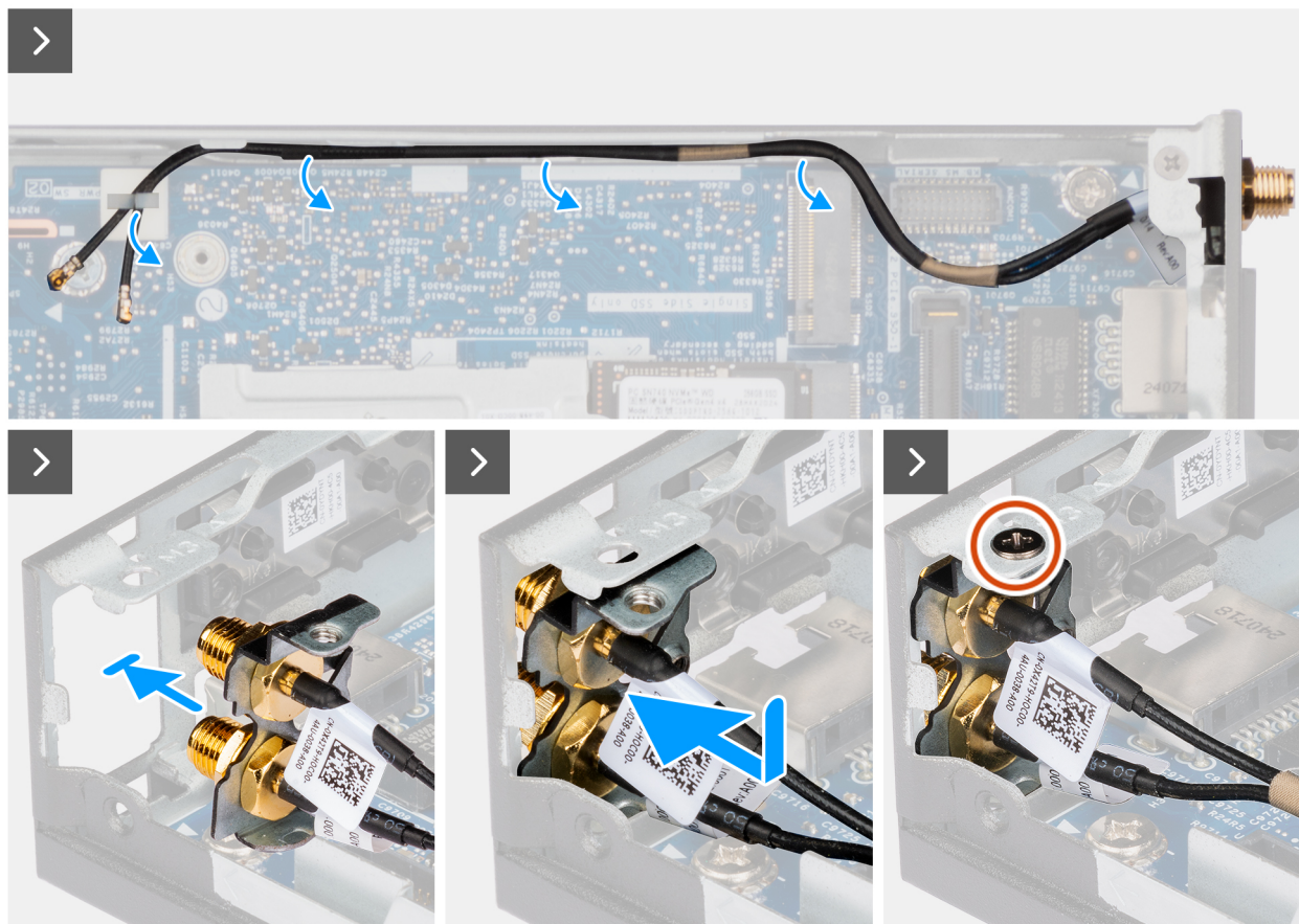
Figura 37. Installazione del modulo dell'antenna SMA
