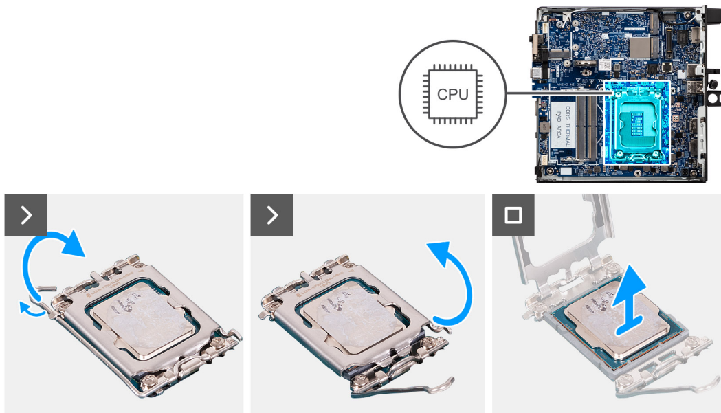
Figura 70. Rimozione del processore
