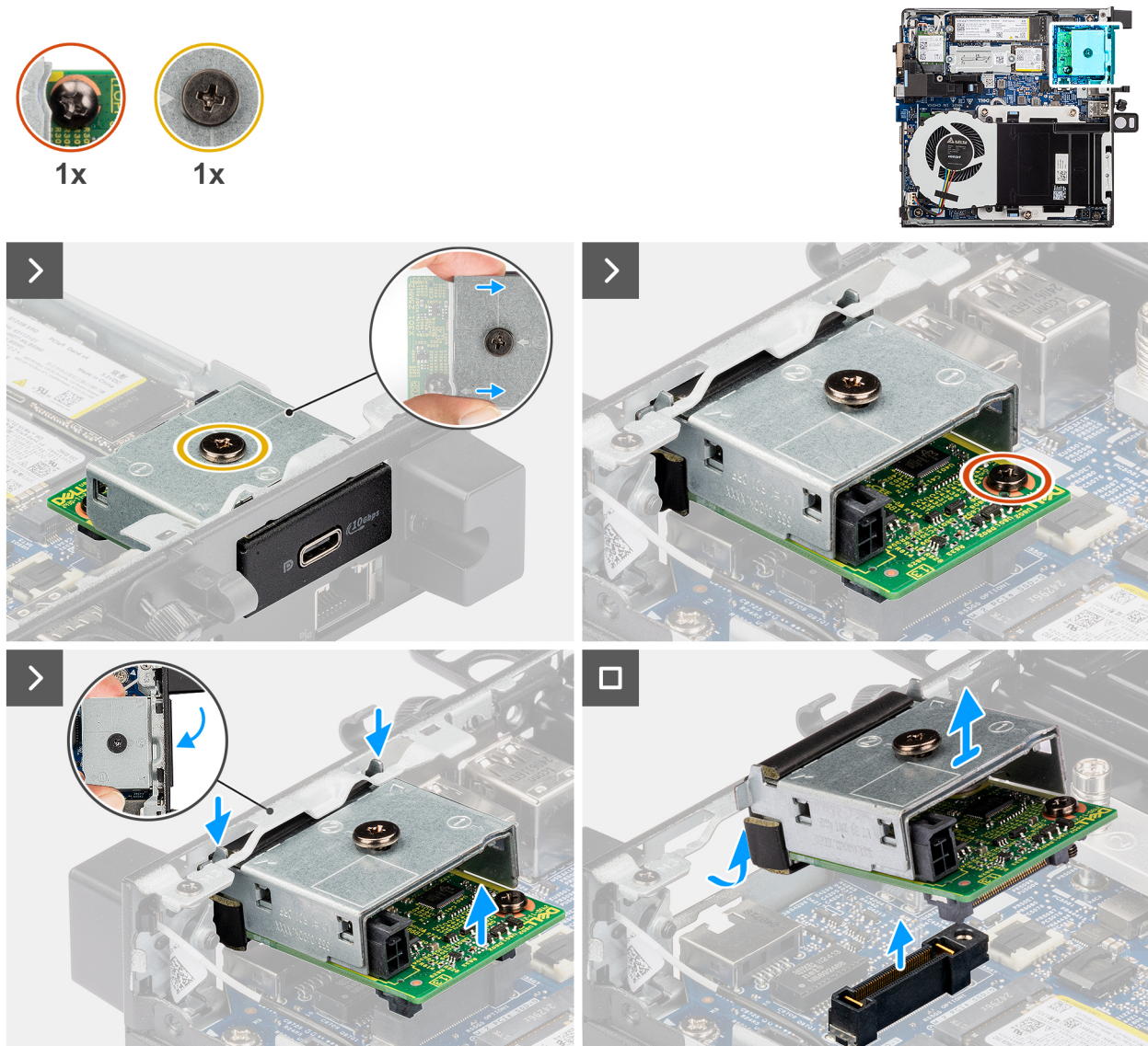
Figura 41. Rimozione del modulo della porta USB Type-C
