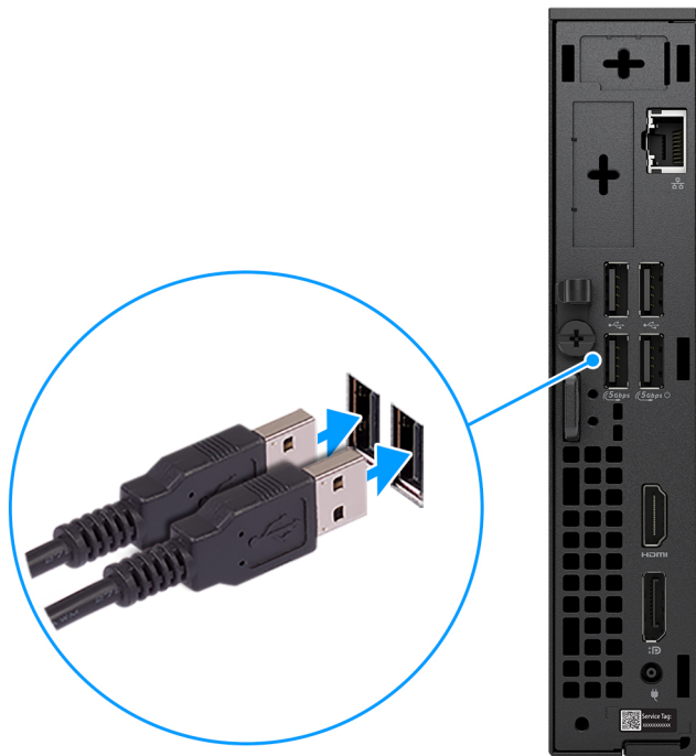
Figura 4. Collegamento di tastiera e mouse a Dell Pro con fattore di forma micro GCM1250
