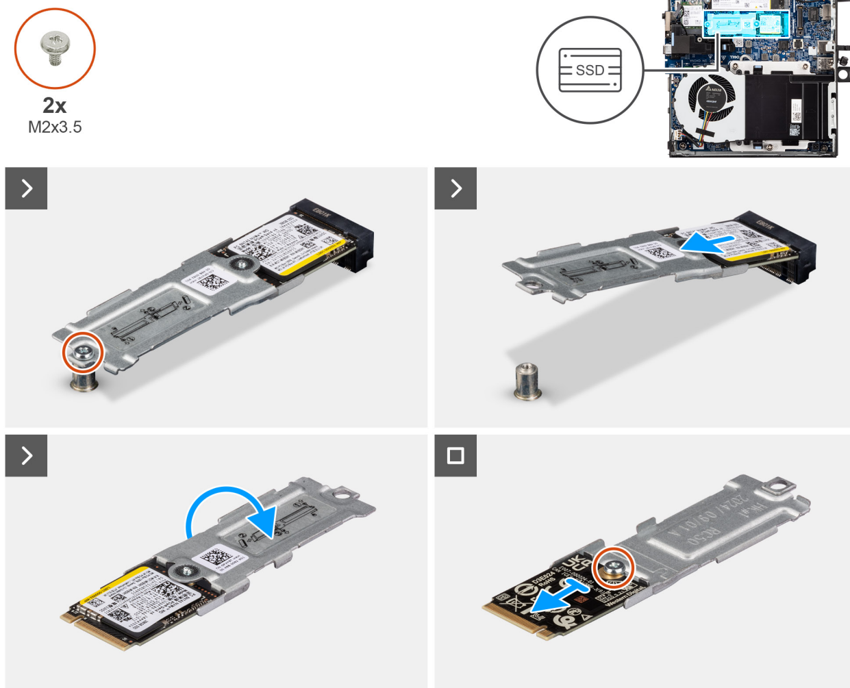
Figura 16. Rimozione dell'unità SSD 2230
