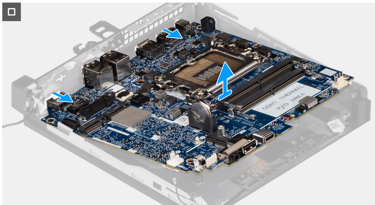
Figura 76. Rimozione della scheda di sistema
