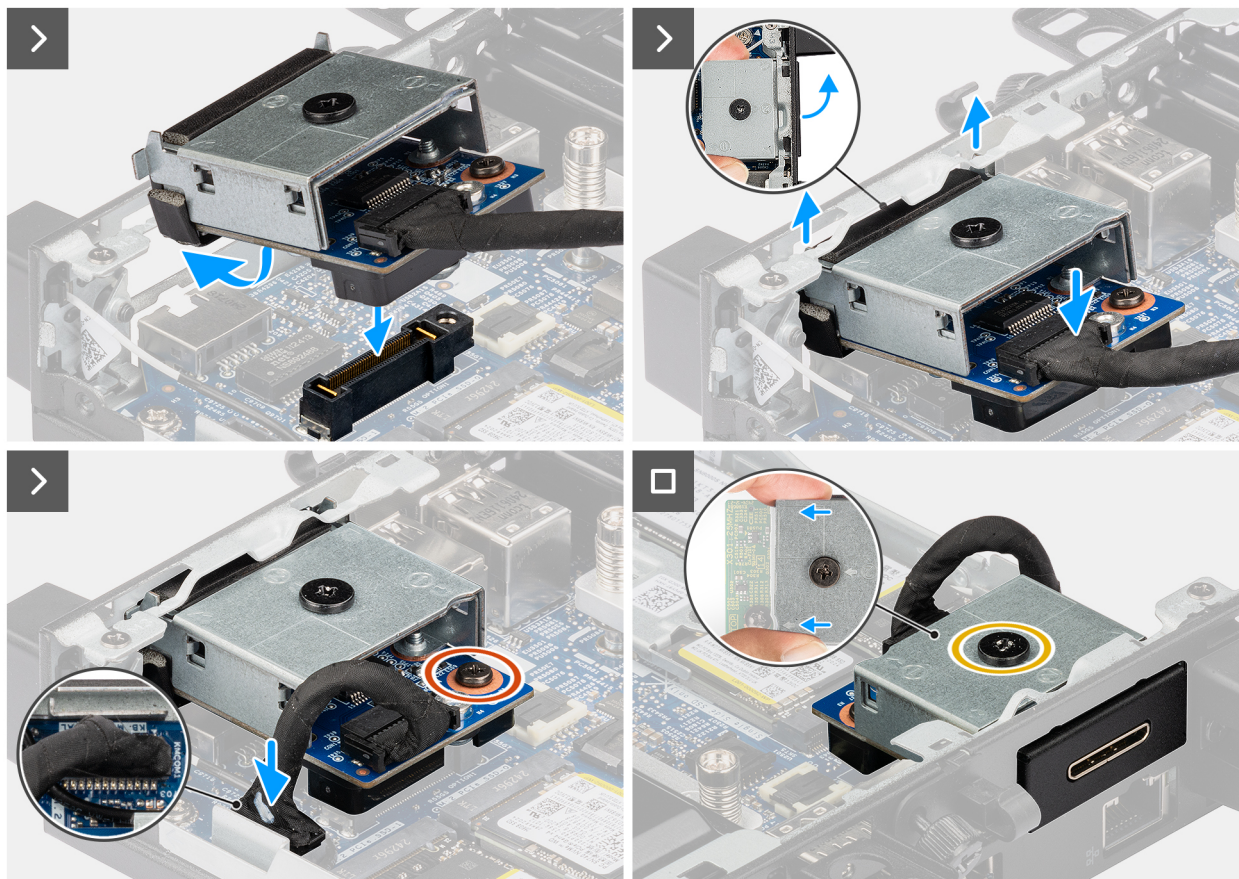
Figura 55. Installazione del modulo della porta PS2
