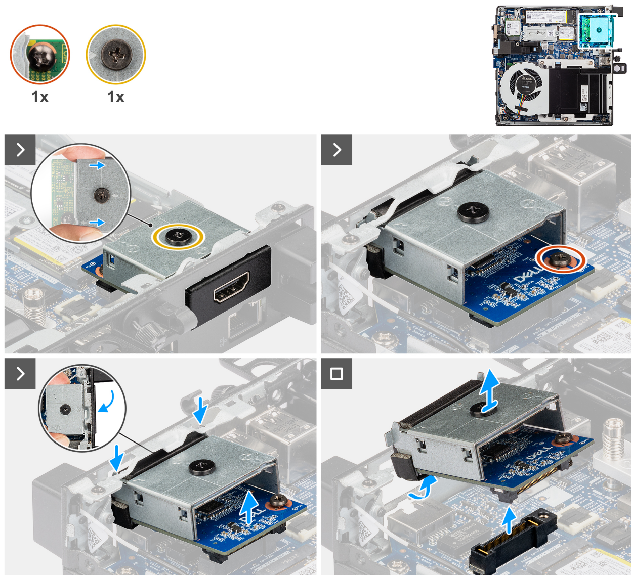
Figura 47. Rimozione del modulo della porta HDMI
