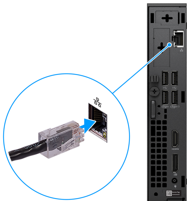
Figura 5. Collegare alla rete tramite un cavo
