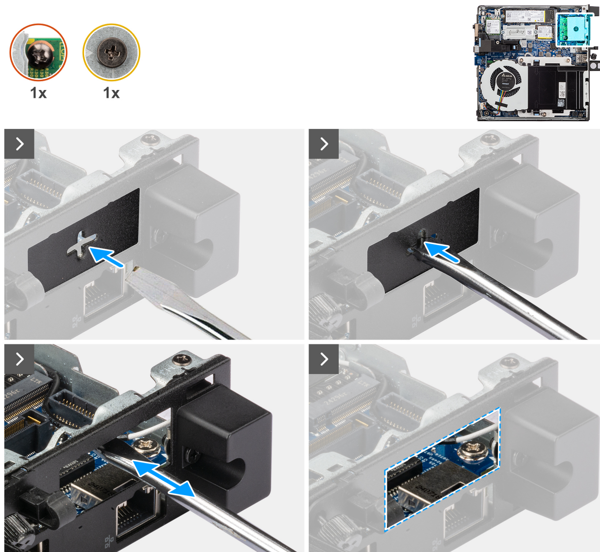
Figura 39. Installazione di un modulo a 2 porte USB 3.2 Gen 2
