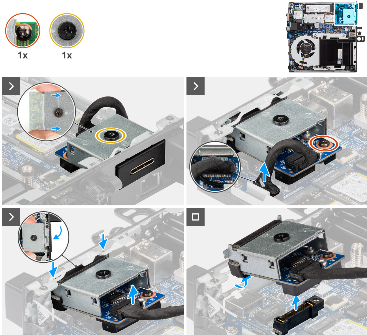
Figura 53. Rimozione del modulo della porta PS2
