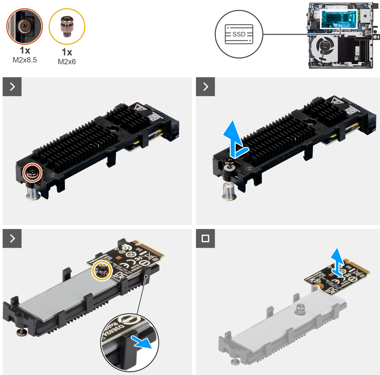
Figura 22. Rimozione dell'unità SSD M.2 2230 PCIe
