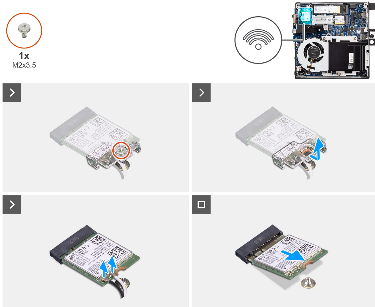
Figura 26. Rimozione della scheda wireless
