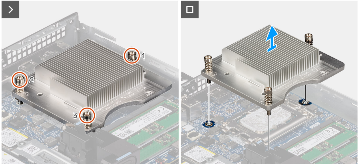
Figura 62. Rimozione del dissipatore di calore
