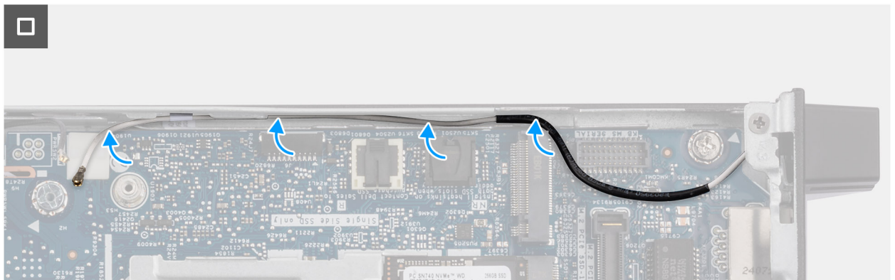
Figura 69. Installazione del modulo dell'antenna (cavo bianco)
