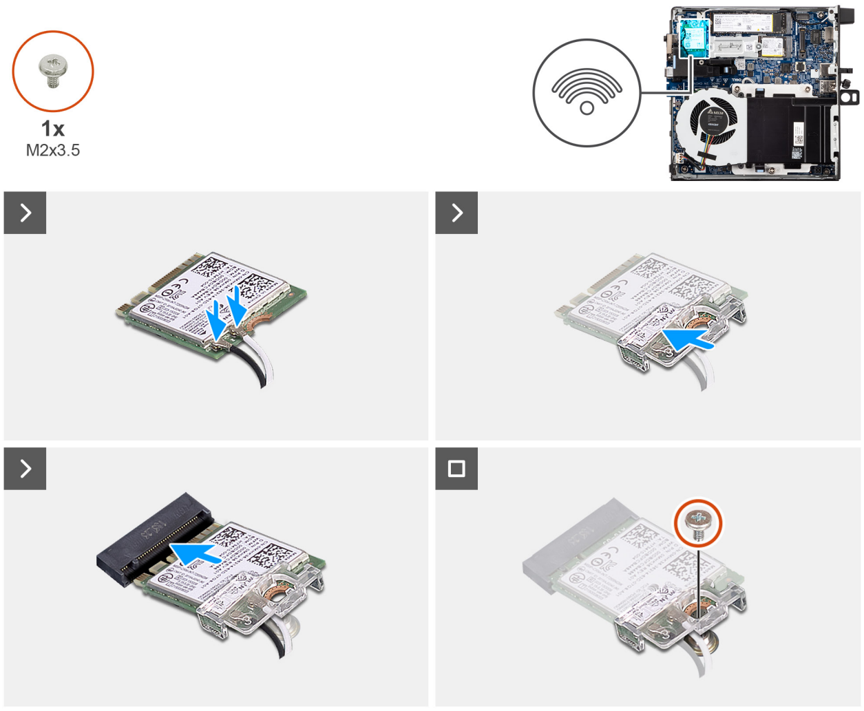
Figura 27. Installazione della scheda wireless
