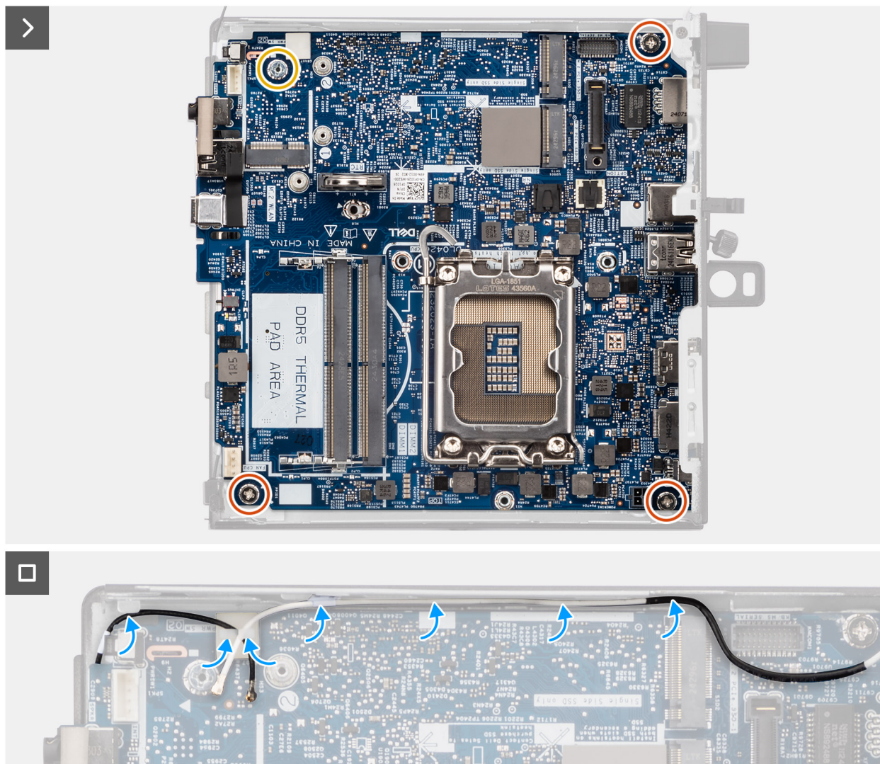
Figura 79. Installazione della scheda di sistema
