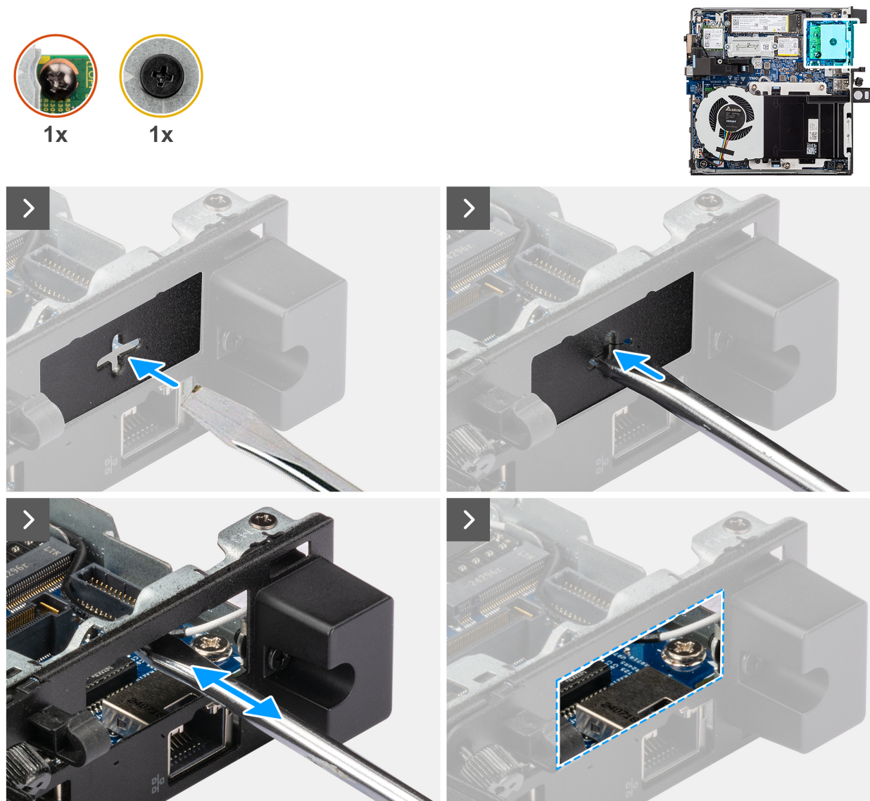
Figura 48. Installazione del modulo della porta HDMI
