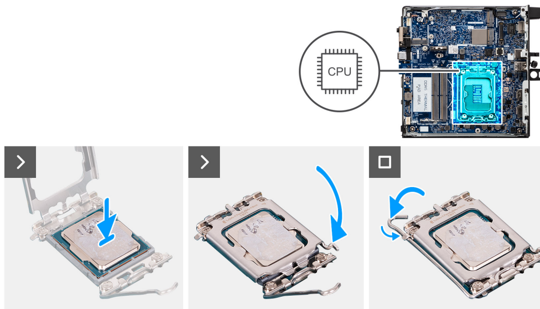
Figura 71. Installazione del processore
