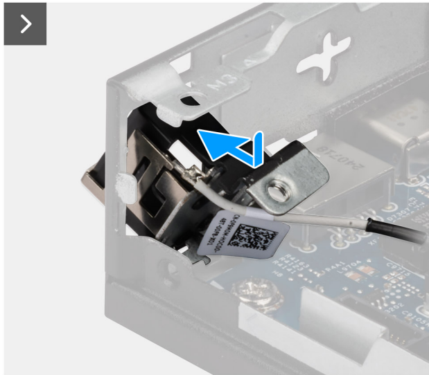
Figura 68. Installazione del modulo dell'antenna (cavo bianco)
