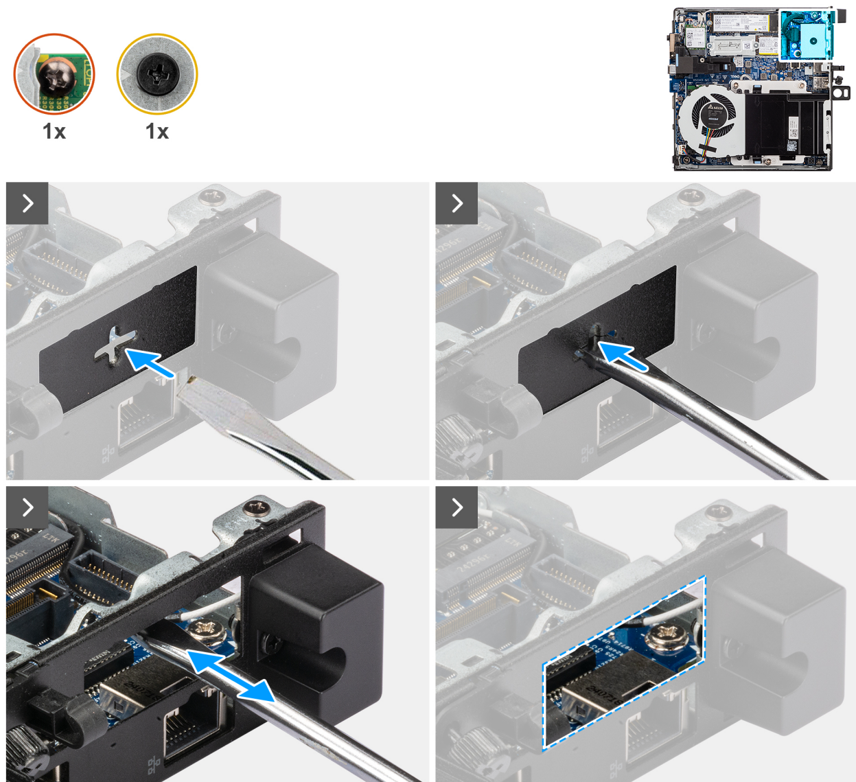
Figura 54. Installazione del modulo della porta PS2
