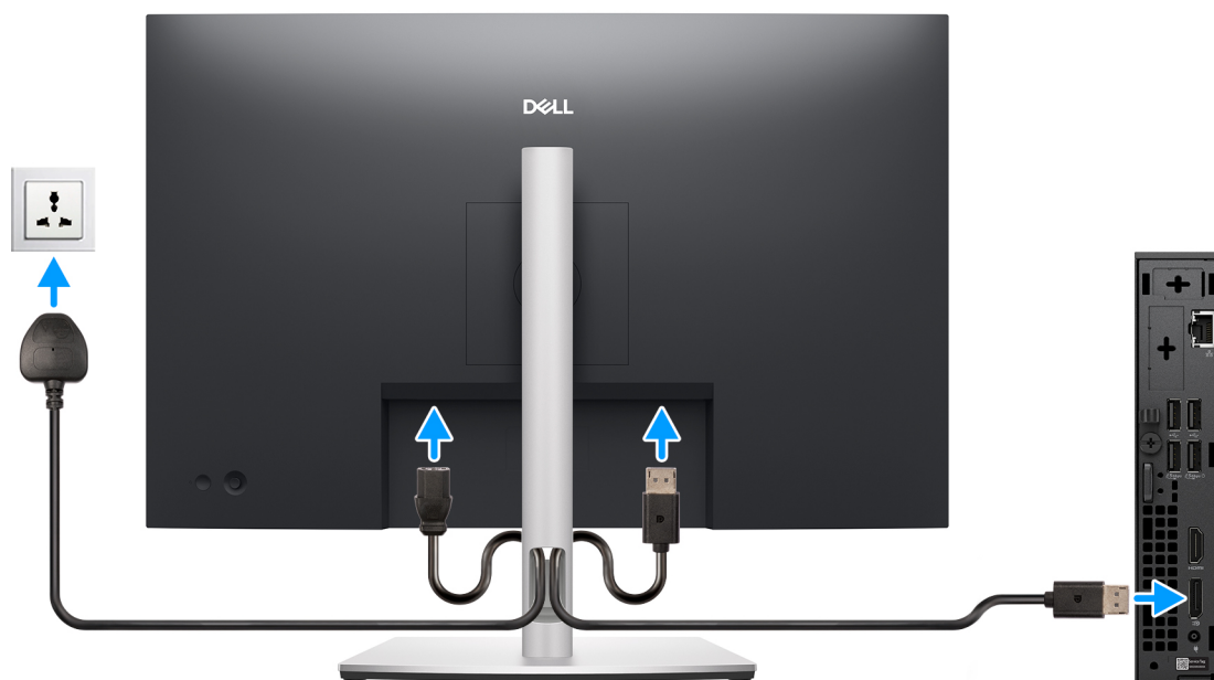
Figura 6. Collegare il display.
