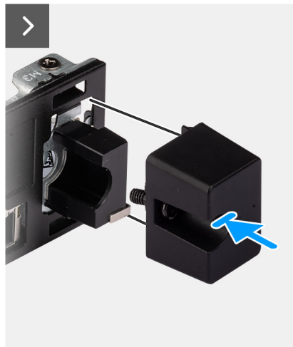
Figura 68. Installazione del modulo dell'antenna (cavo bianco)
