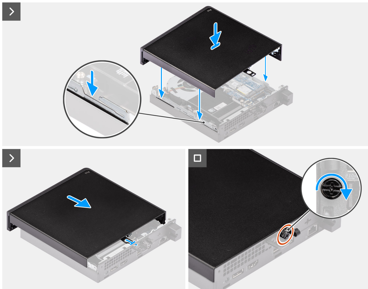
Figura 11. Installazione del coperchio laterale
