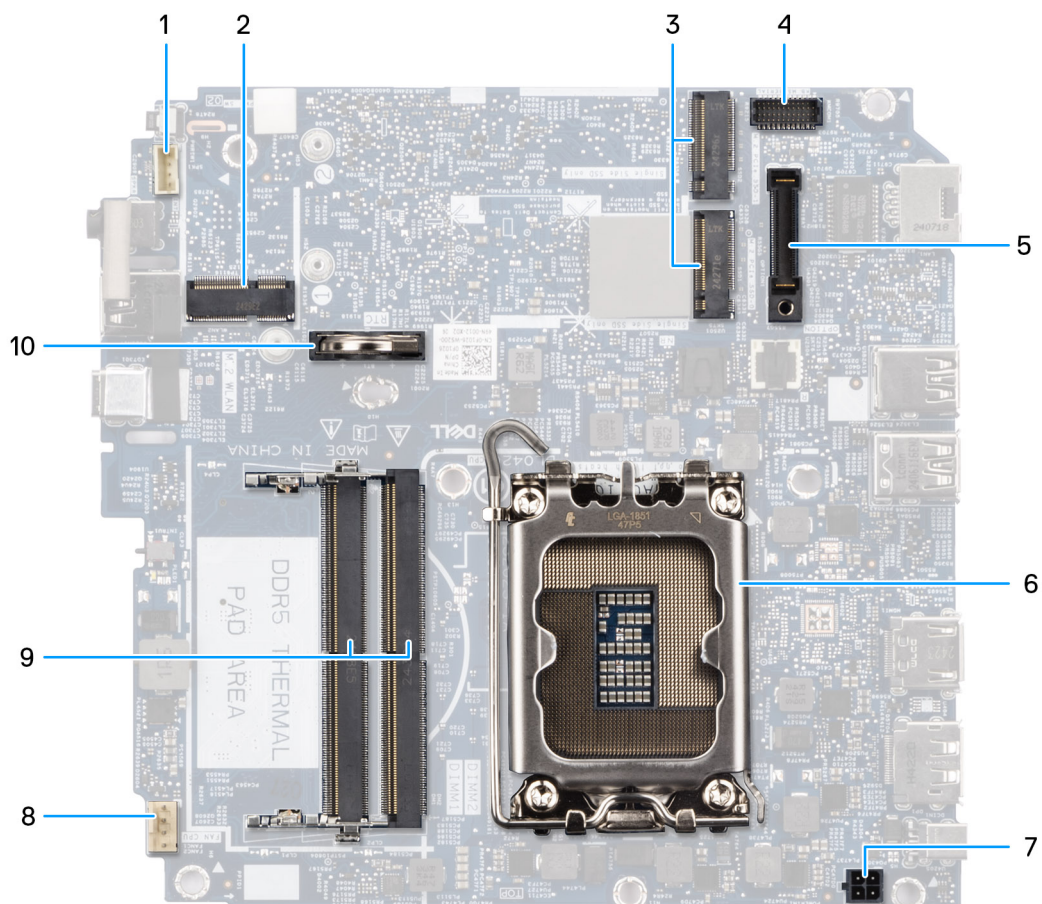
Figura 77. Connettori della scheda di sistema
