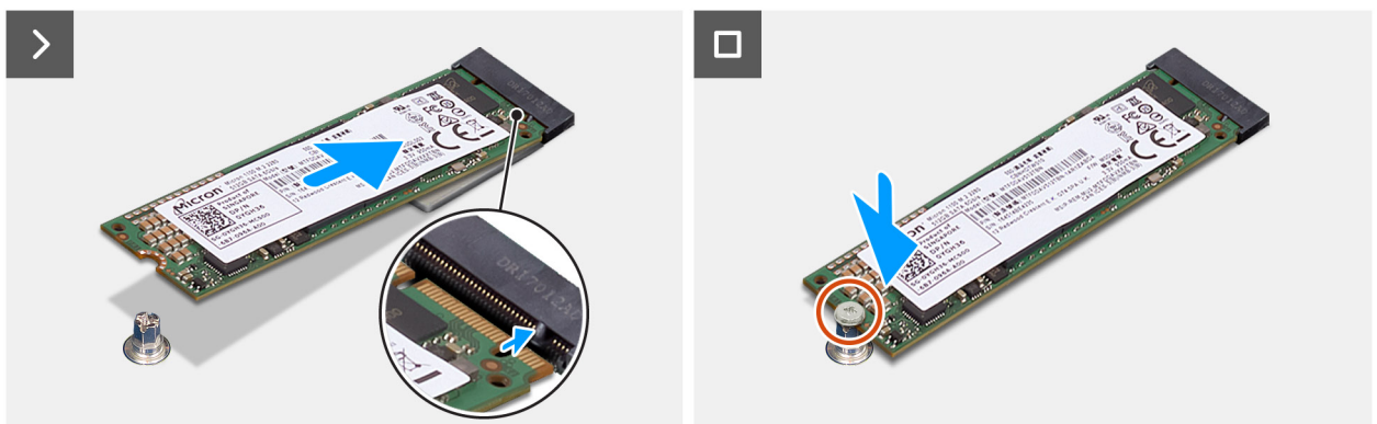
Figura 21. Installazione dell'unità SSD M.2 2280
