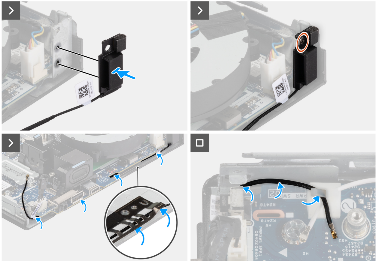
Figura 65. Installazione del modulo dell'antenna (cavo nero)
