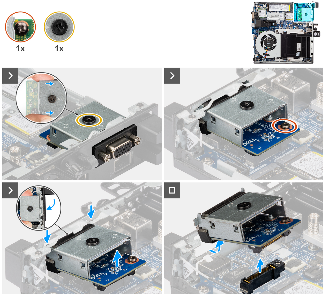
Figura 50. Rimozione del modulo della porta VGA
