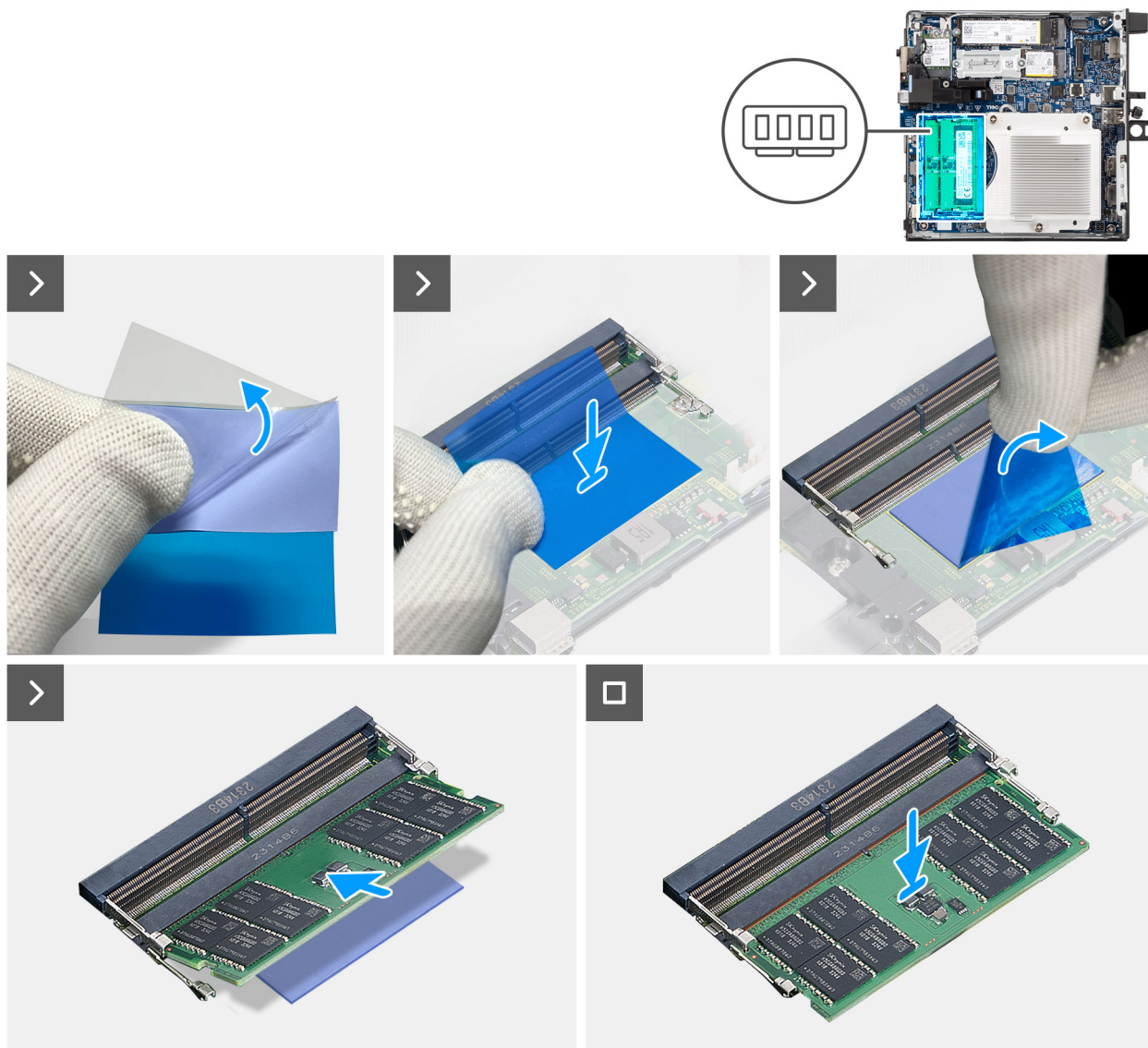
Figura 33. Installazione del modulo di memoria
