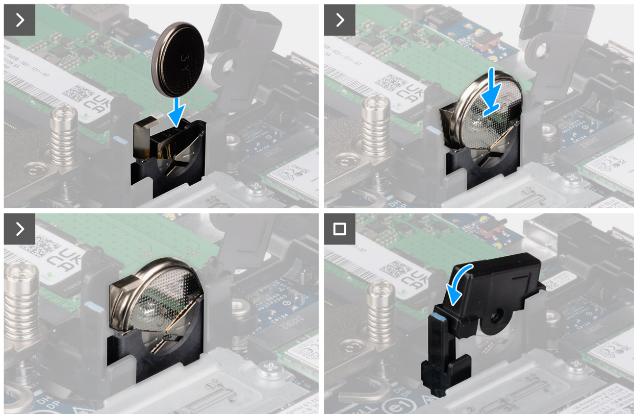
Figura 13. Installazione della batteria a bottone
