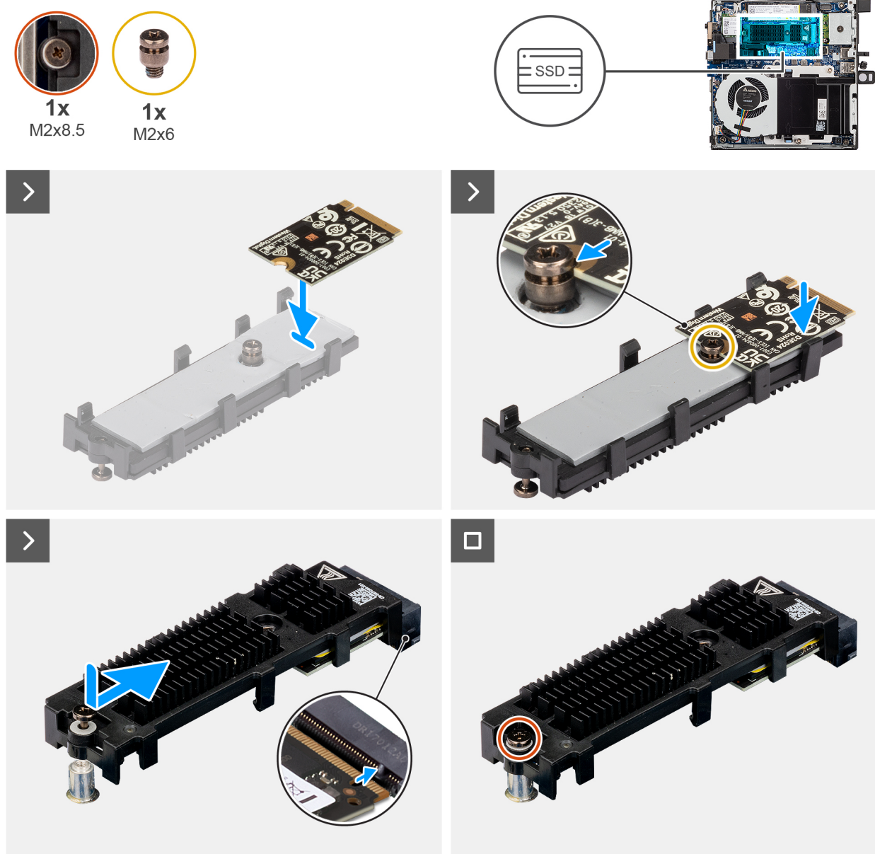
Figura 23. Installazione dell'unità SSD PCIe M.2 2230
