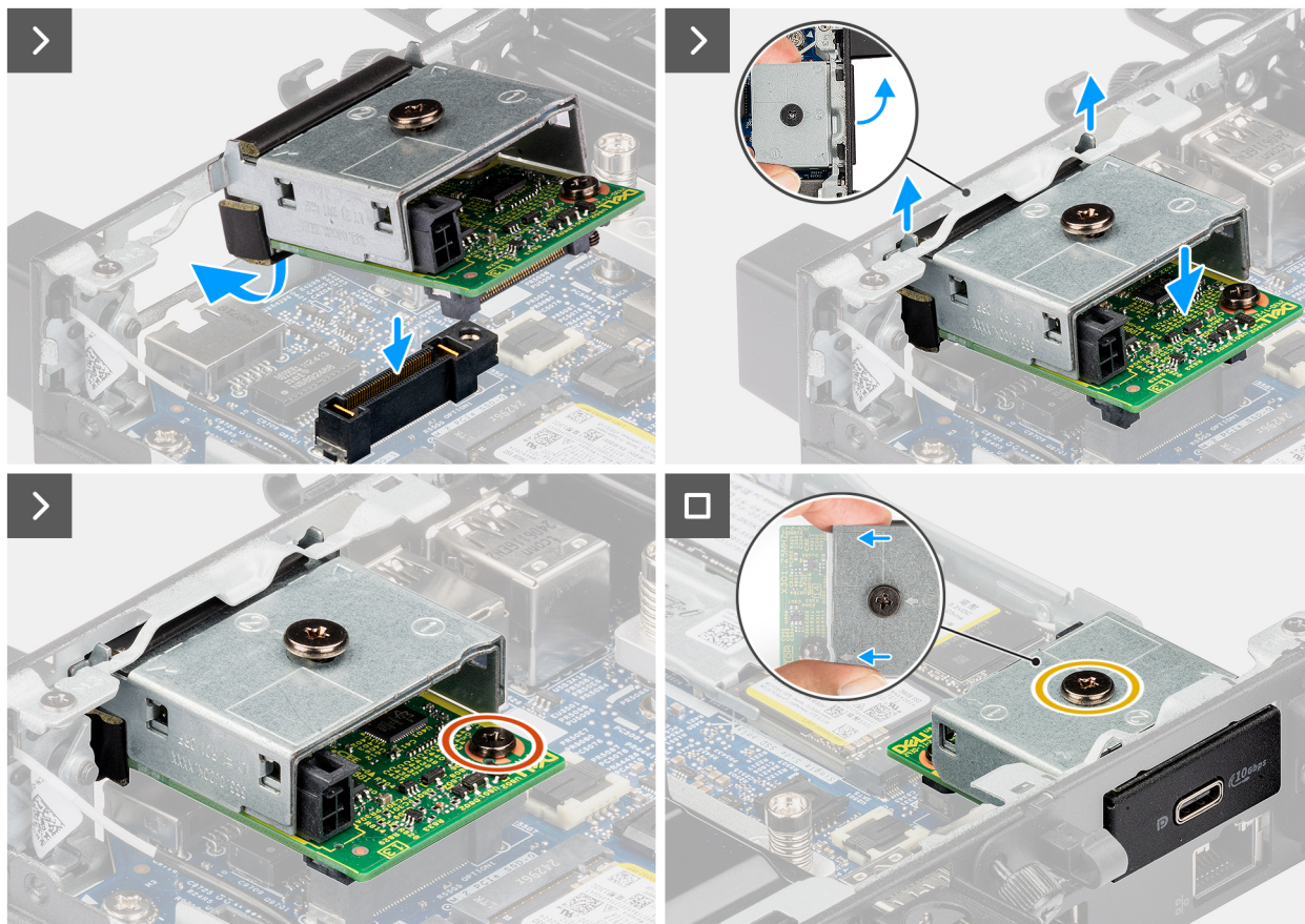
Figura 43. Installazione del modulo della porta USB Type-C
