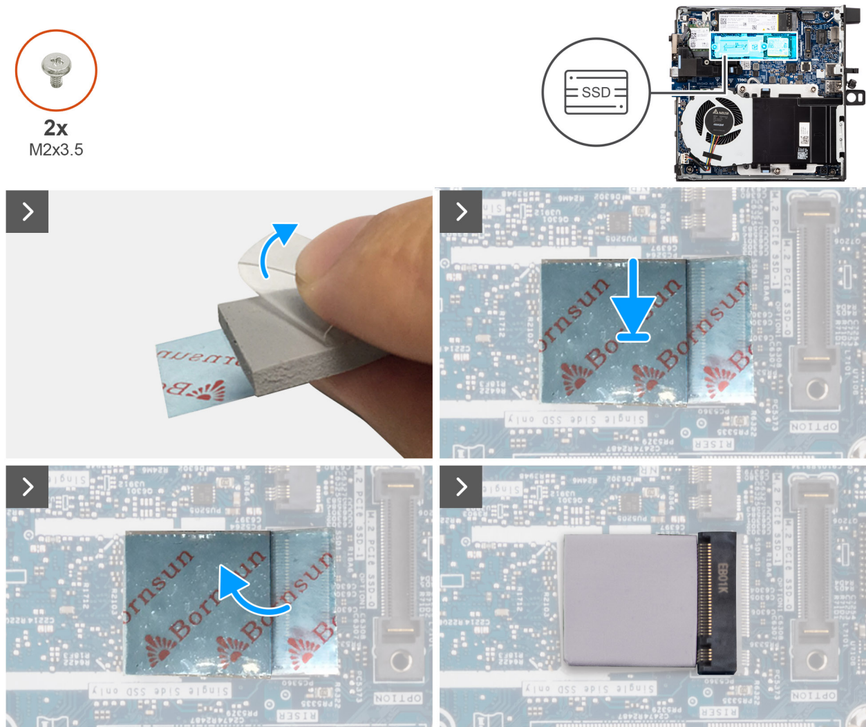
Figura 17. Installazione dell'unità SSD 2230
