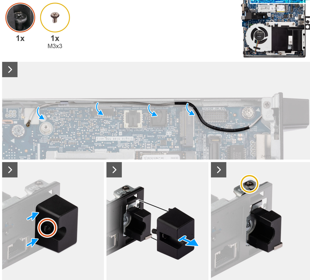
Figura 66. Rimozione del modulo dell'antenna (cavo bianco)
