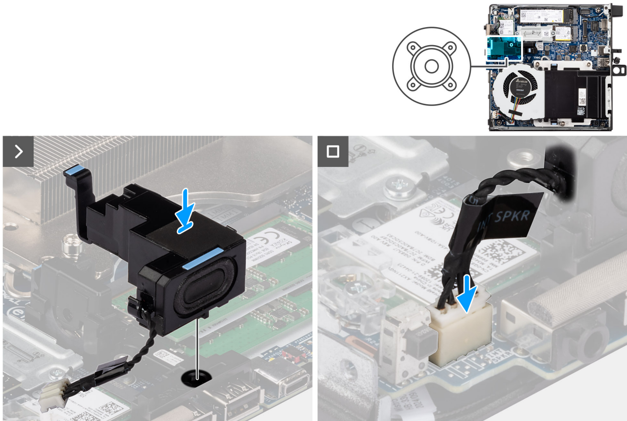
Figura 15. Installazione dell'altoparlante
