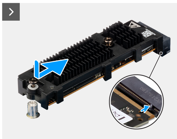
Figura 25. Installazione dell'unità SSD PCIe M.2 2280
