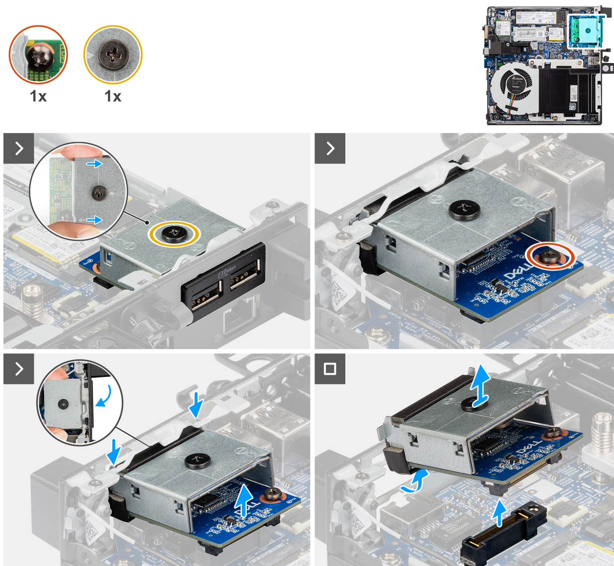
Figura 38. Rimozione del modulo a 2 porte USB 3.2 Gen 2
