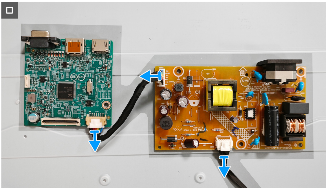
Figura 22. Rimozione della scheda di sistema e della scheda di alimentazione
