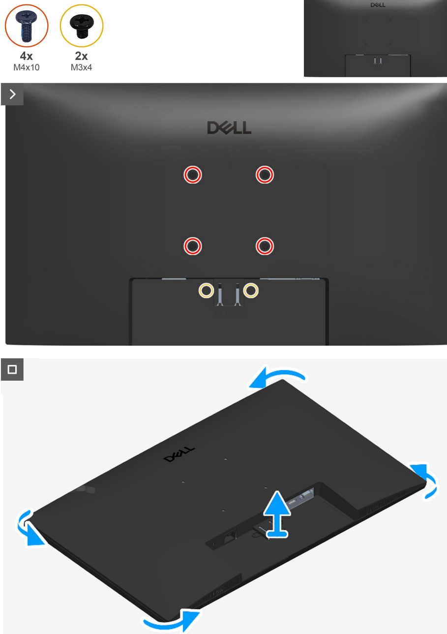
Figura 11. Rimozione del coperchio posteriore
