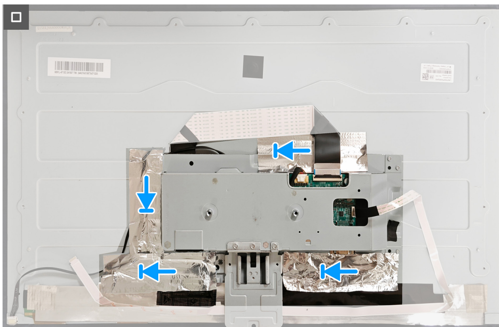
Figura 18. Installazione della schermatura metallica
