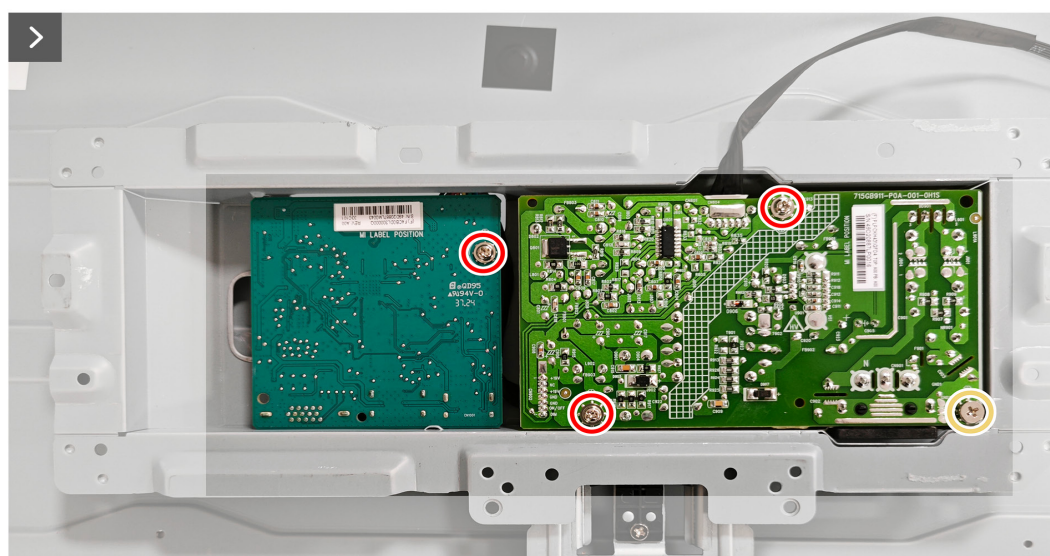
Figura 21. Rimozione della scheda di sistema e della scheda di alimentazione
