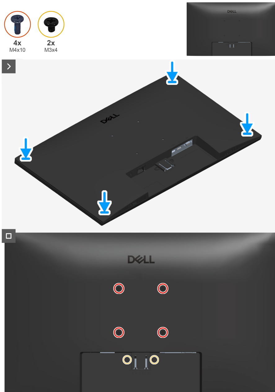
Figura 12. Installazione del coperchio posteriore
