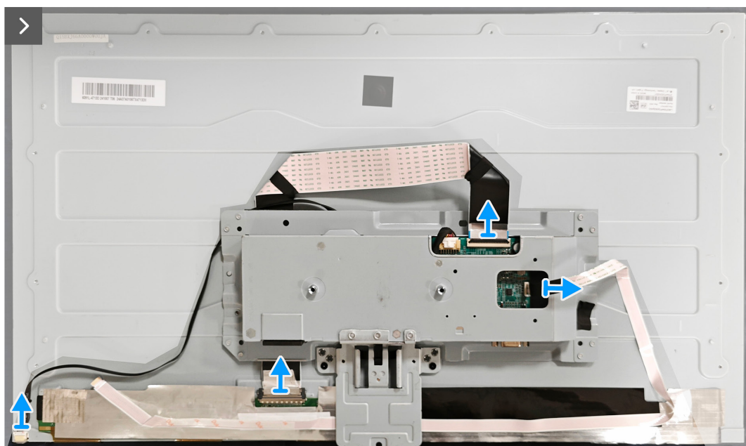
Figura 15. Rimozione della schermatura metallica
