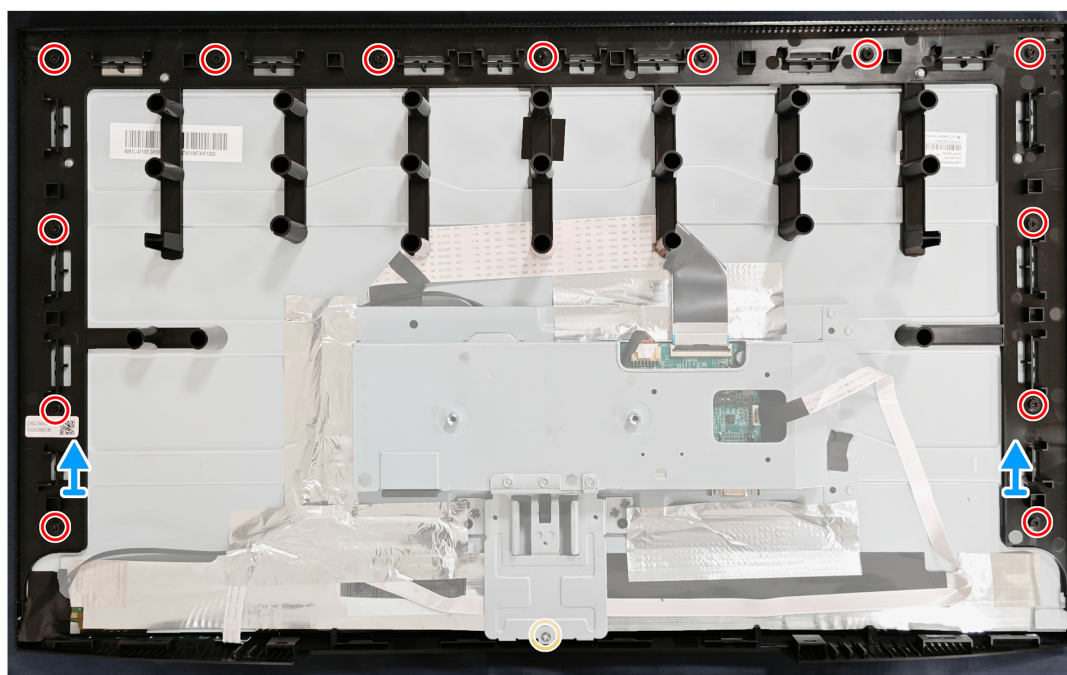
Figura 13. Rimozione della struttura centrale
