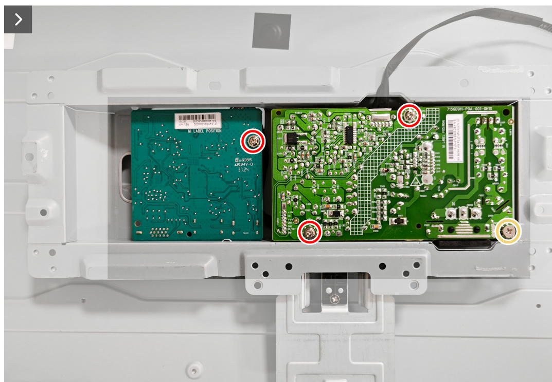
Figura 23. Installazione della scheda di sistema e della scheda di alimentazione
