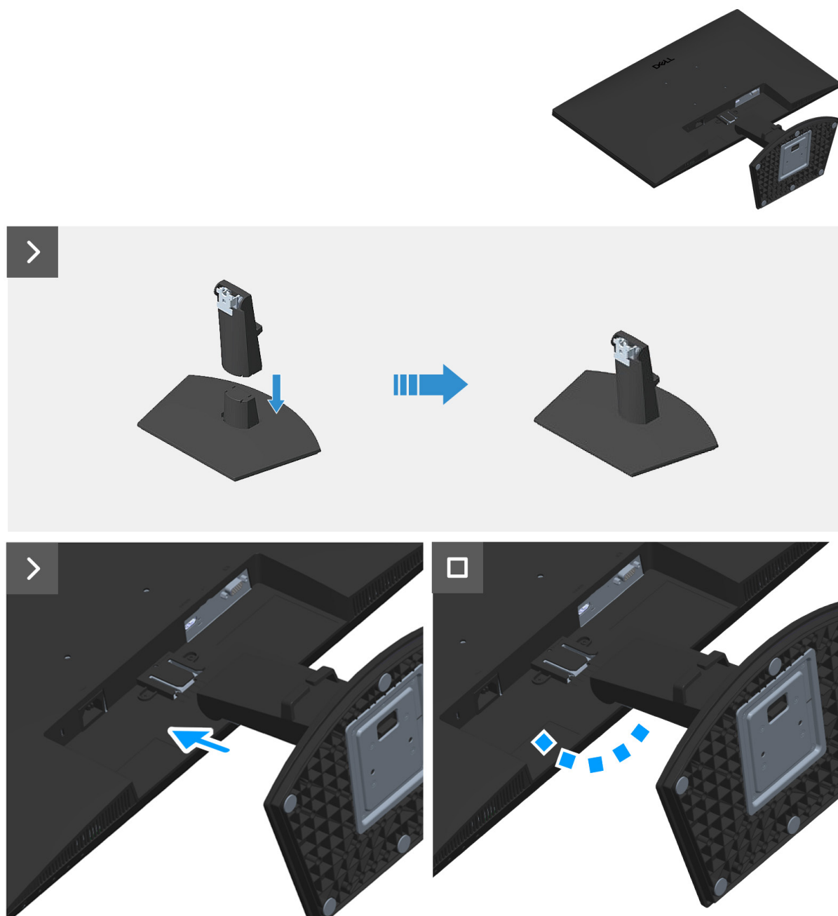
Figura 10. Installazione del supporto
