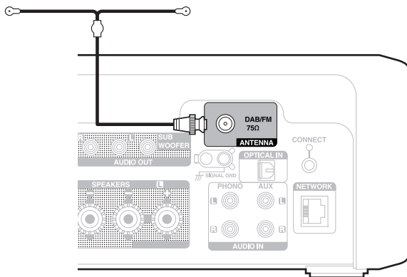
DAB-/UKW-Zimmerantenne (im Lieferumfang enthalten)
